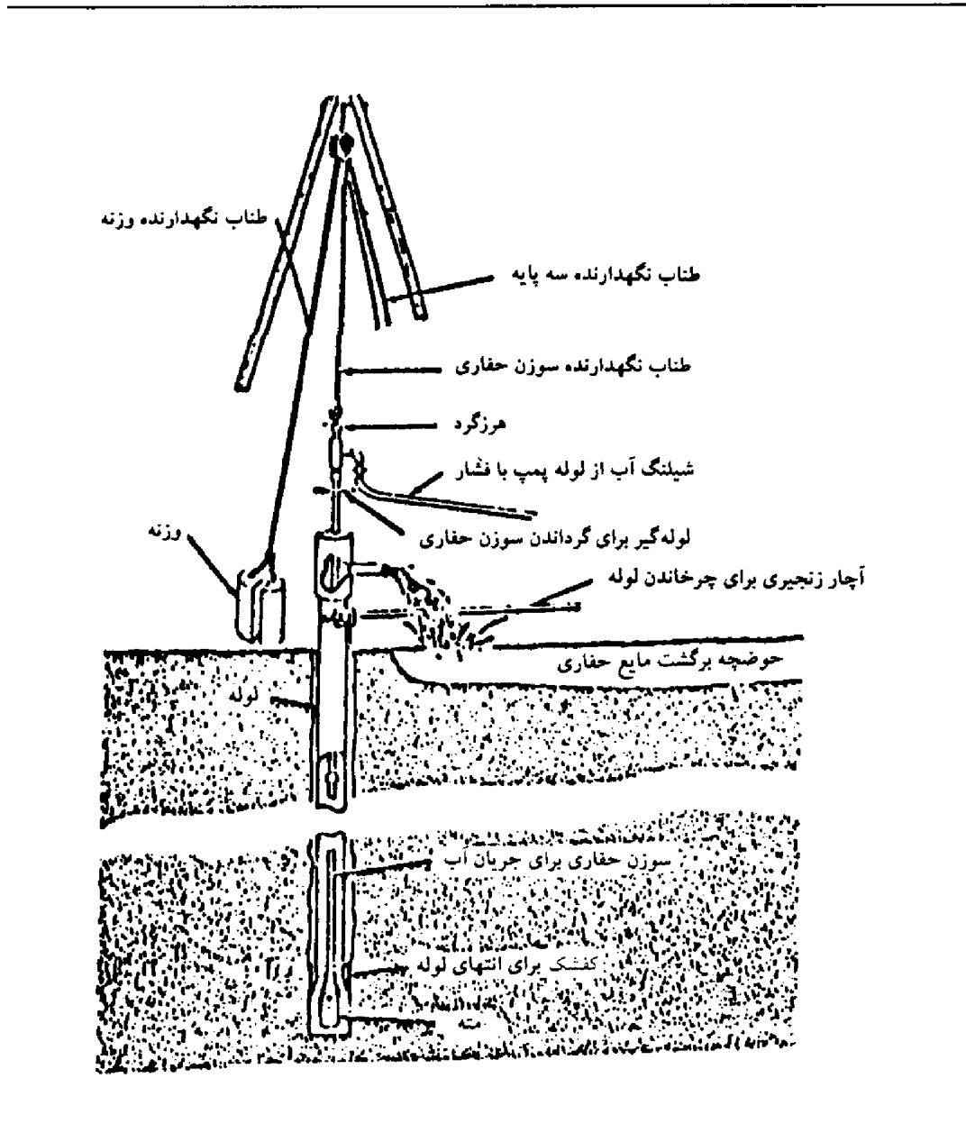
شکل ۱۴- حفاری به روش فشار آب
