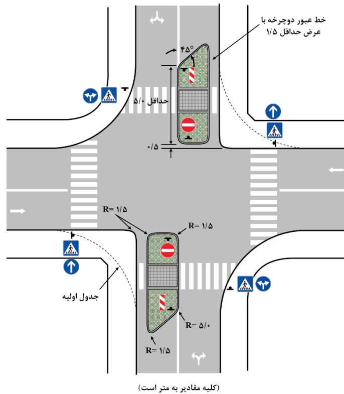
شکل ۷-۲- مشخصات هندسی و علائم انسداد جریان ورودی
