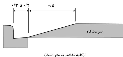
شکل ۳-۳- فاصله عرضی سرعت کاه از جدول آبرو
