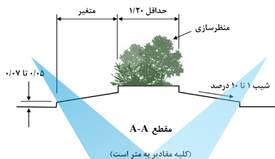
شکل ۴-۱۲- مشخصات هندسی و علائم میدانچه
