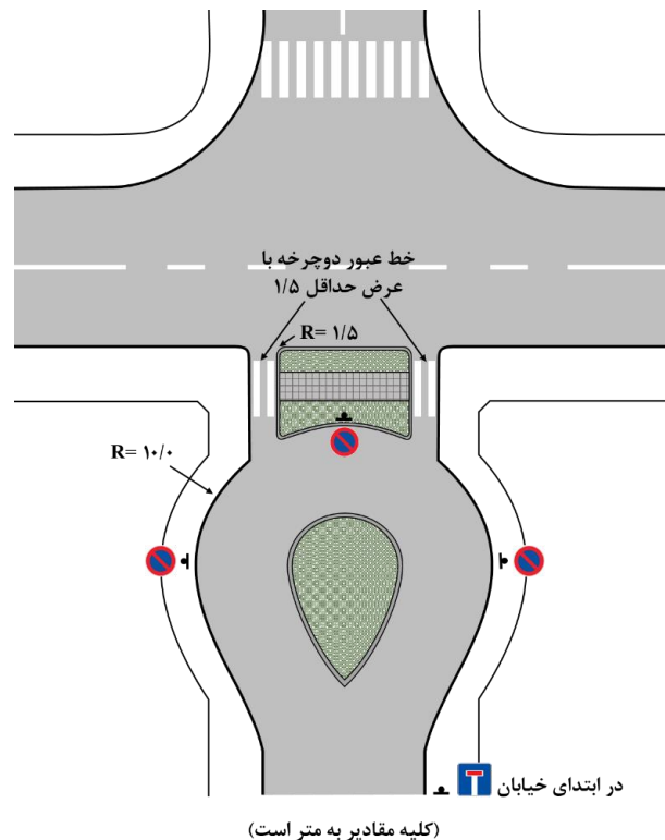
شکل ۵-۷- مشخصات هندسی و علائم انسداد کامل
