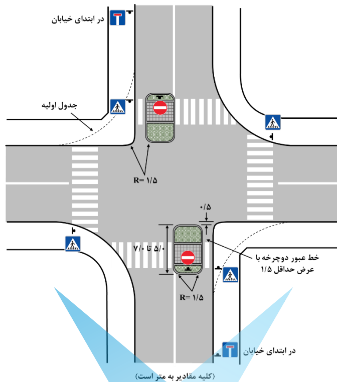
شکل ۷-۳- مشخصات هندسی و علائم انسداد جریان خروجی
