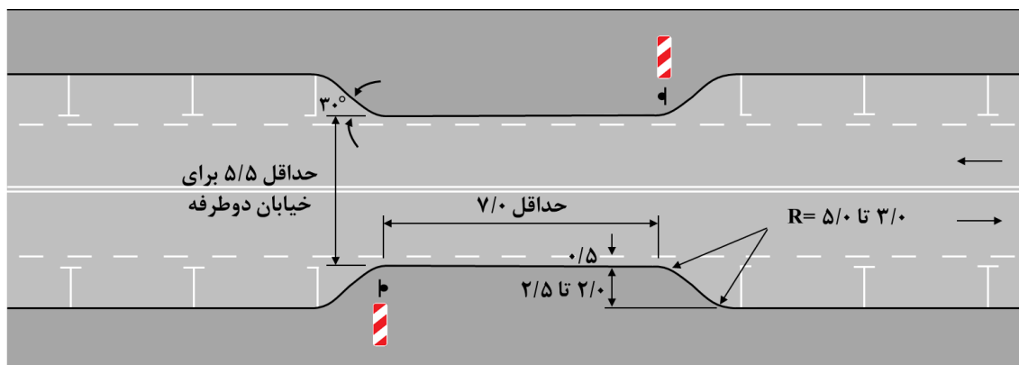
(کلیه مقادیر به متر است)
