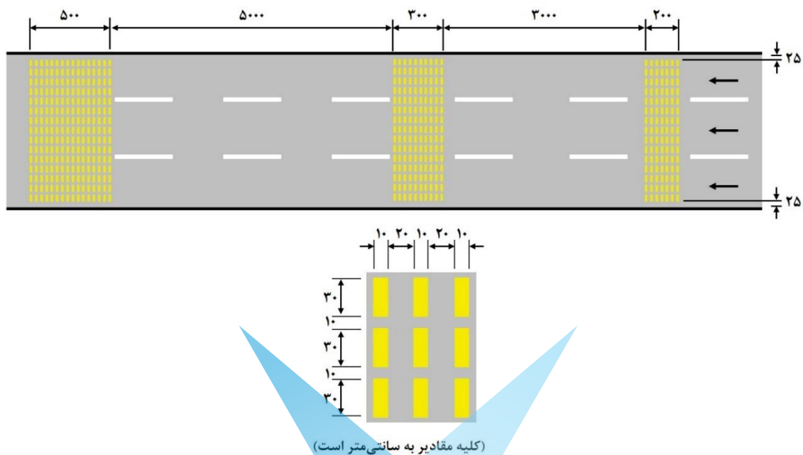
شکل ۹-۵- مشخصات هندسی نوار لرزاننده عرضی در راه‌های با سرعت مجاز بیشتر از ۶۰ کیلومتر بر ساعت
