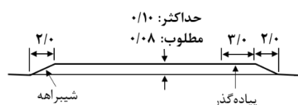
مقطع A-A
