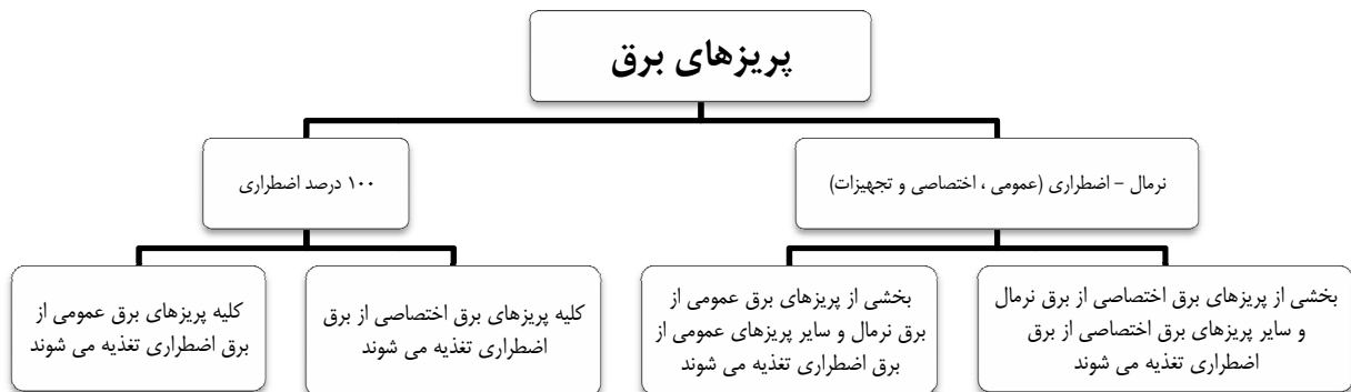
شکل ۵-۴- پریزهای مصارف عمومی
