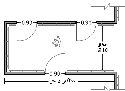
نقشه ۲-۳۹- راهرو با عرض حداقل ۲/۱ متر - مقیاس ۱:۱۰۰
