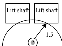
شکل ۵-۱۲- فاصله ی مجاز نصب هر دتکتور با درها
