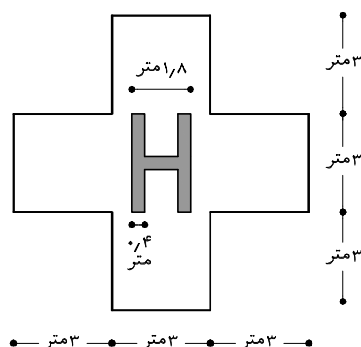
نقشه ۲-۱۸- تعبیه علامت \oplus و H در مرکز هلی‌پد
