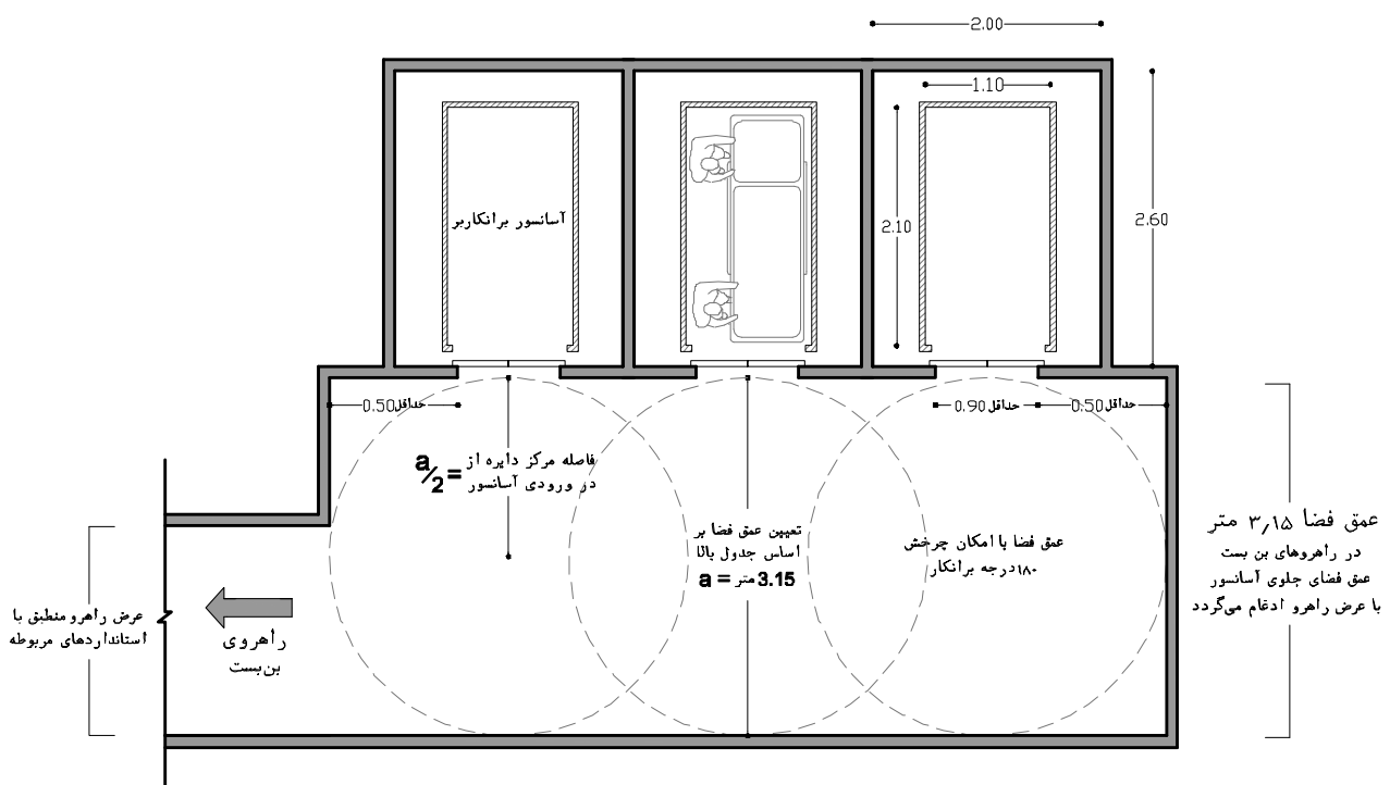
نقشه ۲-۵۰- نحوه تعیین ابعاد جلوی آسانسورها در راهروهای بن بست
