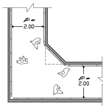
نقشه ۲-۴۲- ایجاد تمهیداتی همچون ایجاد شکستگی در کنج - مقیاس ۱:۱۰۰
