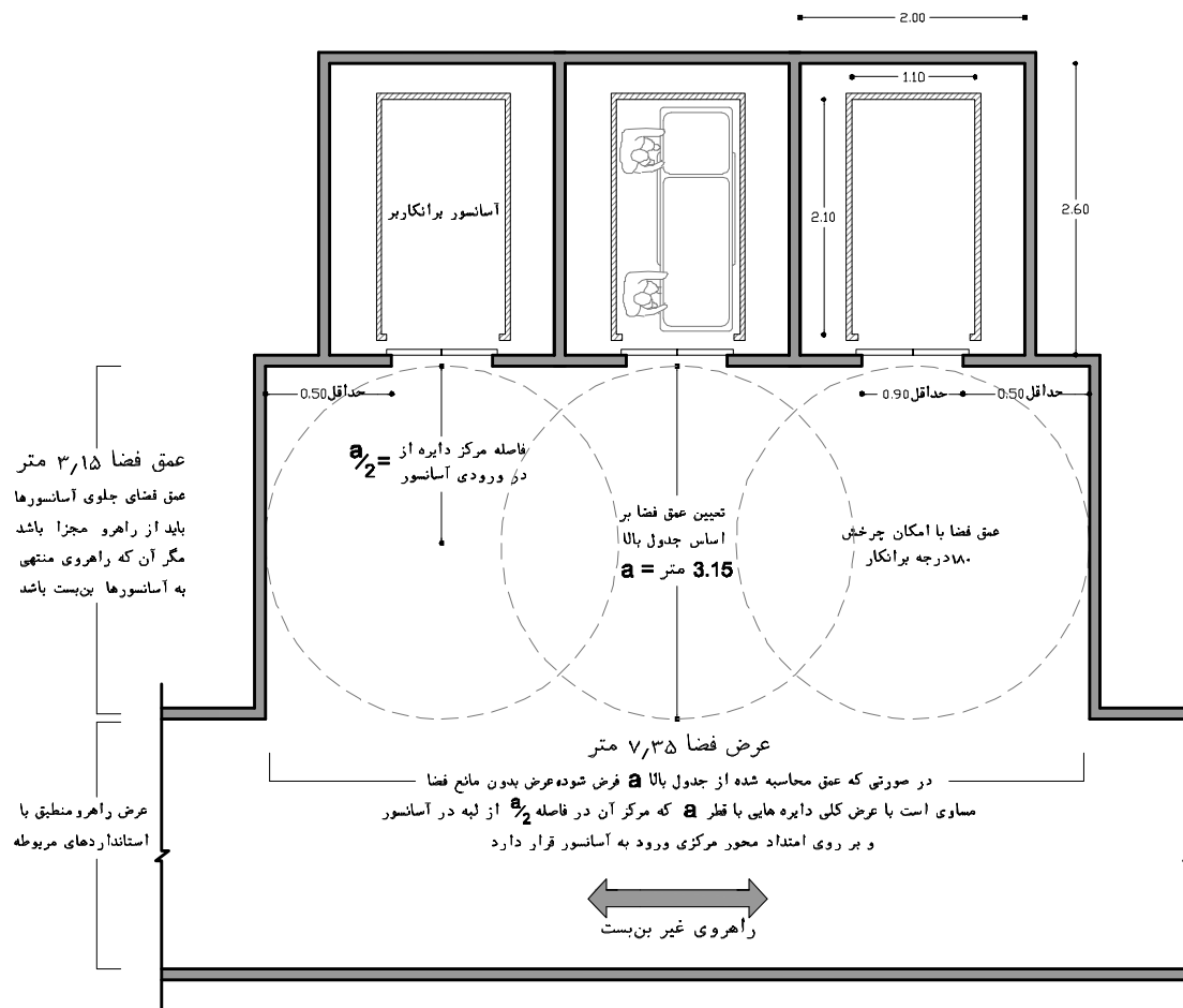
نقشه ۲-۴۹- نحوه تعیین ابعاد جلوی آسانسورها در راهروهای غیر بن بست (بن باز)
