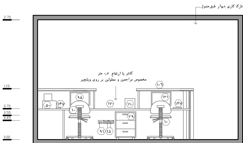
نقشه ۲-۳- نما ۱ - مقیاس ۱:۵۰
