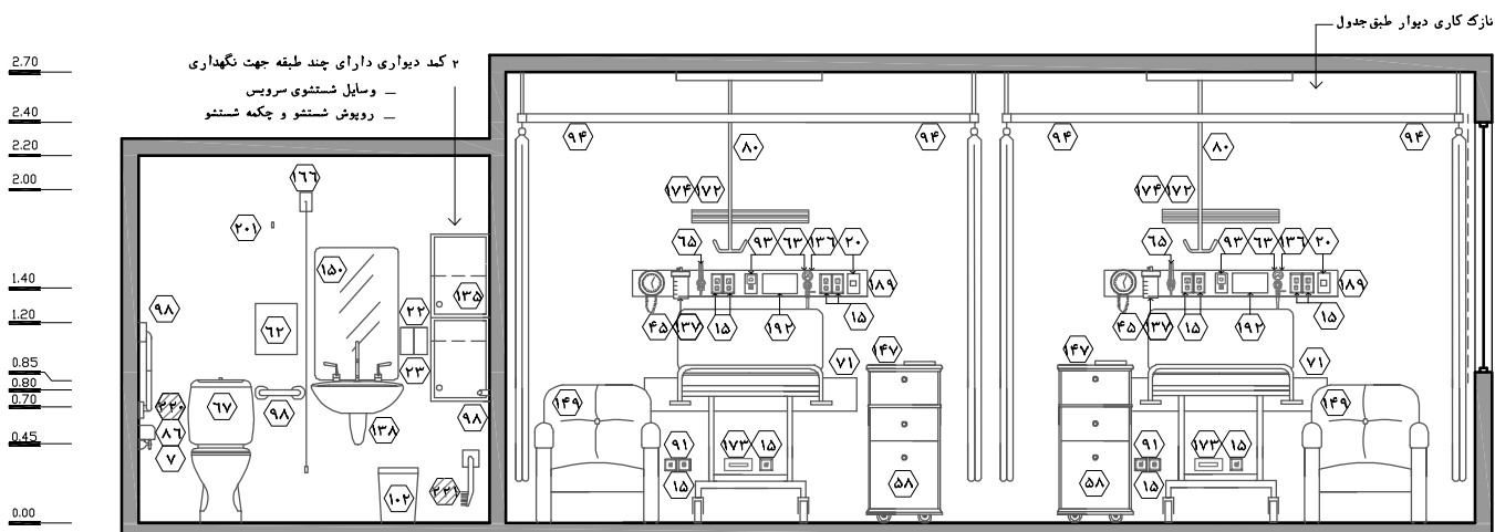
نقشه ۵-۱۵ - نما ۵ - مقیاس ۱:۵۰
