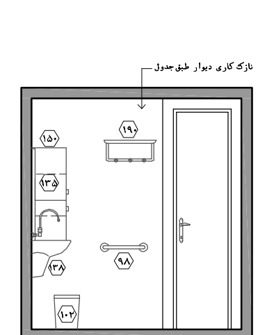
نقشه ۵-۲ - نما ۴ - مقیاس ۱:۵۰
