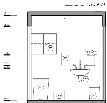
نقشه ۲-۲۵-۶ - نما ۶ - مقیاس ۱:۵۰
