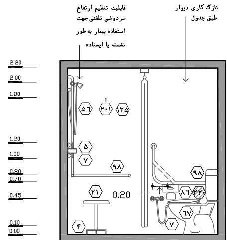
نقشه ۳-۱۳ - نما ۳ - مقیاس ۱:۵۰
