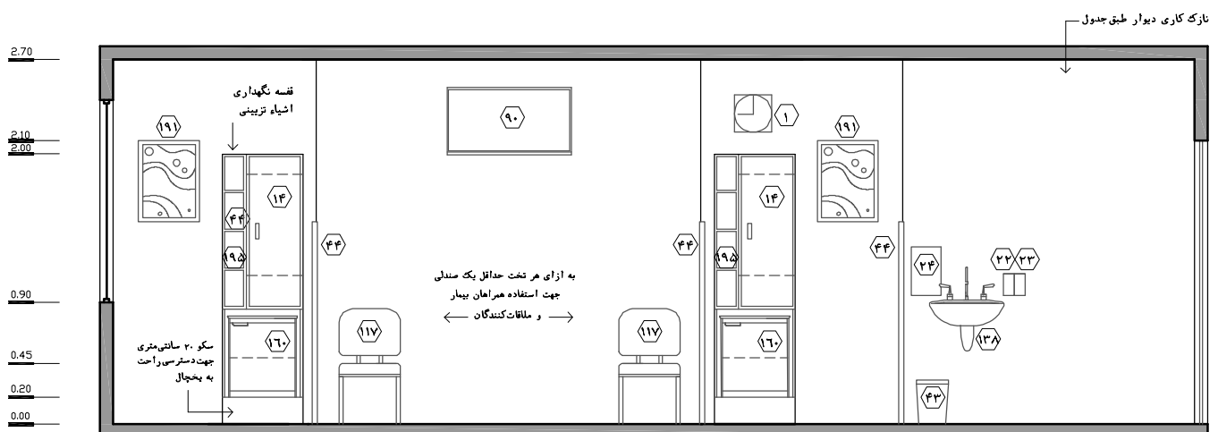
نقشه ۶-۱۶ - نما ۶ - مقیاس ۱:۵۰
