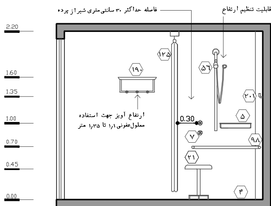
نقشه ۲-۲۰-۱ - نما ۱ - مقیاس ۱:۵۰
