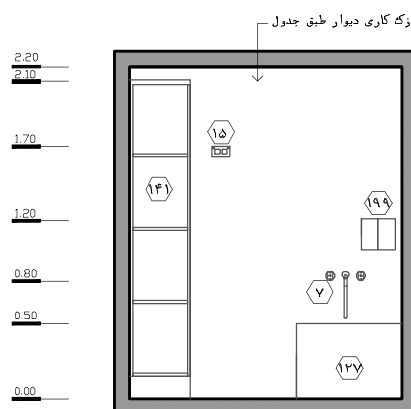
نقشه ۳-۷۱- نما ۳ - مقیاس ۱:۵۰
