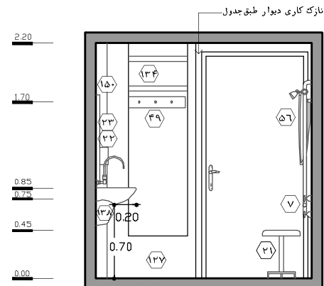
نقشه ۲-۲۳-۴ - نما ۴ - مقیاس ۱:۵۰
