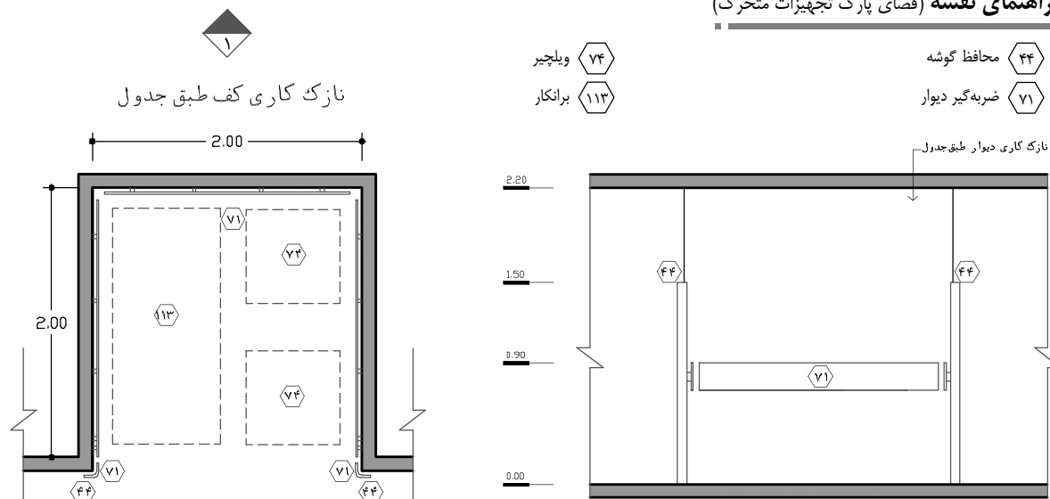
نقشه ۲-۸۳- پلان فضای پارک تجهیزات متحرک - مقیاس ۱:۵۰
