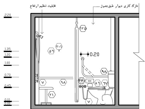
نقشه ۲-۲۱-۲ - نما ۲ - مقیاس ۱:۵۰
