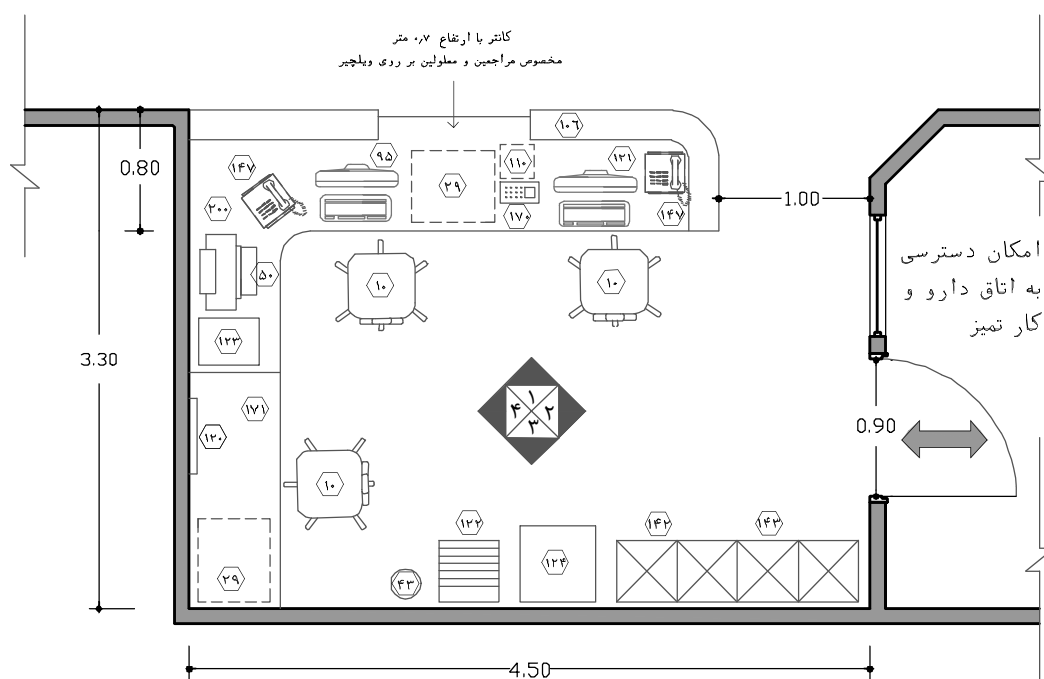
نقشه ۲-۳- پلان ایستگاه پرستاری - مقیاس ۱:۵۰
