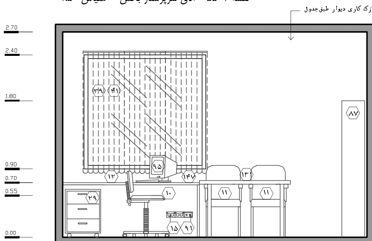
نقشه ۲-۵۵ - اتاق سرپرستار بخش - مقیاس ۱:۵۰
