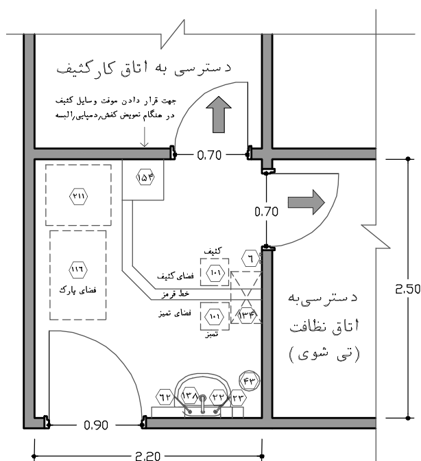
نقشه ۲-۵۷- پلان پیش‌ورودی اتاق کار کثیف - مقیاس ۱:۵۰
