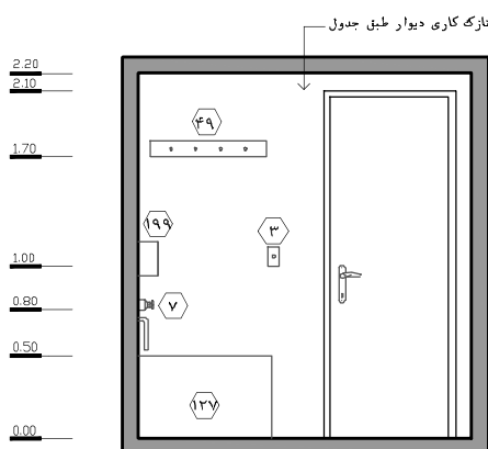
نقشه ۱-۶۹- نما ۱ - مقیاس ۱:۵۰
