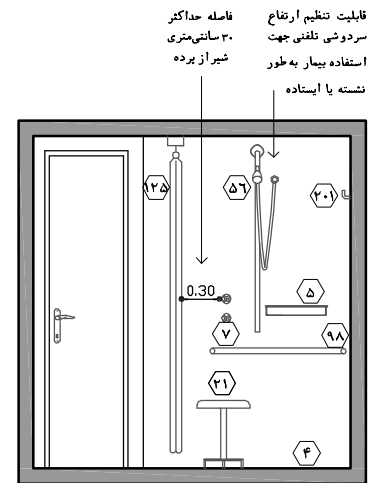
نقشه ۳-۲ - نما ۲ - مقیاس ۱:۵۰
