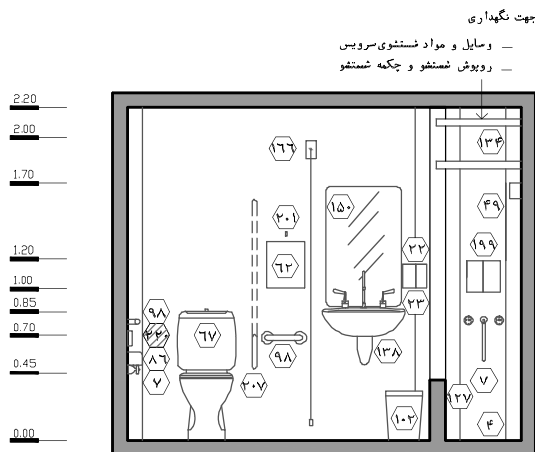
نقشه ۲-۲۲-۳ - نما ۳ - مقیاس ۱:۵۰
