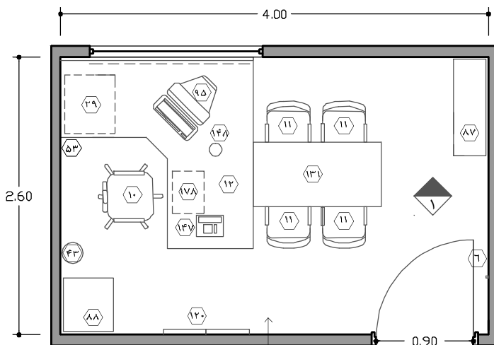
نقشه ۲-۵۵ - اتاق سرپرستار بخش - مقیاس ۱:۵۰
