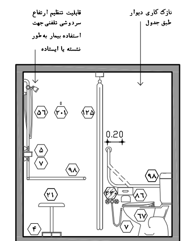
نقشه ۷-۲ - نما ۶ - مقیاس ۱:۵۰
