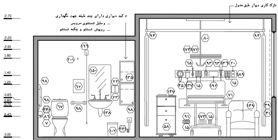
نقشه ۴-۲ - نما ۳ - مقیاس ۱:۵۰
