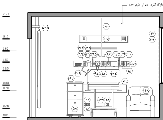
نقشه ۲-۲۴-۵ - نما ۵ - مقیاس ۱:۵۰
