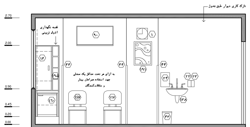
نقشه ۶-۲ - نما ۵ - مقیاس ۱:۵۰
