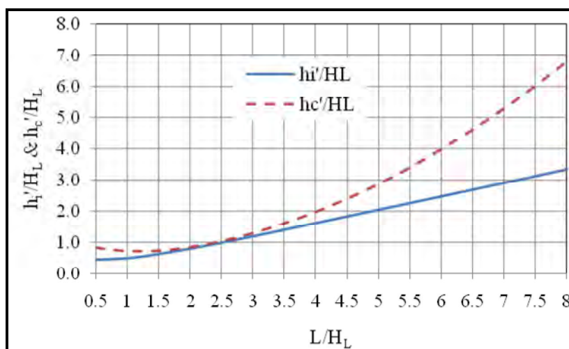
شکل ۹-۳- ضرایب h'_i / H_L و h'_c / H_L برای مخازن مستطیلی با در نظر گرفتن فشار نامتوازن وارد بر پی (IBP) [۴۹]
