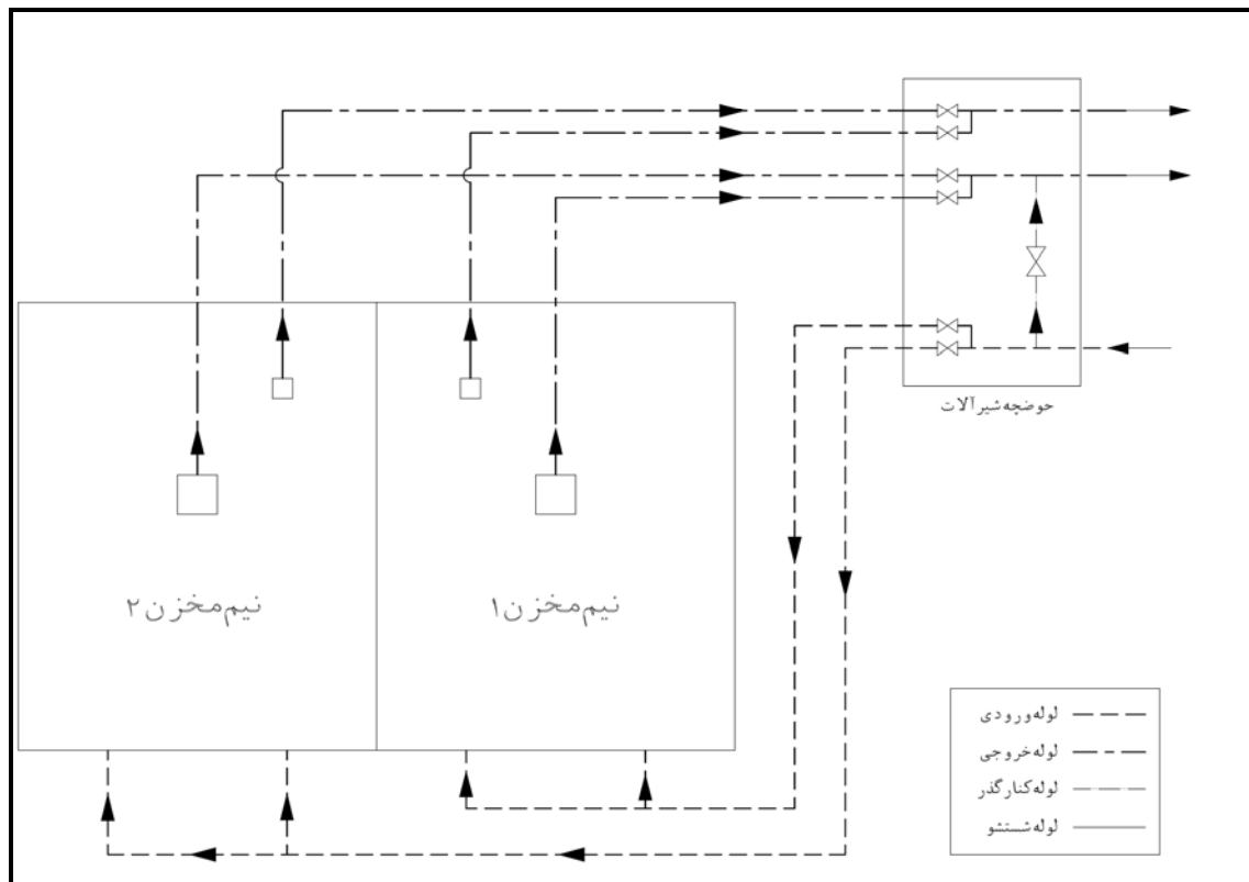
شکل ۶-۴- شکل شماتیک تجميع حوضچه‌های شیرآلات لوله‌های ورودی، خروجی و شستشوی مخزن (این شکل به عنوان نمونه و تنها جهت راهنمایی ارائه شده است)
