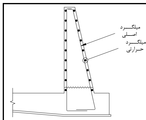
شکل ۴-۱۰- محل قرارگیری میلگردهای حرارتی افقی
