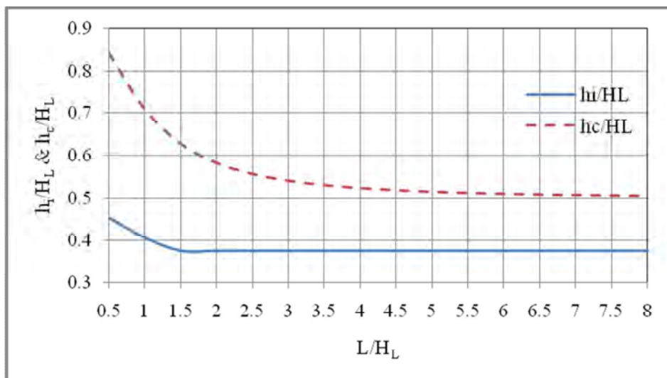
شکل ۳-۷- ضرایب h_i / H_L و h_c / H_L برای مخازن مستطیلی بدون در نظر گرفتن فشار نامتوازن وارد بر پی (EBP) [۴۹]
