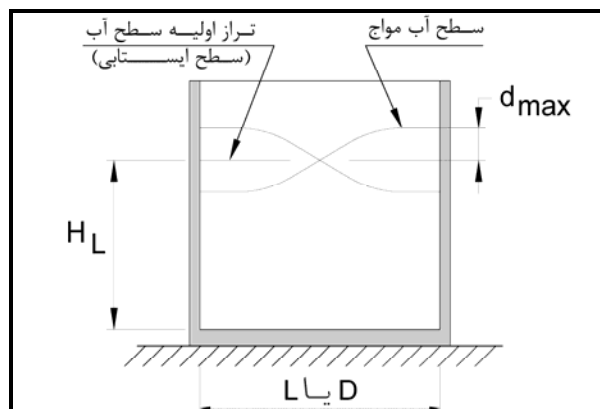
شکل ۳-۱۷- اضافه ارتفاع موج ناشی از ارتعاش افقی جرم موج مایع نگهداری‌شده [۴۹]
