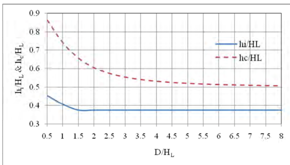
شکل ۳-۸- ضرایب h_i / H_L و h_c / H_L برای مخازن استوانه‌ای بدون در نظر گرفتن فشار نامتوازن وارد بر پی (EBP)
