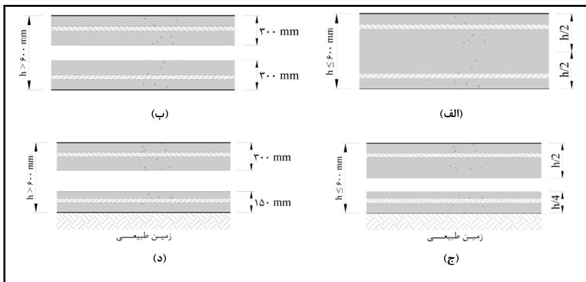
شکل ۴-۱۲- سطح موثر مقطع بتنی برای محاسبه آرماتورهای حرارتی و جمع‌شدگی
