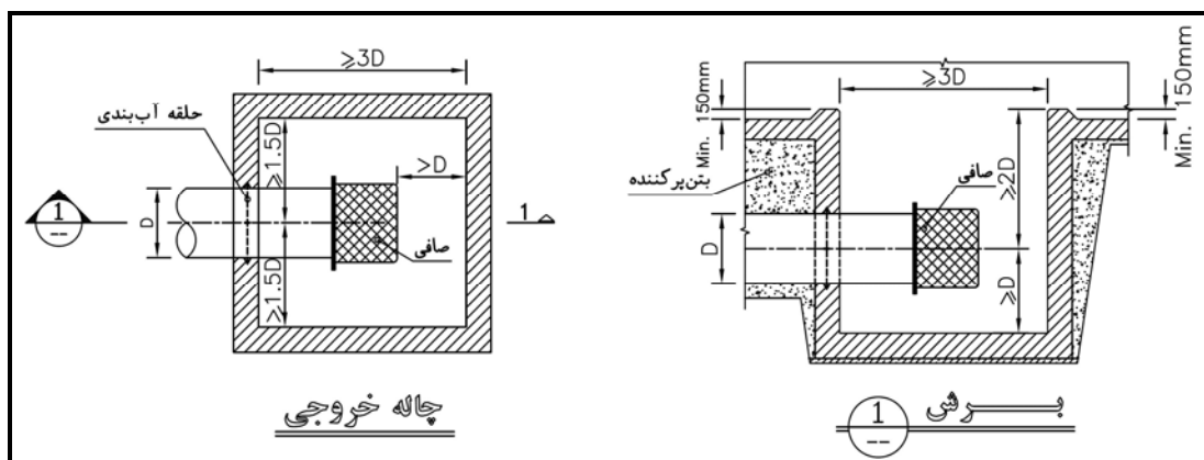
شکل ۱-۶- جزییات نمونه لوله خروجی
