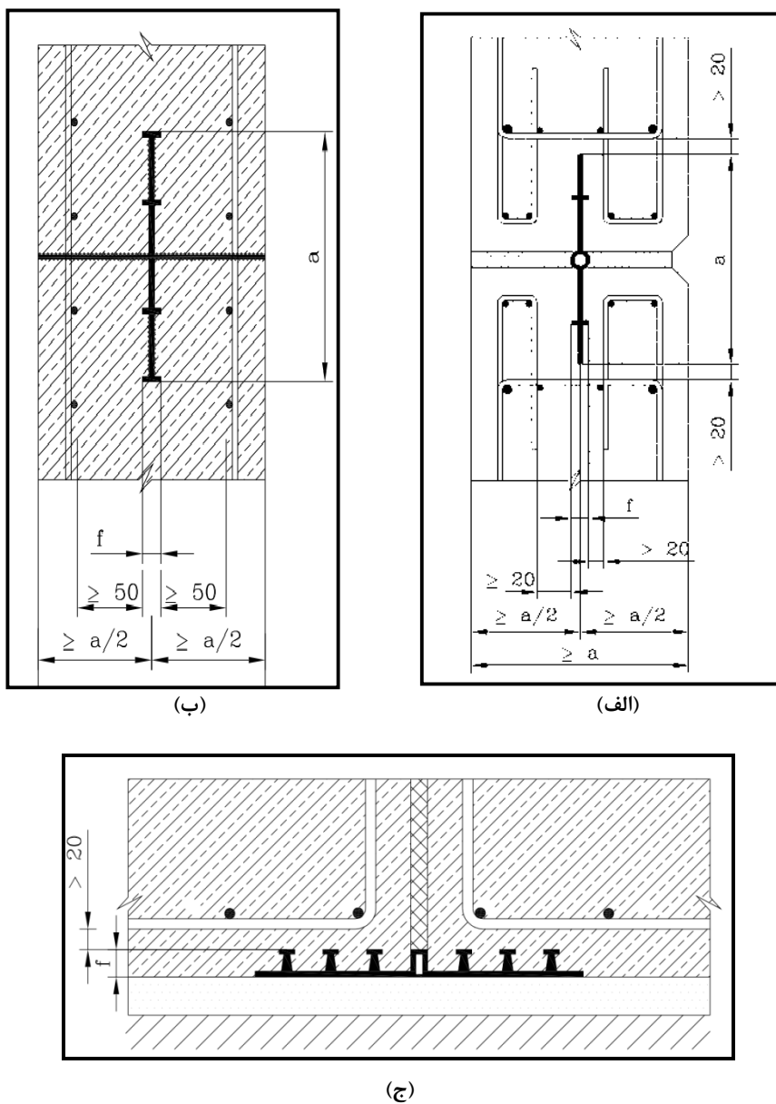
شکل ۵-۱۱- جزییات اجرایی نوارهای آب بند ترموپلاستیک [۸۲-۸۳] (اندازه‌ها به میلی‌متر می‌باشند)
