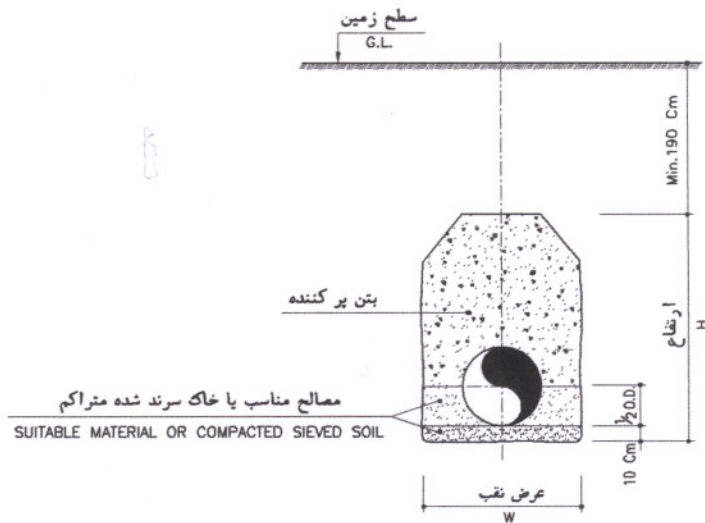
مقطع نقب
