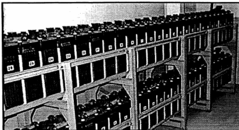
شکل ۱- مهار مناسب باتری ها توسط قفسه های نگهدارنده
