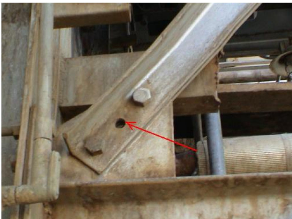
شکل ۲۴- عدم وجود پیچ در المان های سازه ای
