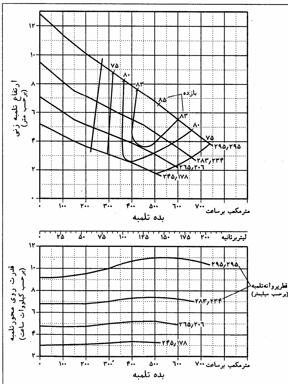
شکل ۲-۴- منحنی مشخصه‌های تلمبه با قطرهای مختلف
