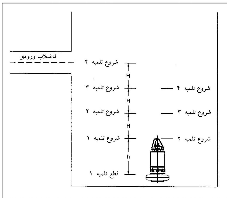
شکل ۶-۸- شیوه قرار گرفتن سطح‌سنجها
