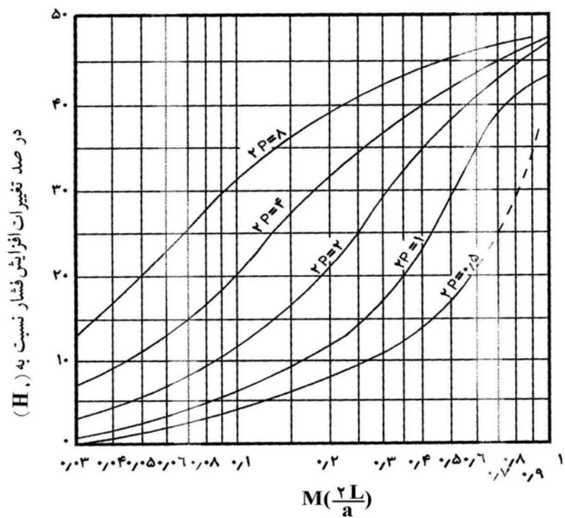
شکل ۵-۹- تغییرات افزایش فشار در محل تلمبه [۱۶]
