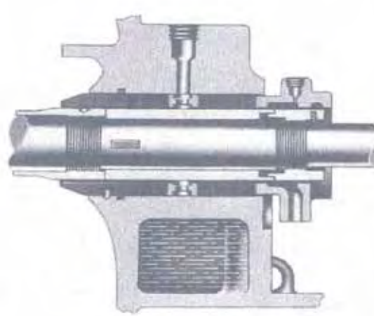
شکل ۷-۲-ب- دو نوع رینگ لترین
