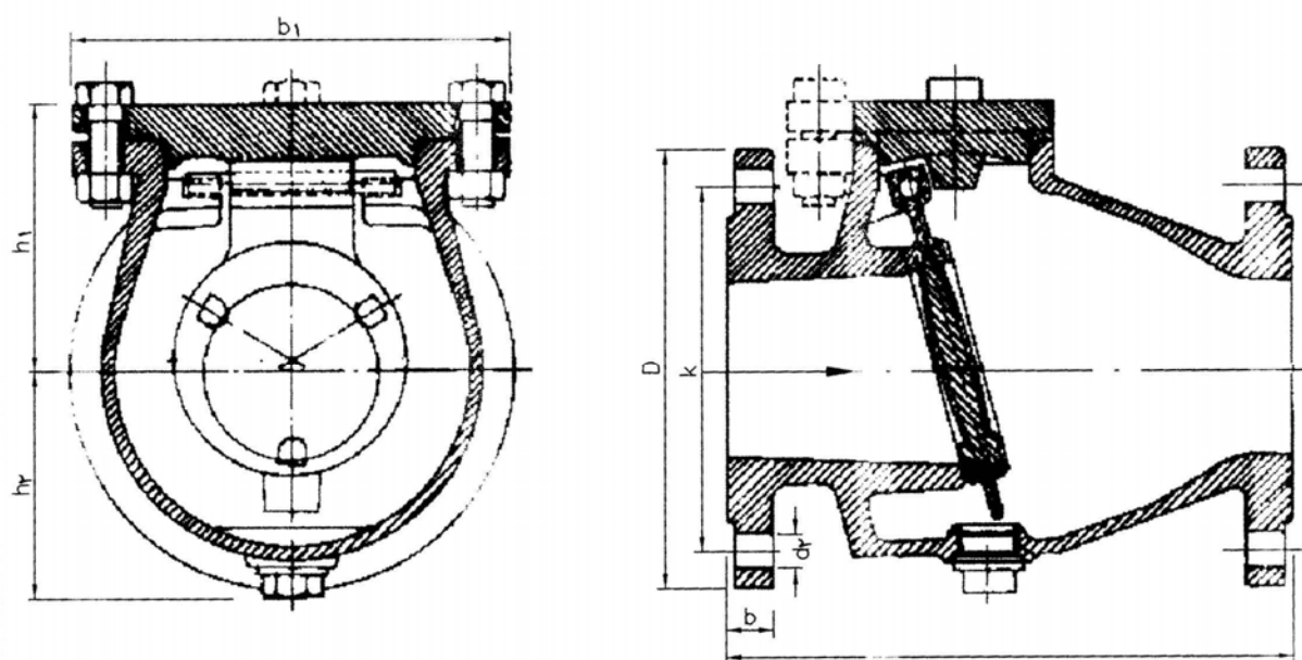
شکل ۵-۴- شیر یکطرفه ساده
