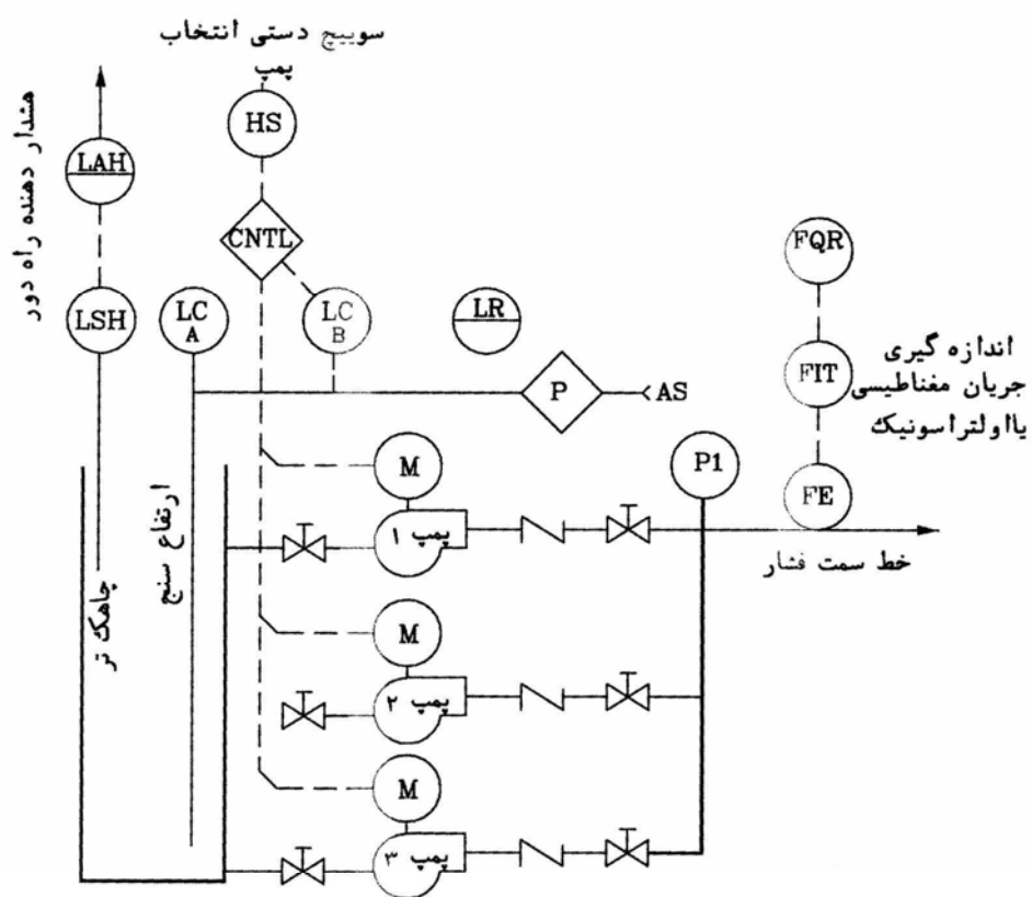
شکل ۷-۴ - P&ID تلمبه خانه فاضلاب نوع کوچک
