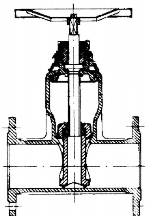
شکل ۵-۵- شیر قطع و وصل
