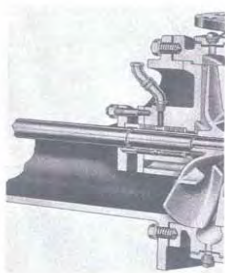
شکل ۷-۲-الف- آب بندی محور تلمبه به صورت لایبی (PACKING)
