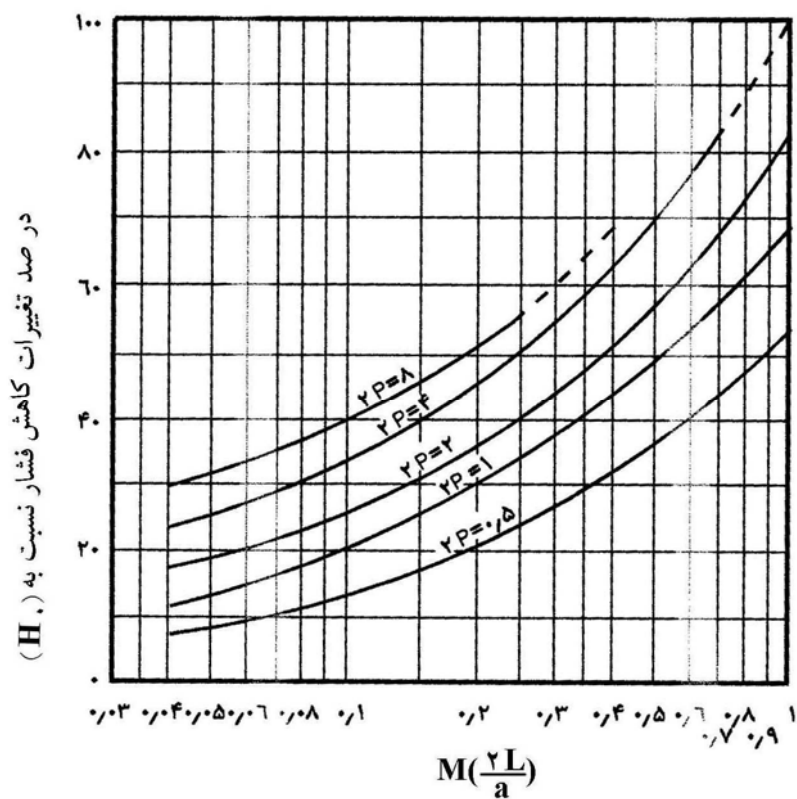
شکل ۵-۸- تغییرات کاهش فشار در نیمه خط انتقال [۱۶]
