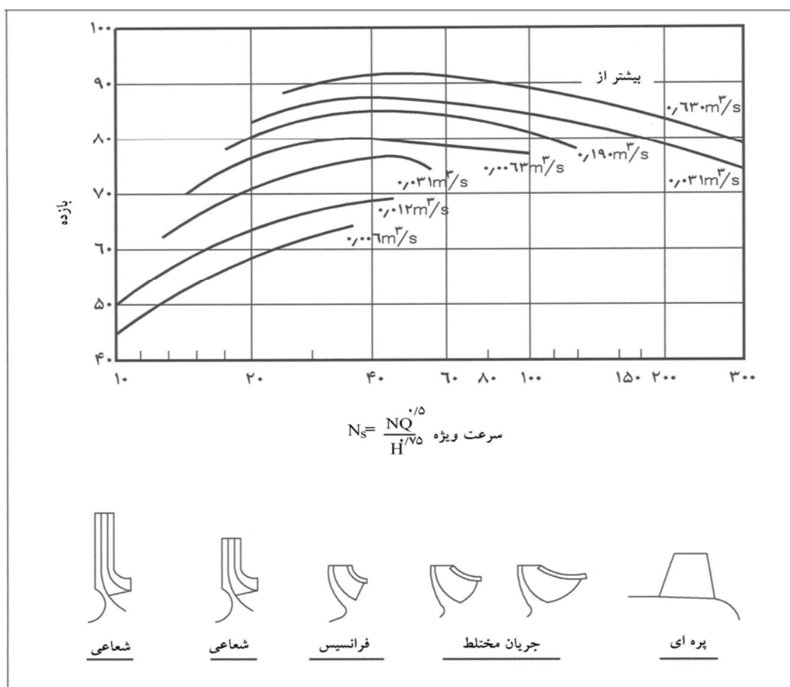
شکل ۲-۲- سرعت ویژه، شکل پروانه و بازده
