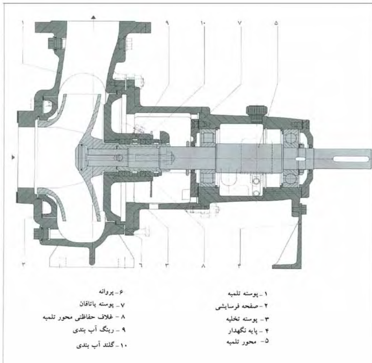
شکل ۴-۴- تلمبه گریز از مرکز افقی قابل نصب در چاهک خشک
