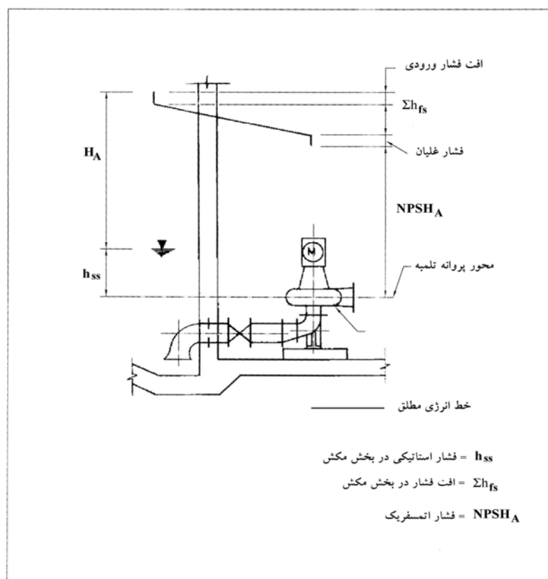
شکل ۴-۱ - عوامل لازم برای محاسبه NPSH_A
