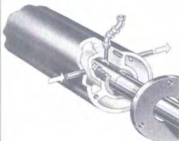
شکل ۷-۲-ب- دو نوع رینگ لترین
