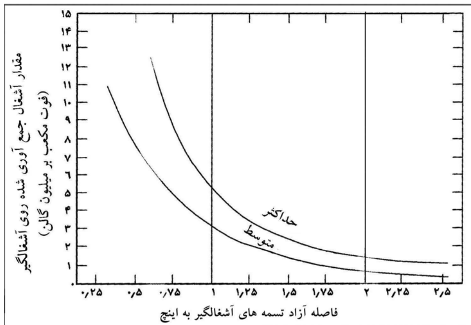
شکل ۸-۱- مقدار آشغال جمع شده روی آشغالگیر بر حسب فاصله آزاد میله‌ها
