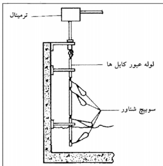
شکل ۷-۱- نحوه استقرار شناورها
