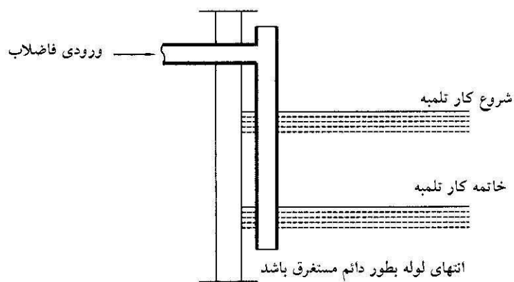
شکل ۶-۱۱-ب - چگونگی تخلیه خط ثقیلی به تلمبه خانه
