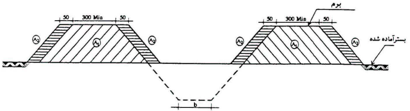
شکل ۶-۴. شمای مقطع خاکریزی
