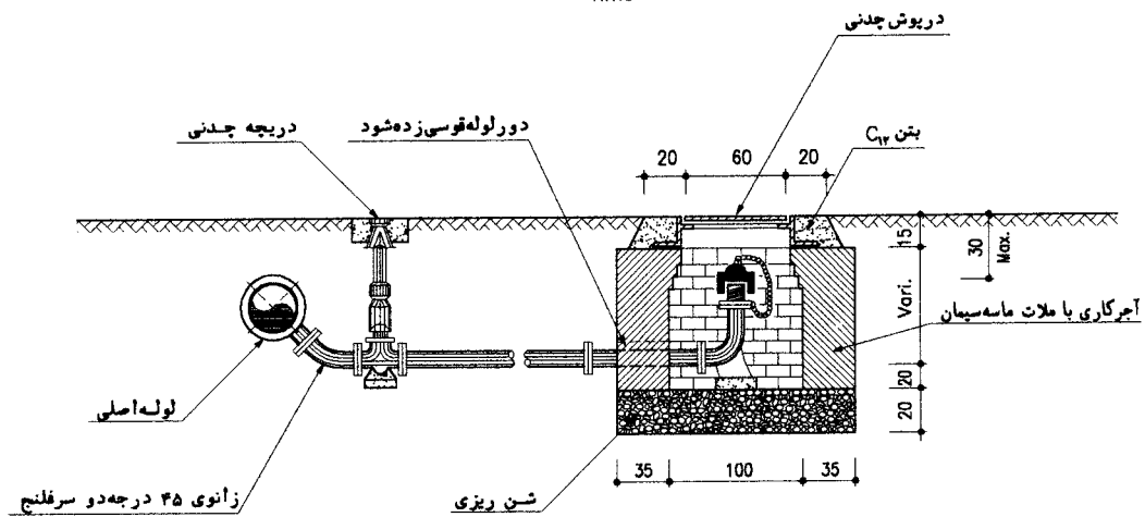
PLAN N.T.S
