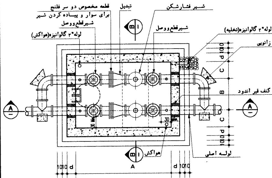
PLAN N.T.S
