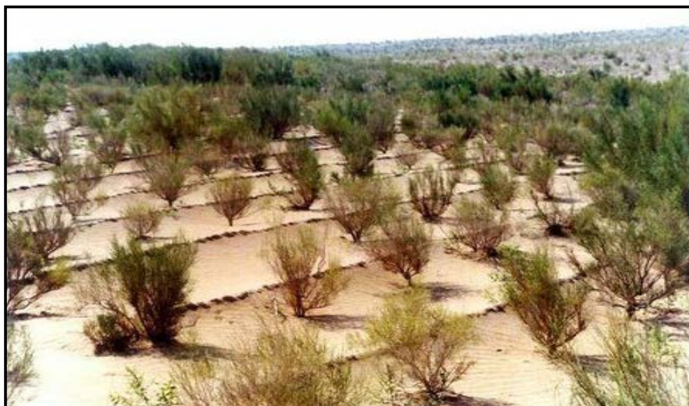
عکس ۳-۵- عملیات توام موانع رسی و کاشت گیاه برای تثبیت شن
