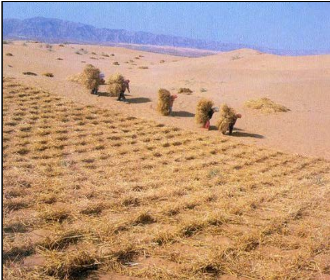
عکس ۶-۳- تثبیت تپه‌ها و پهنه‌های ماسه‌ای با استفاده از ساقه‌های برنج
