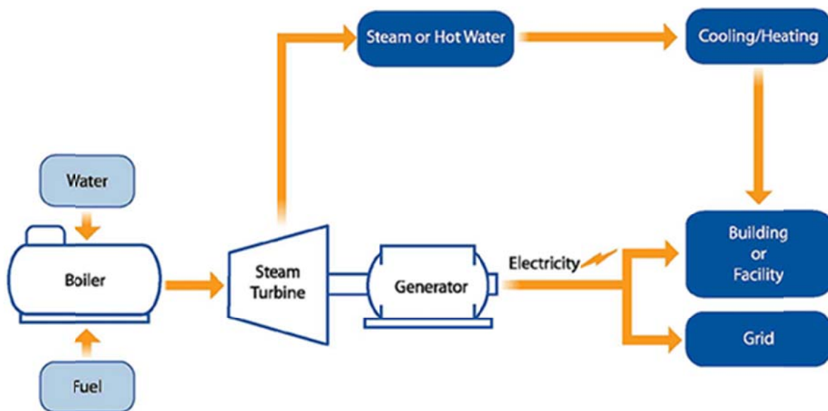
شکل ۲-۲-۲- CHP با چرخه‌ی نزولی
