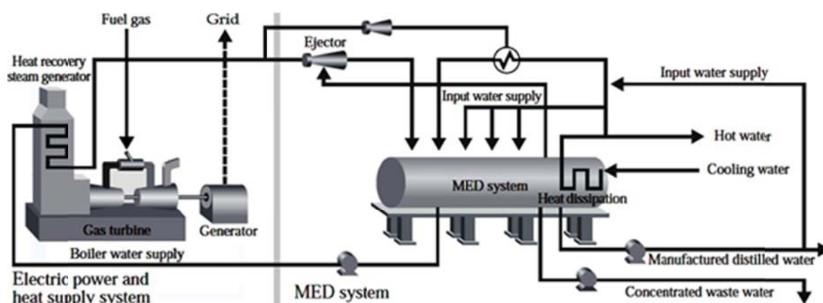
شکل ۷-۴- شماتیک عملکرد سیستم CHP متشکل از توربین گاز، بویلر بازیافت و آب شیرین کن MED [14]
