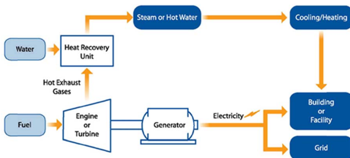
شکل ۱-۲- CHP با چرخه صعودی
