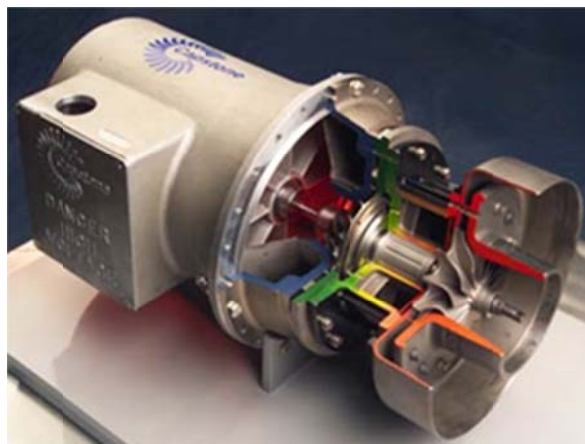
شکل ۲-۷- میکروتوربین با سیکل ساده
