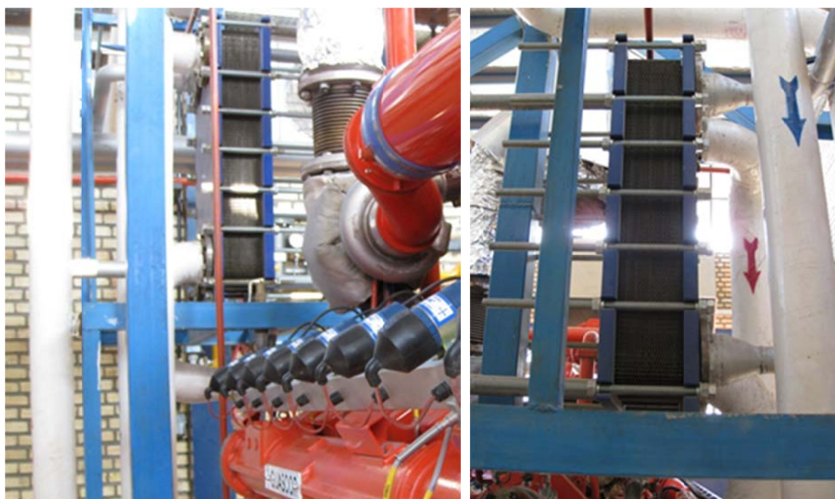
شکل ۴-۱۱- مبدل حرارتی
