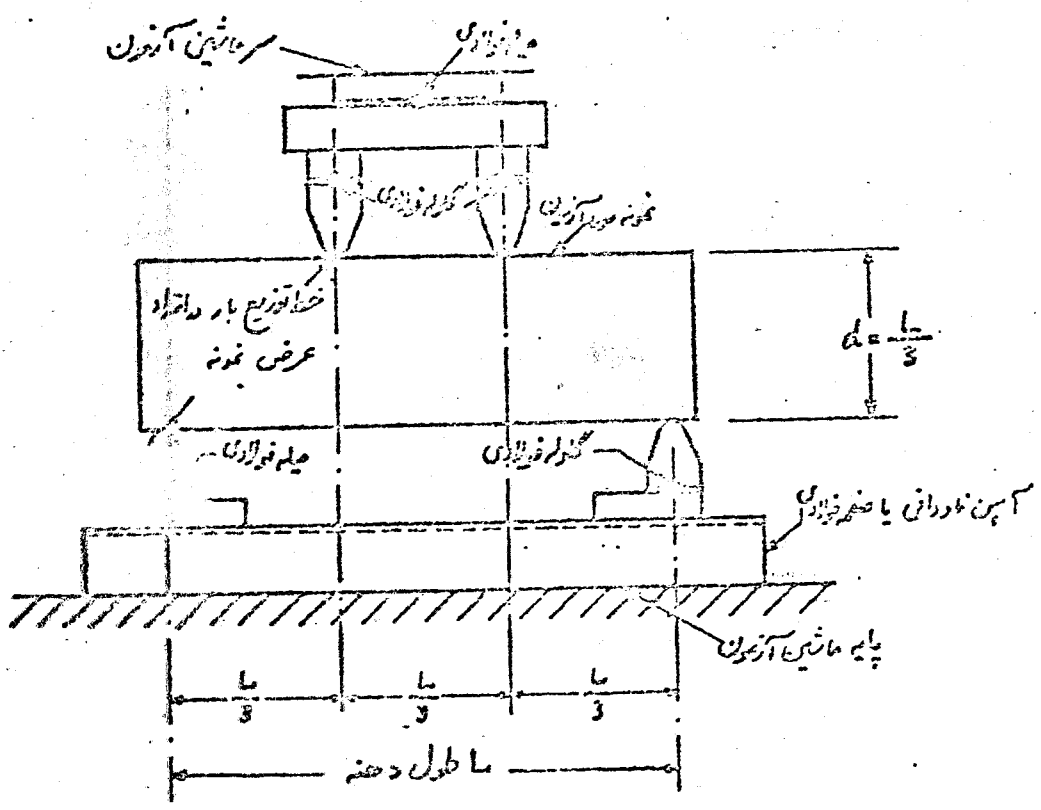
شکل ۱ - شکل هندسی دستگاه آزمون مقاومت خمشی بتون
