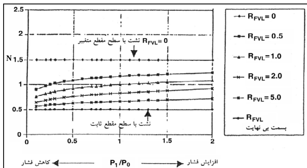
شکل ۴-۱- رابطه بین نسبت فشار و مقدار توان N در نظریه FAVAD [۱۸]
