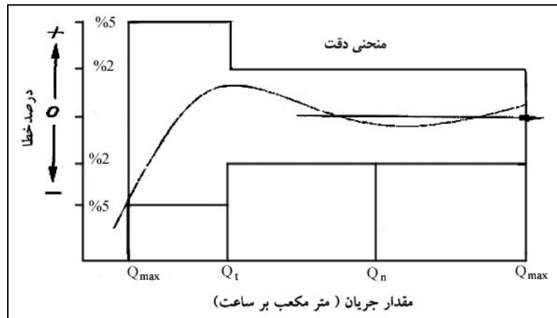
شکل ۱-۲- منحنی عملکرد کنتور
