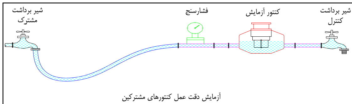
شکل ۲-۲- ابزار آزمایش کنتور در محل
