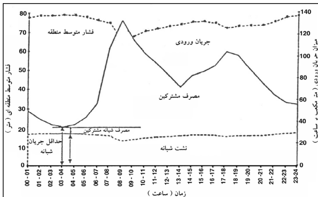
شکل ۱-۳- اجزای اصلی جریان ورودی به سامانه قبل از مدیریت فشار [۱۸]
