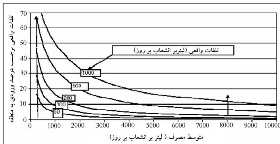
شکل ۱-۱۱- نمودار اثر مصرف بر بیان نشت به صورت درصدی از حجم آب ورودی به منطقه [۱۴]
