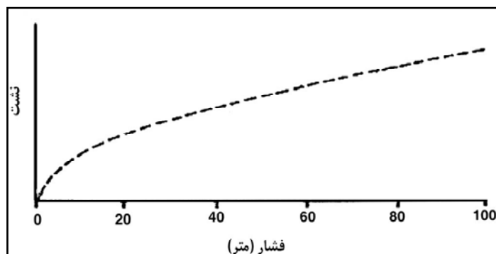
شکل ۱-۱- رابطه بین نشت و فشار برای یک اریفیس [۲۷].
