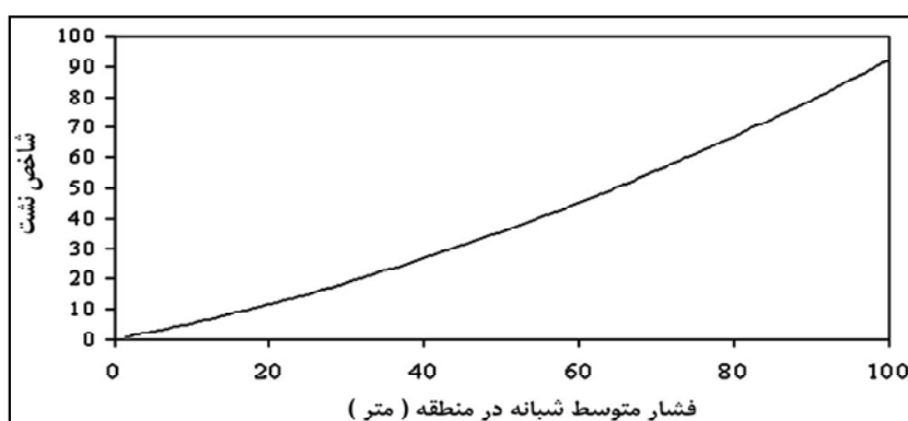
شکل ۱-۲- رابطه نشت - فشار [۲۷]
