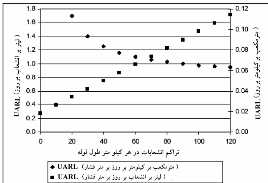
شکل ۱-۱۲- نمودار تغییرات UARL با تراکم انشعابات [۱۴]
