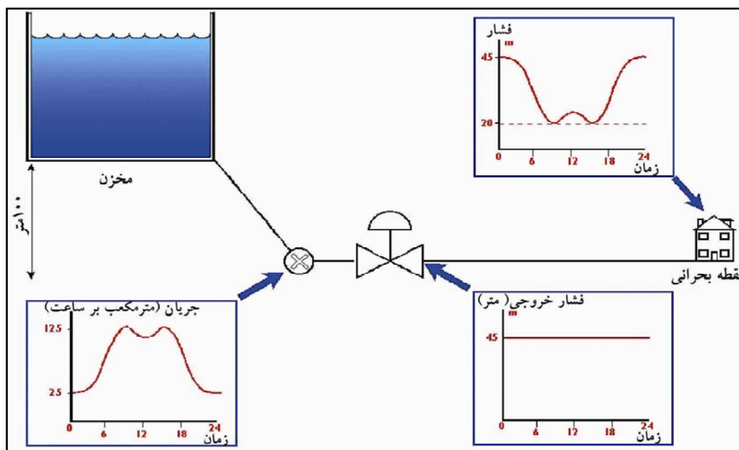
شکل ۳-۱- مدیریت فشار با نصب فشارشکن با خروجی ثابت در شبکه
