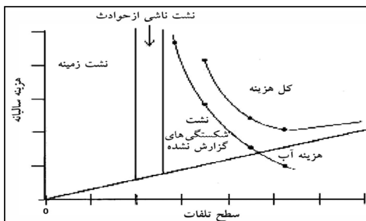
شکل ۴-۳- نمودار سطح اقتصادی کنترل نشت سالانه
