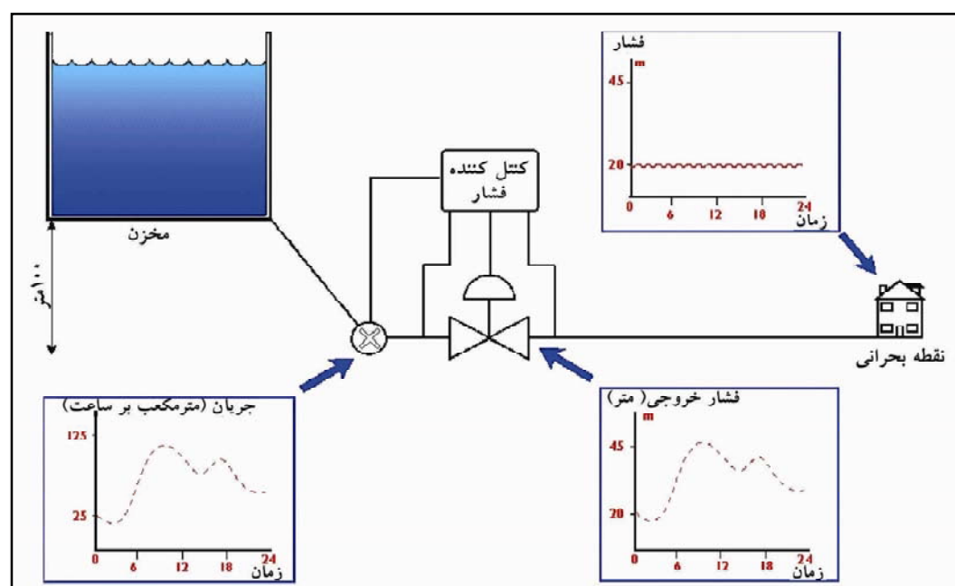
شکل ۳-۲- مدیریت فشار با کنترل هوشمند فشارشکن (تعدیل فشار و اعمال مدیریت مصرف)
