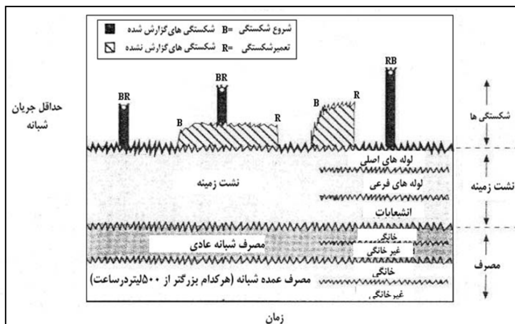
شکل ۱-۵- اجزای حداقل جریان شبانه [۳۰]
