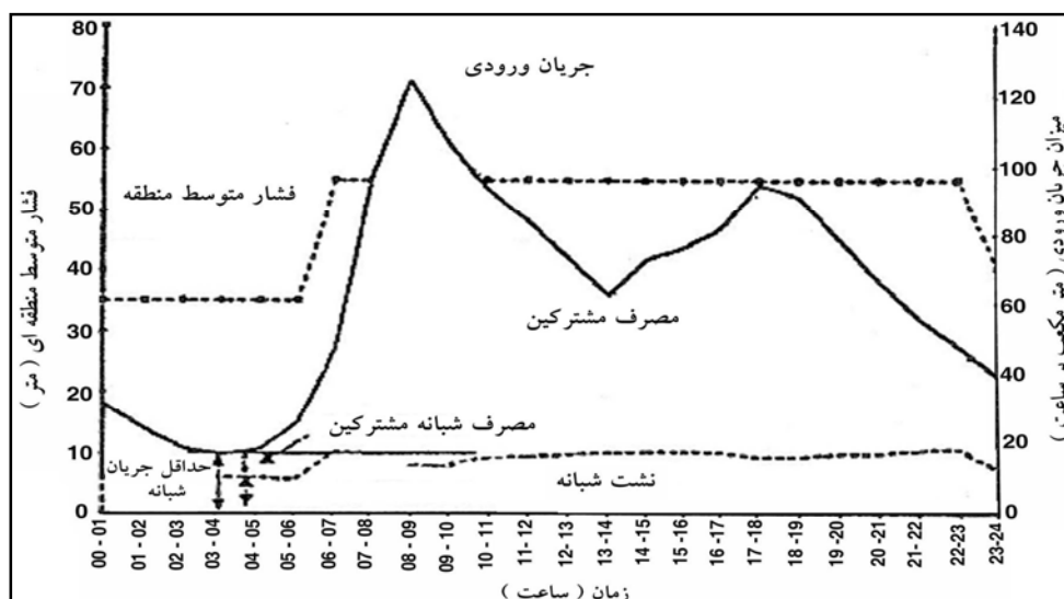
شکل ۱-۱۰- اجزای اصلی جریان ورودی به سامانه توزیع پس از مدیریت فشار [۱۸] (محور افقی متوسط زمان بین دو ساعت را نشان می دهد)
