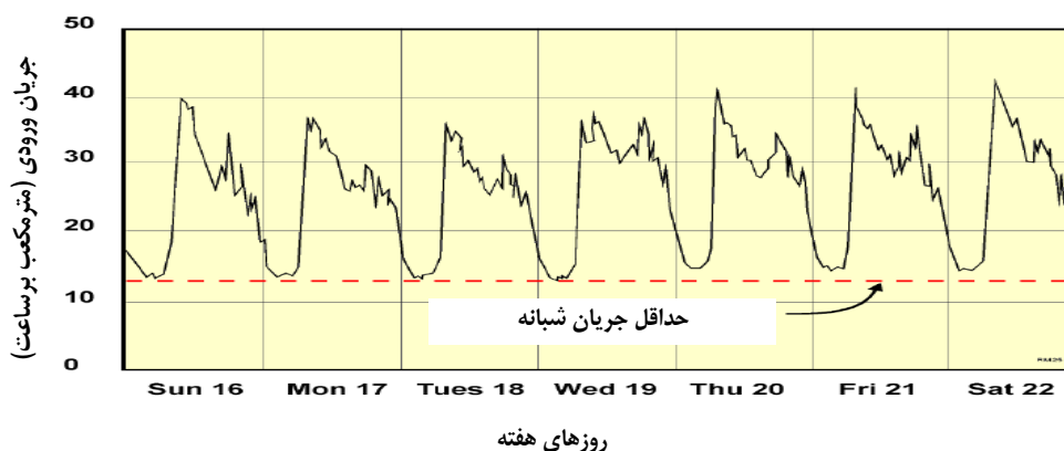
شکل ۱-۷- حداقل جریان شبانه در یک شبکه
