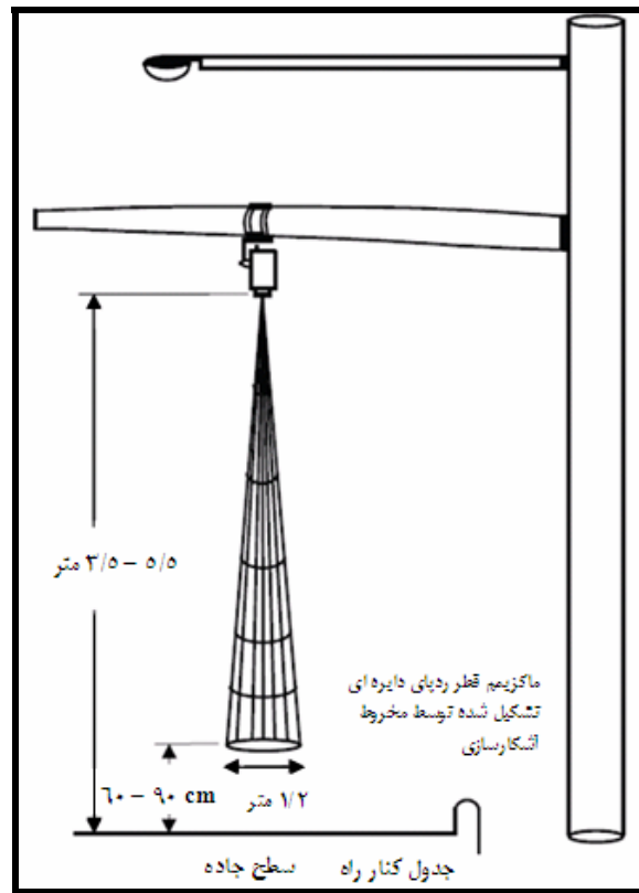
شکل ۴-۵۰- نحوه نصب حسگر مافوق صوت
