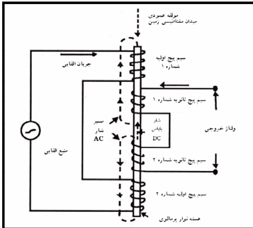
شکل ۲-۱۶- مدار الکتریکی شناسگر مغناطیسی
