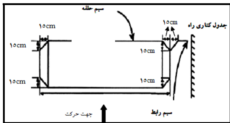
شکل ۲-۶- طرح حلقه القایی عریض
