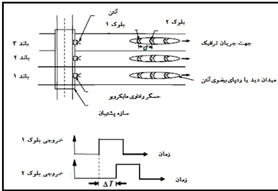
شکل ۲-۲۹- تقسیم کردن میدان دید در جهت حرکت وسیله به چند بلوک
