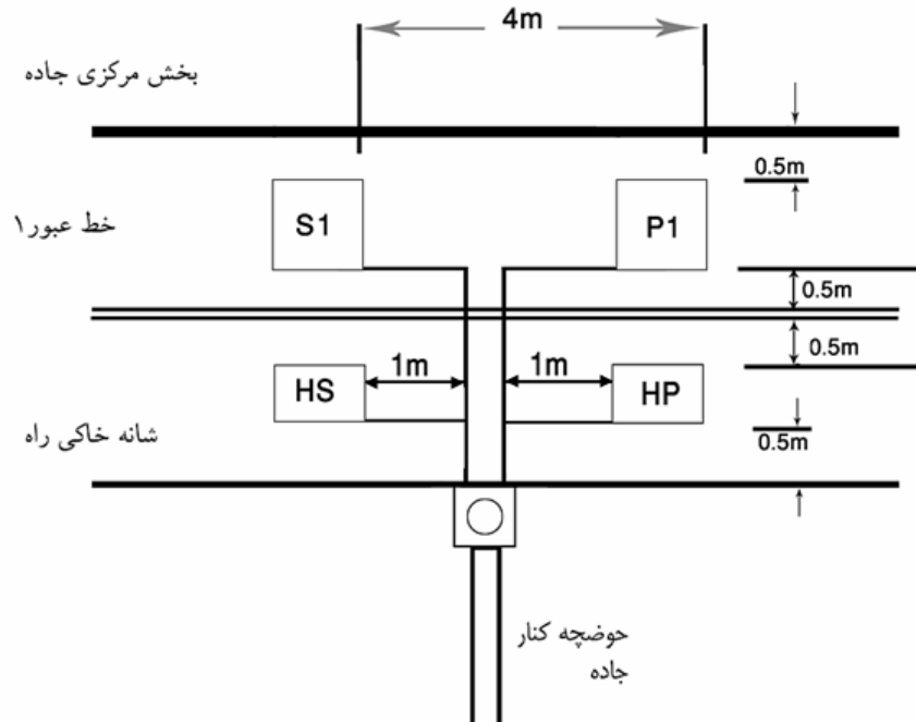
شکل ۱-۴- طرح نصب حلقه القایی در یک خط محور و شانه خاکی راه
