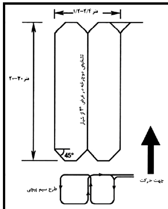
شکل ۷-۲- حلقه‌های چهار قطبی
