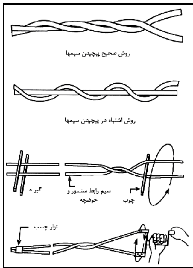
شکل ۴-۱۱- روش‌های پیچیدن کابل رابط حسگر با حوضچه
