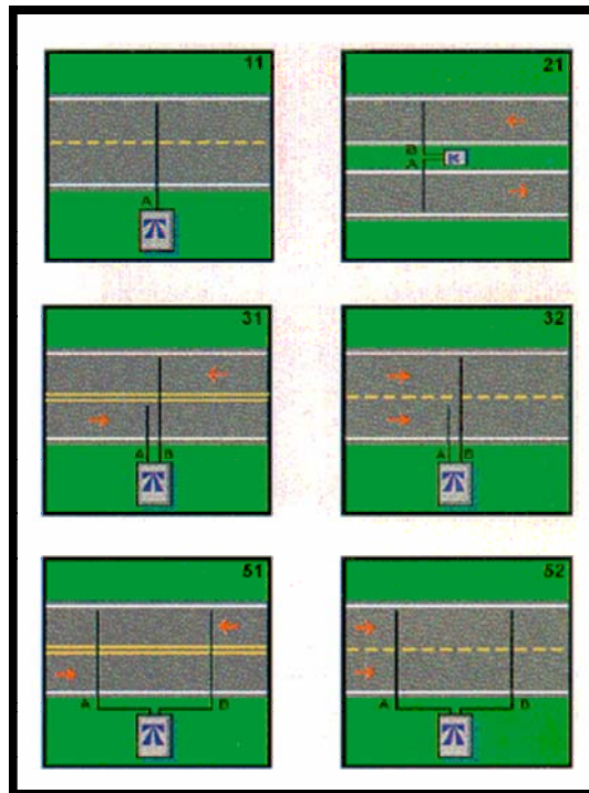
شکل ۲-۱۴- نحوه قرارگیری حسگرهای بادی در انواع جاده‌ها
