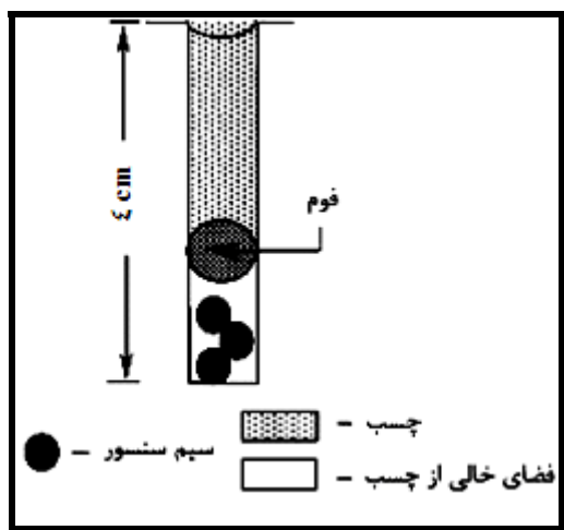
شکل ۴-۹- روش کاربرد فوم
