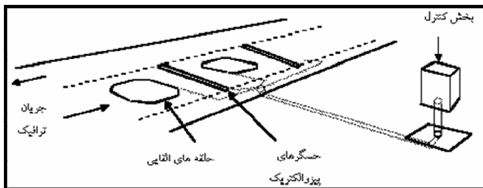
شکل ۲-۲۱- نحوه نصب حسگر پیزو الکتریک در سیستم توزین در حال حرکت
