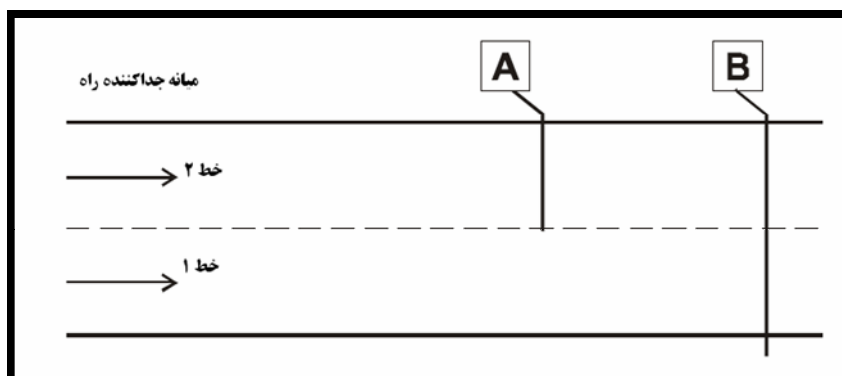
شکل ۴-۲۵- ترددشماری راه چندخطه با استفاده از ترددشمار بادی با یک ورودی تیوپ واحد
