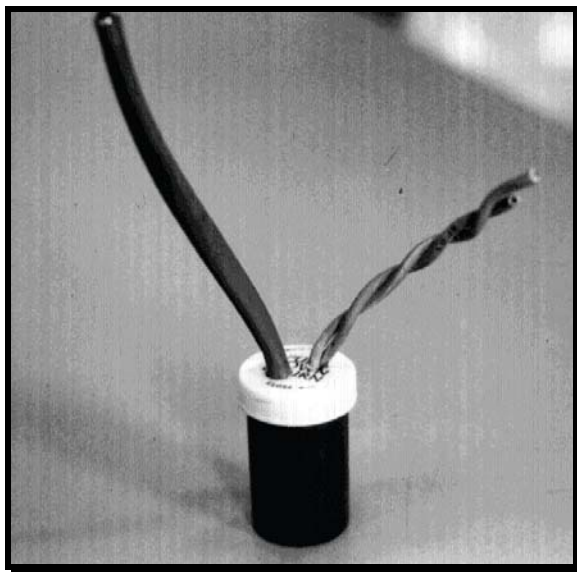
شکل ۴-۱۴- قرار دادن اتصال سیم حلقه و کابل رابط حوضچه و واحد الکترونیک در یک بطری
