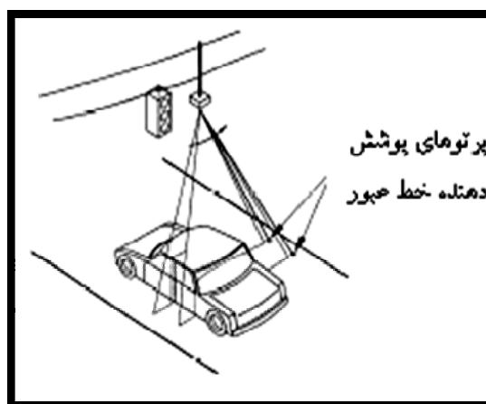
شکل ۲-۳۱- نحوه نصب رادار پرتو لیزری
