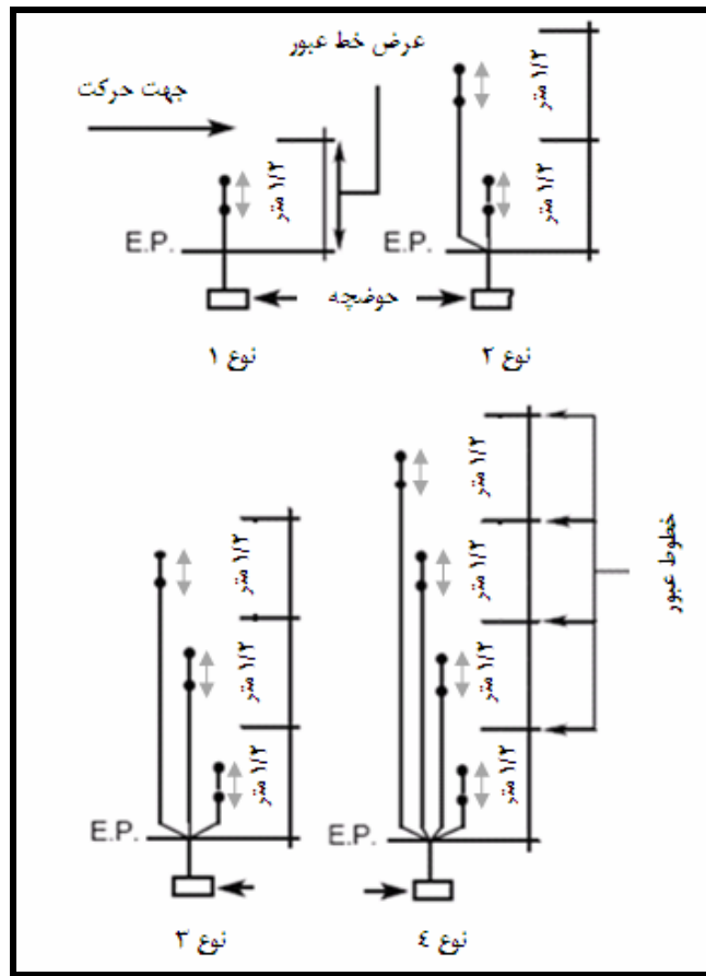
شکل ۴-۲۹- ترکیب‌بندی‌های مختلف مغناطیس‌سنج دوماحوره
