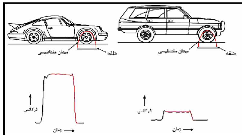
شکل ۲-۳- تغییر فرکانس حلقه حسگر در دو وسیله با ارتفاع متفاوت
