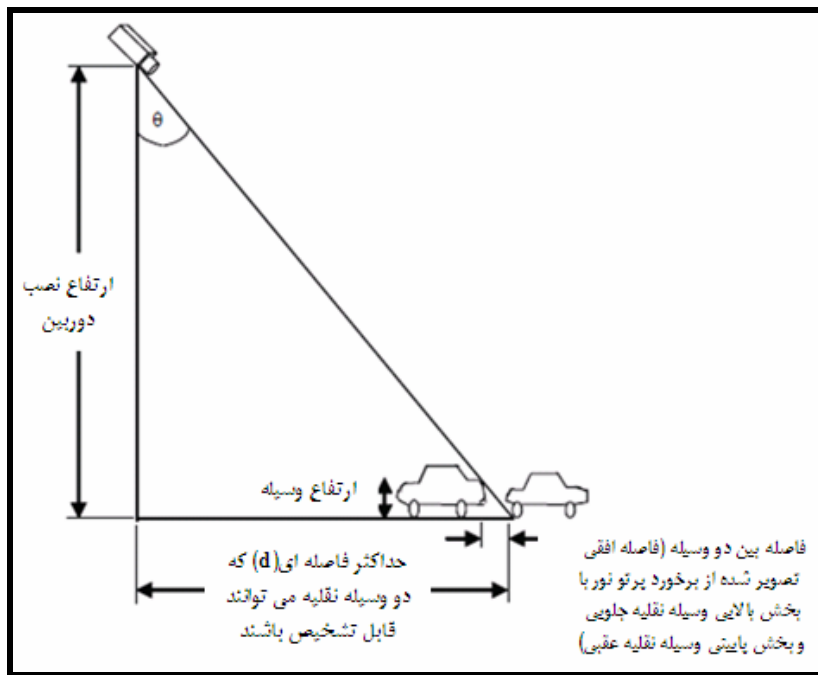
شکل ۴-۴۸- نمایش فاصله قابل تشخیص دو وسیله نقلیه متوالی برای دوربین پردازش تصویر
