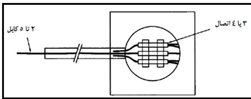
شکل ۴-۲۰- نحوه قرار گرفتن سیم حلقه‌ها و کابل‌ها در حوضچه- پلان
