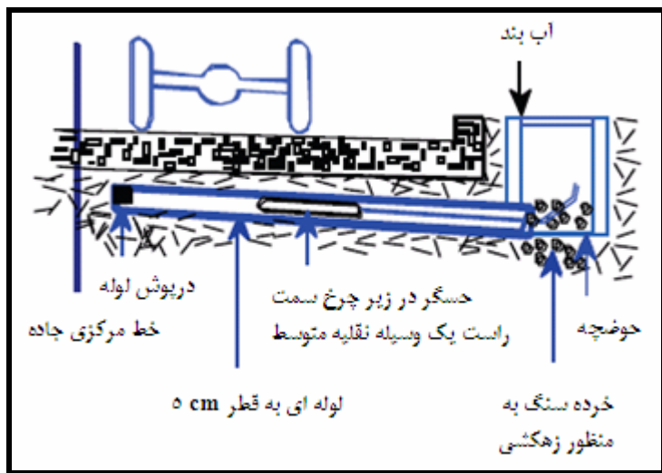
شکل ۴-۳۵- نصب شناسگر مغناطیسی از کناره یا میانه راه
