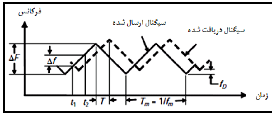
شکل ۲-۲۸- موج پیوسته
