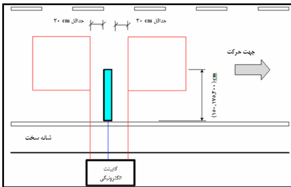
شکل ۴-۴۳- نحوه نصب حسگر کوارتز در یک خط عبور به روش آماری
