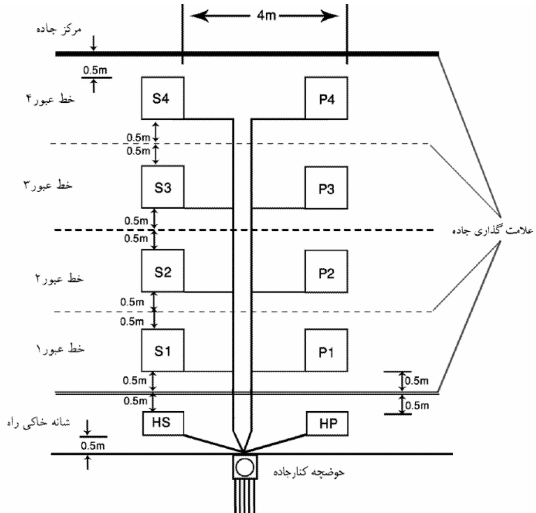
شکل ۵-۴ - طرح نصب حلقه القایی در چهار خط محور و شانه خاکی راه
