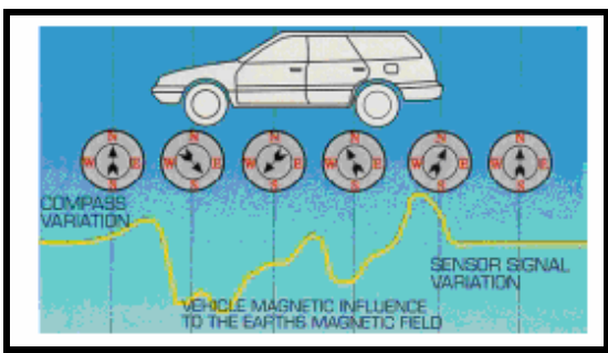
ب- تاثیر جسم فلزی بر میدان مغناطیسی زمین
