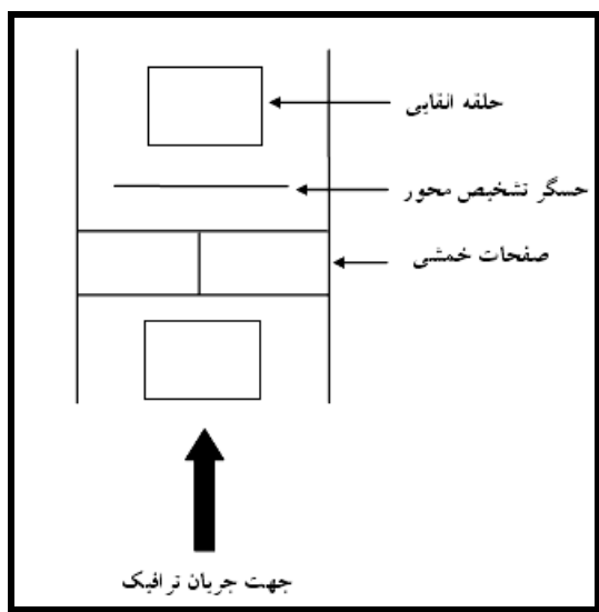
شکل ۴-۳۶- سیستم توزین در حال حرکت صفحه خمشی
