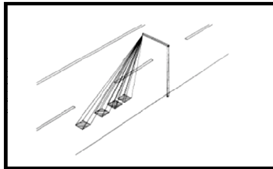
شکل ۲-۳۲- پیکر بندی حسگرهای مادون قرمز غیرفعال با چندین منطقه آشکارسازی
