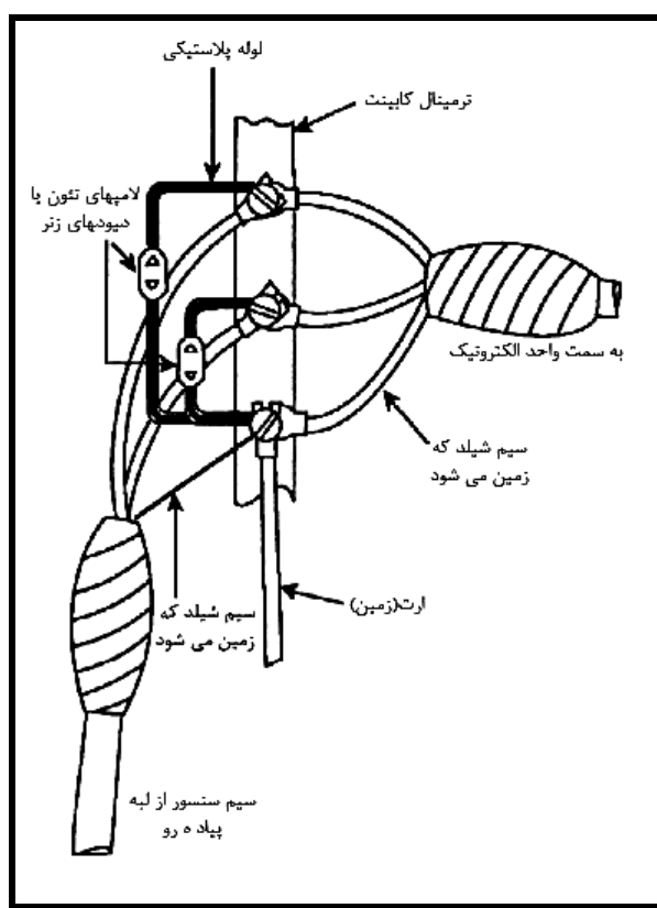
شکل ۴-۲۱- اتصال به زمین کابل رابط در ترمینال کابینت
