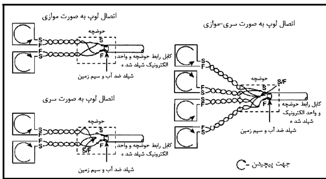
شکل ۴-۱۲- روش‌های به هم تابیدن سیم حسگر برای نصب چند حلقه
