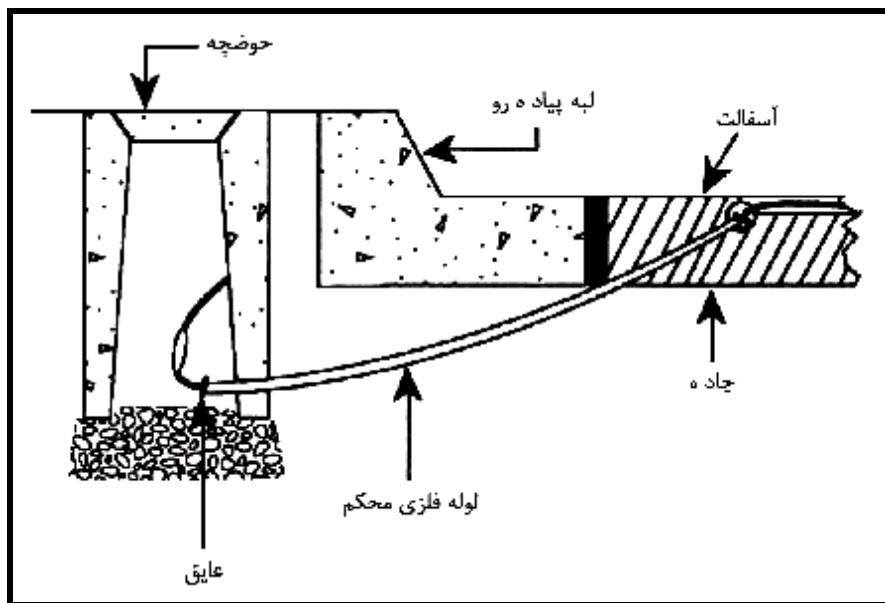
شکل ۴-۱۸- جزئیات قرار دادن سیم رابط برای جداول کم عمق
