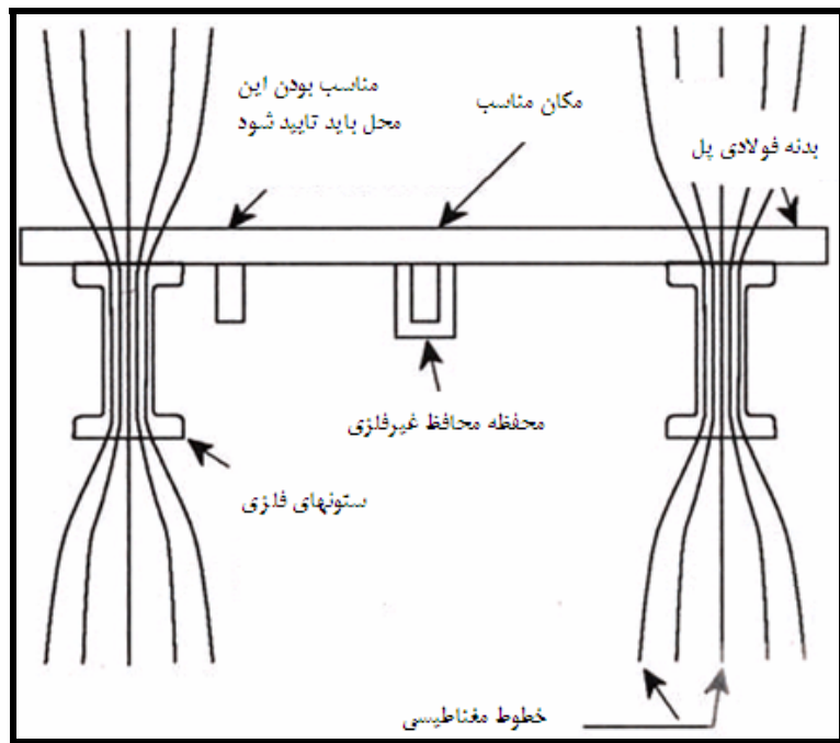
شکل ۴-۲۸- نصب مغناطیس‌سنج‌ها در بدنه پل
