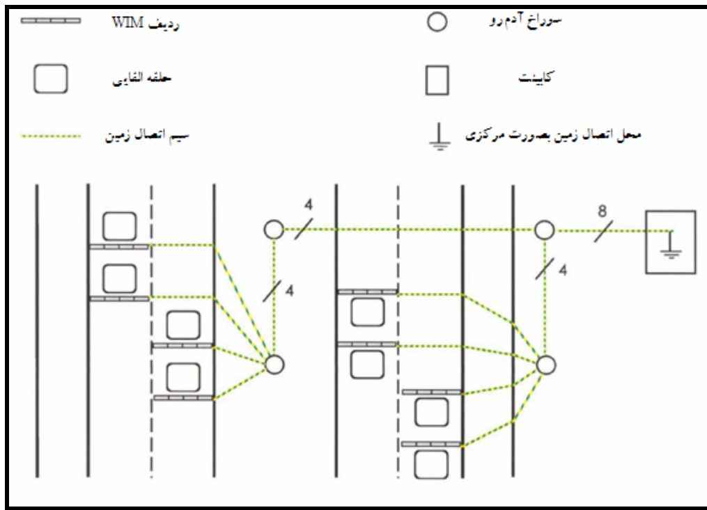
شکل ۴-۴۵ نحوه اتصال به زمین حسگرها در کابینت کنترلر
