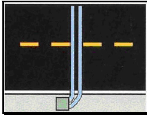
شکل ۴-۲۳- نحوه نصب تیوپ‌ها برای تعیین جهت حرکت وسایل نقلیه
