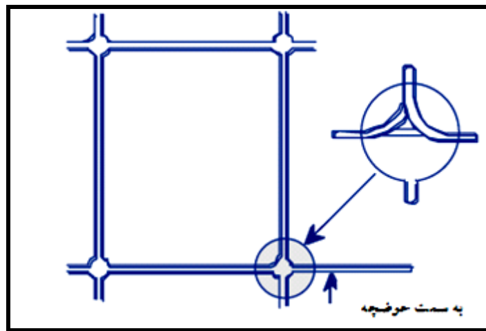
شکل ۴-۸- نمونه برداری با مته در گوشه های حلقه
