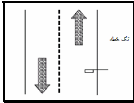
شکل ۴-۳۳- نصب حسگر مغناطیسی در مسیرهای تک خطه منتهی به خط ایست
