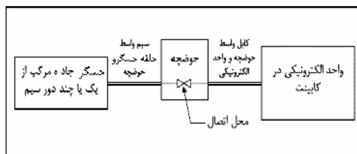
شکل ۲-۱- سیستم شناسگر حلقه القایی
