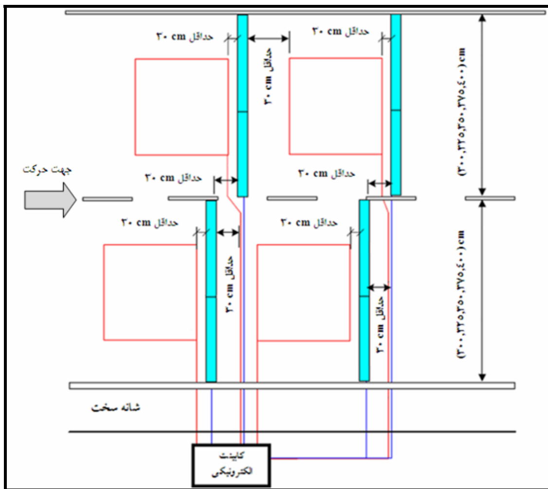
شکل ۴-۴۱- نحوه نصب حسگر کوارتز در دو خط عبور به روش استاندارد
