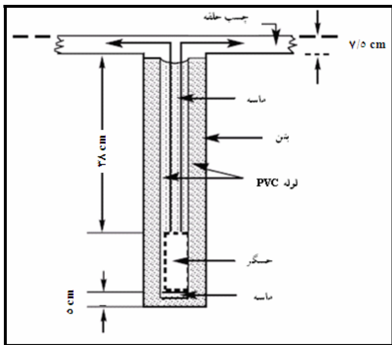
شکل ۴-۳۱- طرح استاندارد برای نصب مغناطیس سنج
