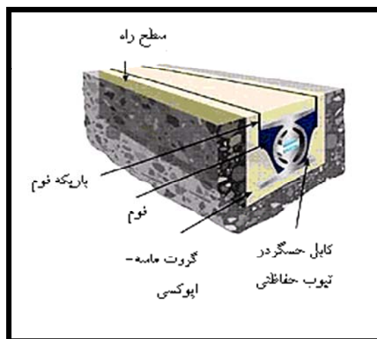
شکل ۲-۲۴- حسگر پیزوالکتریک کوارتز
