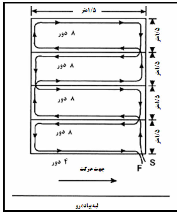
شکل ۲-۱۱- طرح حلقه تشخیص دوچرخه با استفاده از حلقه‌های چهارقطبی پهلوی به پهلوی
