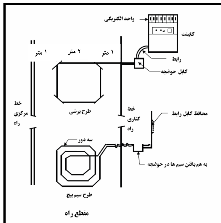
شکل ۲-۲- نمای یک نمونه از حسگر حلقه القایی نصب شده
