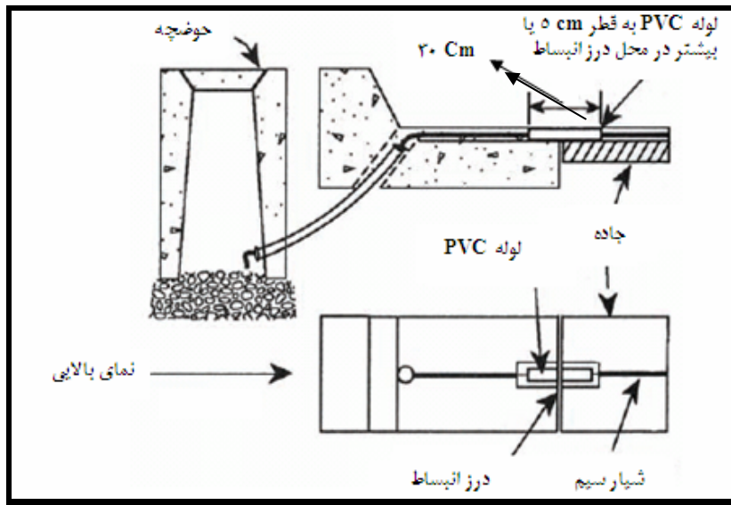
شکل ۴-۱۷- قراردادن سیم رابط حلقه در لوله در محل برخورد با جدول کناری راه
