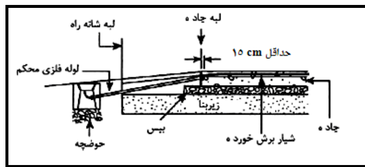
شکل ۴-۱۶- سیم های رابط حلقه در لبه روسازی در غیاب جدول
