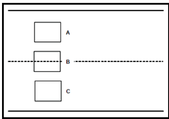
شکل ۴-۶- نحوه نصب یک حلقه القایی اضافه بین دو حلقه به منظور شمارش دقیق تر وسایل نقلیه
