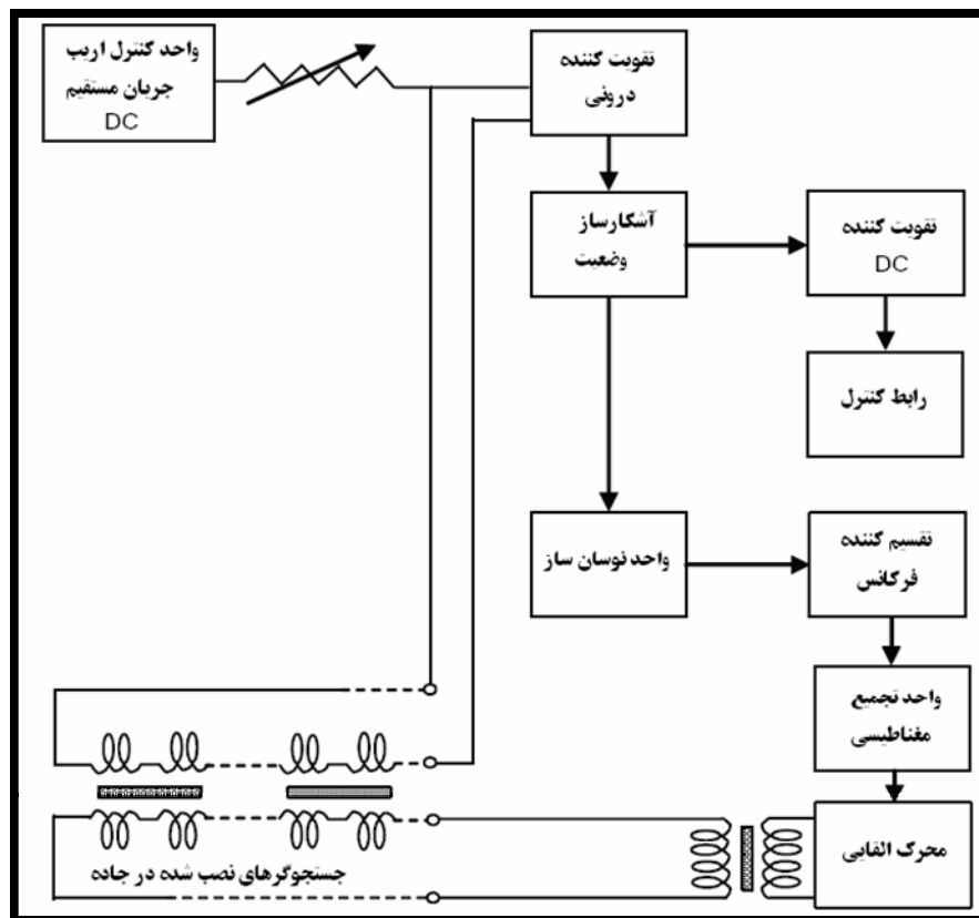
شکل ۲-۱۷- مغناطیس سنج دوماحوری و واحد الکترونیکی معادل مدار الکتریکی
