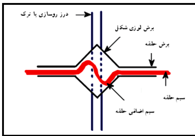
شکل ۴-۱۰- استفاده از برش لوزی شکل در محل تقاطع با درز روسازی
