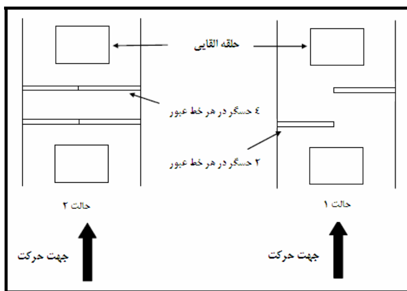
شکل ۴-۳۹- حسگرهای توزین در حال حرکت کوارتز
