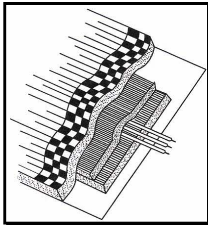
شکل ۲-۱۲- پنج لایه حلقه القایی سیار باز
