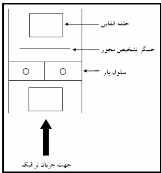
شکل ۴-۴- سیستم توزین در حال حرکت سلول بار
