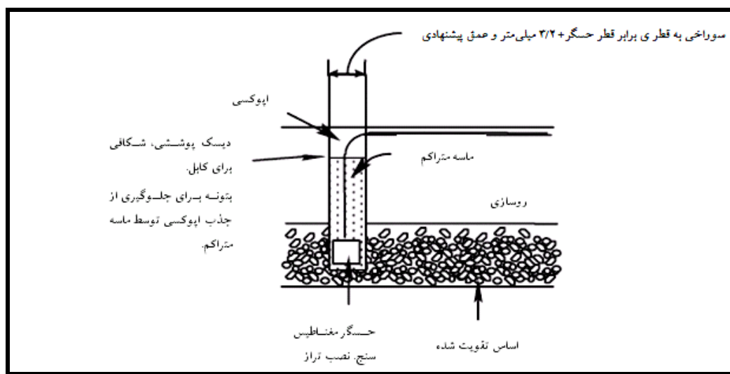
شکل ۴-۳۰- نصب حسگر مغناطیس سنج
