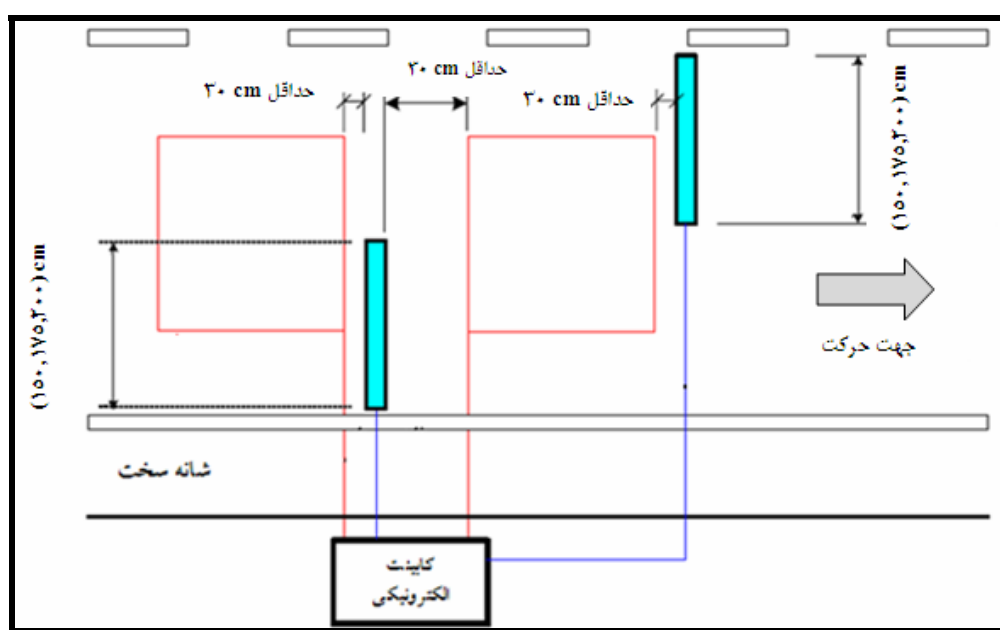
شکل ۴-۴۲- نحوه نصب حسگر کوارتز در یک خط عبور به روش پلکانی
