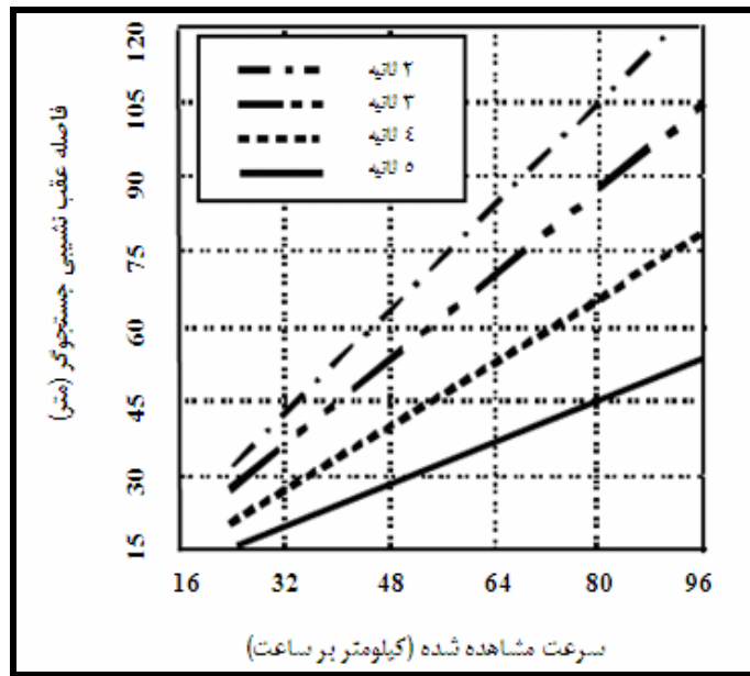
شکل ۴-۳۲- عقب‌نشینی حسگر مغناطیسی از خط ایست براساس سرعت و سرفاصله زمانی مجاز
