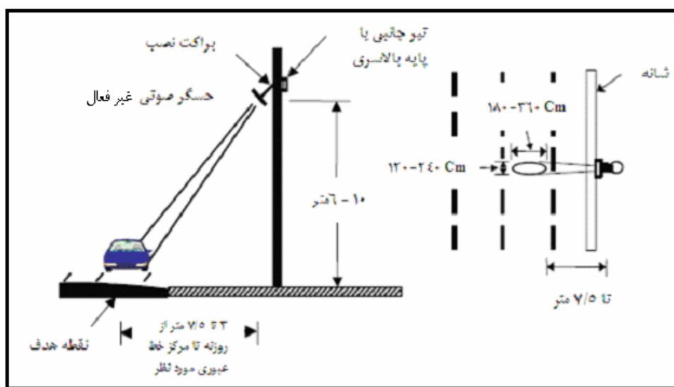
شکل ۴-۵۱- نحوه نصب حسگر صوتی غیر فعال
