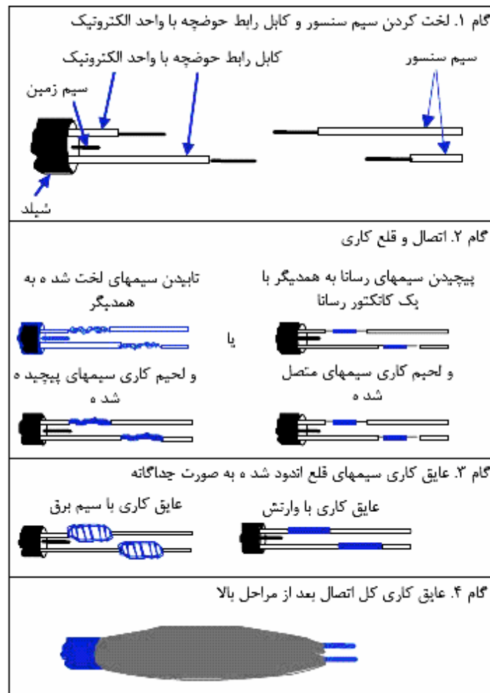
شکل ۴-۱۳- مراحل اتصال سیم حلقه به کابل رابط بین حوضچه و واحد الکتریکی
