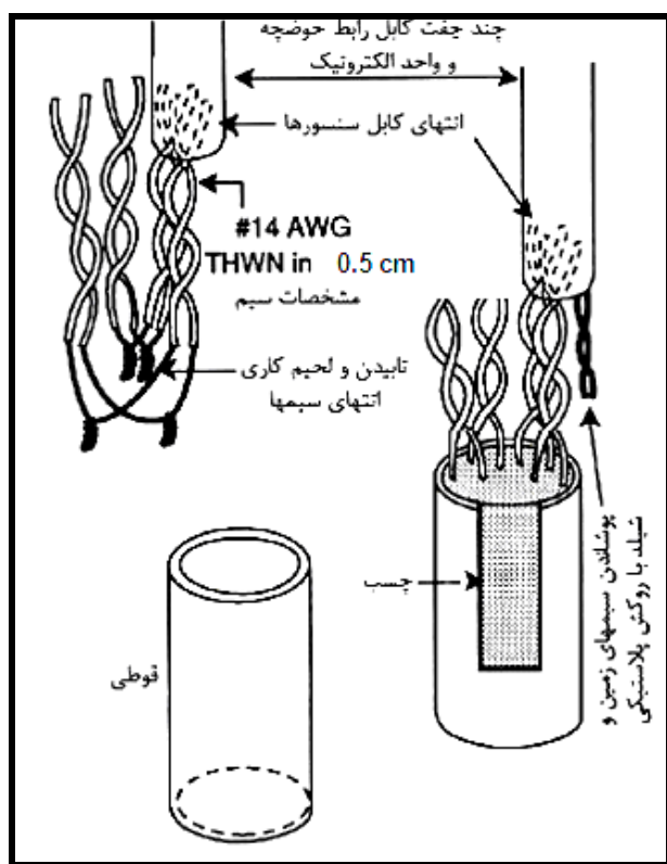
شکل ۴-۱۵- جزئیات تابیدن کابلها در یک بطری
