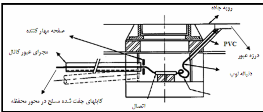
شکل ۴-۱۹- نحوه قرار گرفتن سیم حلقه‌ها و کابل‌ها در حوضچه- برش عرضی
