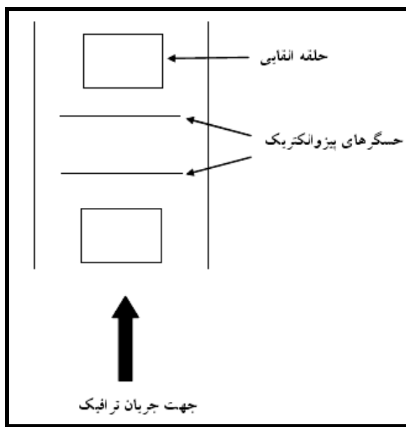
شکل ۴-۳۸- سیستم توزین حین حرکت پیزوالکتریک
