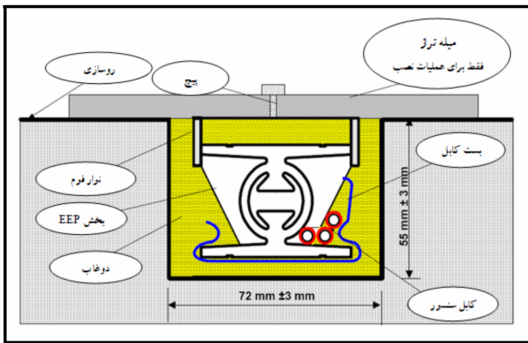
شکل ۴-۴- نحوه قرار گرفتن حسگر در روسازی راه
