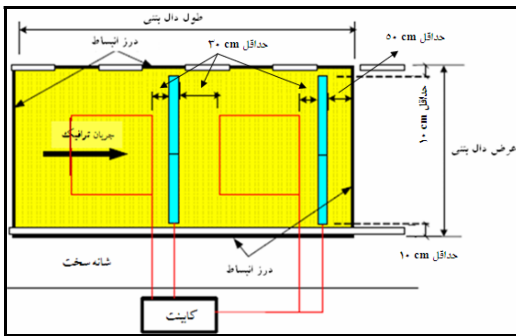
شکل ۴-۴۶- طرح نصب حسگر کوارتز در روسازی بتنی
