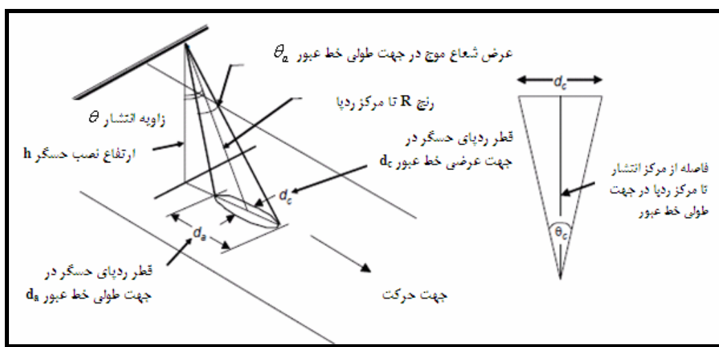
شکل ۴-۴۹- منطقه آشکارسازی حسگر میکروویو برای بازبینی جریان بالادست و پایین دست
