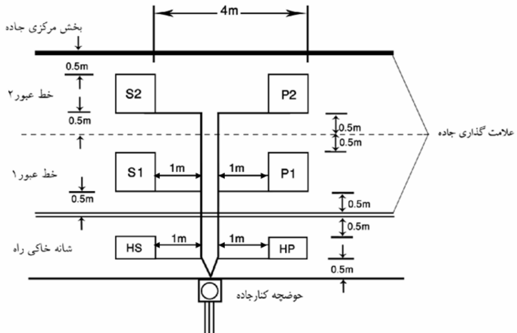
شکل ۳-۴- طرح نصب حلقه القایی در دو خط محور و شانه خاکی راه
