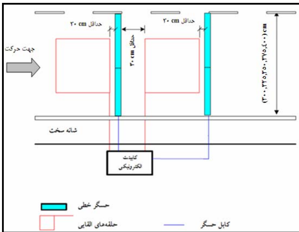
شکل ۴-۴- نحوه نصب حسگر کوارتز در یک خط عبور به روش استاندارد
