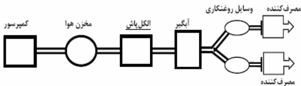
شکل ۱۱-۴- محل نصب دستگاه الکلی پاش
