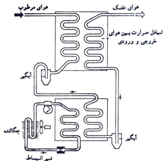
شکل ۹-۲- نحوه‌ی حرکت هوای فشرده در سردکننده‌ی انتهایی.
