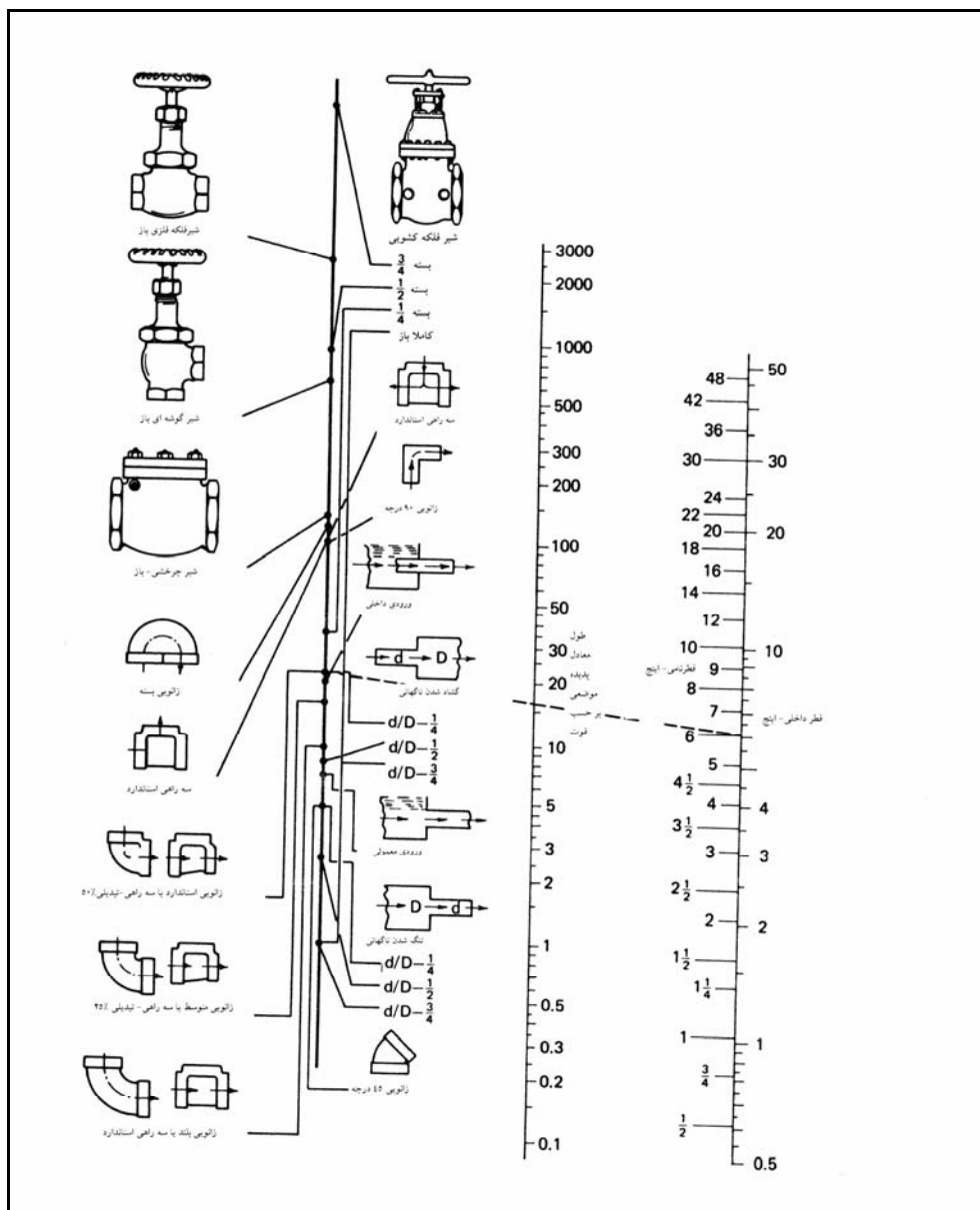
شکل ۶-۱- نمودار محاسبه‌ی طول معادل پدیده‌های موضعی.
