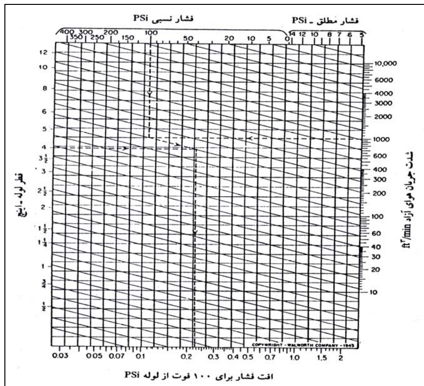
شکل ۵-۲- نمودار پوریفوی برای محاسبه‌ی افت فشار
