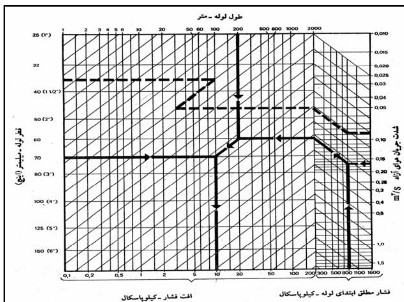
شکل ۵-۱- نمودار اطلس کوپکو برای محاسبه‌ی افت فشار در خط لوله.
