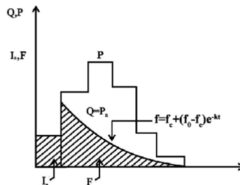
شکل ۴-۴ - تفکیک باران ( P ) به سه مولفه
