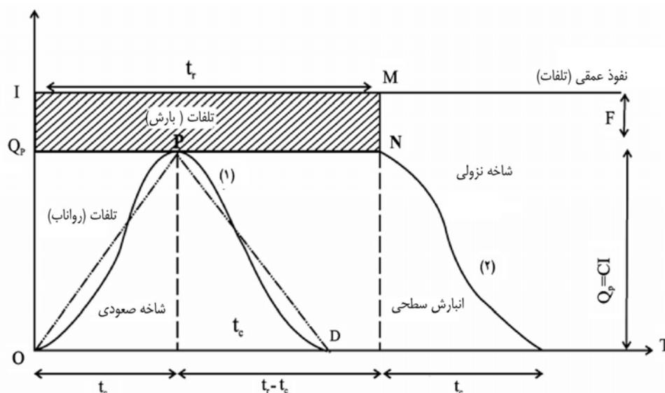
شکل ۱-۴- ویژگی‌های سیلاب در روش استدلالی
