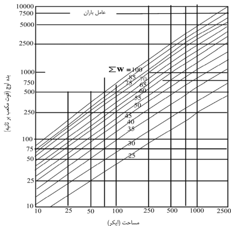
شکل ۴-۲- نمودار برآورد شدت اوج سیلاب با دوره بازگشت پنجاه سال ( Q_{50} )
