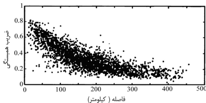
شکل ۳-۲- همبستگی نگار فاصله‌ای ۶۷ ایستگاه [۴۶]
