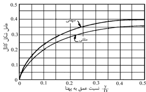
شکل ۱۲-۲- ضریب شکل (c) برای مقاطع مثلثی و سه‌می [۲۸]
