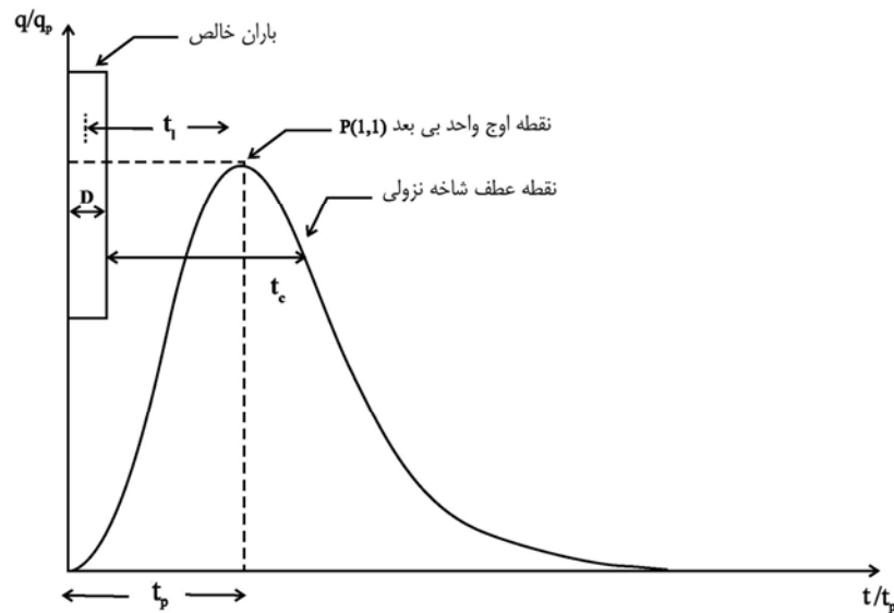
شکل ۴-۷- شکل آبنمود واحد و مشخصات آن
