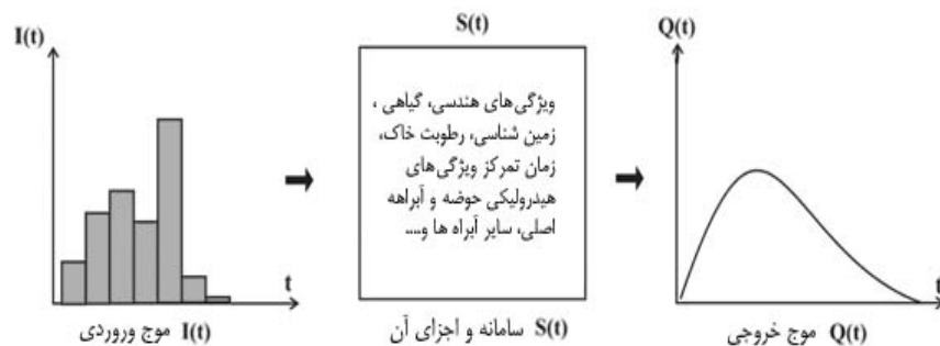
شکل ۲-۱- نمایش موج و سامانه برای یک حوضه آبریز نوعی
