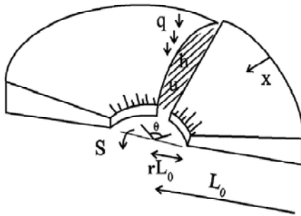
شکل ۲-۱۰-۱- مقطع همگرا [۳۵]
