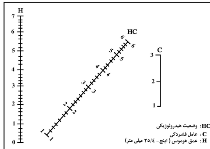
شکل ۲-۸- وضعیت هیدرولوژیکی زمین‌های جنگلی [۱]. عمق هوموس برحسب اینچ است.
