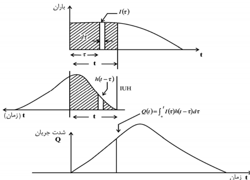
شکل ۴-۸- رابطه بین h(t-\tau) و Q(t) در انتگرال پیچشی
