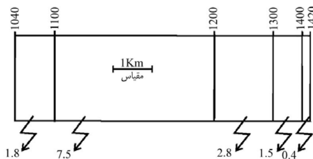
شکل پ.۱-۲- مستطیل معادل حوضه حلویی
