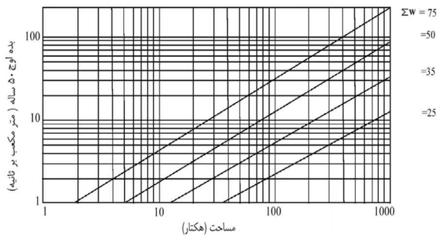
شکل ۴-۳- نمودار برآورد سیلاب پنجاه ساله ( Q_{50} ) به کمک مساحت حوضه (هکتار) و ضریب کوک ( W ) [۳۵، ۸]
