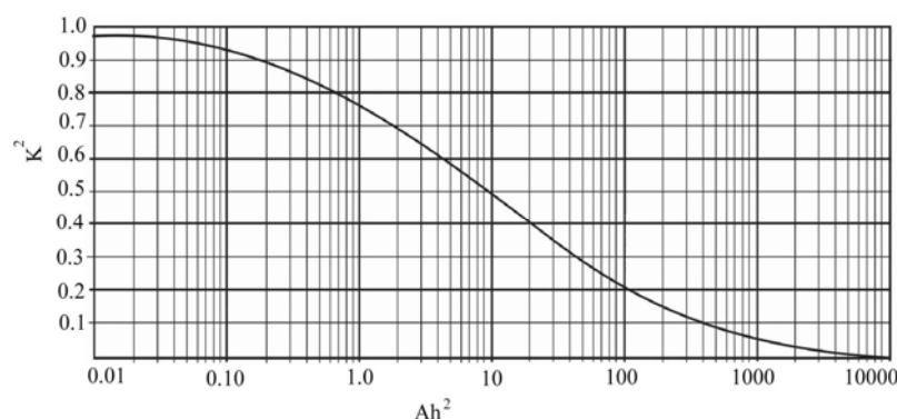
شکل ۳-۳- رابطه بین A/\lambda^2 و K^2 [۳۹]. دقت شود که h = \frac{1}{\lambda} است
