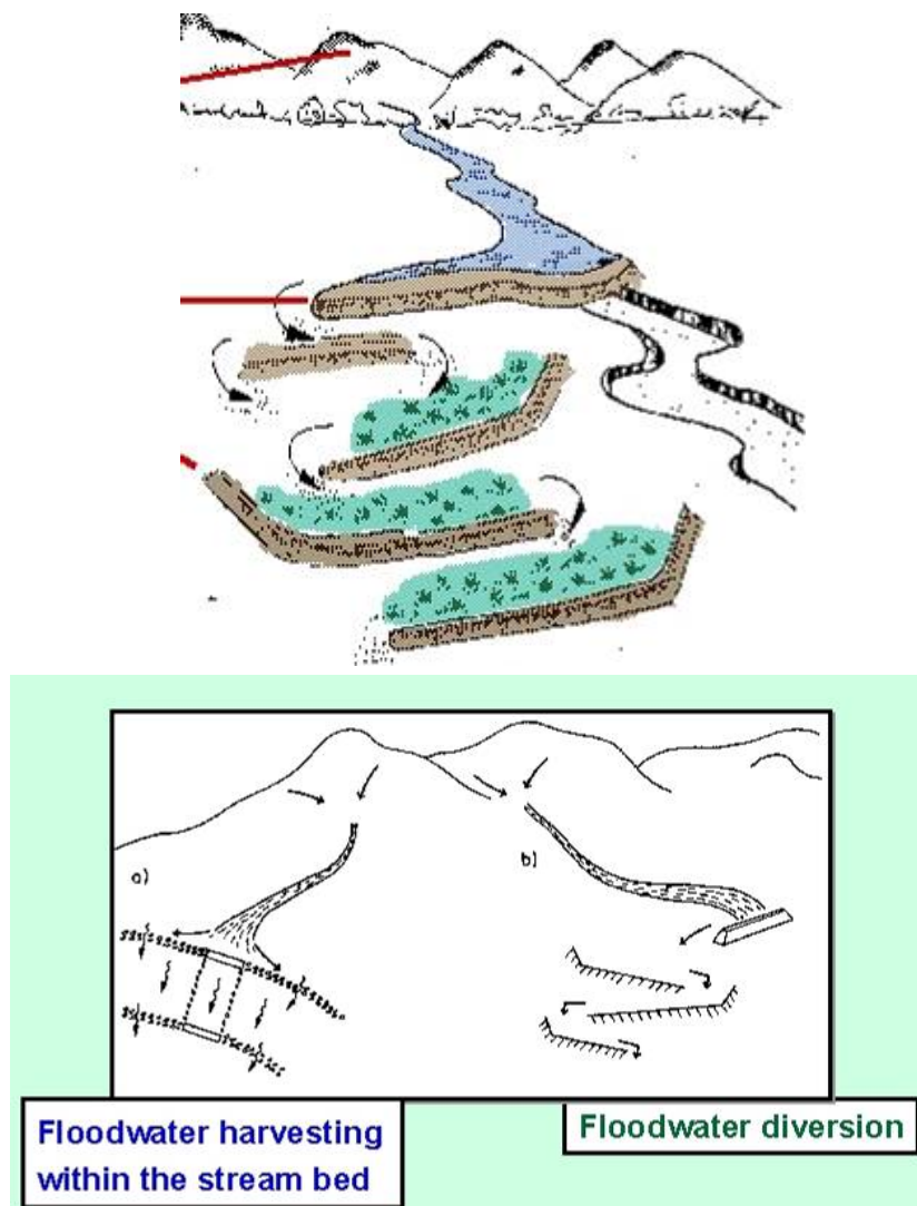
شکل شماره ۷-۱۲- سیستم جمع آوری سیلاب‌ها از بستر رودخانه و پخش سیلاب
