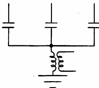
شکل ۲-۴: اتصال ستاره با ترانسفورماتور ولتاژ بین نقطه نوترال و زمین
