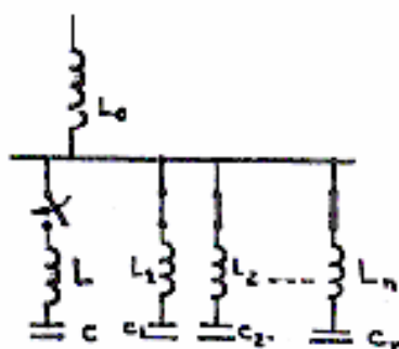
شکل ۱۳-۲: دیاگرام n بانک خازنی موازی
