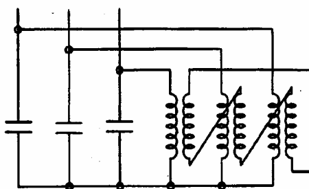
شکل ۲-۶: اتصال ستاره با نقطه نوترال زمین‌نشده همراه با ترانسفورماتورهای ولتاژ با اتصال مثلث باز
