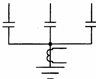
شکل ۲-۳: اتصال ستاره با نقطه نوترال زمین شده از طریق ترانسفورماتور جریان
