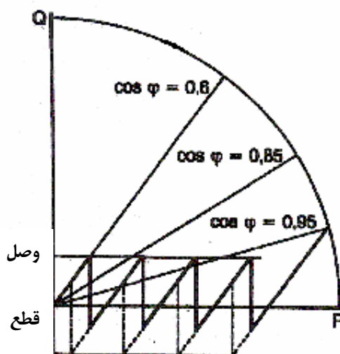
شکل ۲-۹: دیاگرام مربوط به تنظیم بانکهای خازنی در چهار مرحله (خطوط نقطه چین لحظات قطع را نشان می‌دهد.)
