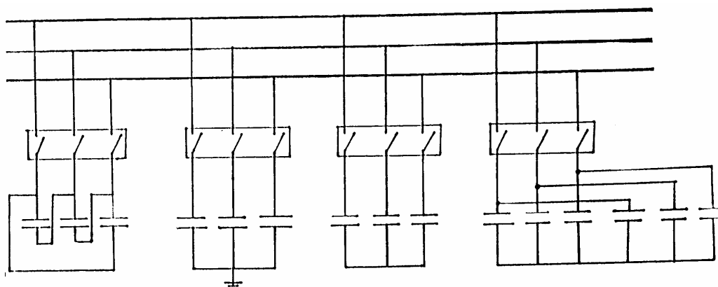
شکل ۱-۸: اتصال مختلف خازنهای موازی
