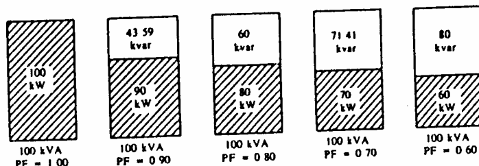
شکل ۴-۱: تغییرات توان راکتیو و اکتیو در اثر تغییرات ضریب توان
