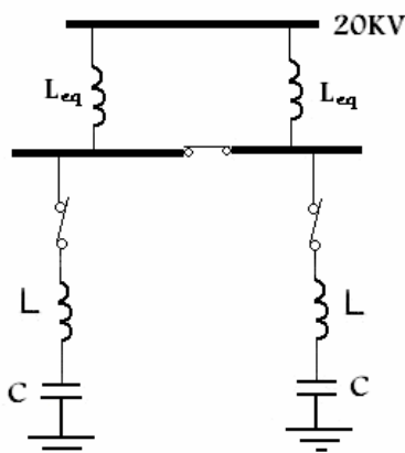
شکل ۲-۳: مدار معادل بانکهای خازنی متصل به شبکه به همراه راکتور سری
