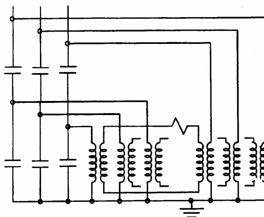
شکل ۲-۷: اتصال ستاره با نقطه نوترال زمین شده همراه با ترانسفورماتورهای ولتاژ نصب شده جهت اندازه‌گیری اختلاف ولتاژ
