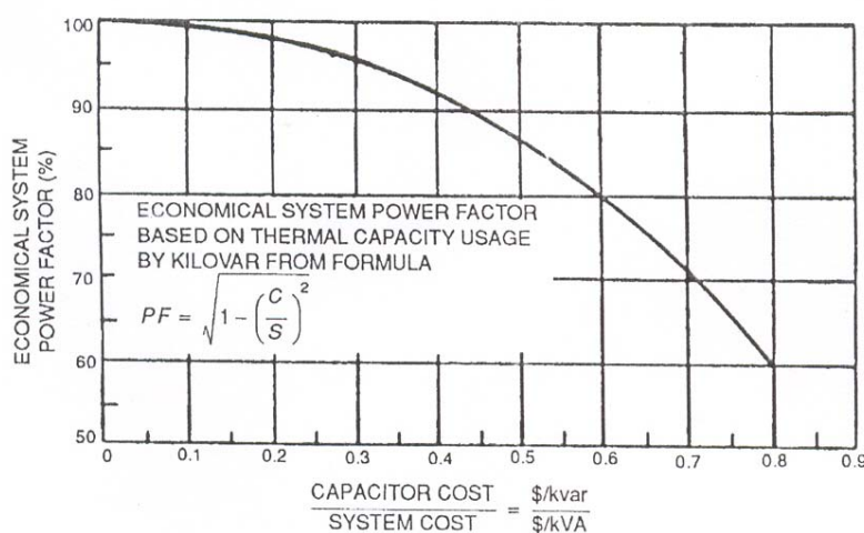
شکل ۷-۱: ضریب توان بهینه سیستم
