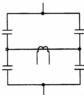
شکل ۲-۸: اتصال پل
