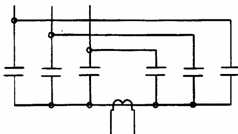
شکل ۲-۵: اتصال ستاره دوبل با نقطه نوترال زمین‌نشده
