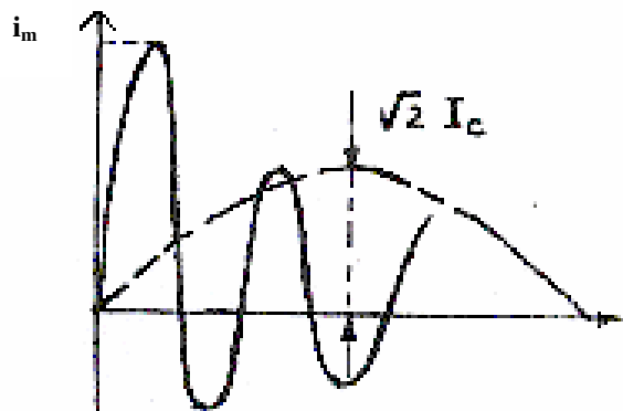
شکل ۲-۱۱: جریان در وصل یک بانک خازنی شارژ نشده (وصل در لحظه پیک ولتاژ شبکه)
