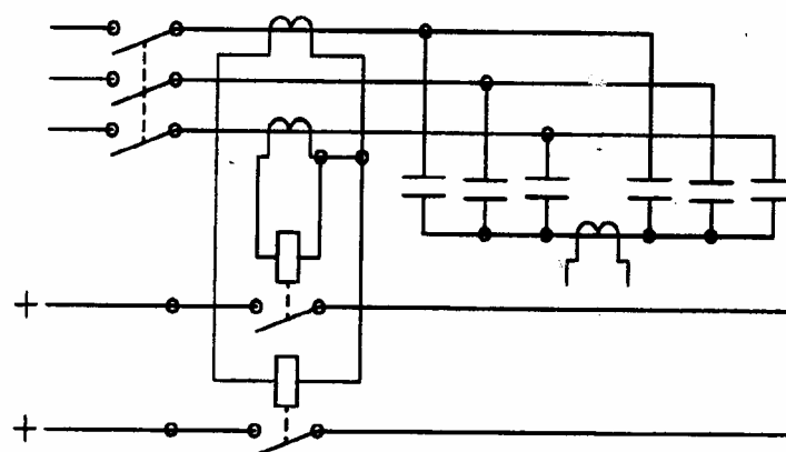
شکل ۲-۲: رله‌های اضافه جریان خط برای بانک خازنی زمین نشده
