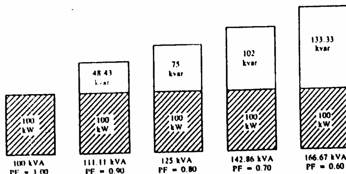
شکل ۱-۳: تغییرات توان ظاهری در اثر تغییر ضریب توان
