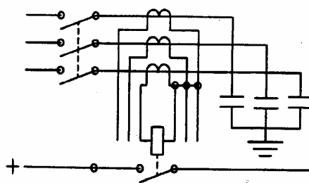
شکل ۲-۱: رله‌های اضافه جریان خط برای بانک خازنی زمین‌شده
