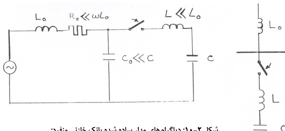
شکل ۲-۱۰: دیاگرام‌های مدار ساده شده بانک خازنی منفرد:
