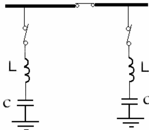
شکل ۲-۴: مدار معادل بانکهای خازنی نمونه طراحی
