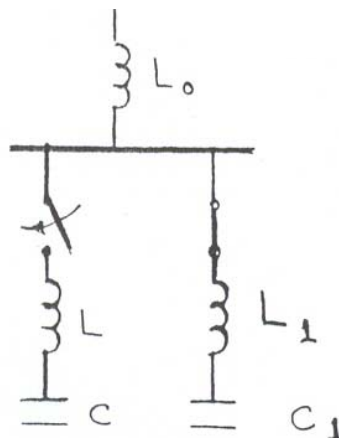
شکل ۲-۱۲: دیاگرام مدار دو بانک خازنی پشت به پشت
