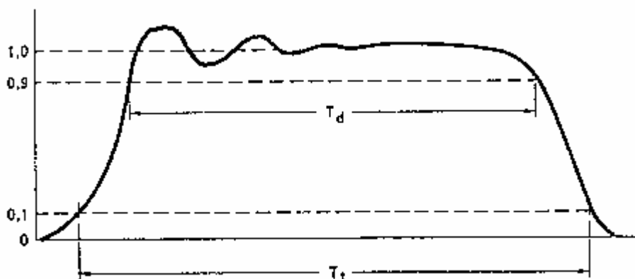
شکل ۱-۱۰: شکل موج ضربه جریان (ولتاژ) مستطیلی
