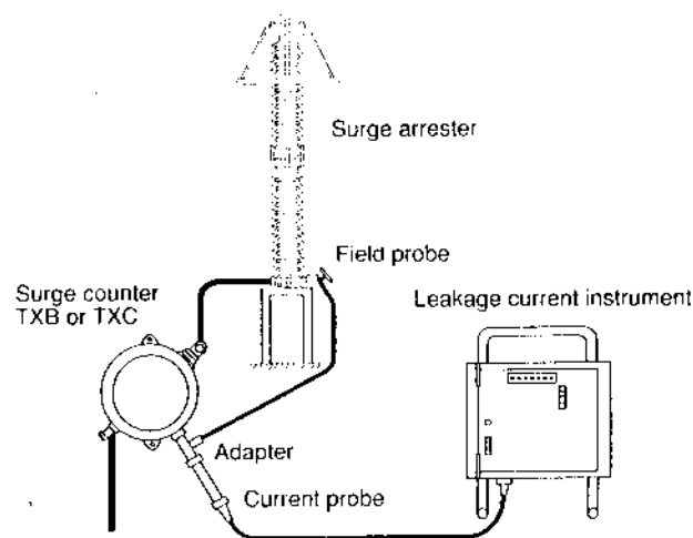
شکل ۴-۵: یک روش نوعی جهت اندازه‌گیری مؤلفه هارمونیک سوم جریان نشتی
