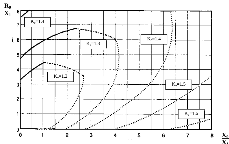
شکل ۲-۱۵: نسبت بین R_0/X_1 و X_0/X_1 برای مقادیر ثابتی از
