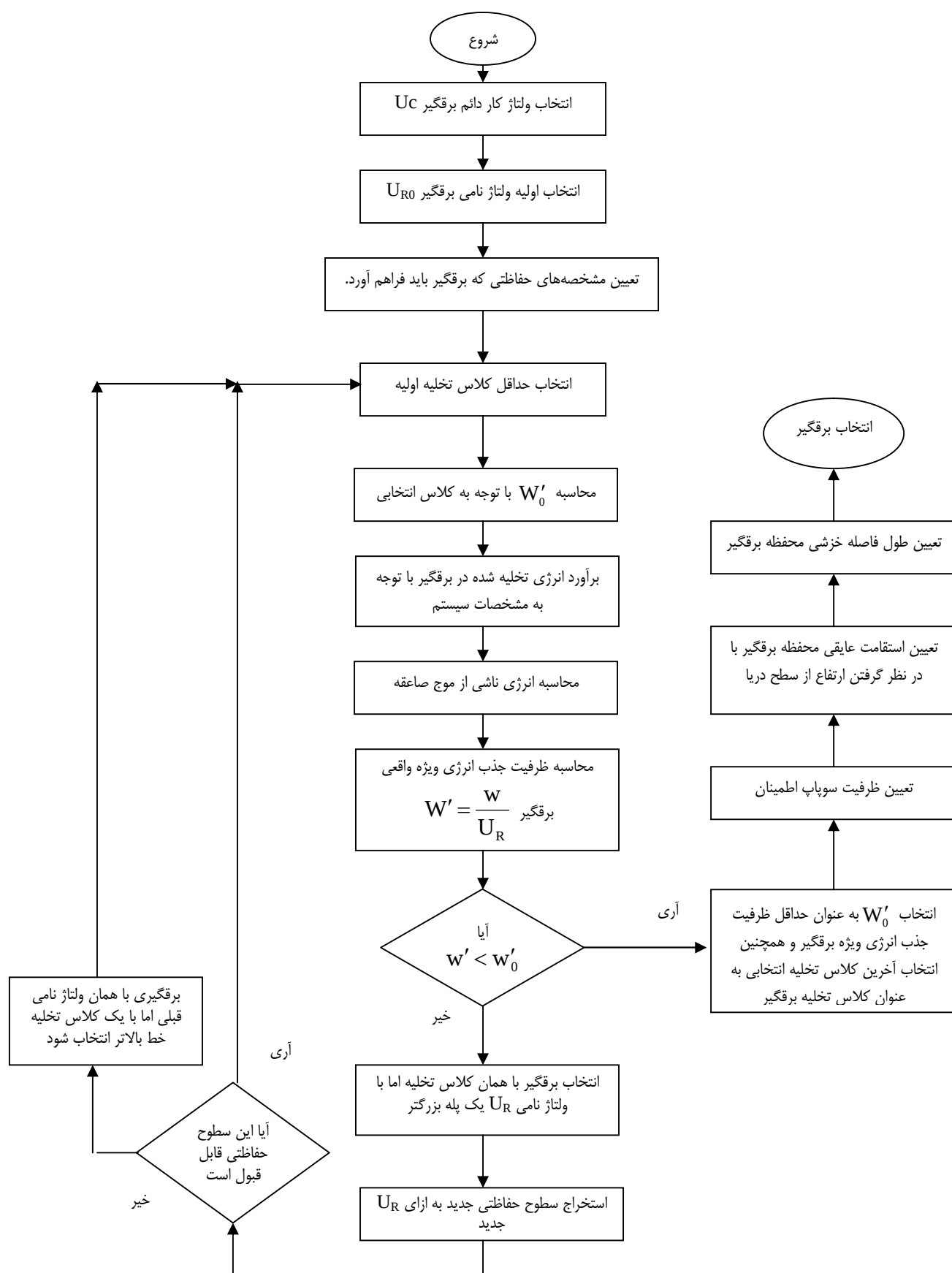
شکل ۲-۱: رویه گام به گام انتخاب پارامترهای برقگیر
