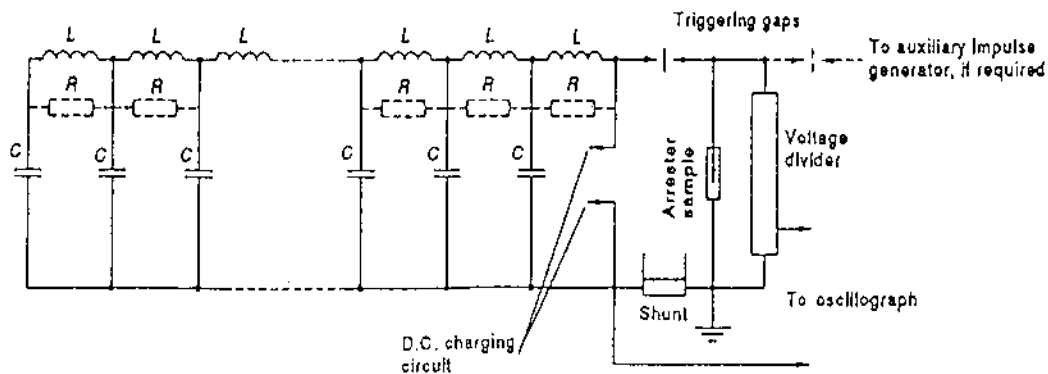
شکل ۳-۳: مدار نوعی مولد موج ضربه با ثوابت توزیع شده جهت انجام آزمون تحمل موج ضربه جریان طولانی مدت
