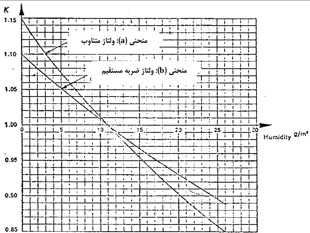
شکل ۲-۱۷: فاکتور K برای جداول (۲-۱۱)
