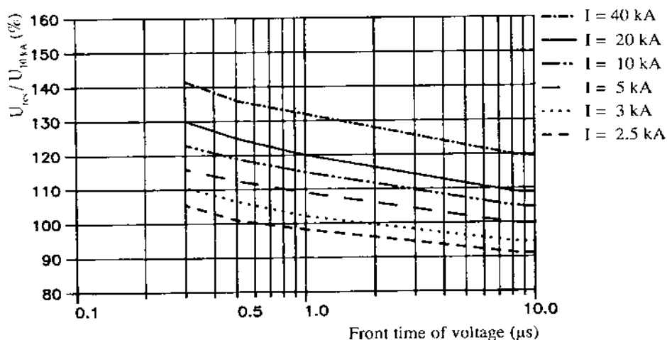
شکل ۲-۷: تغییر ولتاژ تخلیه برقگیر در اثر تغییر زمان پیشانی موج جریان صاعقه
