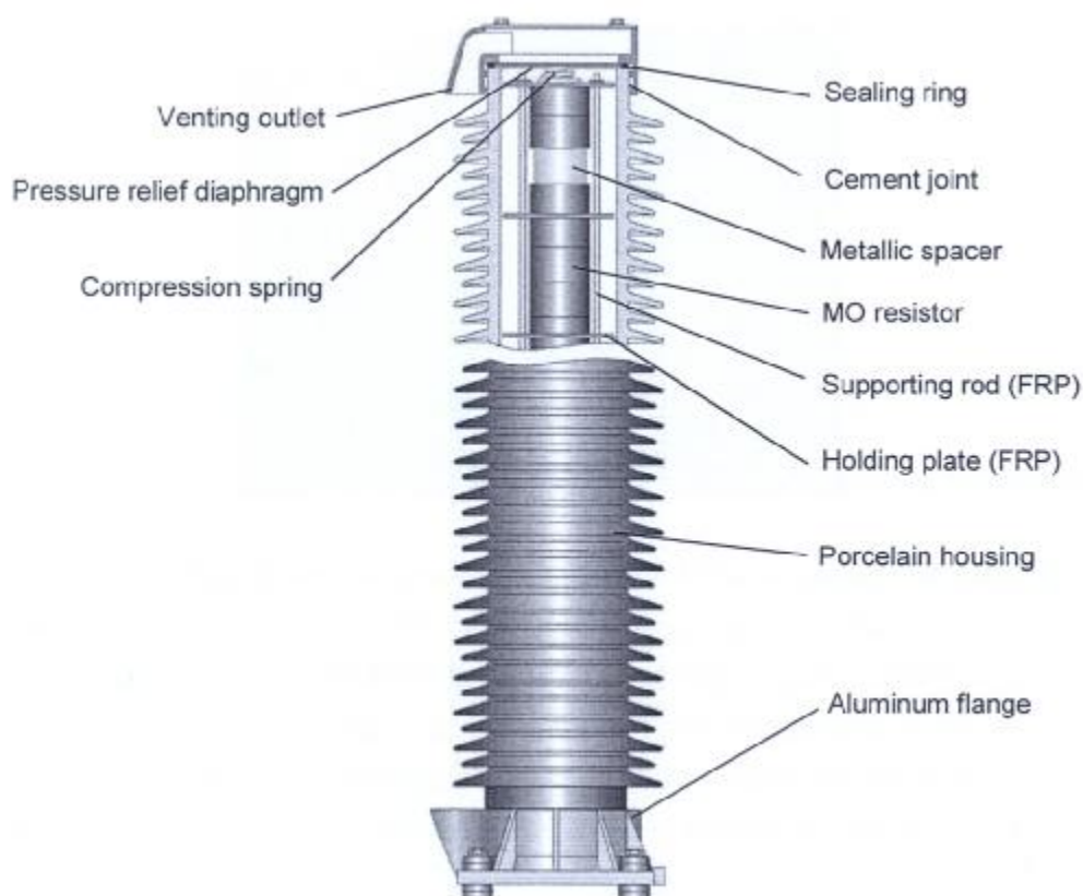
شکل ۲-۲۱: برش شماتیکی از برقگیر
