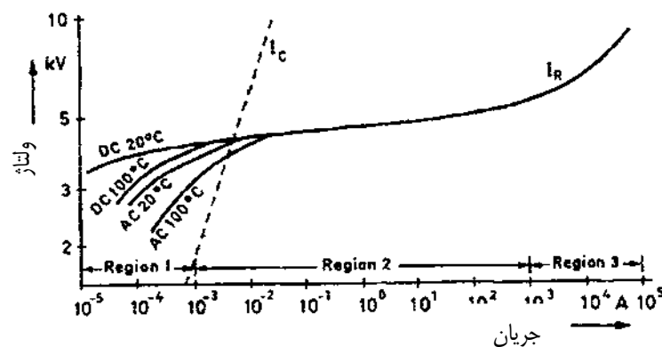
شکل ۴-۱: مشخصه ولت - آمپر دیسکهای اکسید فلز
