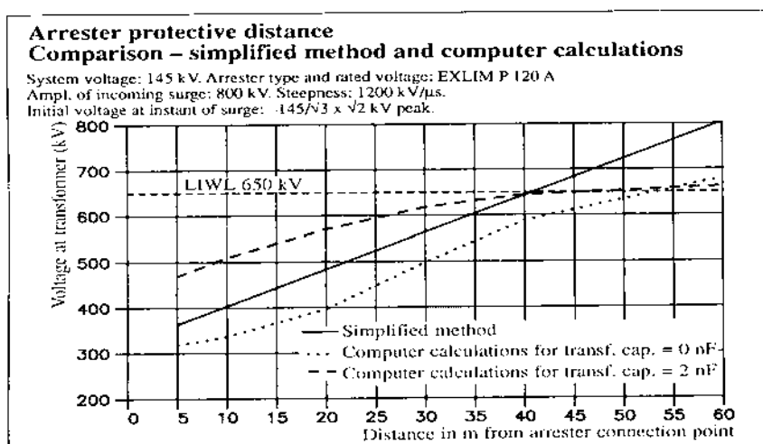
شکل ۲-۶: مقایسه روش محاسبه ساده با محاسبه کامپیوتری فاصله حفاظتی برقگیر
