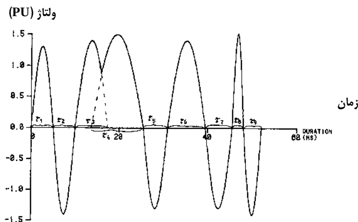
شکل ۲-۱۶: مثالی از TOV متشکل از چندین فرکانس مختلف متفاوت از فرکانس قدرت
