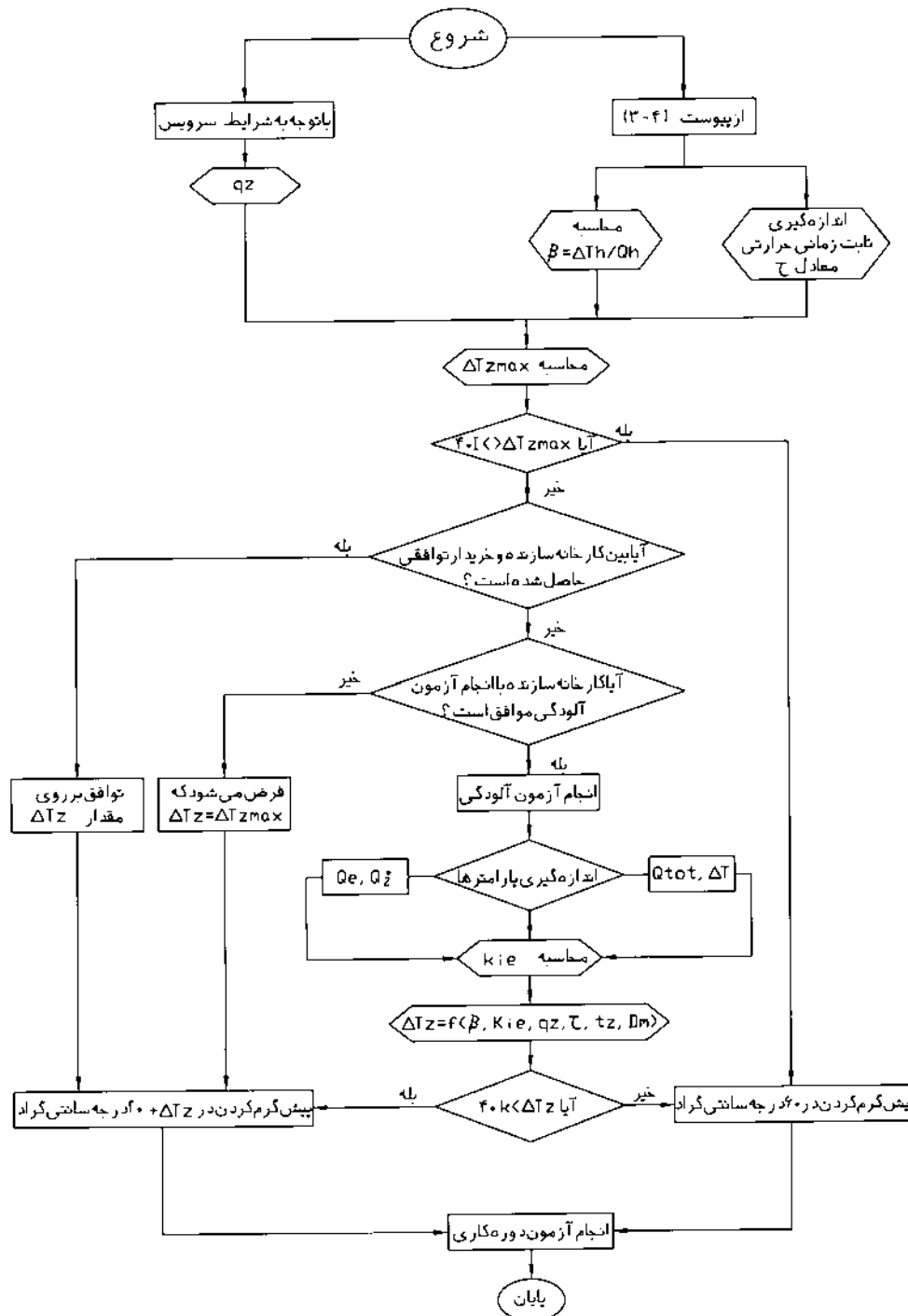
شکل ۳-۲: فلوچارت تعیین دمای شروع آزمون دوره کاری
