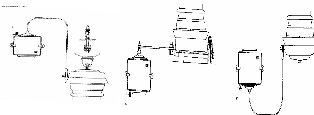
شکل ۴-۴: سه گونه مختلف اتصال ترمینال زمین برقگیر به ترمینال مخصوص شمارنده موج ضربه
