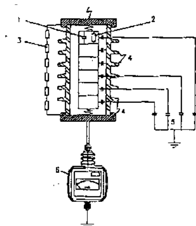
شکل ۱-۷: مدار نوعی جهت ثبت تخلیه و جریان نشتی برقگیر
