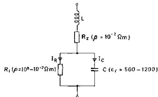
تسکل ۳-۱: مدار معادل دیسکهای اکسید فلز برفکیر
