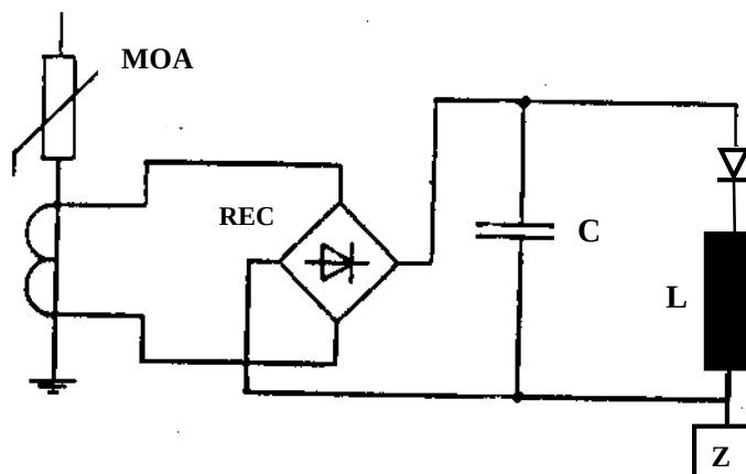
شکل ۱-۶: مدار نوعی دیگری جهت ثبت تخلیه از طریق برقگیر
