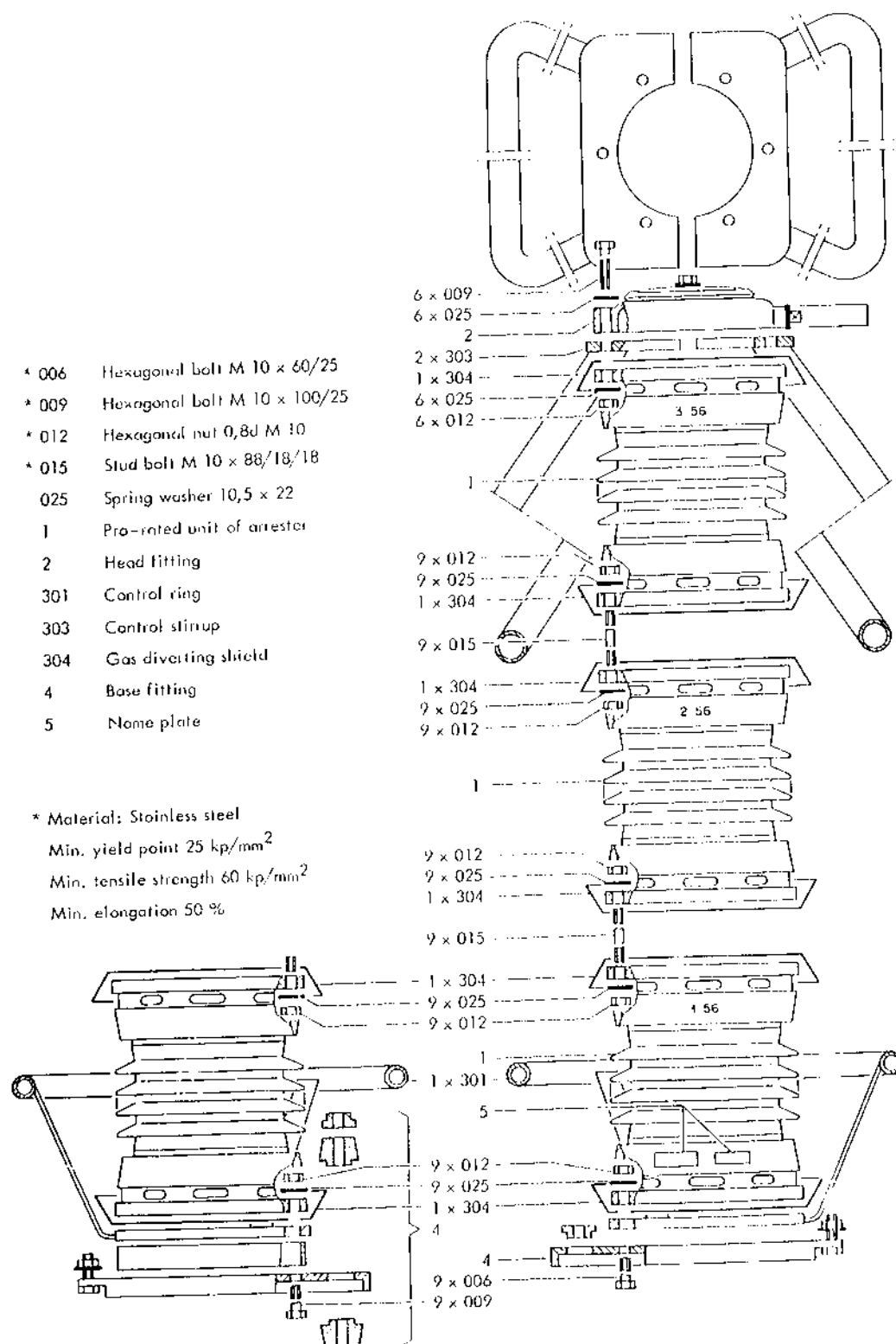
شکل ۴-۲: مونتاژ یک نمونه برقگیر
