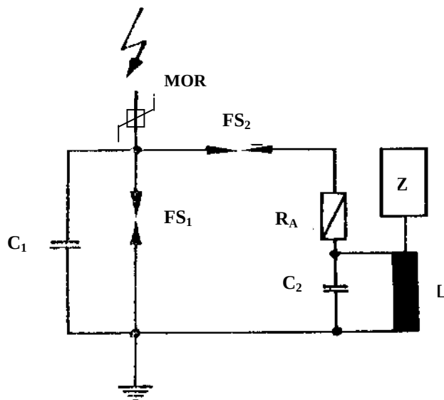
شکل ۱-۵: مدار نوعی جهت ثبت تخلیه از طریق برقگیر
