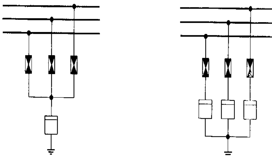
شکل ۴-۳: دو فرم متداول برای نصب شمارنده موج ضربه در سیستم‌های سه‌فاز
