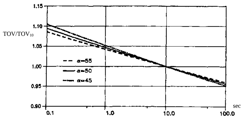
شکل ۳-۲: منحنی قابلیت TOV بر حسب زمان برای یک برقگیر با \alpha های متفاوت
