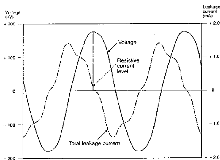
شکل ۴-۶: شکل موجهای جریان نشتی و ولتاژ اعمالی به یک برقگیر ZnO نمونه
