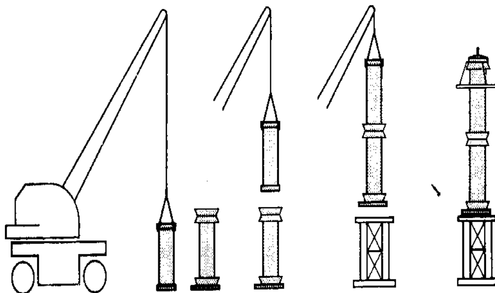
شکل ۴-۱: نحوه مونتاژ و سوار کردن برقگیر
