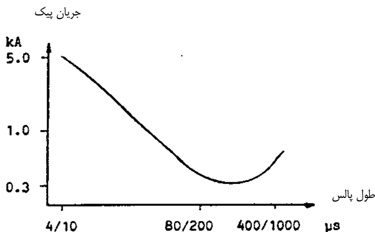
شکل ۸-۱: معیار عدم افزایش در شماره‌های برقگیر
