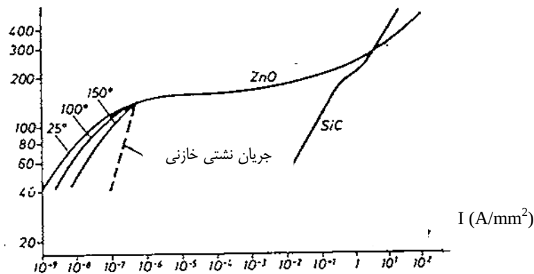
شکل ۱-۲: مشخصه ولت - آمپر برقگیرهای ZnO و SiC
