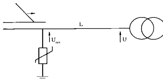
شکل ۵-۲: دیاگرام ساده‌ای جهت ارزیابی اثر فاصله برقگیر از موضع تحت حفاظت
