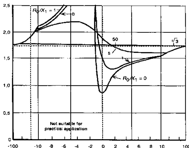
شکل ۲-۱۱: ضریب اتصال زمین براساس X_0/X_1 به ازای R_1 \ll X_1 , R=0
