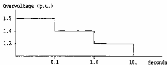
شکل ۴-۲: مثالی از منحنی اضافه ولتاژهای موقت ظاهر شده در یک سیستم ۴۰۰ کیلوولت
