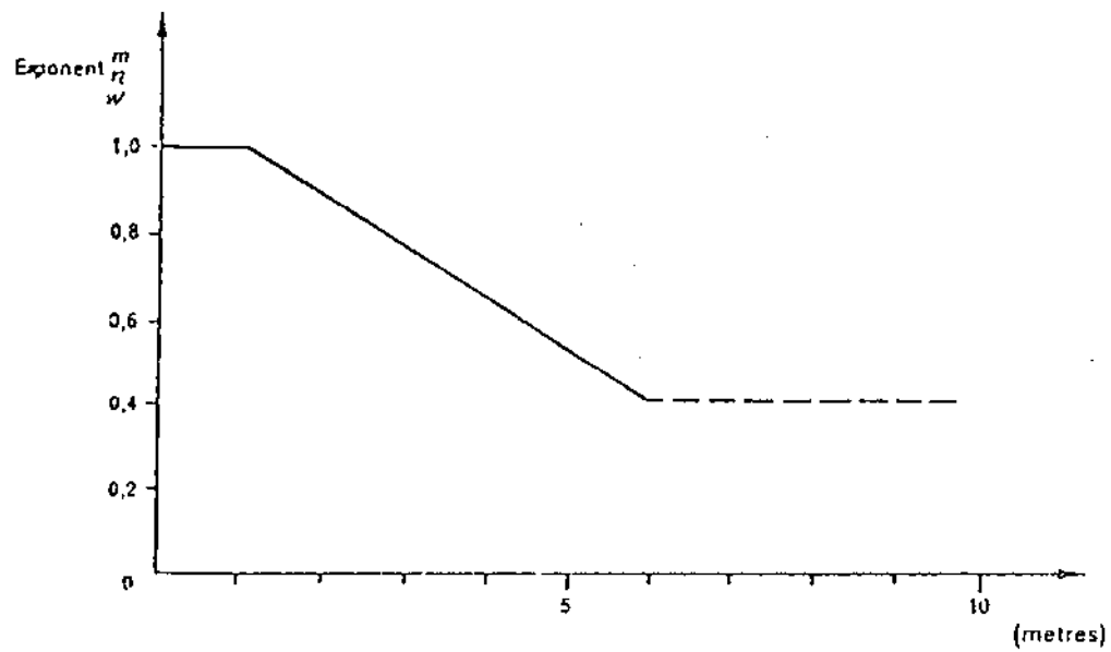
شکل ۲-۱۸: ضرایب m , n و w برای الکترودهای جدول (۲-۱۱) برحسب فاصله بین الکترودها
