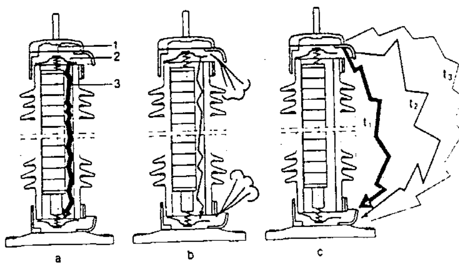
شکل ۲-۱۹: نمایش شماتیک از عملکرد سوپاپ اطمینان برقگیر در مواقع اضافه بار شدن آن
