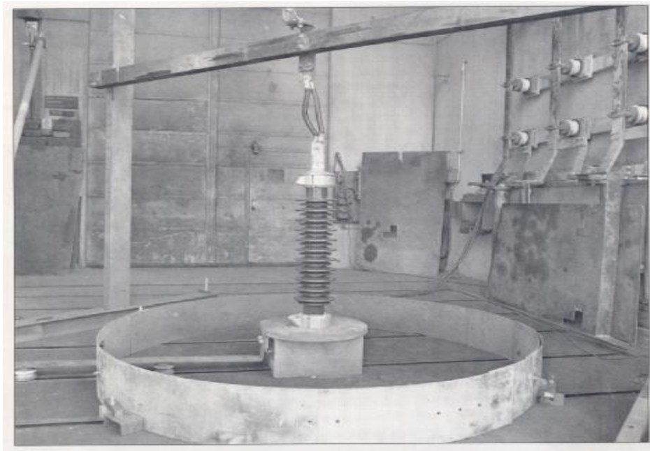
شکل ۳-۱: نحوه انجام آزمون سوپاپ اطمینان برقگیر
