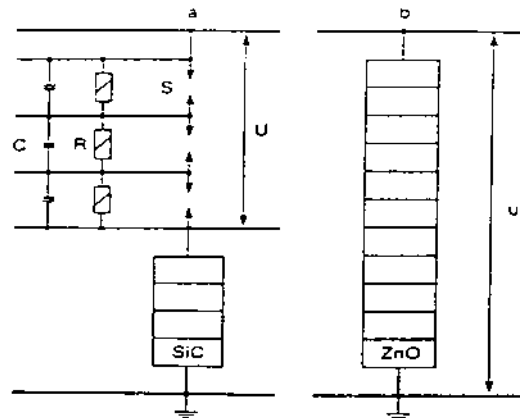
شکل ۱-۱: ساختمان شماتیک برقگیرهای ZnO و SiC
