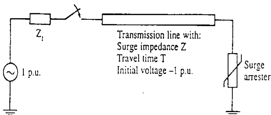
شکل ۲-۹: یک مدل ساده تکفاز جهت برآورد تقریبی از ظرفیت جذب انرژی ویژه برقگیر
