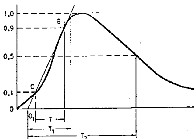
شکل ۹-۱: شکل موج ضربه جریان و پارامترهای مشخصه آن
