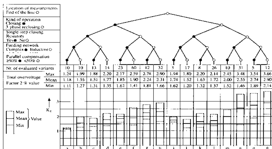
شکل ۱۰-۲: فاکتور ارزیابی حداکثر ولتاژ ظاهر شده در سیستم براساس مشخصات سیستم
