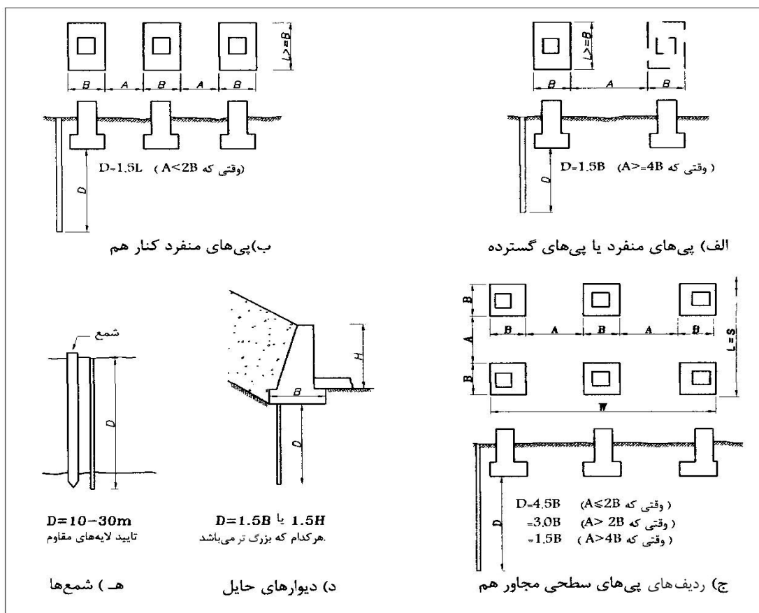
شکل ۴-۱- عمق پیشنهادی گمانه‌ها برای پی‌های نقطه‌ای [۱]
