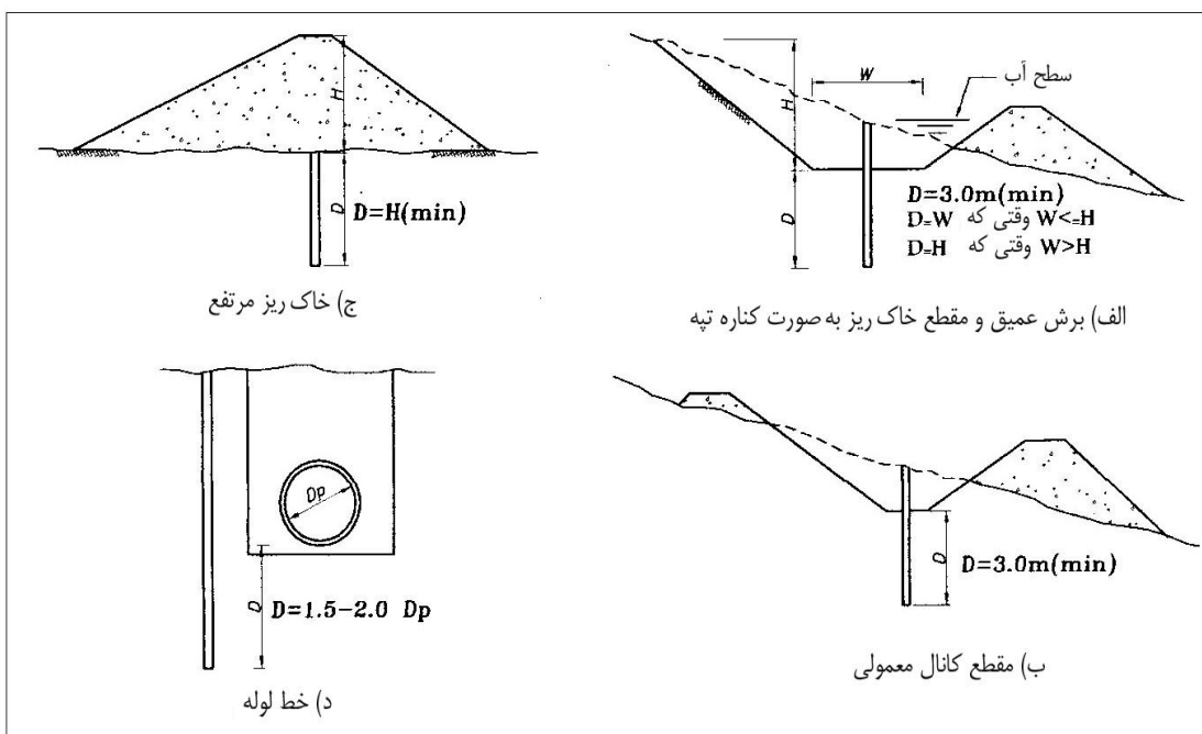
شکل ۴-۲- عمق پیشنهادی گمانه‌ها برای سازه‌های نواری [۱]
