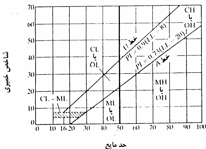
شکل ۳-۲: نمودار خمیری
