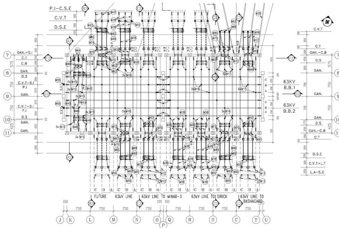
شکل ۵-۲: نقشه جانمایی پستی که در بخش ۲-۵ آورده شده است.
