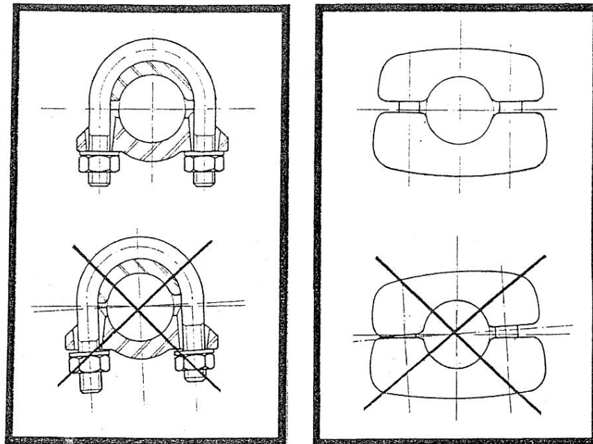
شکل ۴-۲: وضعیت قرارگیری صحیح و ناصحیح روپندها و پیچ‌های U شکل رابط
