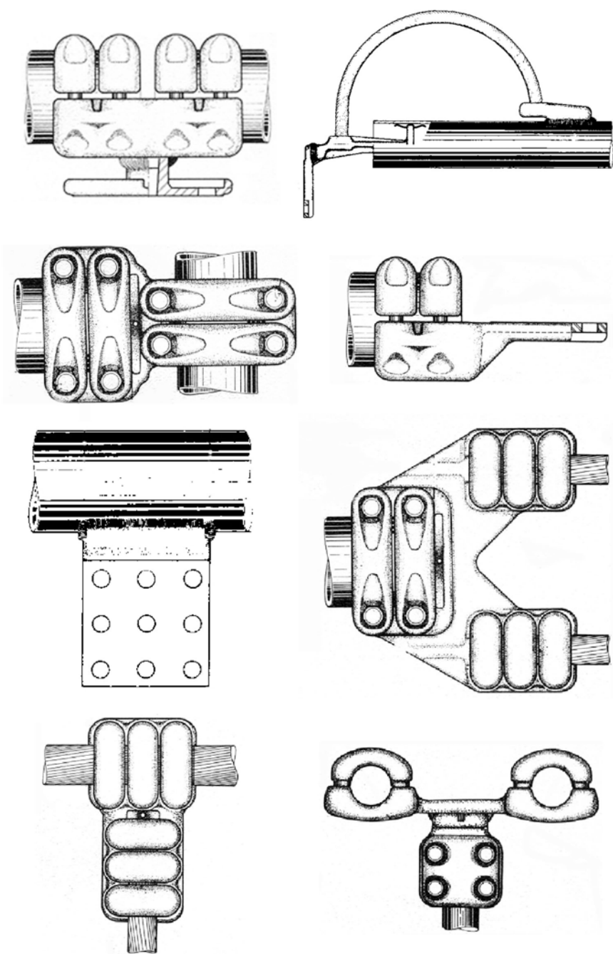
شکل ۱-۱: نمونه‌هایی از براق‌آلات مورد استفاده در پست‌های فشار قوی (ادامه)
