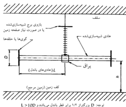
شکل ۳-۱۶: آرایش آزمونی نمونه _ ساختار آویزی
