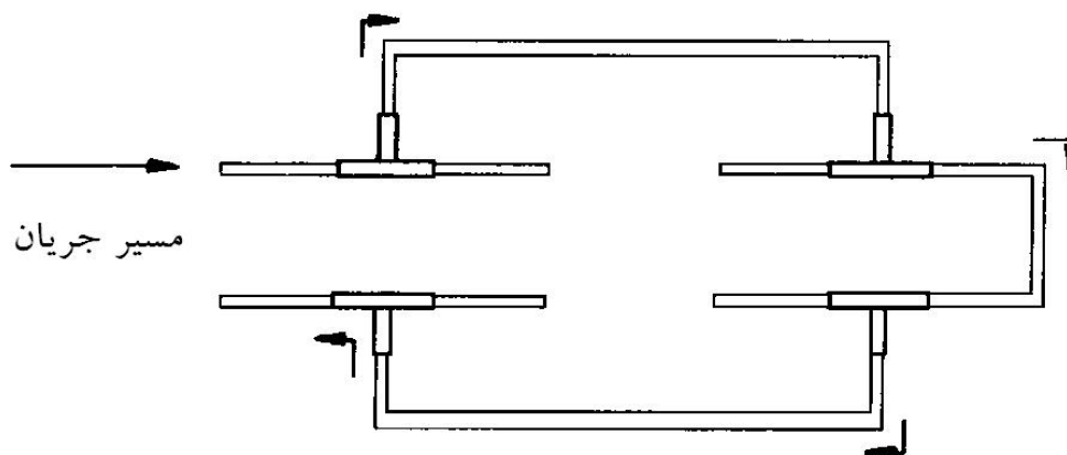
شکل ۳-۲۷: مدار نمونه جهت دوره حرارتی مفصل‌های رده B - سائز هادی‌های اصلی و انشعابی یکسان می‌باشد.
