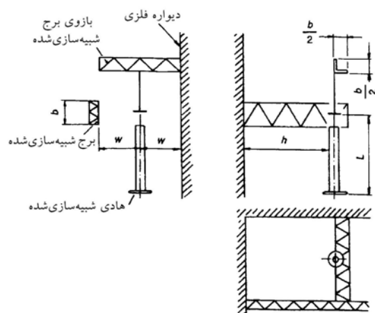
شکل ۳-۱۴: آرایش آزمونی برای ساختار کششی به صورت آویزان از سقف (آرایش سوم)
