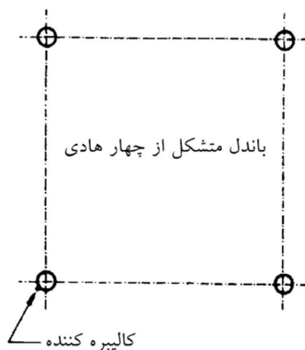
شکل ۳-۳۴: محل قرارگیری کالیبره کننده در یک باندل چهارتایی
