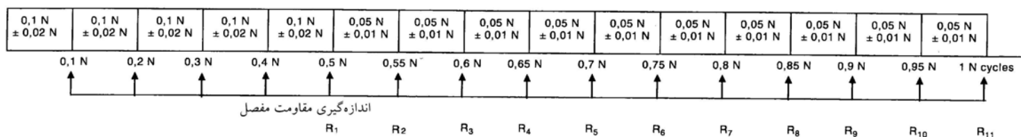
شکل ۳-۳۰: جزئیات توالی کامل آزمون دوره حرارتی
