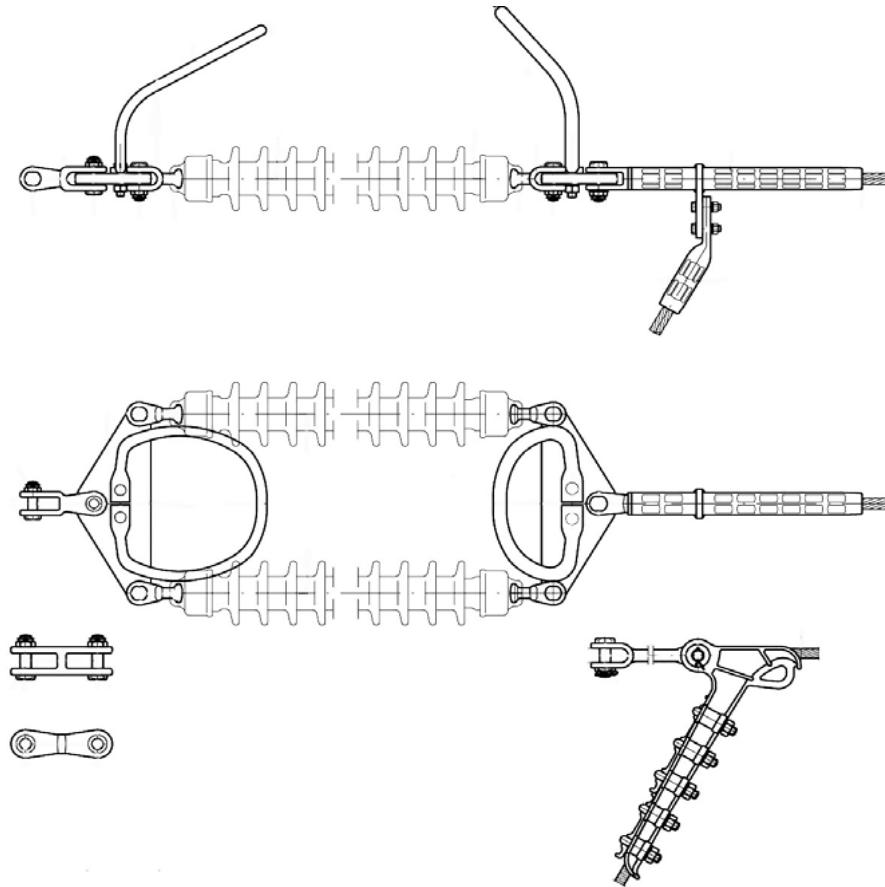
نقشه شماره ۱۲: زنجیره مقره کششی دو ستونه جهت یک هادی فاز و متشکل از واحد مقره‌های یکپارچه
