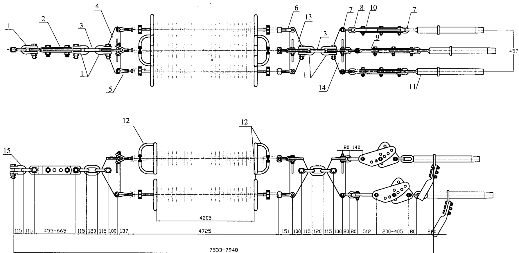
نقشه شماره ۱۷: زنجیره مقره کششی دو ستونه جهت سه هادی فاز و متشکل از واحد مقره‌های بشقابی
