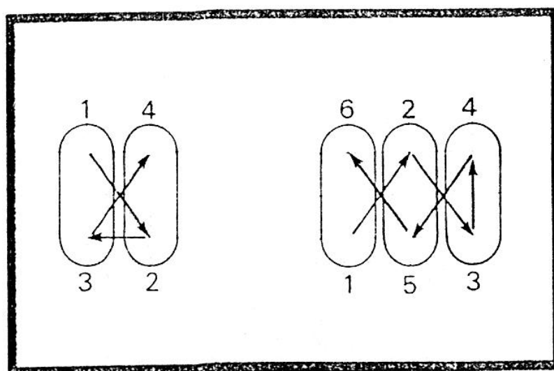
شکل ۴-۱: توالی صحیح سفت‌نمودن پیچ‌های رابط
