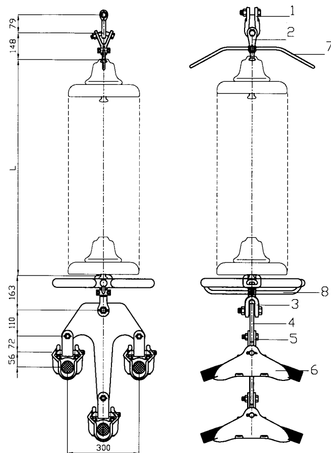
نقشه شماره ۵: زنجیره مقره آویزی یک ستونه جهت سه هادی فاز و متشکل از واحد مقره‌های بشقابی
