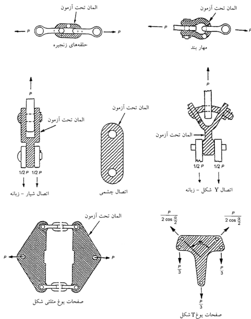
شکل ۳-۱: یراق آلات مجموعه مقره و یراق آلات سیم زمین (این دیاگرام‌ها نمونه‌ای از روش‌های بارگذاری یراق آلات در هنگام انجام آزمونهای مکانیکی را نشان می‌دهند).
