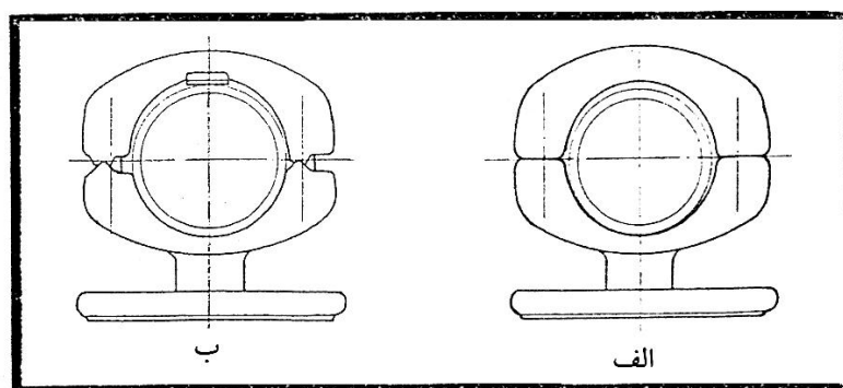
شکل ۴-۶: وضعیت صحیح قرارگیری روبندها در رابط‌های لغزشی الف: روبند معمولی _ ب: روبند دو منظوره (ثابت یا لغزشی)
