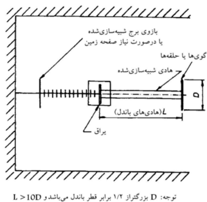
شکل ۳-۱۷: آرایش آزمونی نمونه _ ساختار کششی
