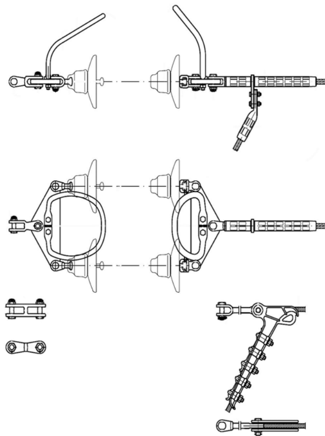
نقشه شماره ۱۱: زنجیره مقره کششی دو ستونه جهت یک هادی فاز و متشکل از واحد مقره‌های بشقاب‌ی
