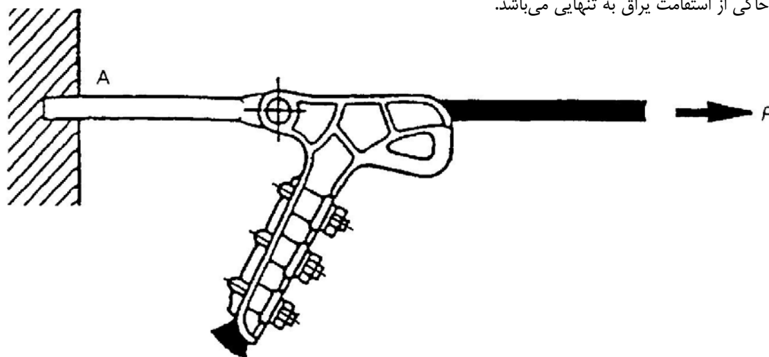
شکل ۳-۸: یک روش نوعی از نحوه انجام آزمون نیروی تخریب مکانیکی و نیروی شکست مکانیکی بر روی کلمپهای کششی و مفصل‌های کششی
