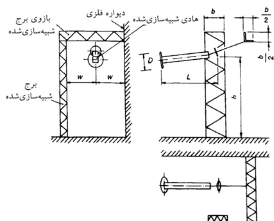
چ شکل ۳-۱۳: آرایش آزمونی برای ساختار کششی (آرایش سوم)
