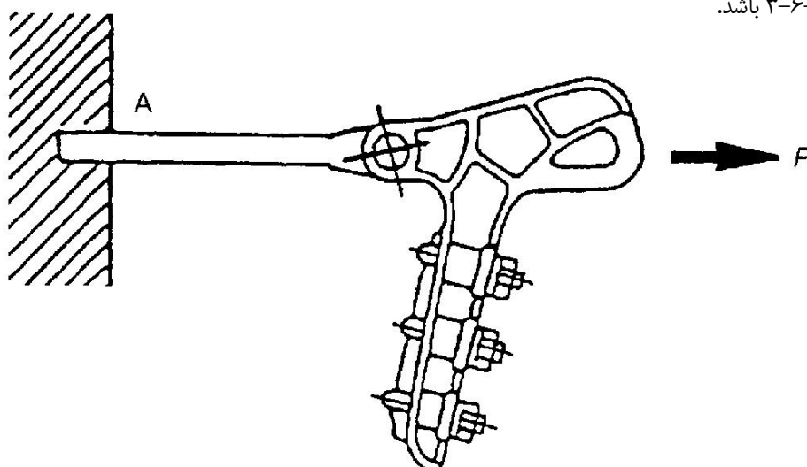
شکل ۳-۹: یک روش نوعی از نحوه انجام آزمون نیروی تخریب و نیروی شکست مکانیکی بر روی قطعه الحاقی تعبیه شده جهت استفاده در هنگام نصب
