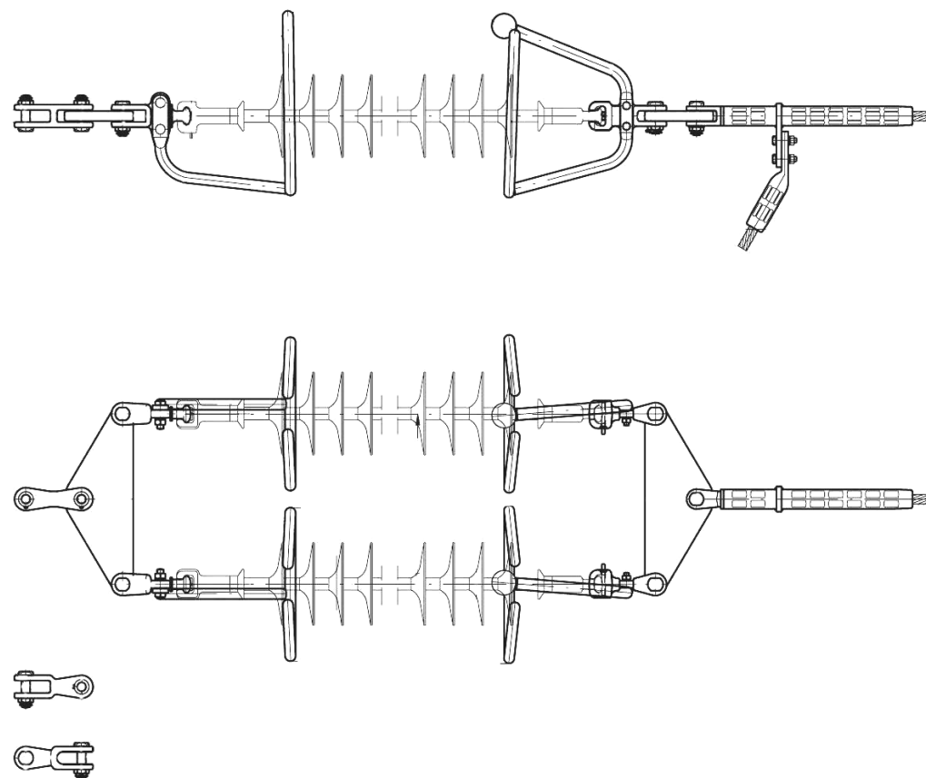
نقشه شماره ۱۳: زنجیره مقره کششی دو ستونه جهت یک هادی فاز و متشکل از واحد مقره‌های ترکیبی
