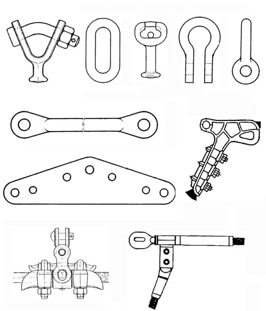
شکل ۱-۱: نمونه‌هایی از یراق‌آلات مورد استفاده در پست‌های فشار قوی
