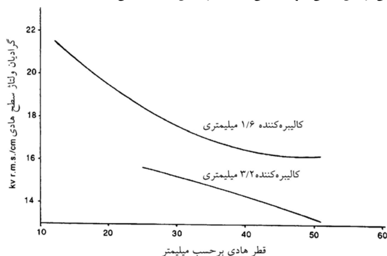
شکل ۳-۳۳: گرادیان نوعی آغاز کروناي مثبت برای کالیبره‌کننده‌های مختلف و سائزهای متفاوتی از هادی
