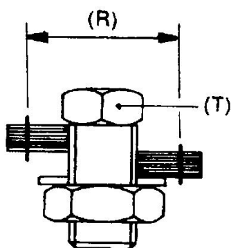
شکل ۲۴-۳: مفصل از نوع پیچی
