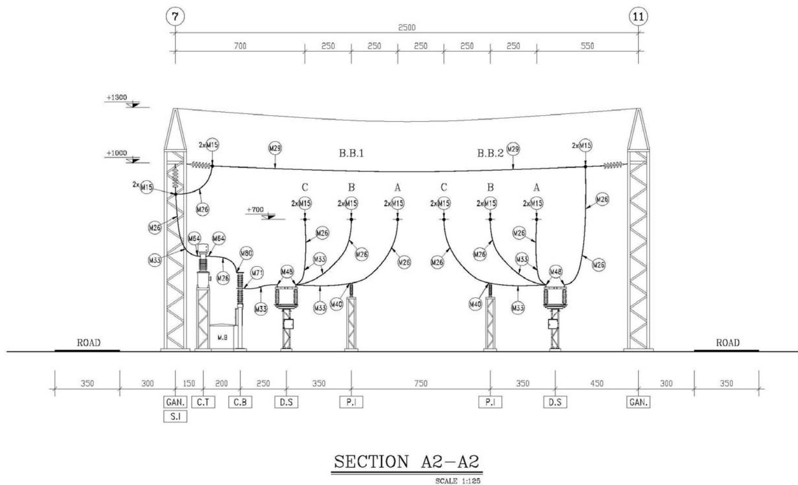
شکل ۲-۱۱: نقشه‌های مقاطع پستی که در بخش ۲-۵ آورده شده است.
