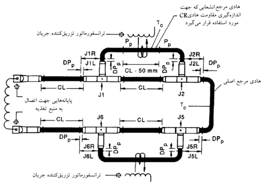
شکل ۳-۲۶: مدار نمونه جهت دوره حرارتی مفصل‌های رده B - سائز هادی‌های اصلی و انشعابی با هم متفاوت می‌باشد.
