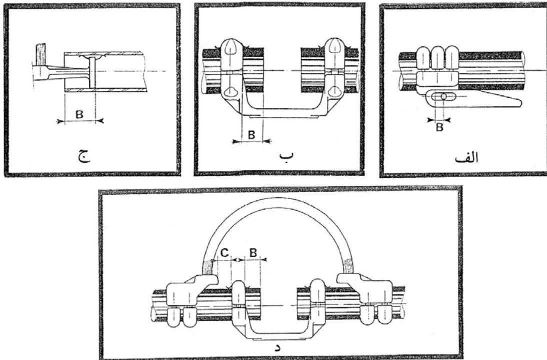
شکل ۴-۷: وضعیت قرارگیری هادی لوله‌ای و کلمپ‌های اتصالی در رابط‌های انبساطی
