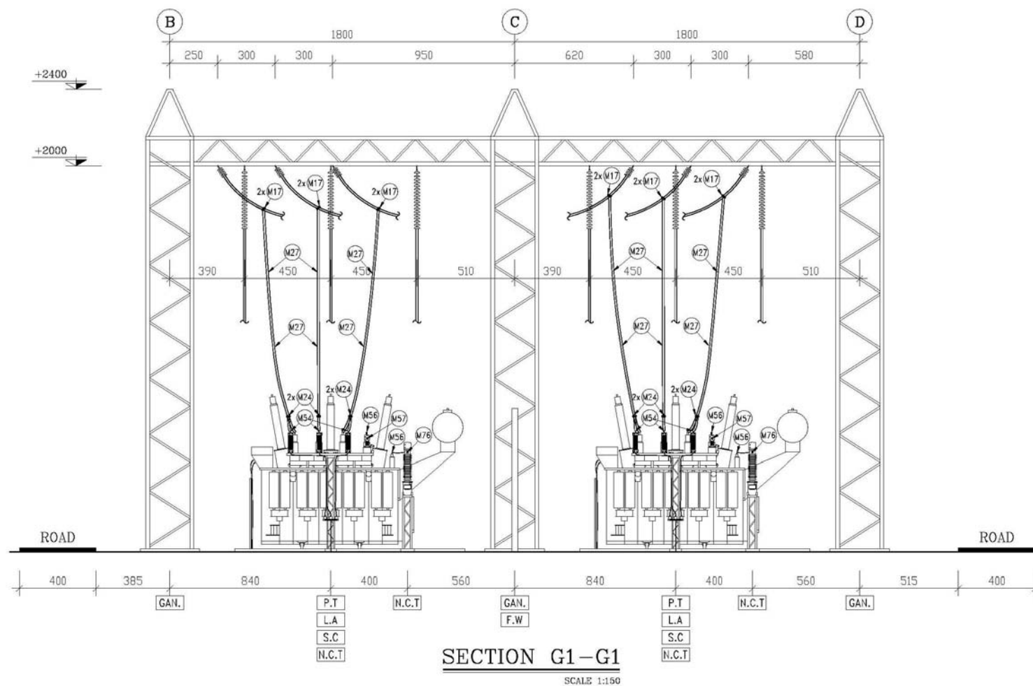
شکل ۲-۱: نقشه‌های مقاطع پستی که در بخش ۲-۵ آورده شده است.
