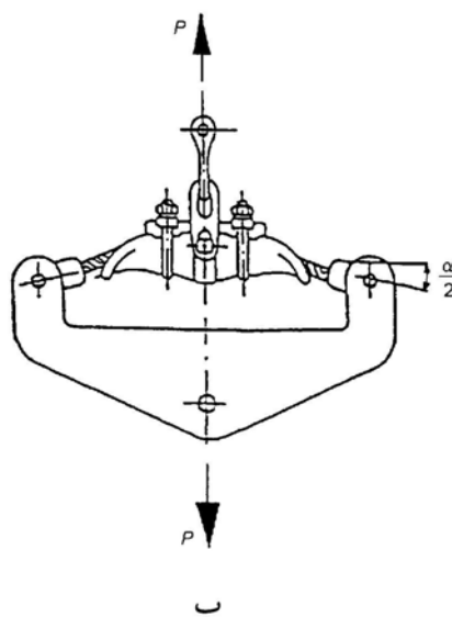
شکل ۳-۳: نحوه اعمالی نیرو در آزمون نیروی تخریب و نیروی شکست مکانیکی مربوط به کلمپ آویزی
