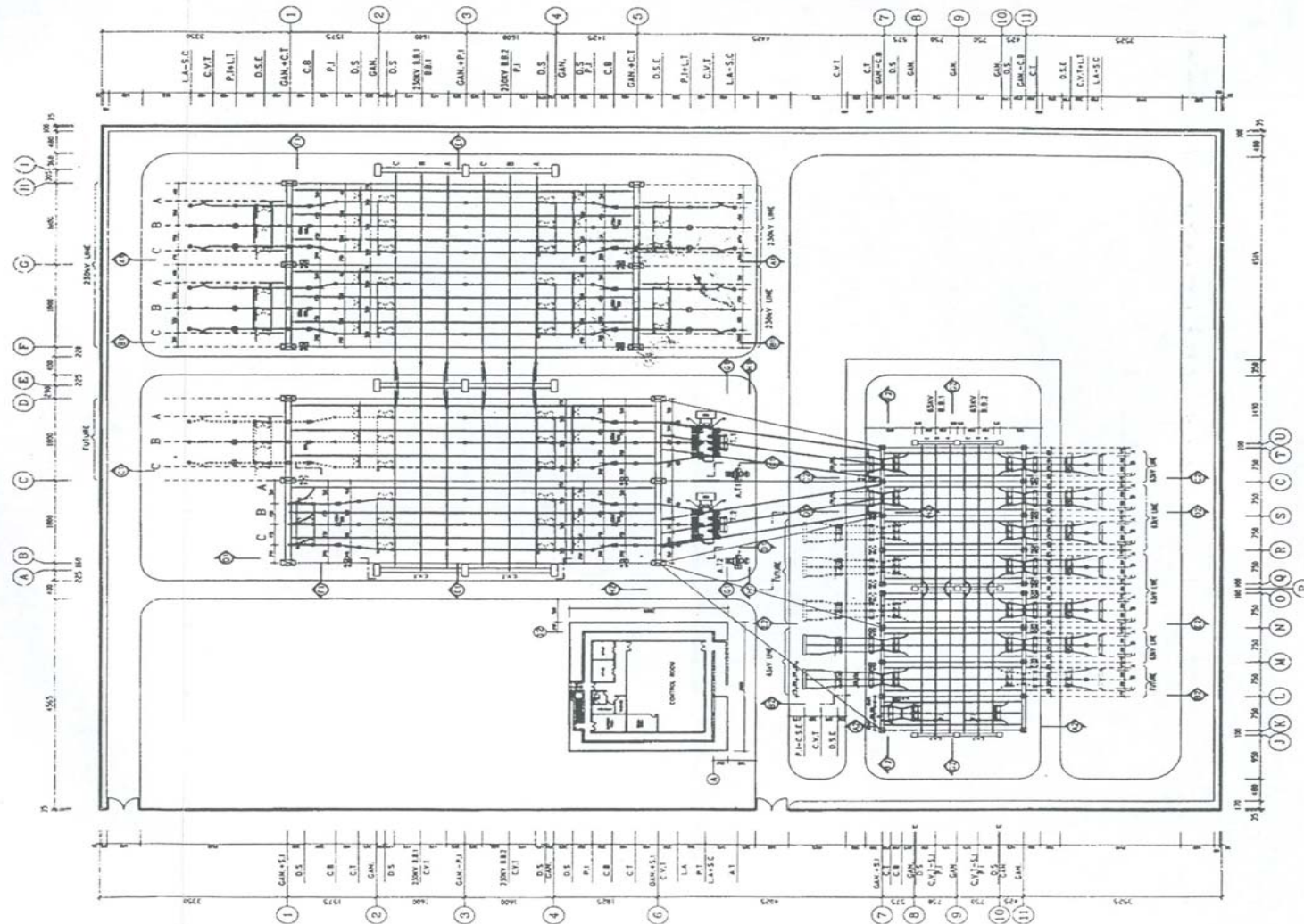
شکل ۲-۱: نقشه جانمایی پستی که در بخش ۲-۵ آورده شده است.
