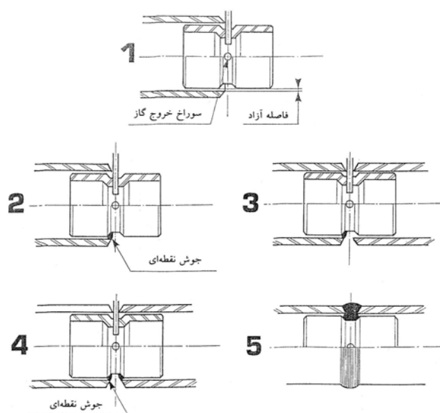
شکل ۳-۴: نحوه اتصال دو هادی لوله ای از طریق عملیات جوشکاری
