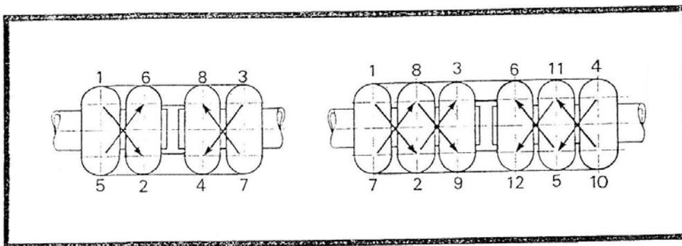
شکل ۴-۵: توالی صحیح سفت‌نمودن پیچ‌ها در دو نمونه رابط ثابت کوپلر
