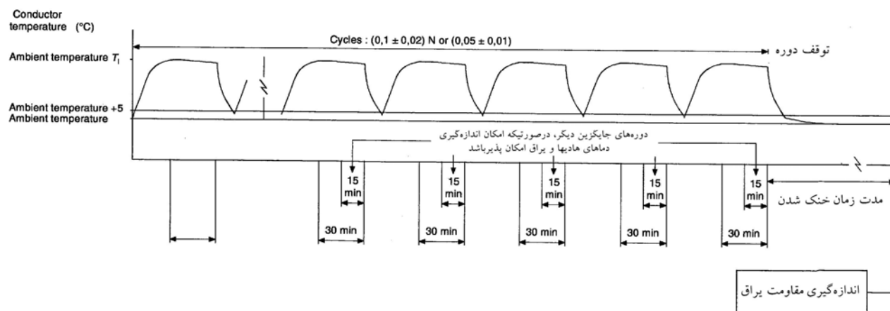
شکل ۳-۳۱: توالی \frac{N}{10} یا \frac{N}{20} دوره‌های آزمون دوره حرارتی
