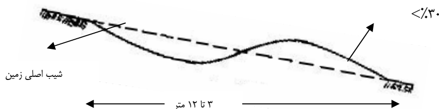
شکل شماره ۷ - نمونه‌ای از بانکت انحنایی شکل
