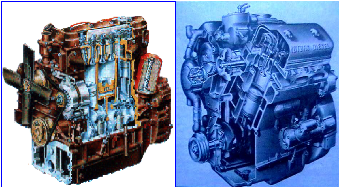
شکل شماره ۴-۴- دسته بندی موتورها براساس آرایش سیلندرها (سمت راست: یک نمونه موتور خورجینی با آرایش ۷ شکل سیلندرها - سمت چپ: یک نمونه موتور ردیفی با آرایش سیلندرها)
