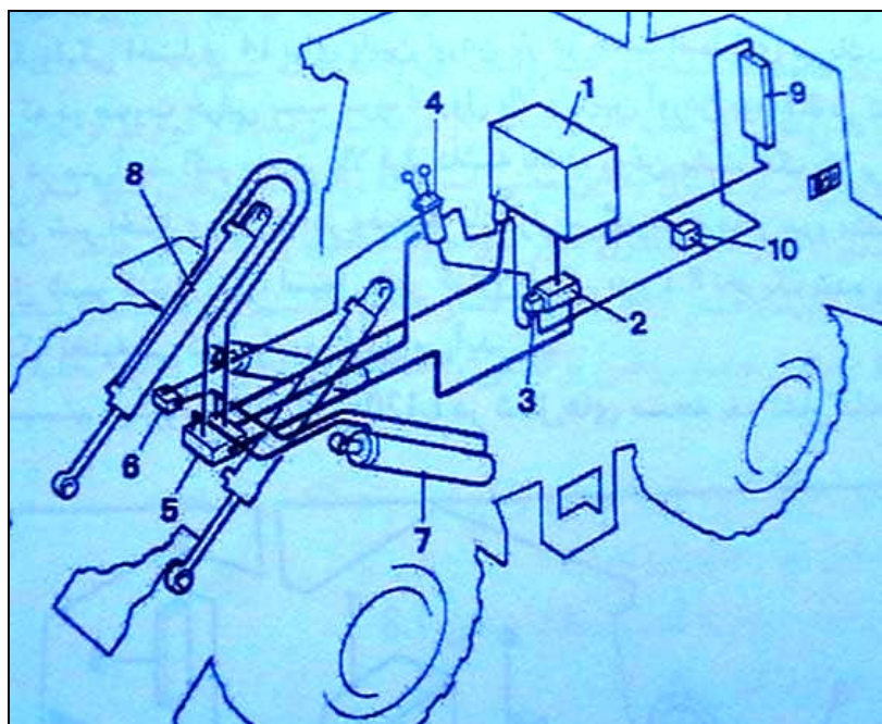
شکل شماره (۴-۳۹) - اجزاء تشکیل دهنده سیستم هیدرولیک کار در یک لودر:
