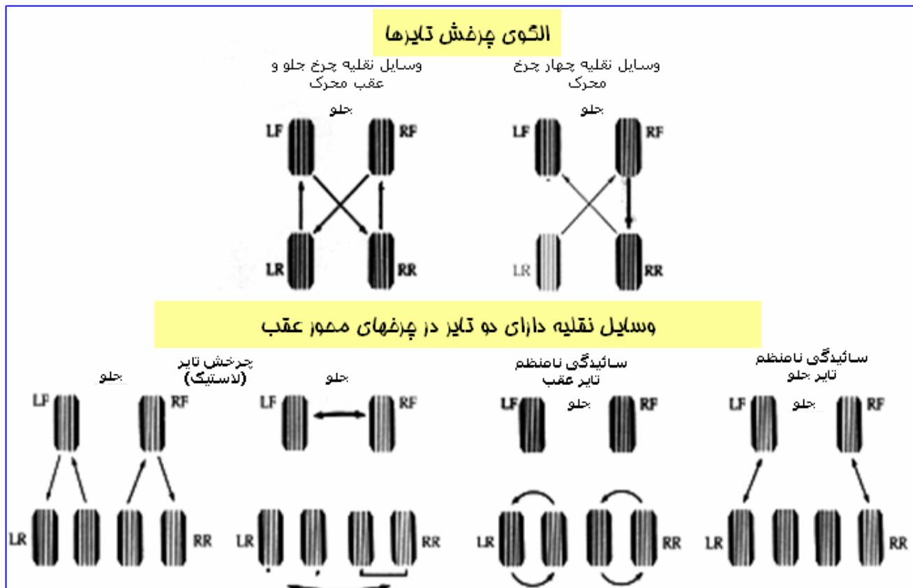
شکل شماره (۵-۱۵)- نحوه چرخش لاستیکها (تایرها)
