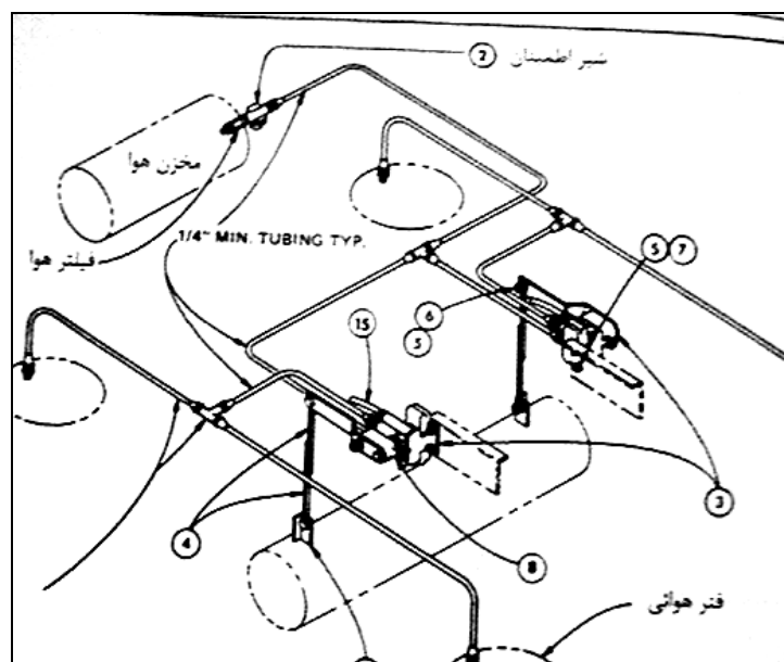
شکل شماره (۴-۵۹)- مدار سیستم تعلیق هوایی
