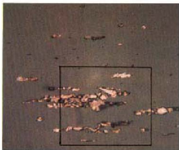
Fig. 1.5.1 Opt. M. 225X 100µm
