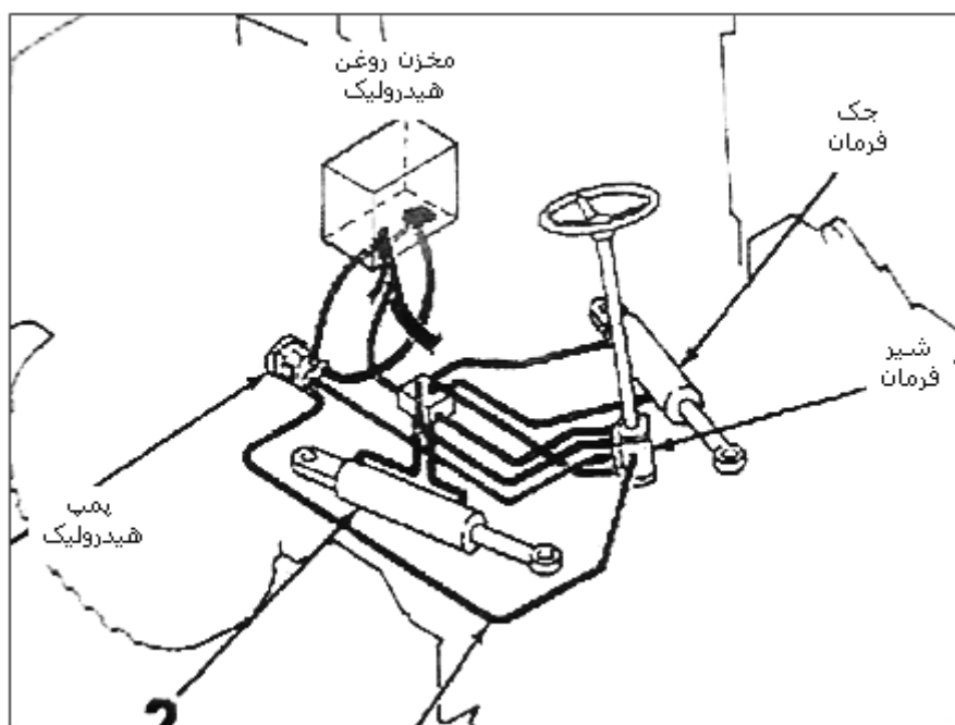
شکل شماره (۴-۵) - شماتیک سیستم فرمان هیدرولیک و اجزاء تشکیل دهنده آن
