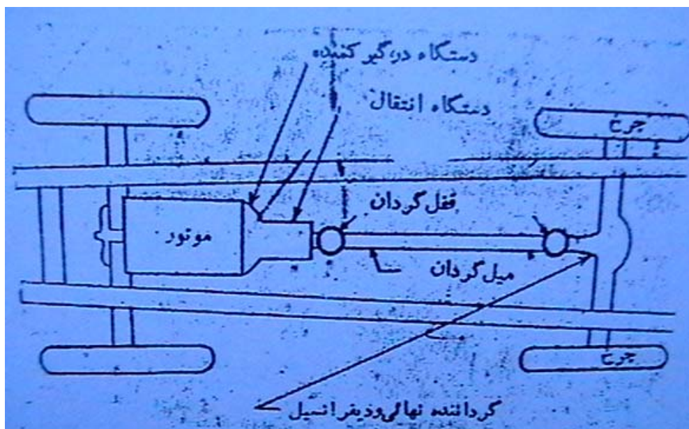
شکل شماره (۴-۳۲) - سیستم انتقال قدرت مکانیکی
