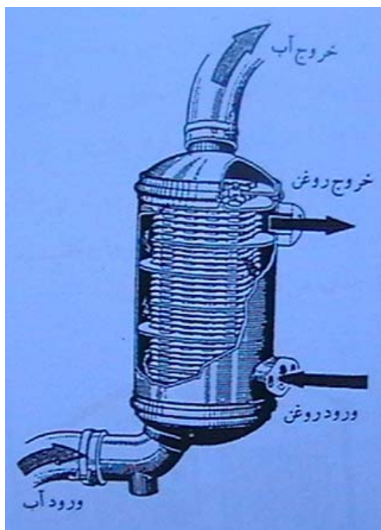
شکل (۴-۲۷) - رادیاتور روغن در سیستم روغنکاری موتور
