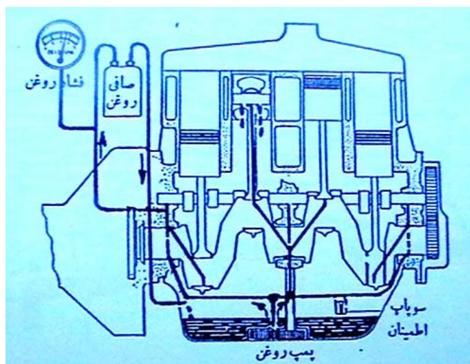
شکل شماره (۴-۲۳) - شماتیک جریان روغنکاری فشاری
