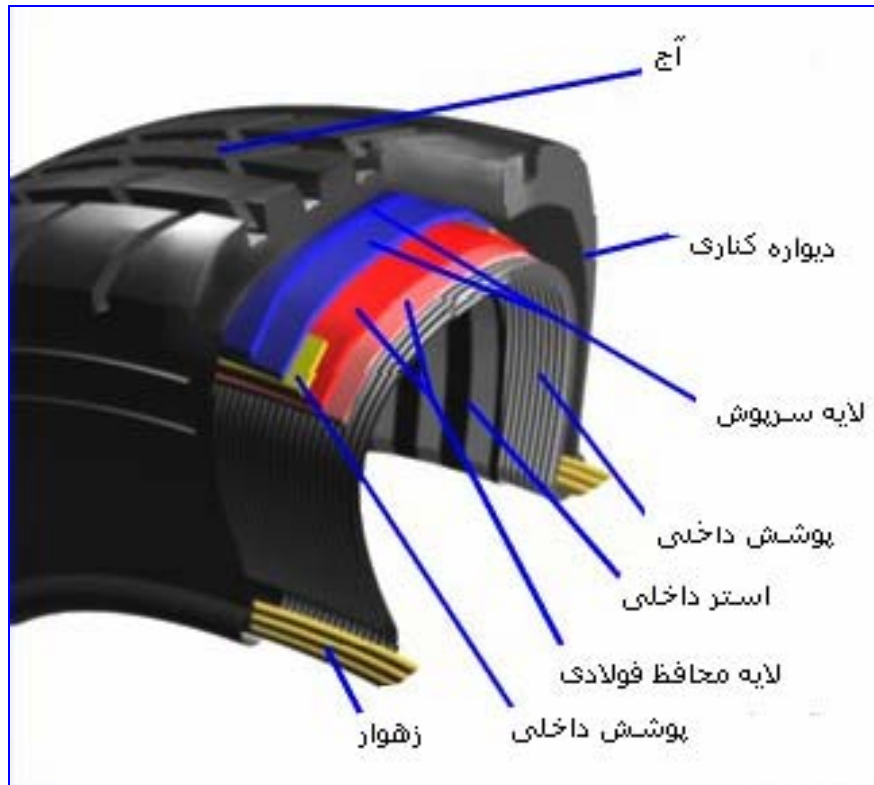
شکل شماره (۵-۵) - اجزاء تشکیل دهنده تایر رویی (شامل : آج- دیواره کناری - لایه سربوش - پوشش داخلی - استر داخلی - لایه محافظ فولادی و زهوار)
