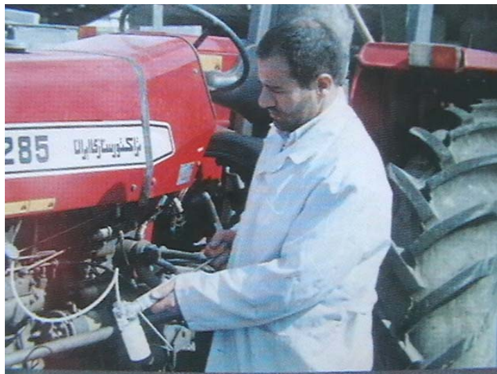
شکل شماره (۶-۱۵)- نمونه گیری از روغن موتور یک دستگاه تراکتور به کمک پمپ خلاء
