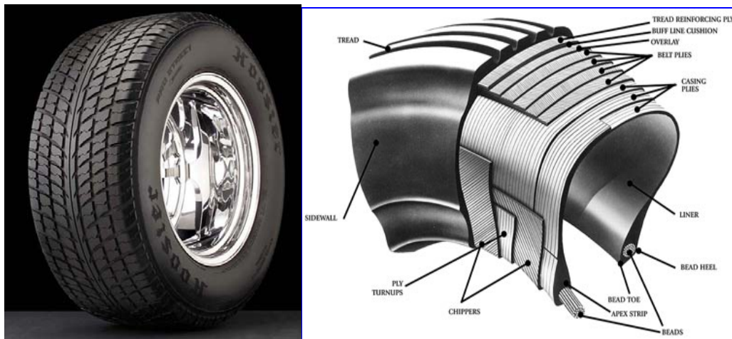
شکل شماره (۵-۳) - ساختار تایر رادیال (Radial)
