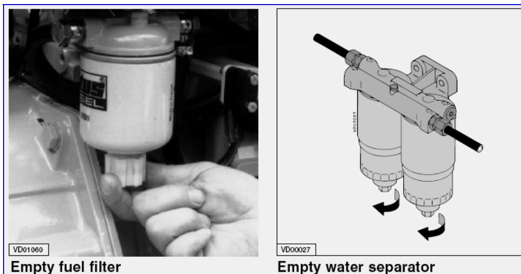
شکل شماره (۴-۳۲) - تخلیه فیلتر و آب گیر در سیستم سوخت
