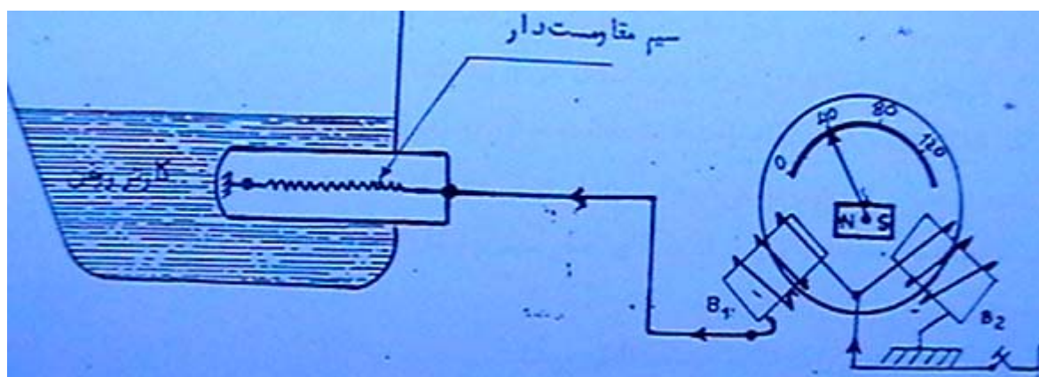
شکل (۴-۲۹) - حرارت سنج روغن موتور
