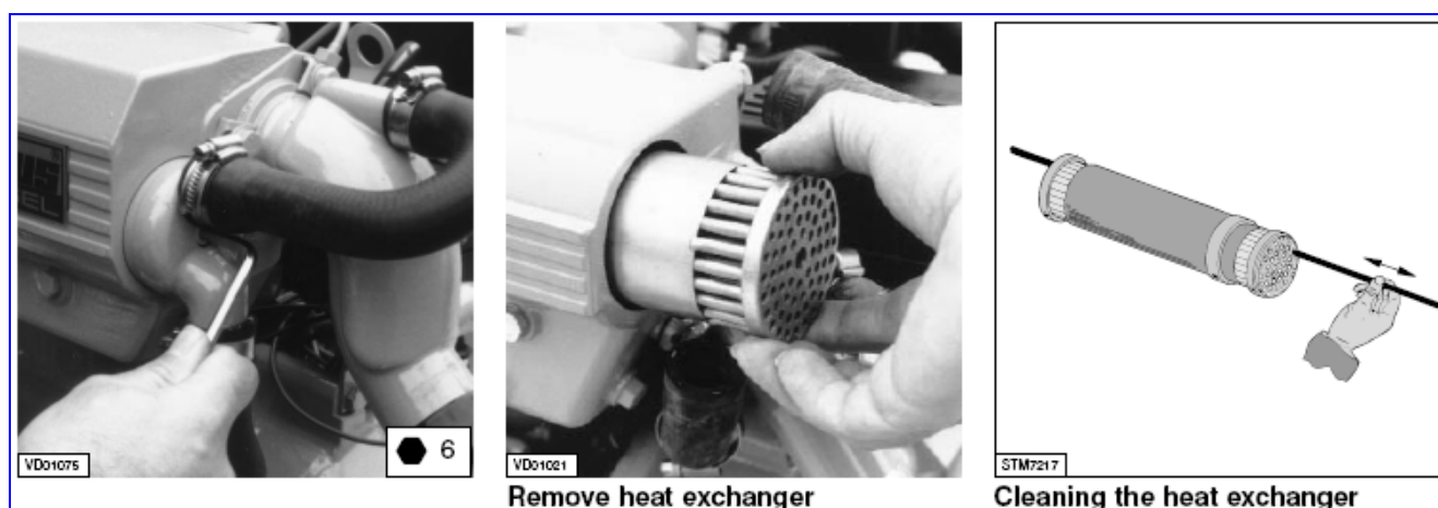
شکل شماره (۴-۲۱) - نظافت مبدل حرارتی در موتورهای دیزل
