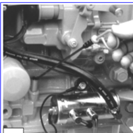
۱- بیرون آوردن میله روغن
