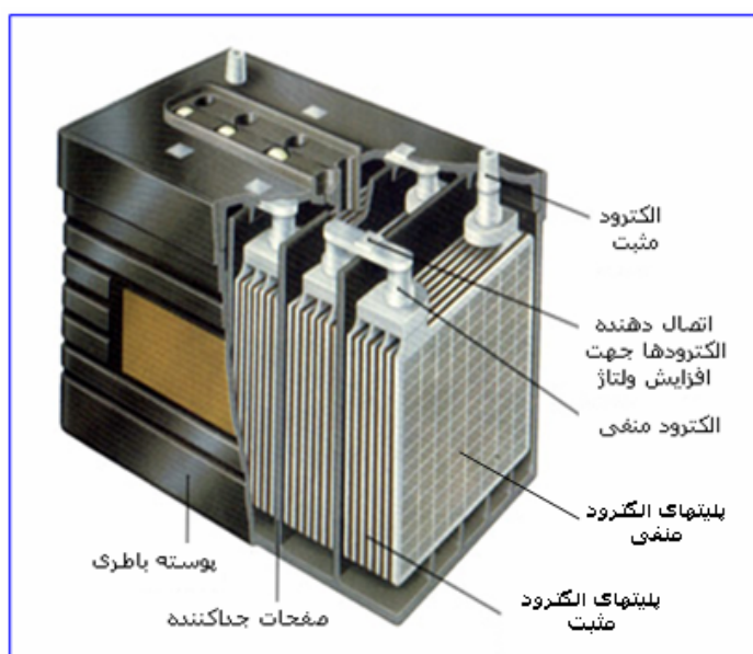
شکل شماره (۴-۸) - اجزاء تشکیل دهنده یک باطری (پوسته باطری - الکتروود مثبت - الکتروود منفی - اتصال دهنده الکتروودها جهت افزایش ولتاژ - پلیت‌های الکتروود منفی - پلیت‌های الکتروود مثبت - صفحات عایق جداکننده)
