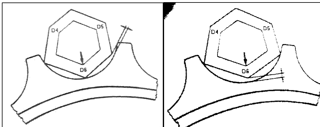
شکل شماره (۴-۵۷) - نحوه استفاده از گیج در دنده اسپراکت
