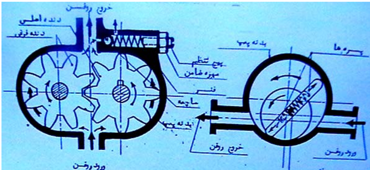
شکل (۴-۲۴) - شماتیک پمپهای روغن - پمپ پره ای (تصویر سمت راست) - پمپ دنده ای (تصویر سمت چپ)
