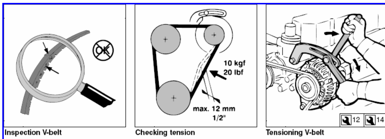
شکل شماره (۴-۱۳) - برنامه های مربوط به تسمه پروانه در موتور شامل بازرسی تسمه ، کنترل میزان کشش تسمه و نحوه تنظیم آن
