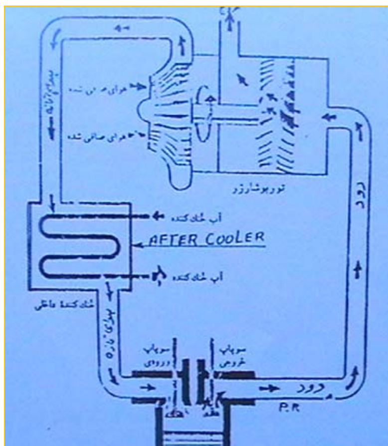
شکل شماره (۴-۱۷)- نمایی شماتیک از یک سیستم توربوشارژر در جدول شماره (۳-۴) برنامه سرویس و نگهداری ذکر شده برای سیستم هوارسانی، ذکر گردیده است:
