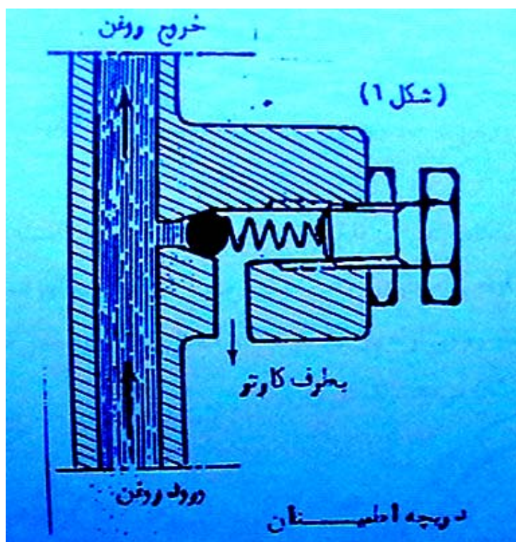
شکل (۴-۲۵) - شماتیک رگولاتور تنظیم فشار روغن در سیستم روغنکاری موتور
