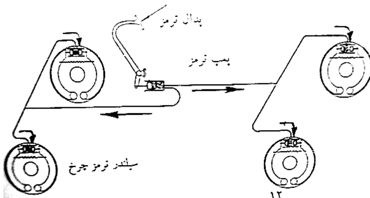
شکل (۴-۴۸) - ساختمان ترمز هیدرولیکی
