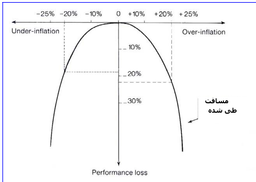
نمودار (۱-۵)- تاثیر کم بادی یا پر بادی بر عمر تایر
