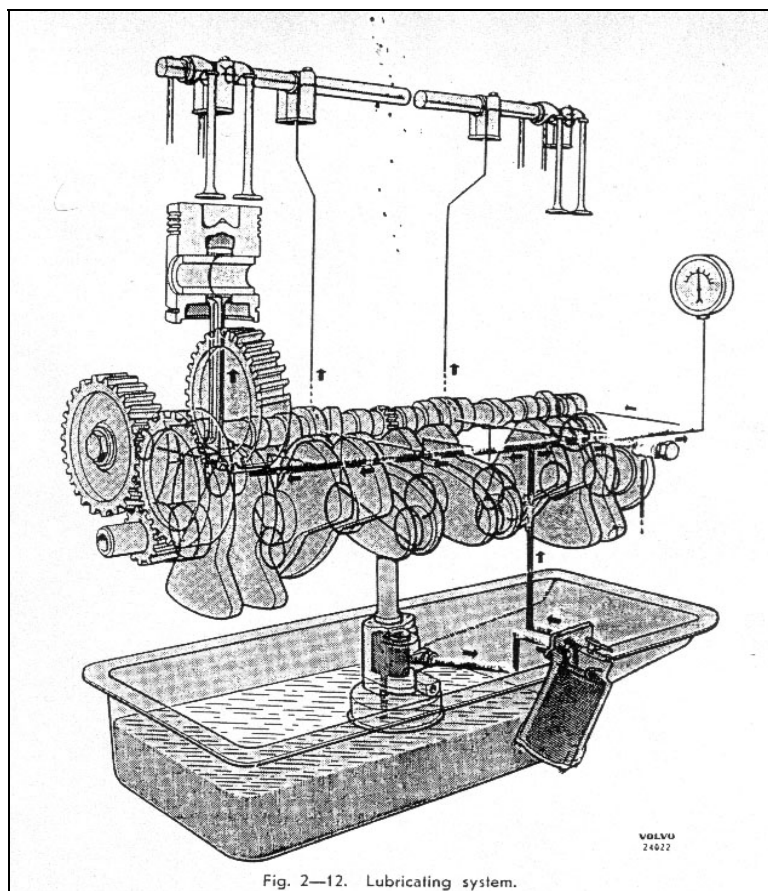
شکل (۳-۱)- سیستم روانکاری یک موتور دیزل
