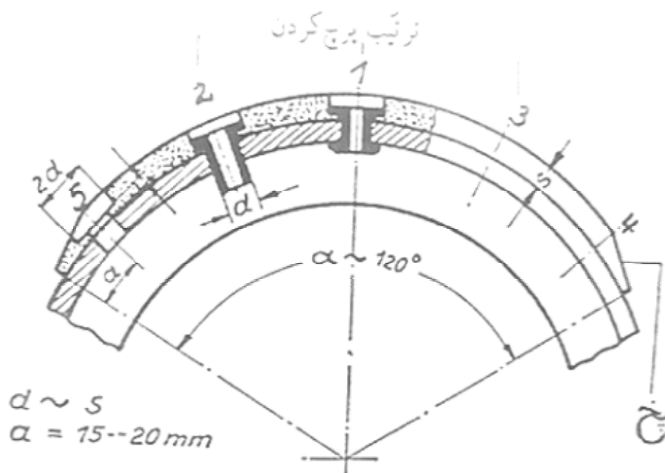
شکل (۴-۴) - شماتیک قسمتی از یک کفشک و لنت ترمز
