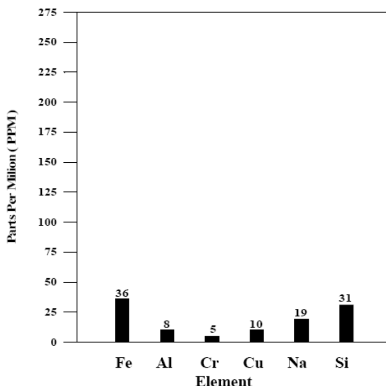
نمودار شماره ۶-۷) آنالیز روغن ناشی از ازدیاد ماده ضد کف در روغن
