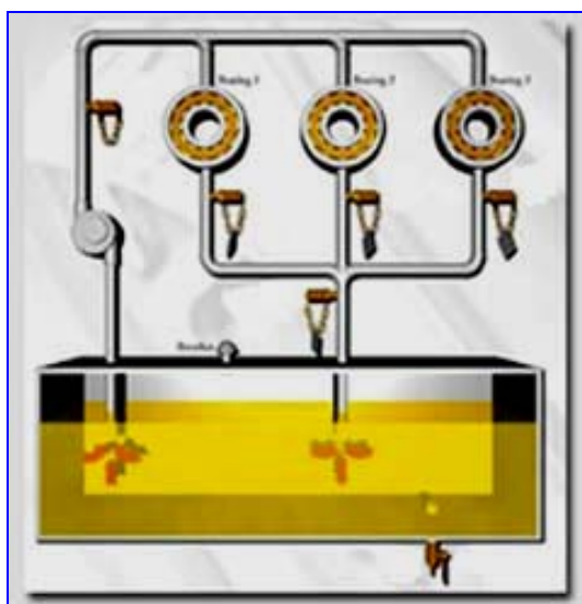
شکل شماره (۶-۱۳) - مدلی از نصب شیرهای سوزنی در لاین سیستم روغنکاری
