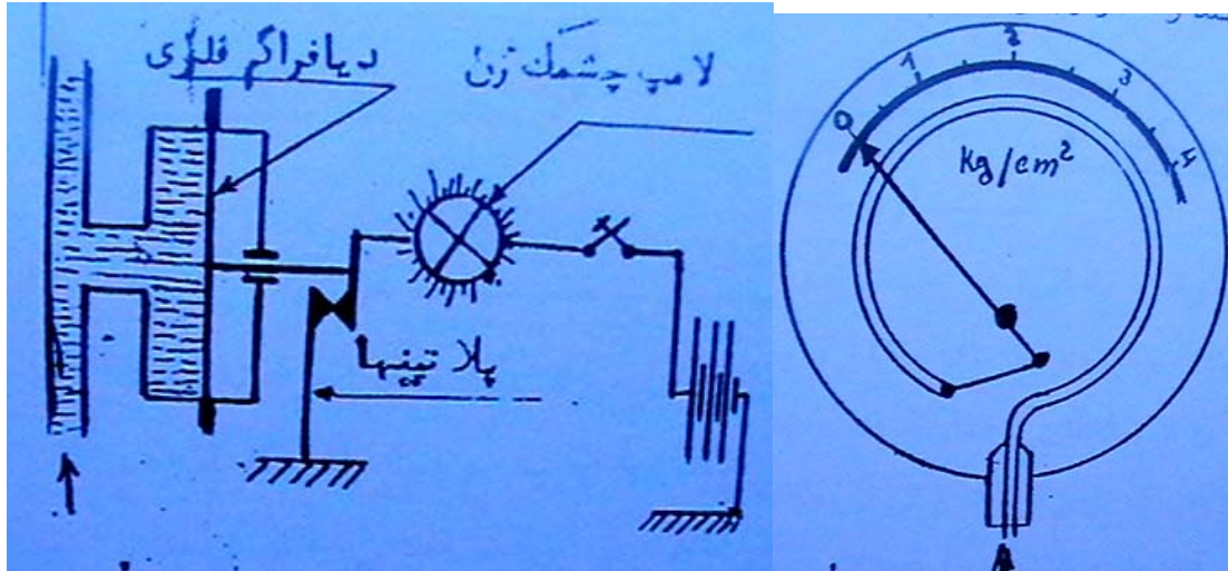
شکل (۴-۲۸)- فشارسنج مکانیکی (تصویر سمت راست)- فشارسنج الکتریکی (تصویر سمت چپ)
