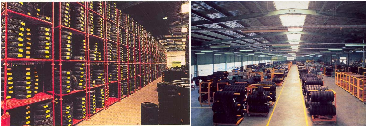
شکل شماره (۵-۱۳) - نمونه هایی از انبارش لاستیکها ( تصاویر مربوط به انبار یک کارخانه لاستیک سازی در کشور پرتغال می‌باشد )
