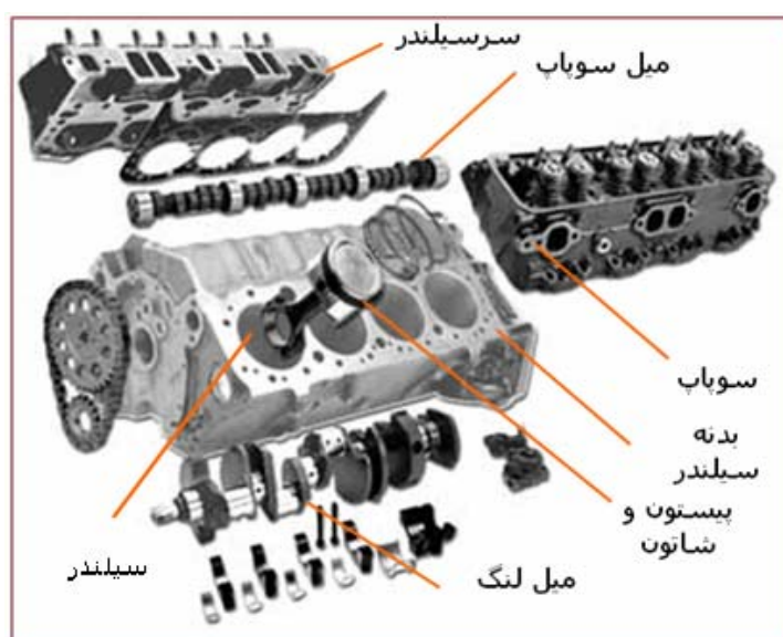
شکل شماره (۳-۴) - اجزاء اصلی تشکیل دهنده بدنه موتور دیزل
