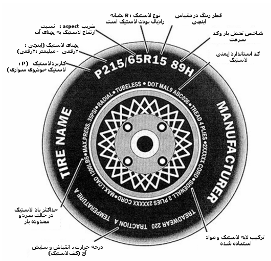
شکل (۵-۶) - نمونه ای از مشخصات مندرج روی بدنه لاستیک (تایر) رادیال
