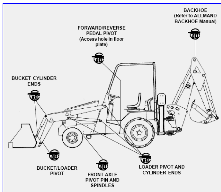
شکل شماره (۴-۳۸) - نقاط نیازمند گریسکاری در اعضاء کارساز ماشین نشان داده شده است.
