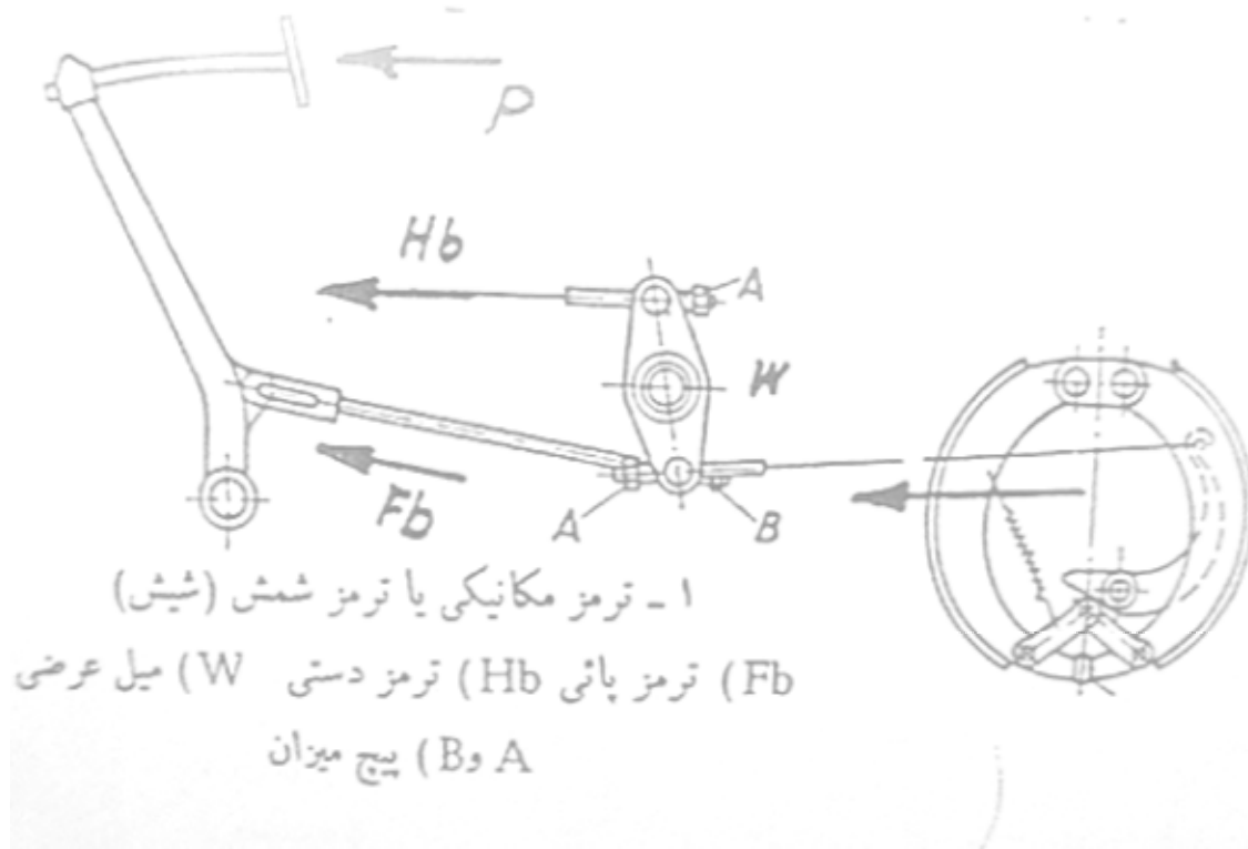
شکل (۴-۴۷) - شماتیک ترمز مکانیکی
