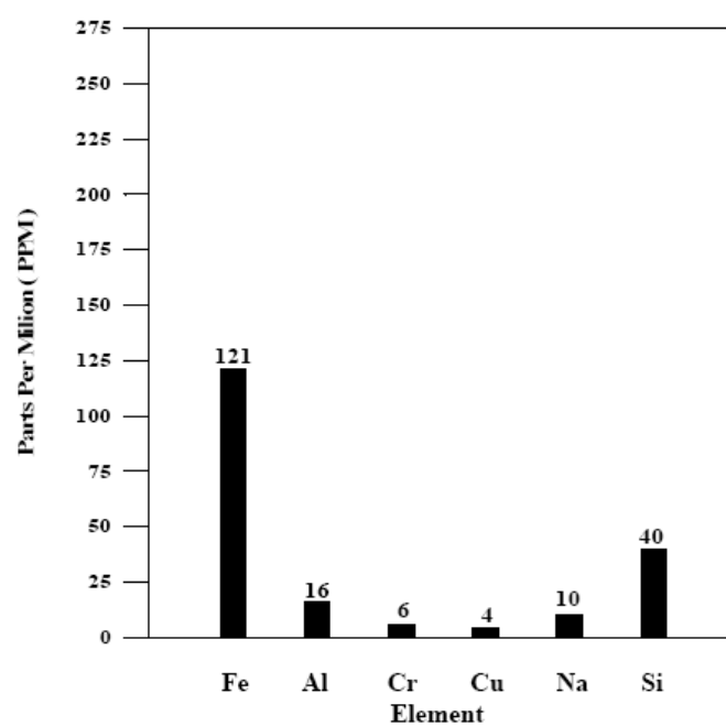
شکل شماره (۶-۶) - سایش رینگ، پیستون و بوش پیستون ناشی از گرد و غبار
