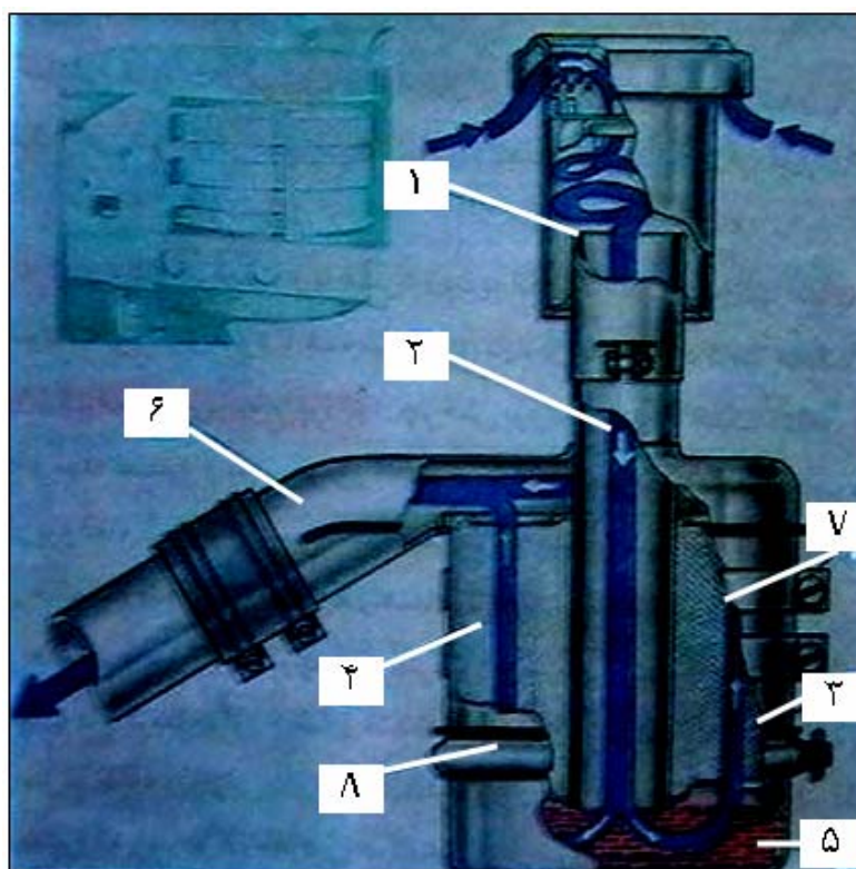
شکل شماره (۴-۱۵) - اجزاء صافی هوای روغنی که شامل اجزاء زیر می‌باشد:
