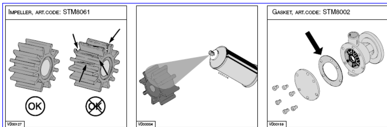
شکل شماره (۴-۲۰) - دمنوتاژ واتر پمپ (هر ۱۰۰۰ ساعت کار)، سرویس و کنترل وضعیت دنده ها و فیلتر
