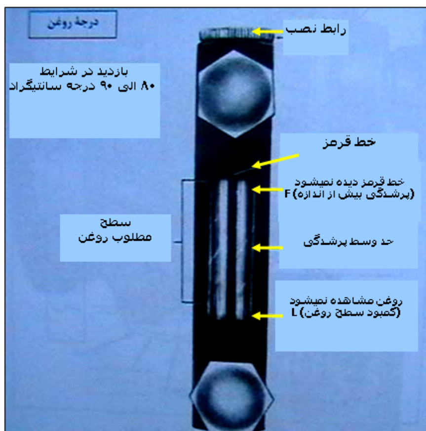
شکل شماره (۴-۳۷)- نمایی از گیج میزان روغن در گیربکس هیدرولیک
