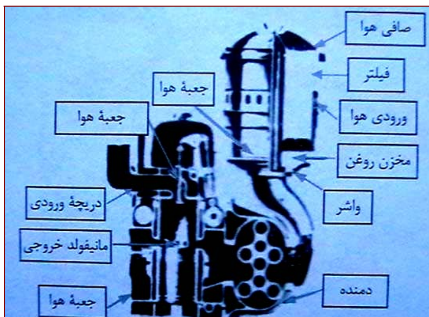
شکل شماره (۴-۱۴)- اجزاء سیستم هوارسانی در یک موتور دیزل
