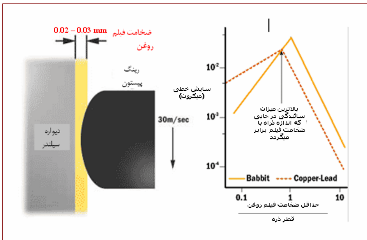
شکل (۳-۳) - وضعیت روغن بین دیواره سیلندر و رینگ پیستون در موتور
