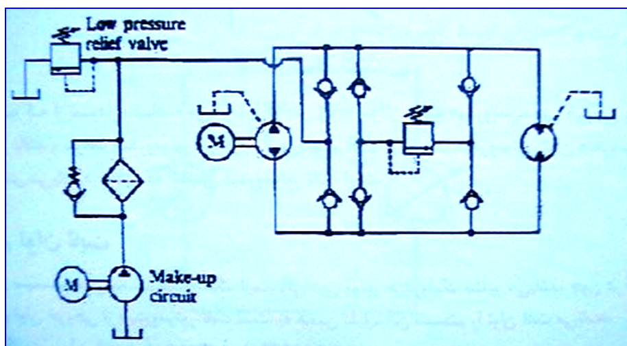
شکل شماره (۴-۳۳)- نقشه هیدرولیکی یک سیستم انتقال قدرت هیدرواستاتیکی مدار بسته
