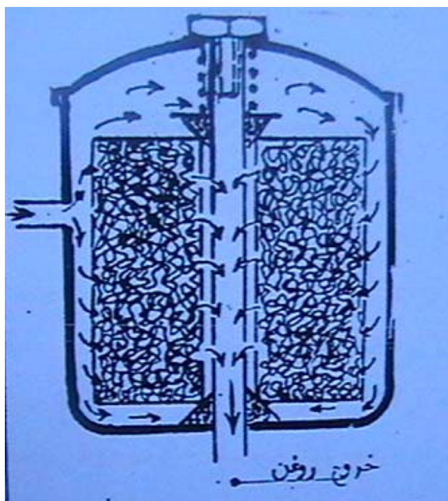
شکل (۴-۲۶)- فیلتر روغن در سیستم روغنکاری موتور
