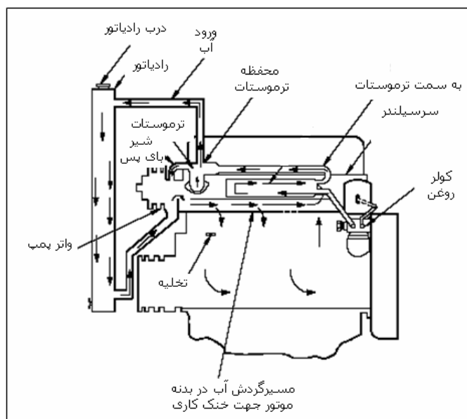
شکل شماره (۴-۱۸)- نمای شماتیک یک نمونه سیستم خنک کاری در موتور دیزل
