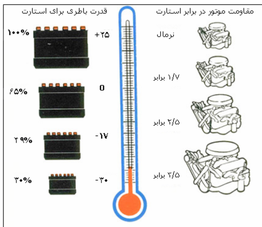
شکل شماره (۴-۱۲)- میزان مقاومت موتور در برابر استارت و قدرت باطری برای استارت در دمای کاری مختلف
