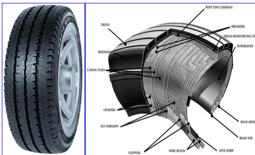
شماره (۵-۲) - ساختار تایر معمولی
