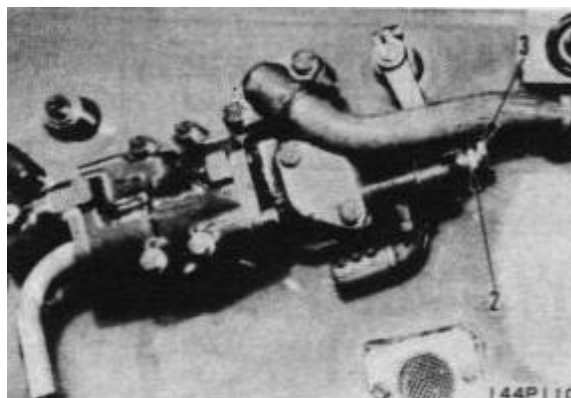
شکل (۴-۴۳)- نحوه تنظیم شیر فشار شکن
