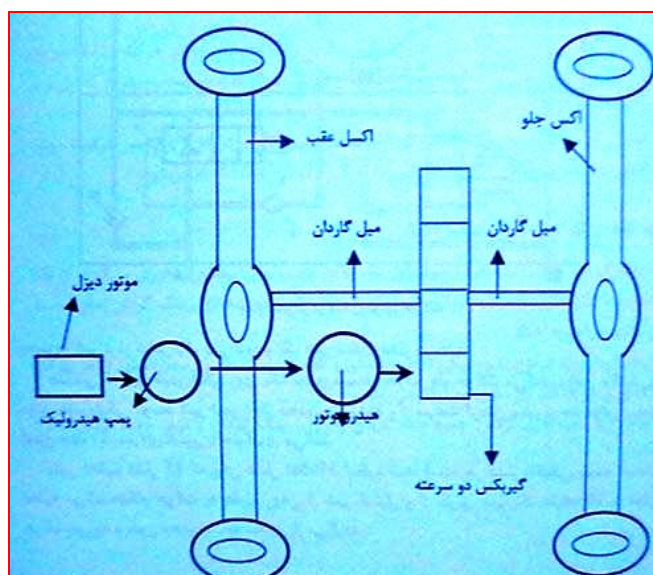
شکل شماره (۴-۳۵)- شکل شماتیک کارکرد سیستمهای انتقال قدرت هیدرواستاتیک
