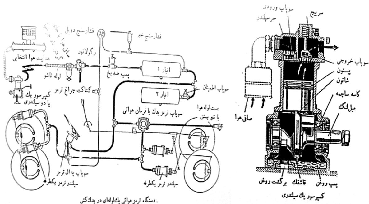
شکل (۴-۴۹) - نمایی شماتیک از اجزاء ترمز هوایی در يدك كش
