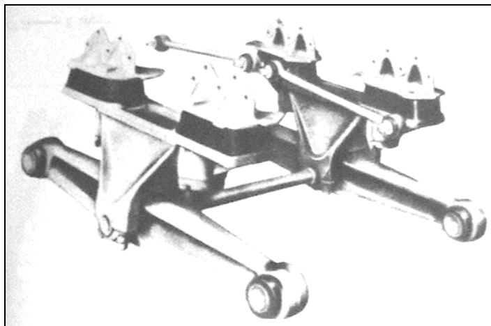
شکل شماره (۴-۵۸)- تصویری از یک سیستم تعلیق یا بالشتک لاستیک
