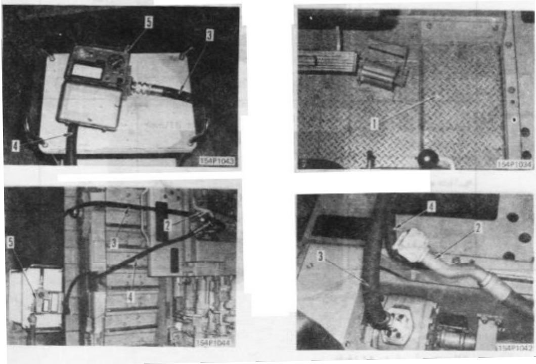
شکل شماره (۴-۴۵)-اندازه گیری دبی سیستم هیدرولیکی
