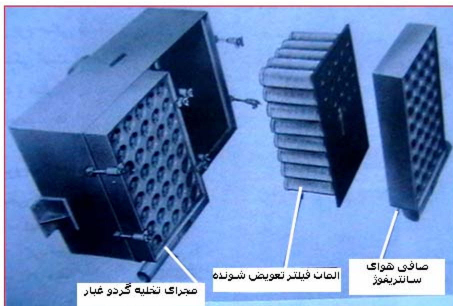
شکل شماره (۴-۱۶)- اجزاء صافی هوا از نوع فار که شامل اجزاء زیر می باشد: صافی هوای سانتریفوژ (صافی مرحله اول)- المان فیلتر تعویض شونده (فیلتر مرحله دوم)- مجرای تخلیه گرد و غبار
