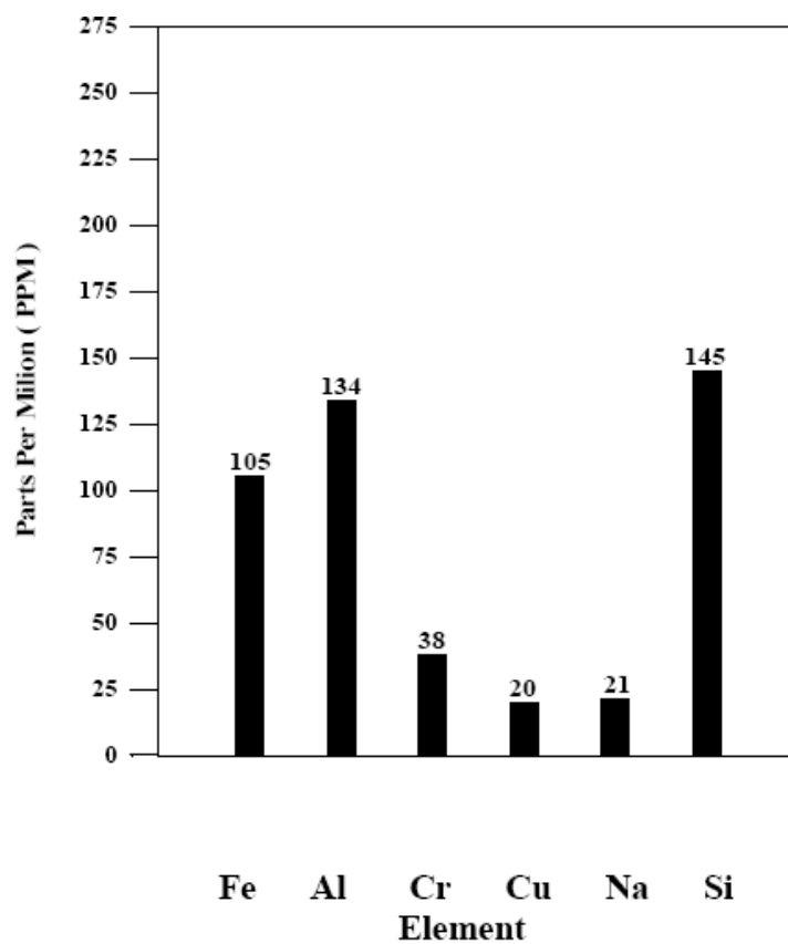
نمودار شماره (۶-۶) - آنالیز روغن ناشی از خرابی سیستم سوخت
