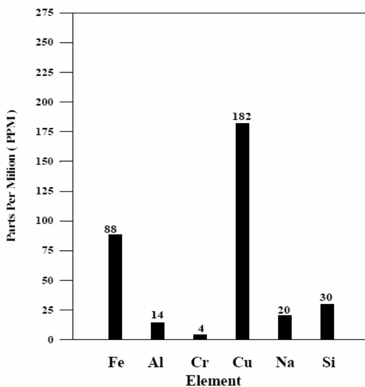
نمودار شماره (۲-۶) - آلودگی گردوغبار و سایش در قسمتهای پایینی موتور
