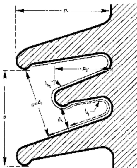
شکل ۲-۴: نمونه چترهای دیگر
