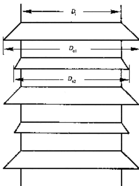
شکل ۲-۸: مقره اتکایی با چترهای متفاوت
