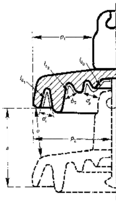
شکل ۲-۵: مقره‌های بشقاب‌ی از نوع Cap & Pin
