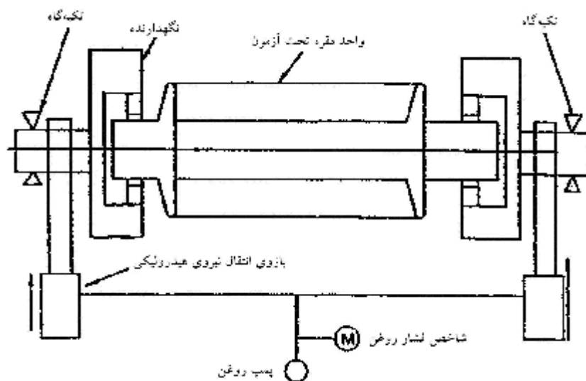
شکل ۳-۶: شماتیک تجهیز آزمونی قابل استفاده در روش آزمون به طریق اعمال ممان خمشی یکنواخت
