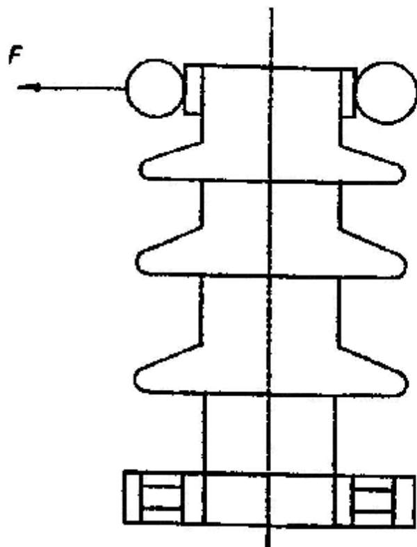
شکل ۳-۸: شماتیک تجهیز آزمونی قابل استفاده در روش آزمون به طریق اعمال نیروی خمشی
