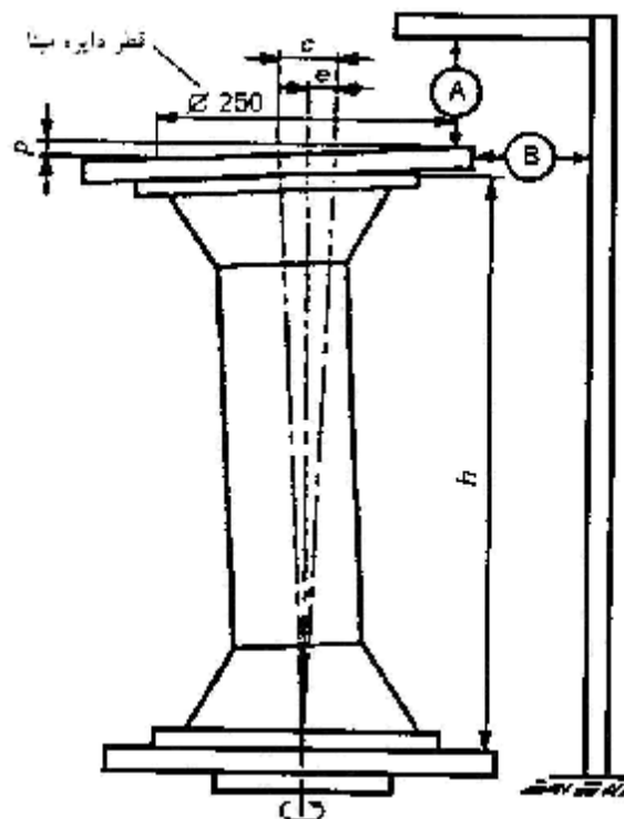
شکل ۳-۱: آرایش آزمون مورد استفاده جهت بررسی توازی سطوح انتهایی و انحراف از مرکز مقره اتکایی
