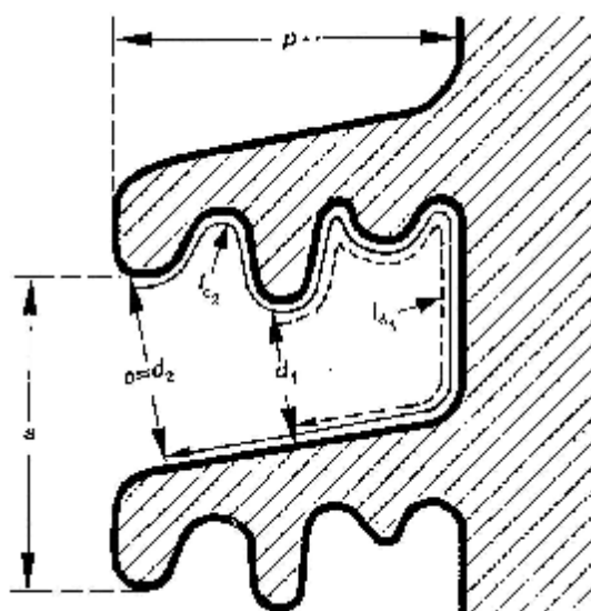
شکل ۲-۶: چترهای با شیارهای زیرین
