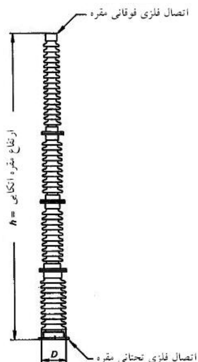
شکل ۱-۱: یک نمونه از مقره‌های اتکایی مورد استفاده در پست‌های فشارقوی فضای باز با فیتینگهای بیرونی ۱
