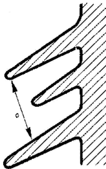
شکل ۲-۱: حداقل فاصله C مابین چترها
