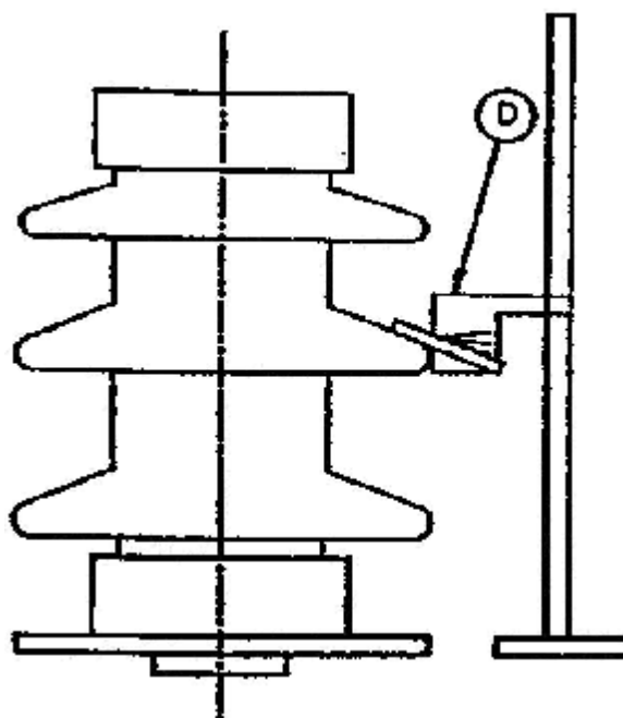
شکل ۳-۴: آرایش آزمونی مورد استفاده جهت بررسی شیب چتر مقره اتکایی
