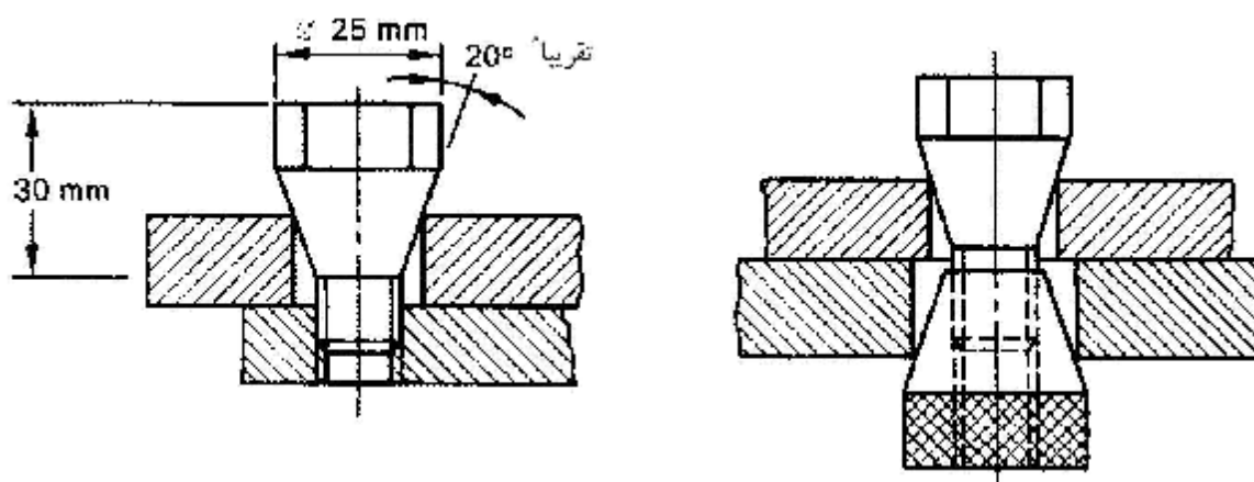
شکل ۳-۵: روشهایی برای اتصال مقره اتکایی به صفحه چرخان و دستیابی به هم مرکزی آنها
