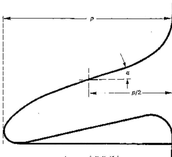
شکل ۲-۲: شیب چترها
