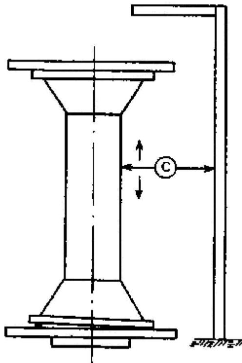
شکل ۳-۳: آرایش آزمونی مورد استفاده جهت بررسی میزان خمیدگی مقره اتکایی
