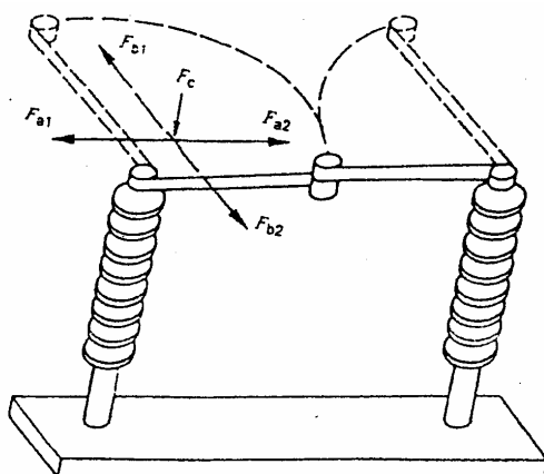
شکل ۲-۱: نیروی مکانیکی نامی وارده بر ترمینالها (سگسیونر افقی با قطع از یک نقطه)
