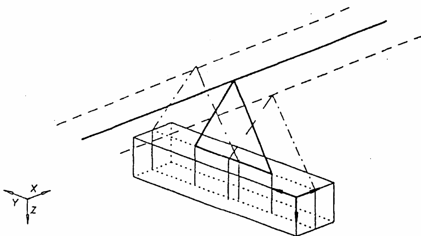
شکل ۳-۶: کنتاكت ثابت، موازی با پایه سکسیونر
