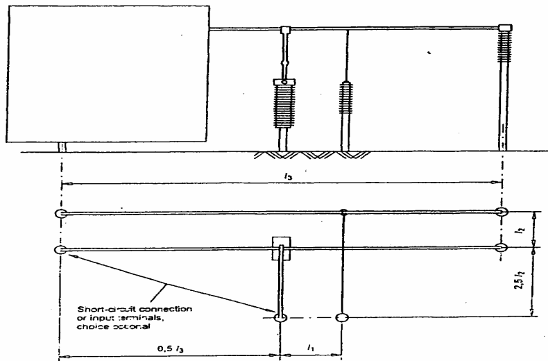
شکل ۳-۴: چیدمان آزمون تکفاز برای سکسیونرهای با فاصله عایقی عمودی با هادی رشته‌ای
