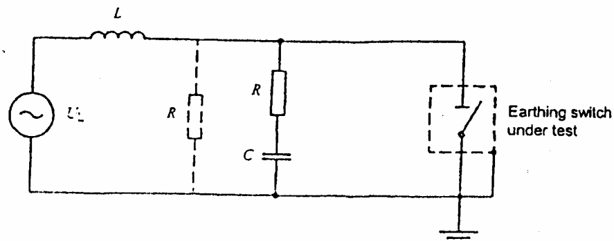
شکل ۳-۹: مدار آزمون برای آزمونهای قطع و وصل جریان القایی الکترومغناطیسی
