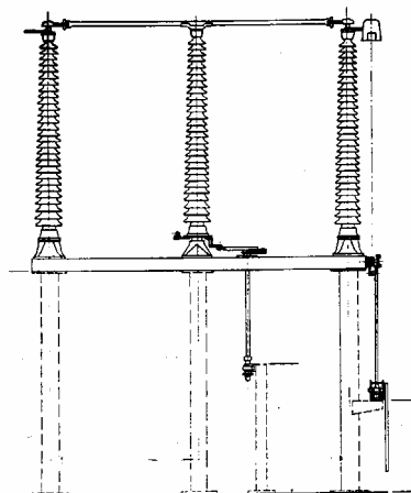
شکل ۲-۱: سکسیونر افقی با قطع از دو نقطه
