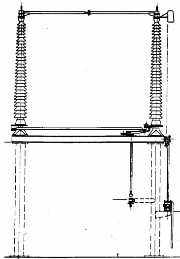
شکل ۱-۱: سکسیونر افقی با قطع از یک نقطه
