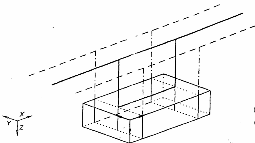
شکل ۳-۶: کنتاكت ثابت، موازی با پایه سکسیونر
