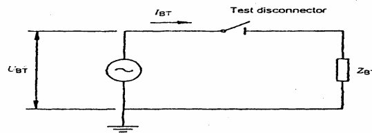
مدار آزمون A
