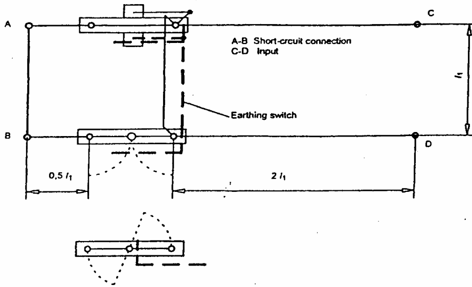
شکل ۳-۳: چیدمان آزمون تکفاز برای سکسیونرهای افقی
