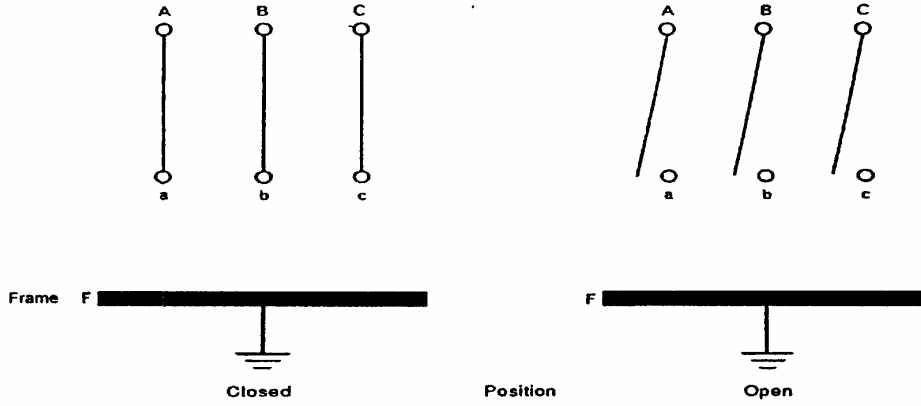
شکل ۱-۳: دیاگرام اتصالات پل‌های یک سکسیونر
