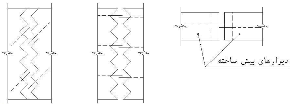
شکل ۹-۶-۲-ت درز اره‌ای
