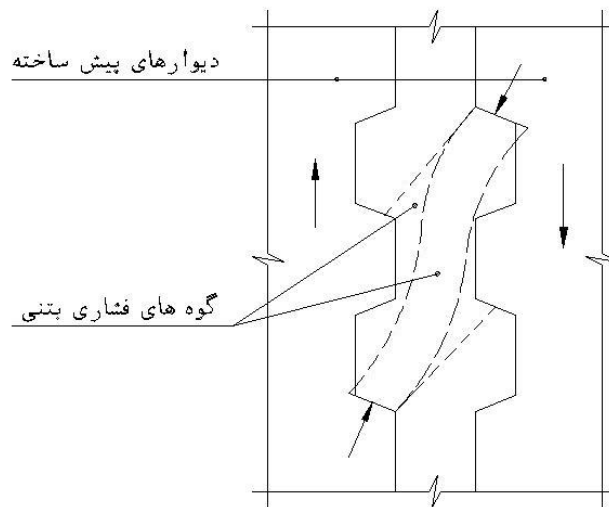
شکل ۹-۶-۲-ت گوه های فشاری در درزهای کنگره ای
