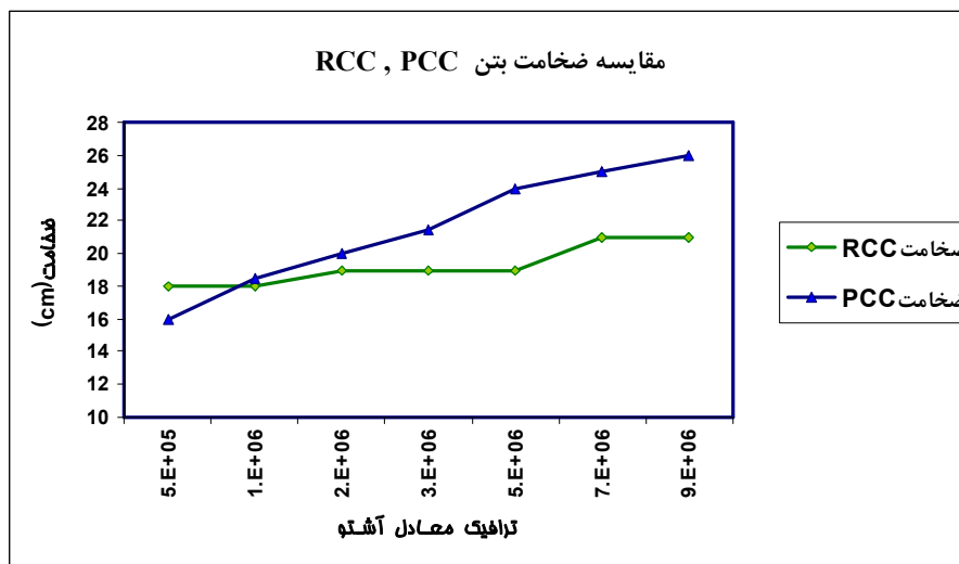
شکل ۸-۵ مقایسه ضخامت بتن در روسازی RCC و PCC در ترافیک تفاوت
