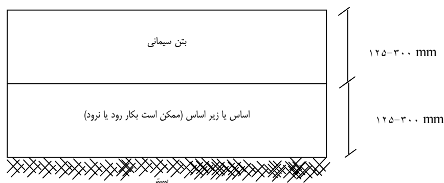
شکل ۱-۲ تیپ یک روسازی بتنی
