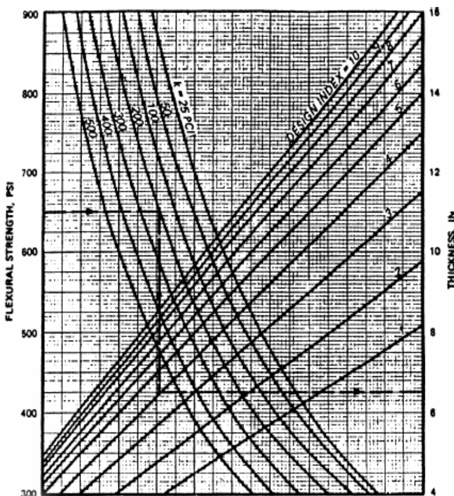
شکل ۷-۹ گراف طراحی گروه مهندسين ارتش آمریکا [۴]
