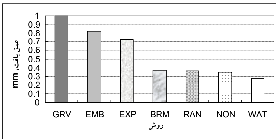
شکل ۳-۷ مقدار عمق بافت (TD) روشهای مختلف در زمان تکمیل پروژه
