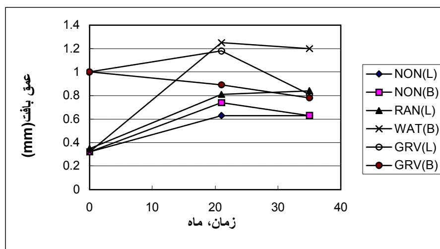
شکل ۳-۹ تغییرات عمق بافت (TD) نسبت به زمان در پروژه ذویان
