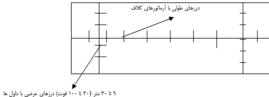
شکل ۲-۳ تیپ روسازی بتنی مسلح درزدار
