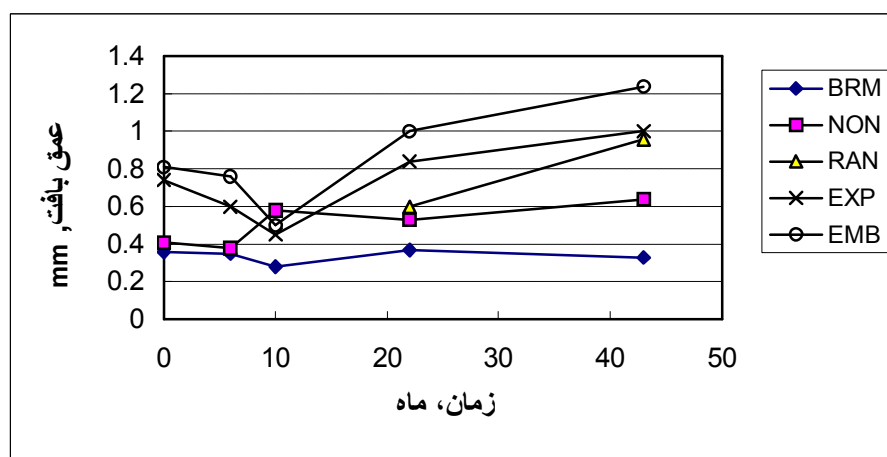
شکل ۳-۸ تغییرات عمق بافت (TD) نسبت به زمان در پروژه تانینانگ
