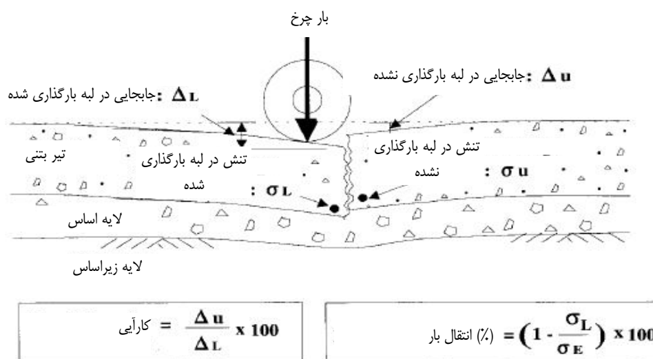
شکل ۱-۷ مکانیسم انتقال بار و کارایی از قفل و بست بین دانه‌ای [۳]
