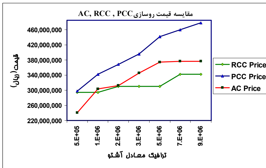
شکل ۸-۶ مقایسه قیمت برای سه نوع روسازی AC و RCC و PCC
