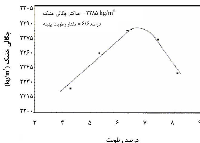
شکل ۳-۲ رابطه چگالی - درصد رطوبت برای بتن‌های غلتکی
