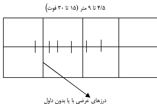
شکل ۲-۲ تیپ روسازی بتنی ساده درزدار
