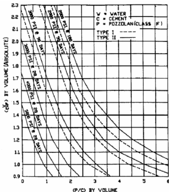
شکل ۲-۵ رابطه بین مقاومت فشاری بتن غلتکی و نسبت آب به مواد سیمانی، به ازای نسبت‌های مختلف پوزولان به سیمان
