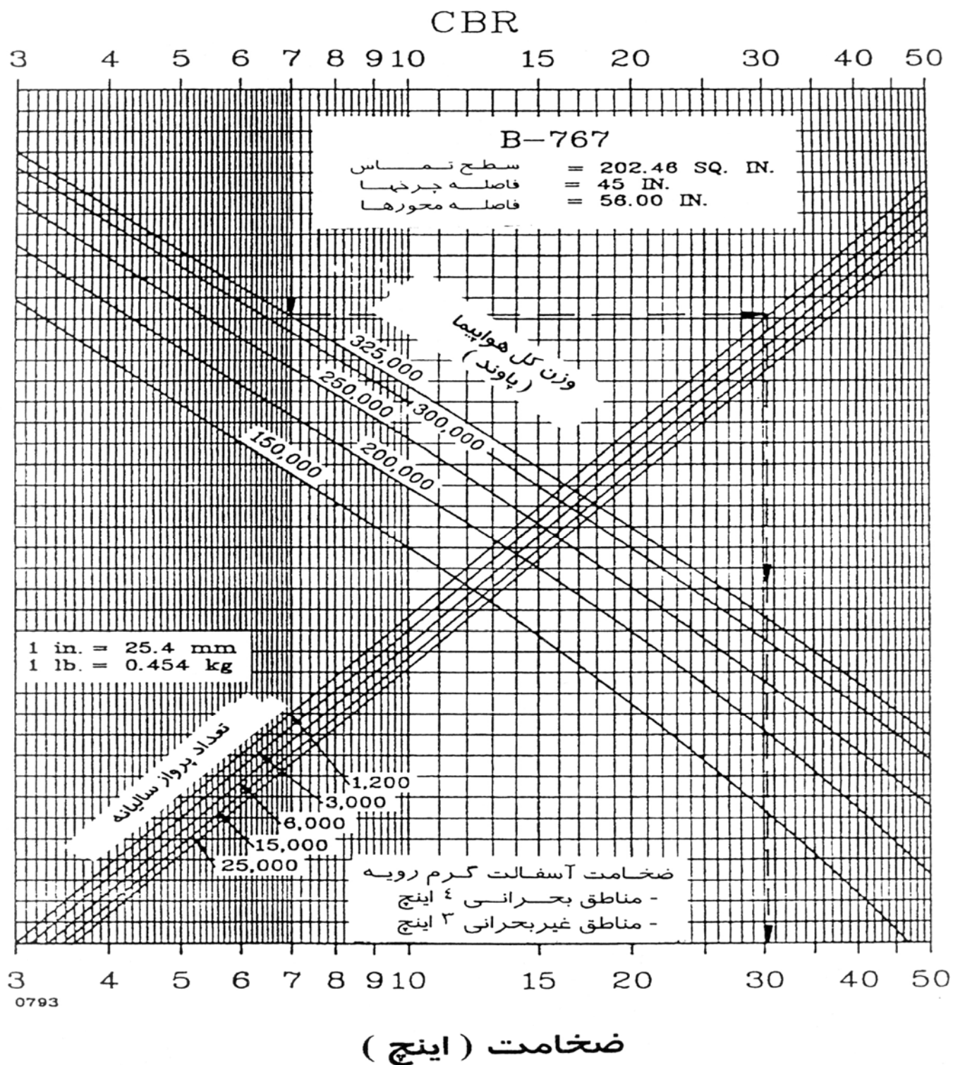
شکل (۳-۱۰) - منحنی طرح روسازی انعطاف پذیر برای هواپیماهای B767
