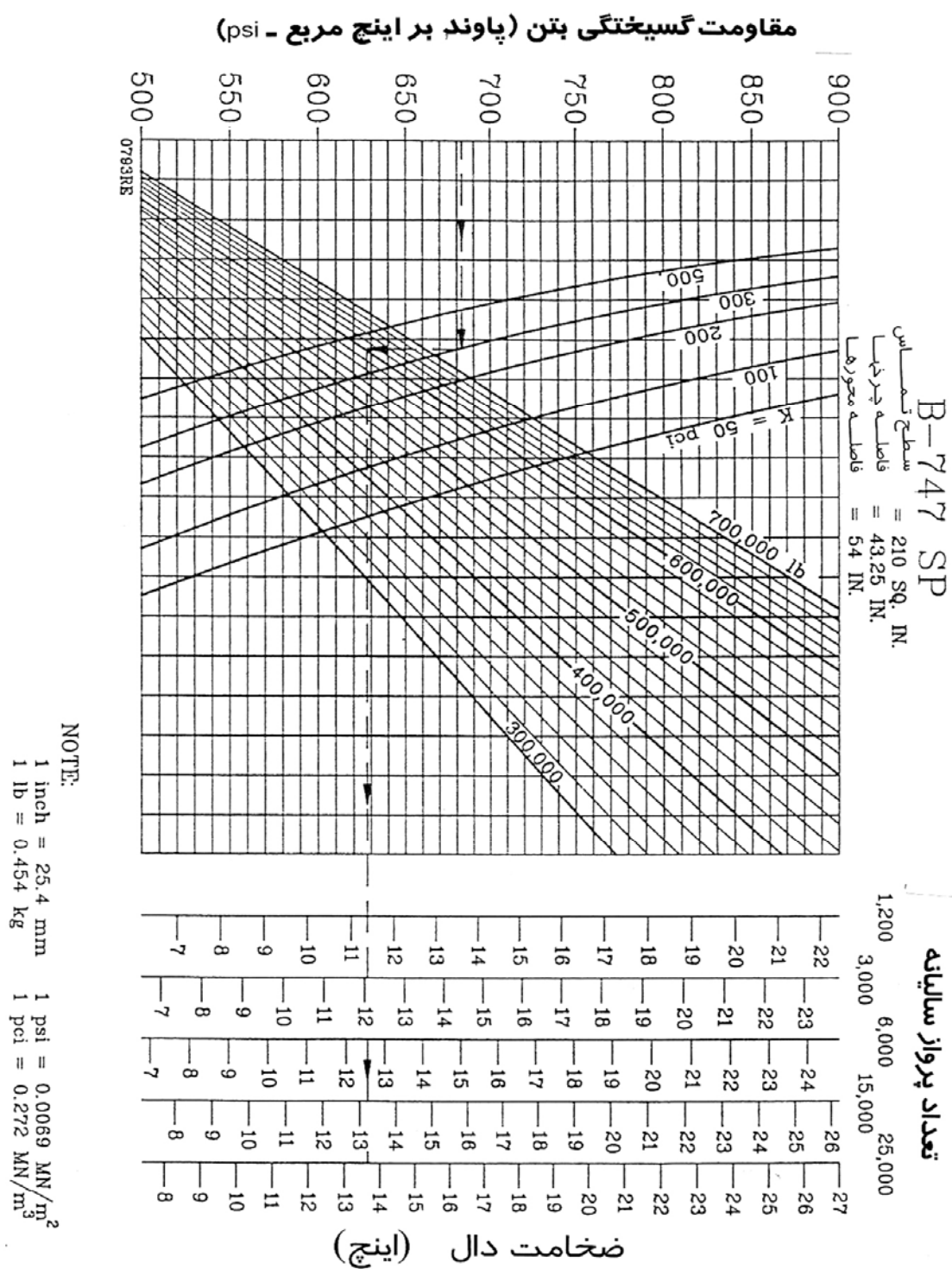
شکل (۳-۳۵) - منحنی انتخابی طرح روسازی صلب برای هواپیمای B747-SP
