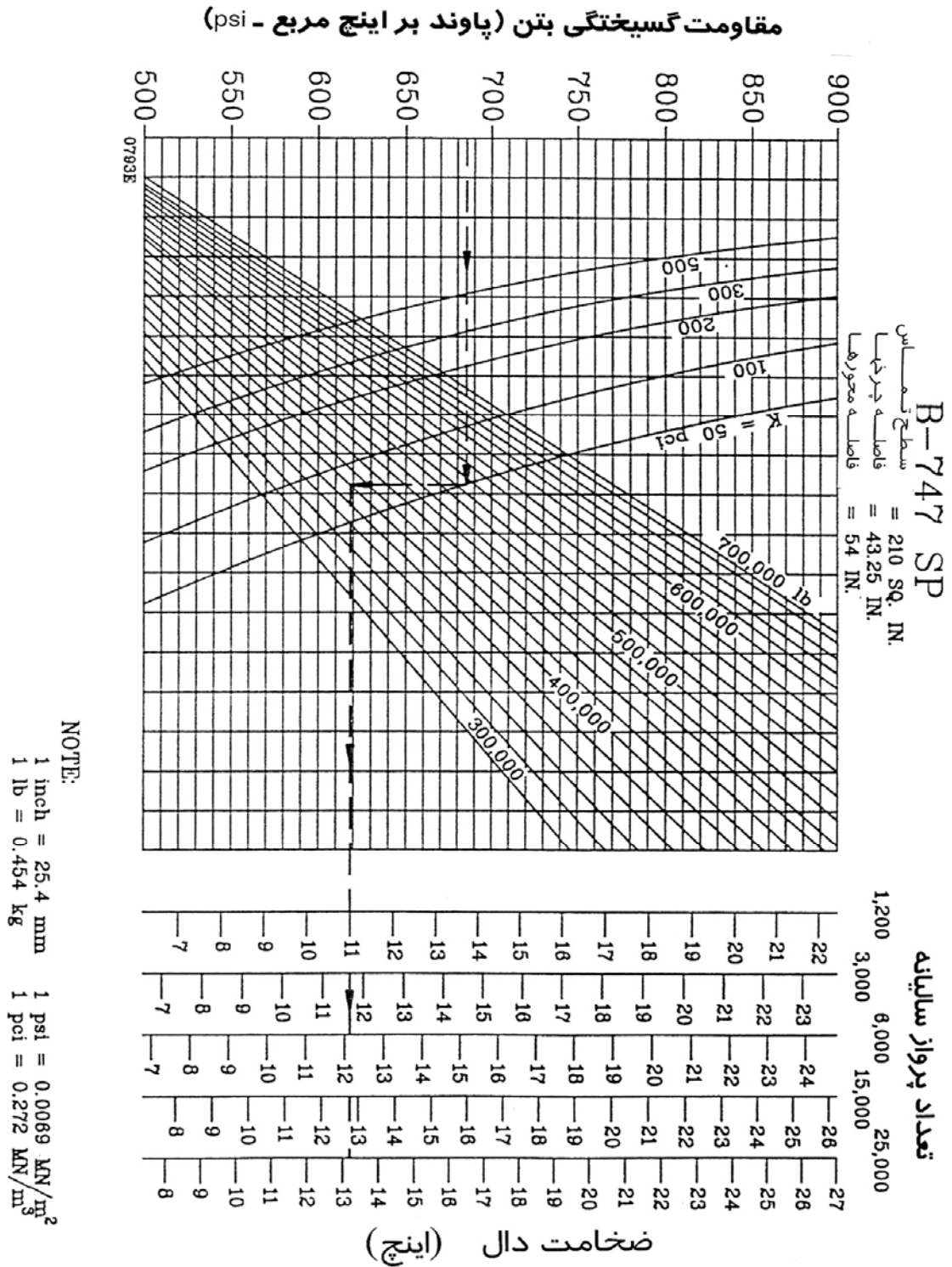
شکل (۳-۲۴) - منحنی طرح روسازی صلب برای هواپیمای B747-SP
