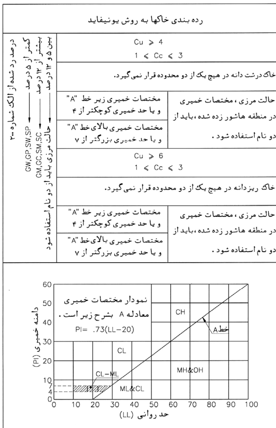
شکل (۲-۲) - معیارهای طبقه بندی خاک
