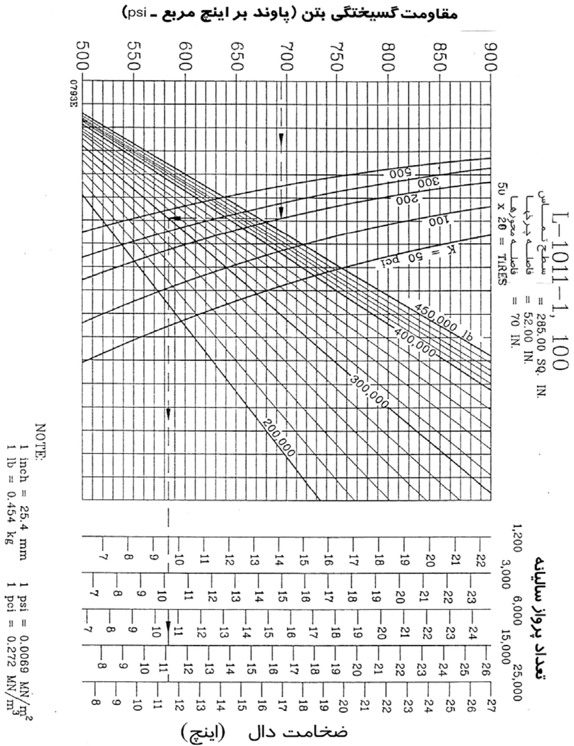
شکل (۳-۳) - منحنی طرح روسازی صلب برای هواپیماهای L1011-1, 100
