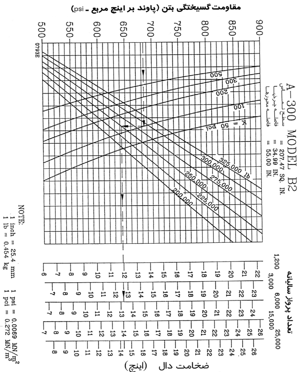
شکل (۳-۲۱) - منحنی طرح روسازی صلب برای هواپیمای A-300 مدل B2
