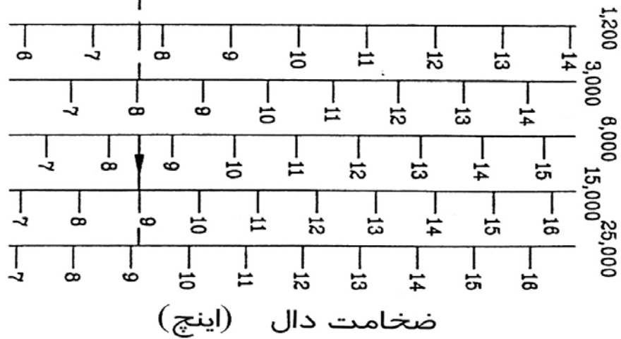
شکل (۳-۱۸) - منحنی طرح روسازی صلب برای چرخ تکی
