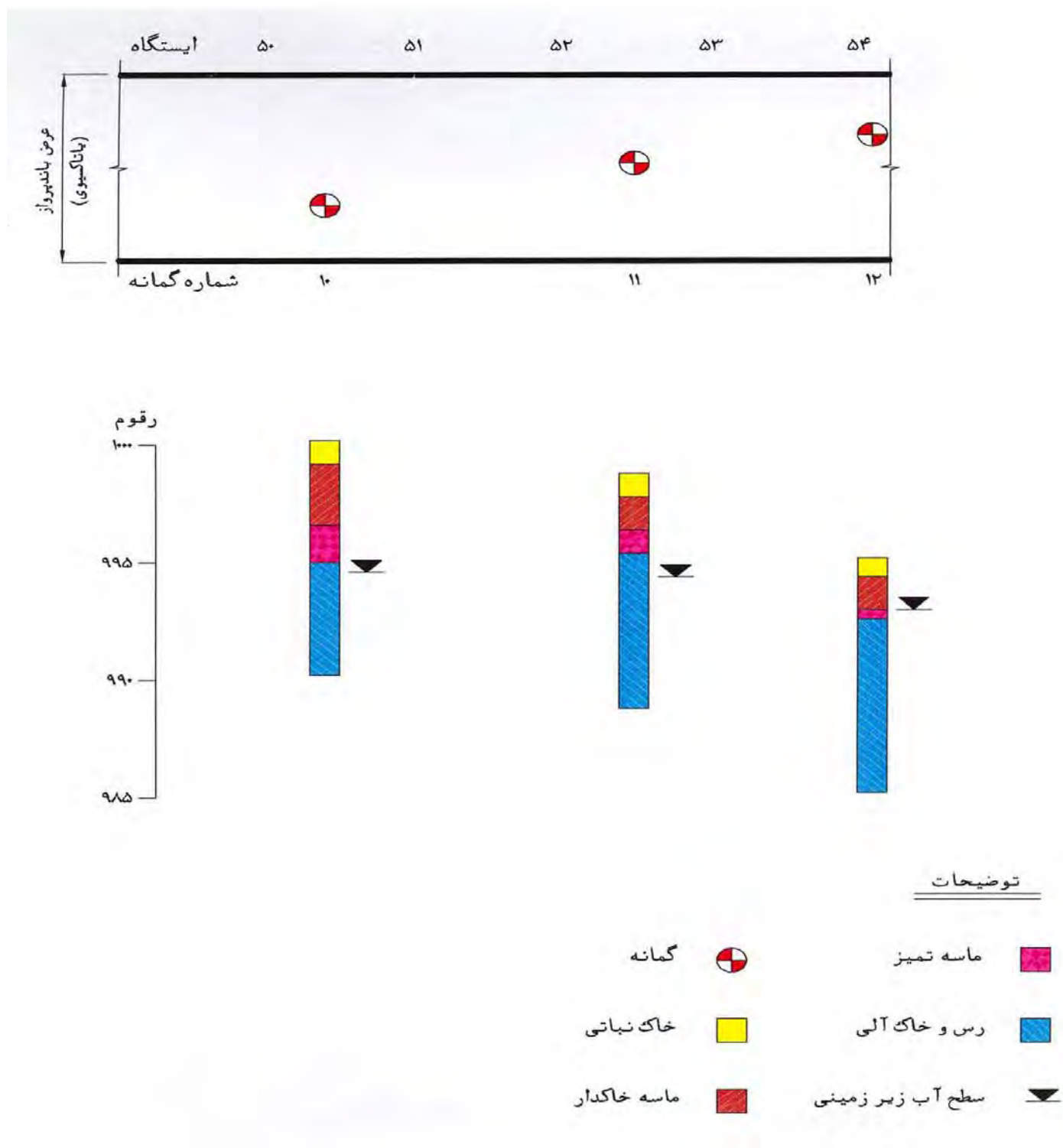
شکل (۲-۱) - نقشه نمونه موقعیت گمانه زنی و نیمرخ ارتفاعی آن
