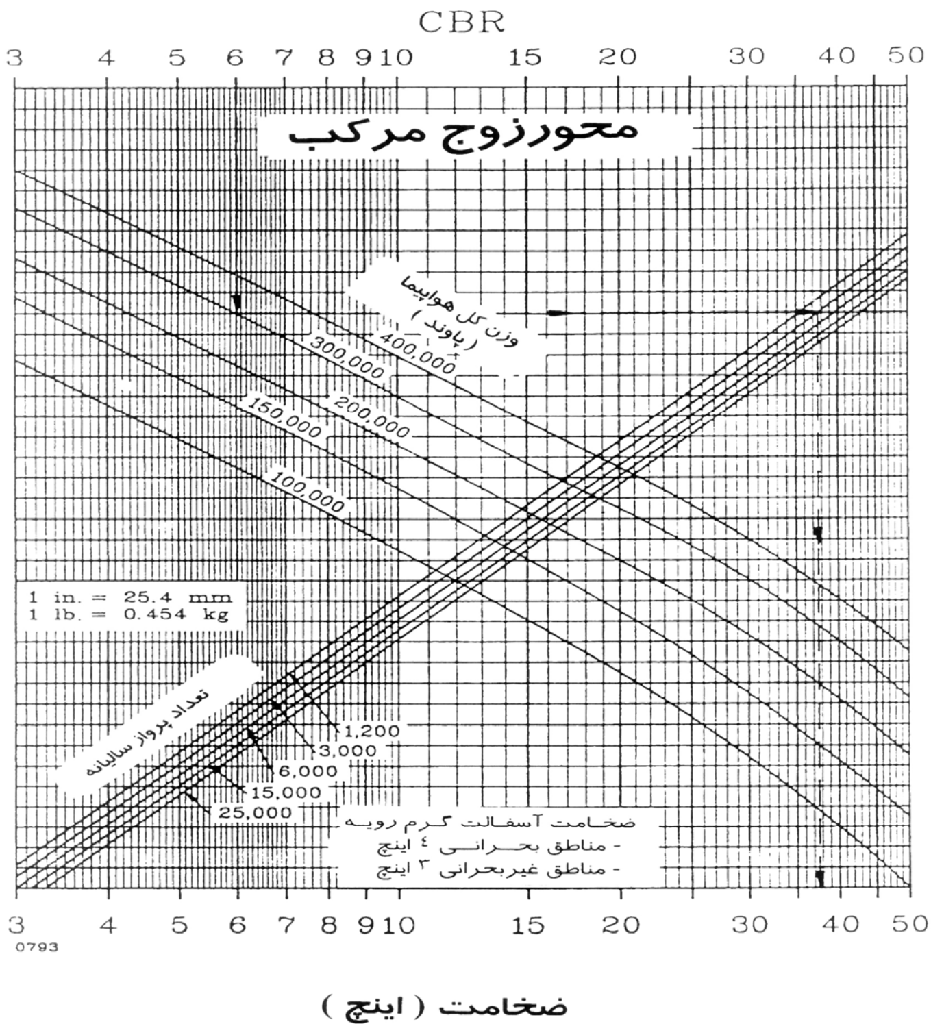
شکل (۳-۴) - منحنی طرح روسازی انعطاف پذیر برای چرخ زوج مرکب
