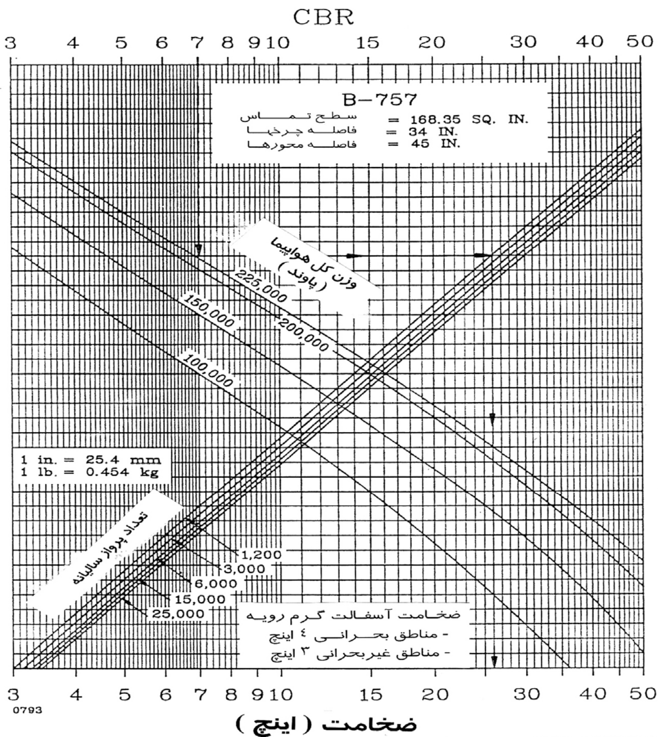
شکل (۳-۹) - منحنی طرح روسازی انعطاف پذیر برای هواپیماهای B757
