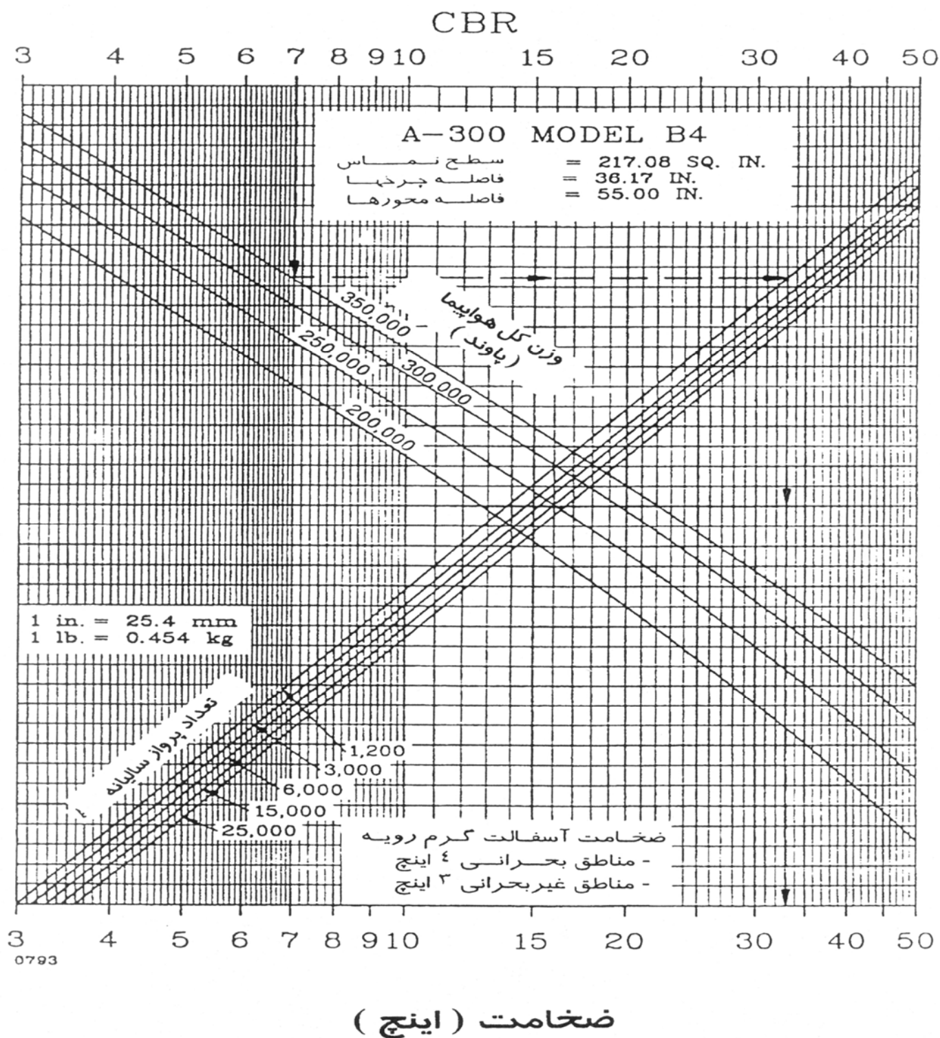
شکل (۳-۶) - منحنی طرح روسازی انعطاف پذیر برای هواپیمای A-300 مدل B4
