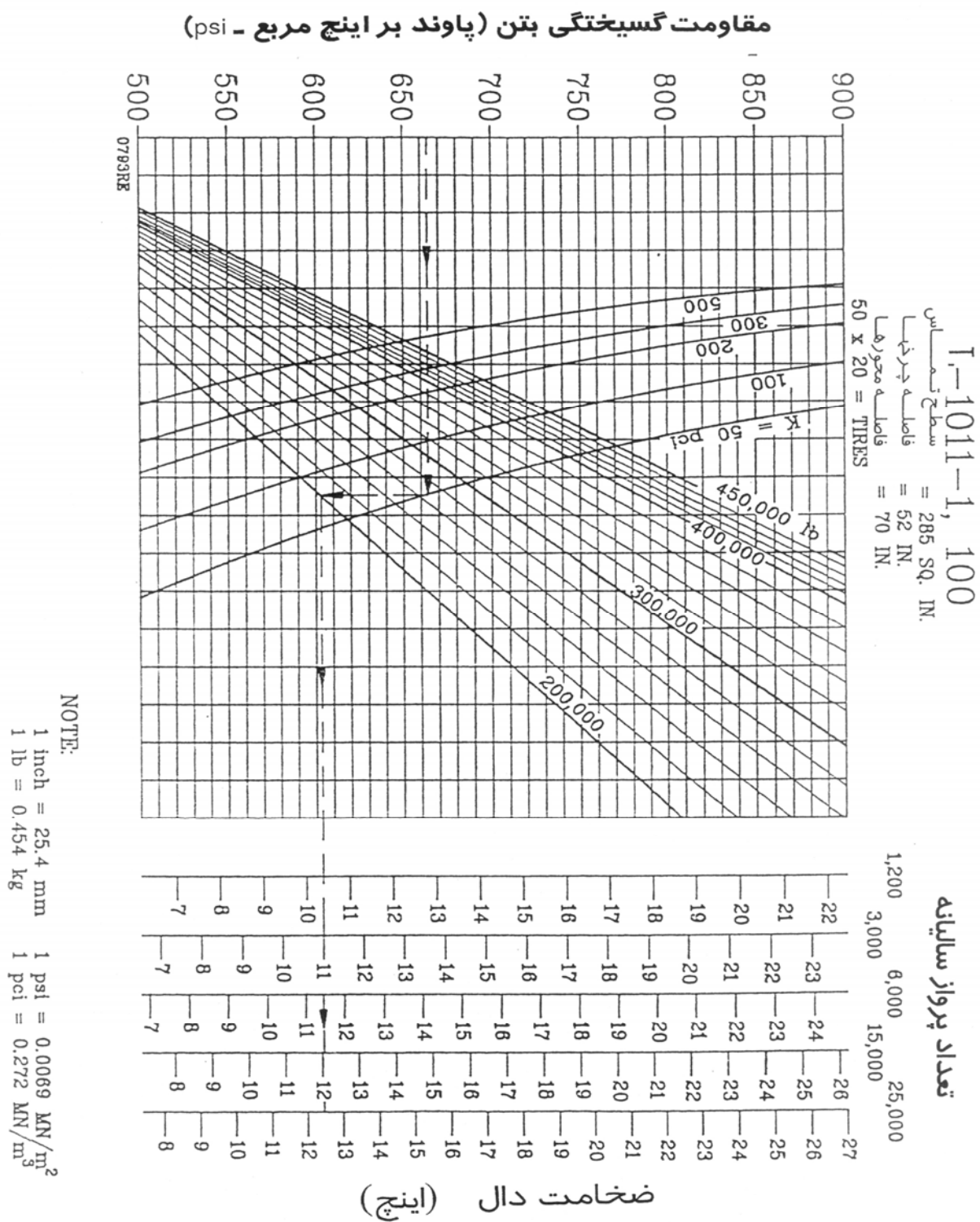
شکل (۳-۴) - منحنی انتخابی طرح روسازی صلب برای هواپیماهای L1011-100, 100
