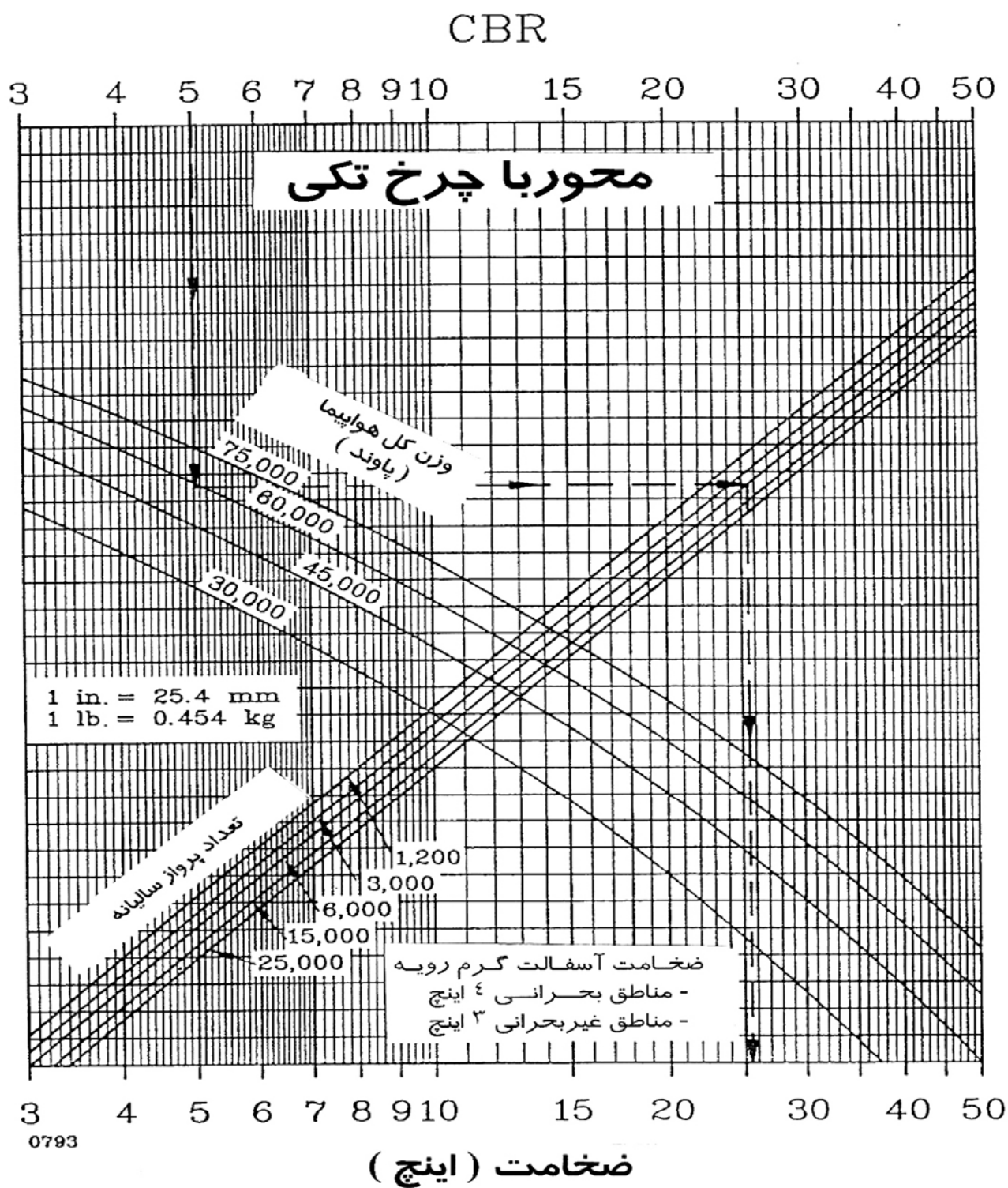
شکل (۲-۳) - منحنی طرح روسازی انعطاف پذیر برای چرخ تکی
