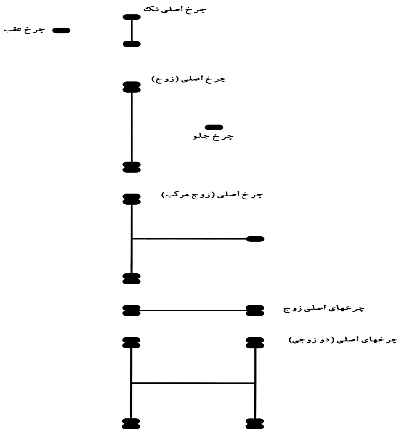
شکل (۳-۱) - آرایش انواع چرخهای هواپیما
