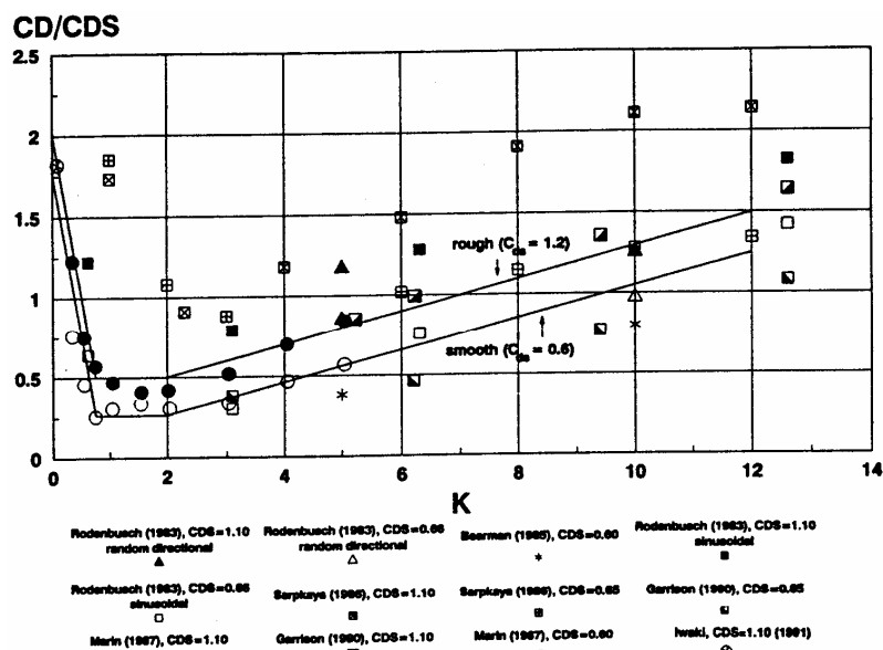
شکل پ-۶ ضریب درگ به صورت تابعی از K
