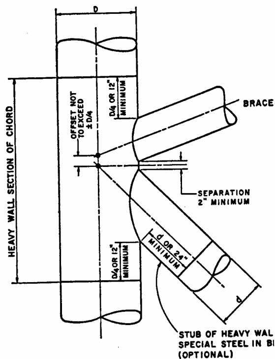
شکل ۳-۴ جزئیات اتصال لوله‌ای ساده
