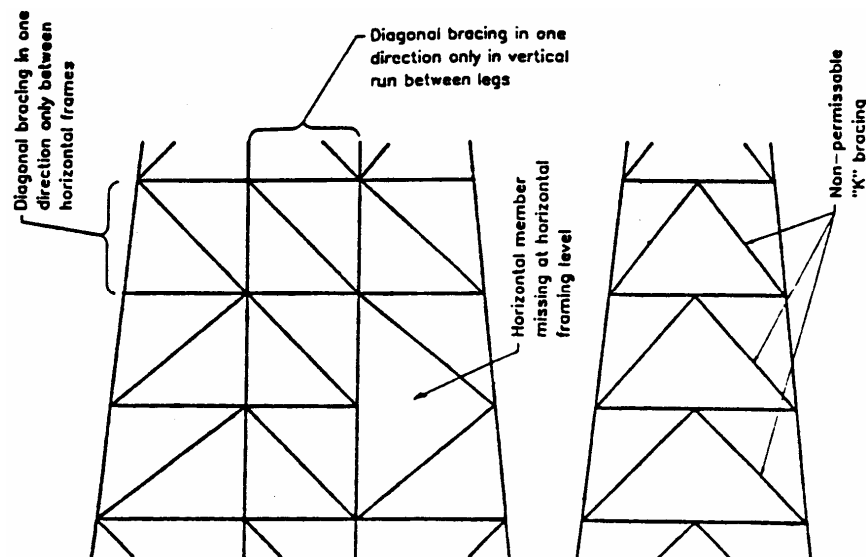
شکل ۲-۵ نمونه‌هایی از قابهایی که ضوابط بند ۲-۳-۴-۱ را اقلان نمی‌نماید.
