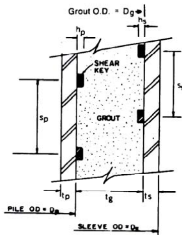
شکل ۱-۵ شمع تزریق شده به اتصال سازه، به همراه کلیدهای برشی
