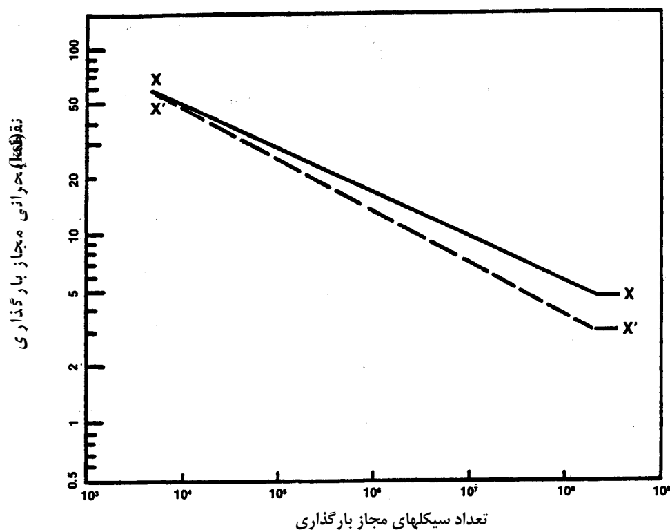
شکل ۳-۸ منحنی S-N برای تحلیل اتصالات لوله‌ای
