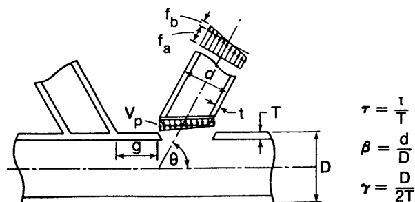
شکل ۲-۳ اتصال لوله‌ای ساده
