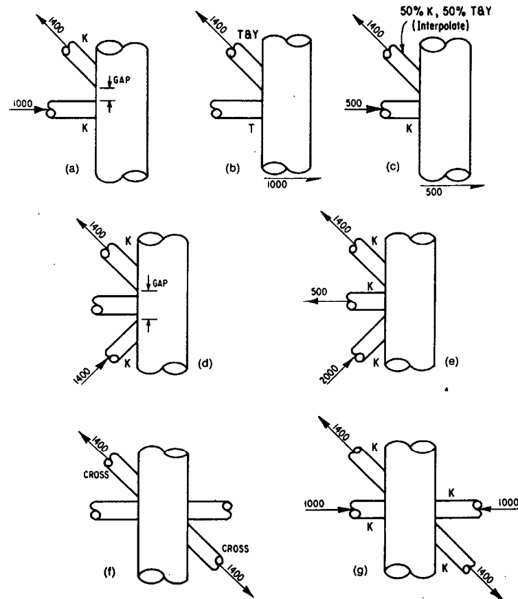
شکل ۳-۳ دسته‌بندی اتصالات لوله‌ای
