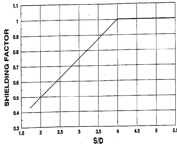
شکل ۳-۲ ضریب پوشش برای نیروهای موج وارد بر لوله‌های صورت تابعی از فاصله لوله‌ها
