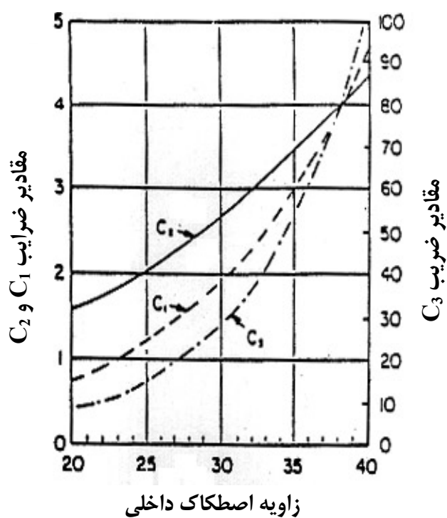
شکل ۴-۳ ضرایب C_1 ، C_2 و C_3
