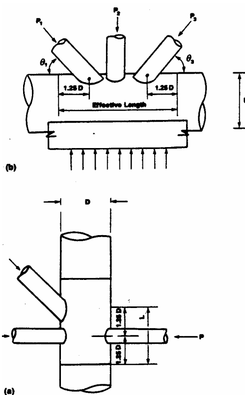
شکل ۳-۷ طول مؤثر عضو اصلی اتصالات لوله‌ای
