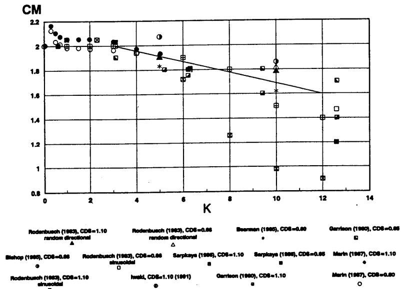
شکل پ-۷ ضریب اینرسی به صورت تابعی از K
