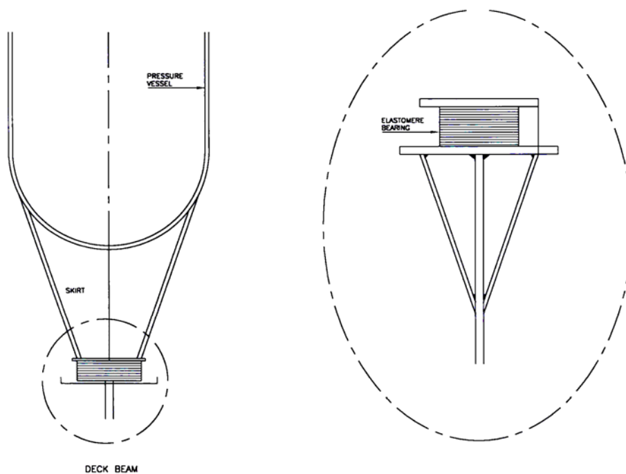
شکل ۵-۳ نحوه اتصال مخزن تحت فشار استوانه‌ای به عرشه
