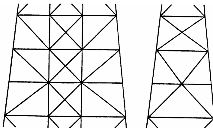
شکل ۲-۶ نمونه‌هایی از قاب‌هایی که ضوابط بند ۲-۳-۴-۴ را اقلان می‌نماید.
