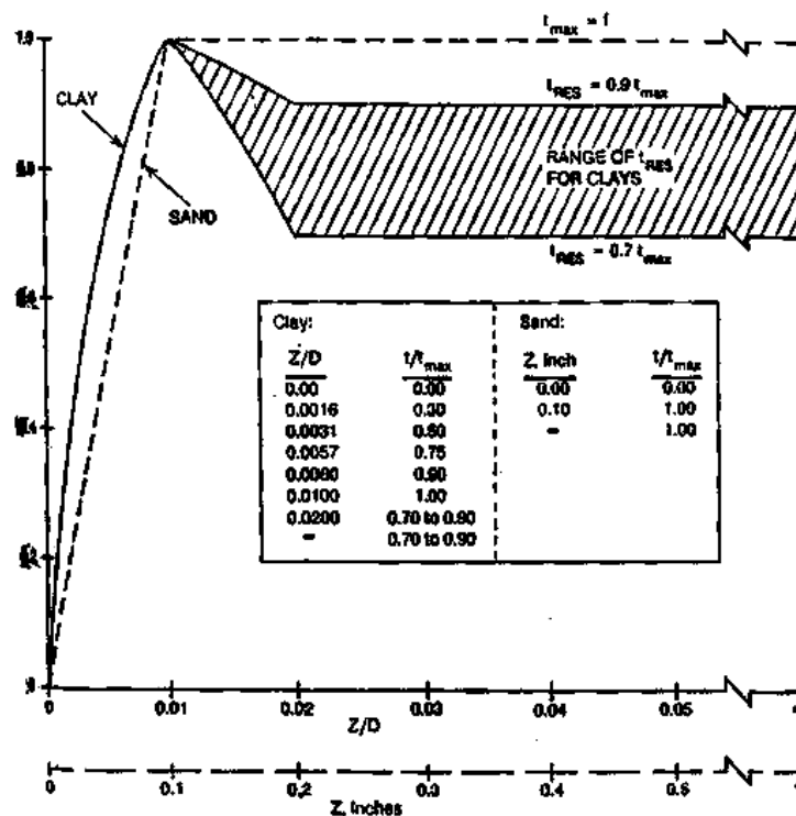
شکل ۴-۱ منحنیهای تیپ انتقال بار محوری - جابه‌جایی شمعها
