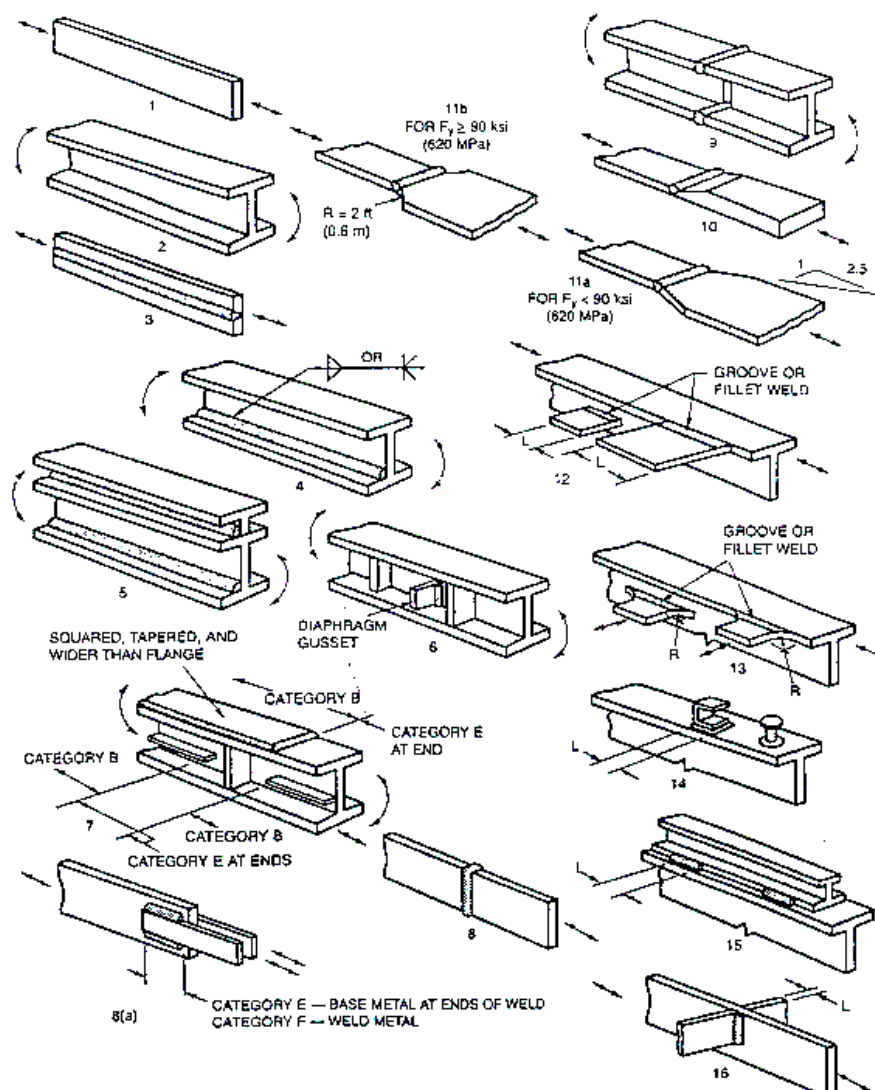
شکل ۳-۹ انواع اتصالات جوشی غیر لوله‌ای
