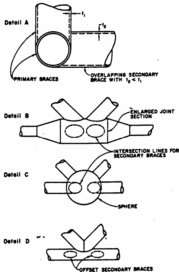
شکل ۳-۶ اتصالات متراکم
