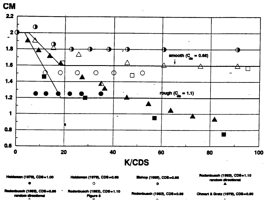
شکل پ-۸ ضریب اینرسی به صورت تابعی از K/C_{DS}
