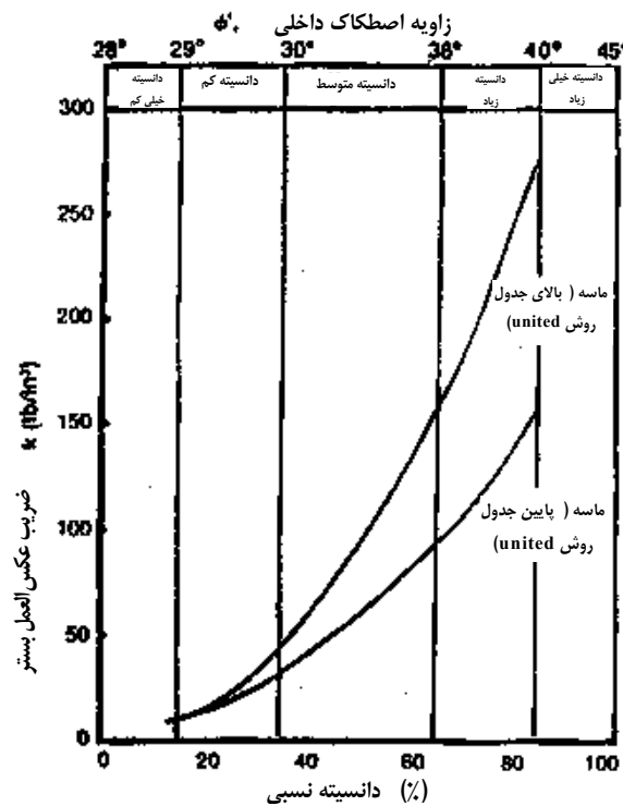
شکل ۴-۴ ضرایب بستر
