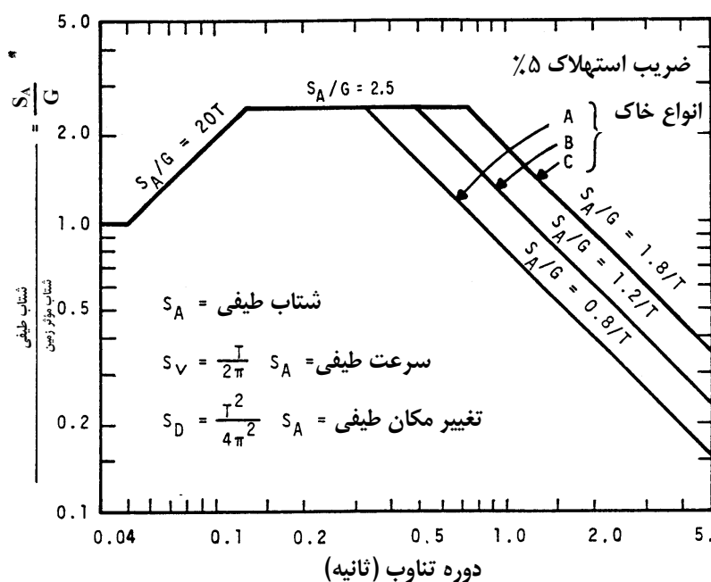
شکل ۲-۴ طیفهای پاسخ به مقیاس در آمده
