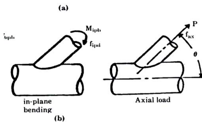
شکل ۳-۱۳ حالت‌های بارگذاری و نقاط بحرانی در اتصالات لوله‌ای
