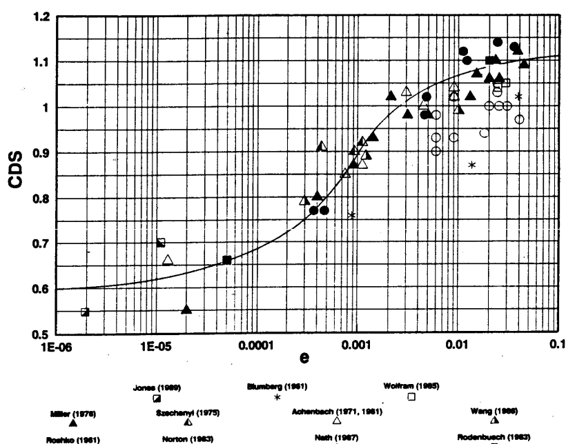
شکل پ-۴ وابستگی ضریب درگ جریان دایم به زبری سطحی نسبی
