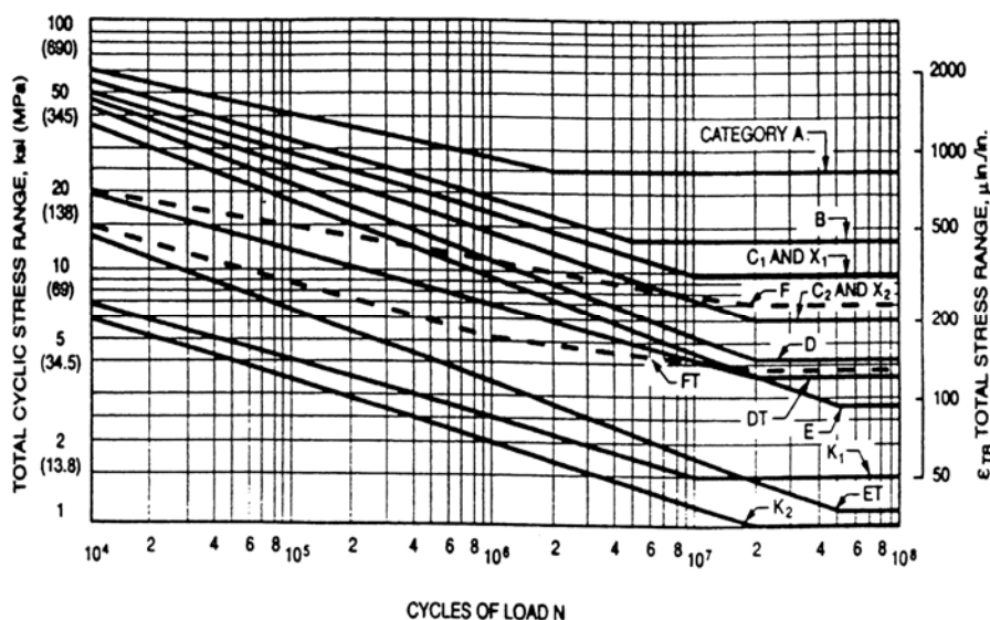
شکل ۳-۱۲ منحنیهای S-N برای اتصالات جوشی در اعضای لوله‌ای (به استثنای اتصالات لوله‌ای) برای سرویس در شرایط اتمسفری
