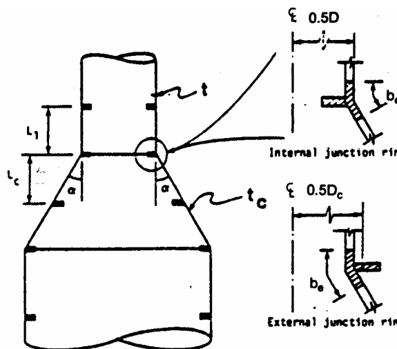
شکل ۳-۱ تبدیل مخروطی
