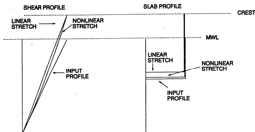
شکل پ-۲ دامنه کاربرد تئوریهای مختلف امواج
