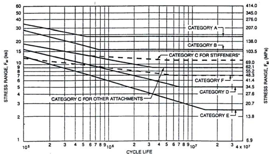
شکل ۳-۱۱ منحنیهای S-N برای اتصالات غیر لوله‌ای در اجزای فاقد درجه نامعینی برای سرویس در شرایط اتمسفری
