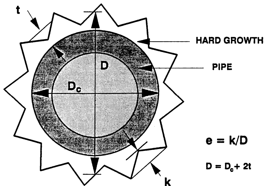
شکل پ-۳ ارتفاع و ضخامت زبری سطح
