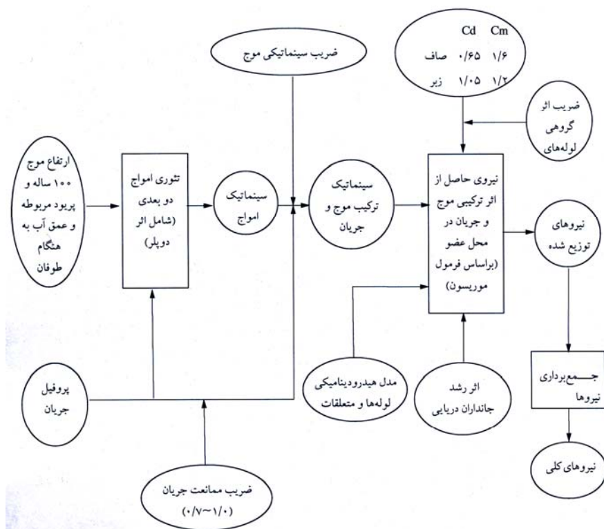
شکل ۲-۱ روش انجام محاسبات نیروهای حاصل از ترکیب موج و جریان در تحلیل استاتیکی
