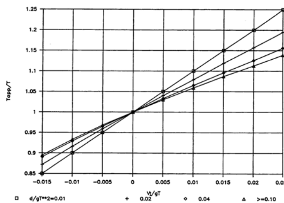
شکل ۲-۲ تغییرات دوره تناوب ظاهری موج بر اثر جریان
