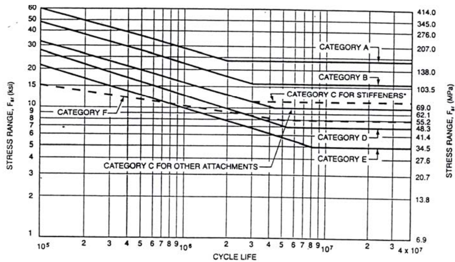
شکل ۳-۱۰ منحنیهای S-N برای اتصالات غیر لوله‌ای در اجزای دارای درجه نامعینی برای سرویس در شرایط اتمسفری
