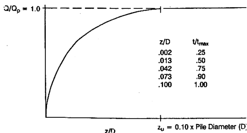
شکل ۲-۴ منحنی جابه‌جایی - مقاومت نوک شمع
