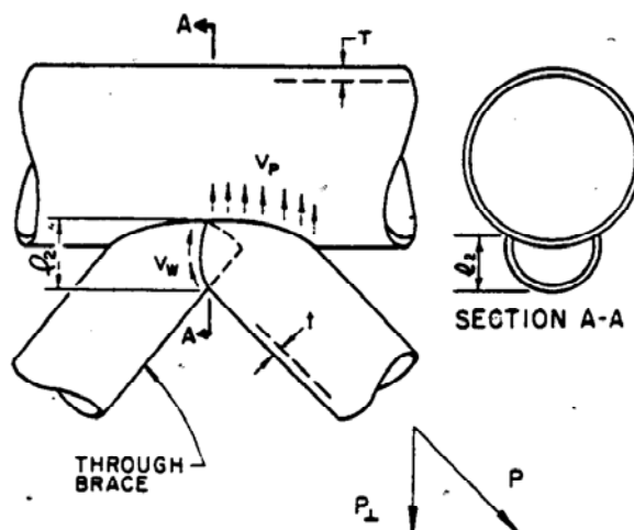
شکل ۳-۵ اتصالات لوله‌ای همپوشان
