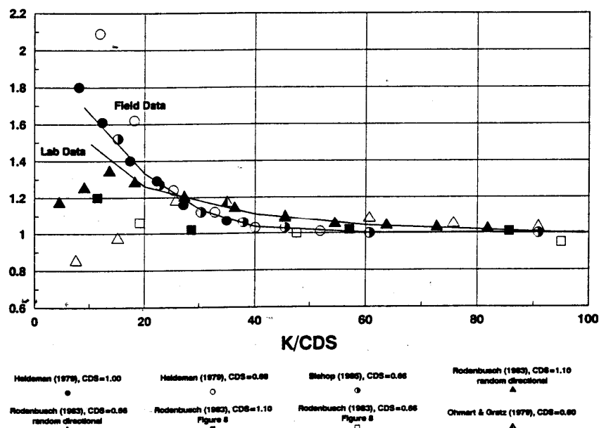
شکل پ-۵ ضریب درگ به صورت تابعی از K/CDS
