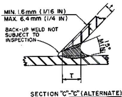
شکل ۷-۱ جزئیات اتصالات جوشی لوله‌ای
