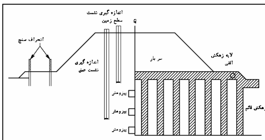
شکل ۷-۲: زهکش قائم در ترکیب با پیش‌بارگذاری
