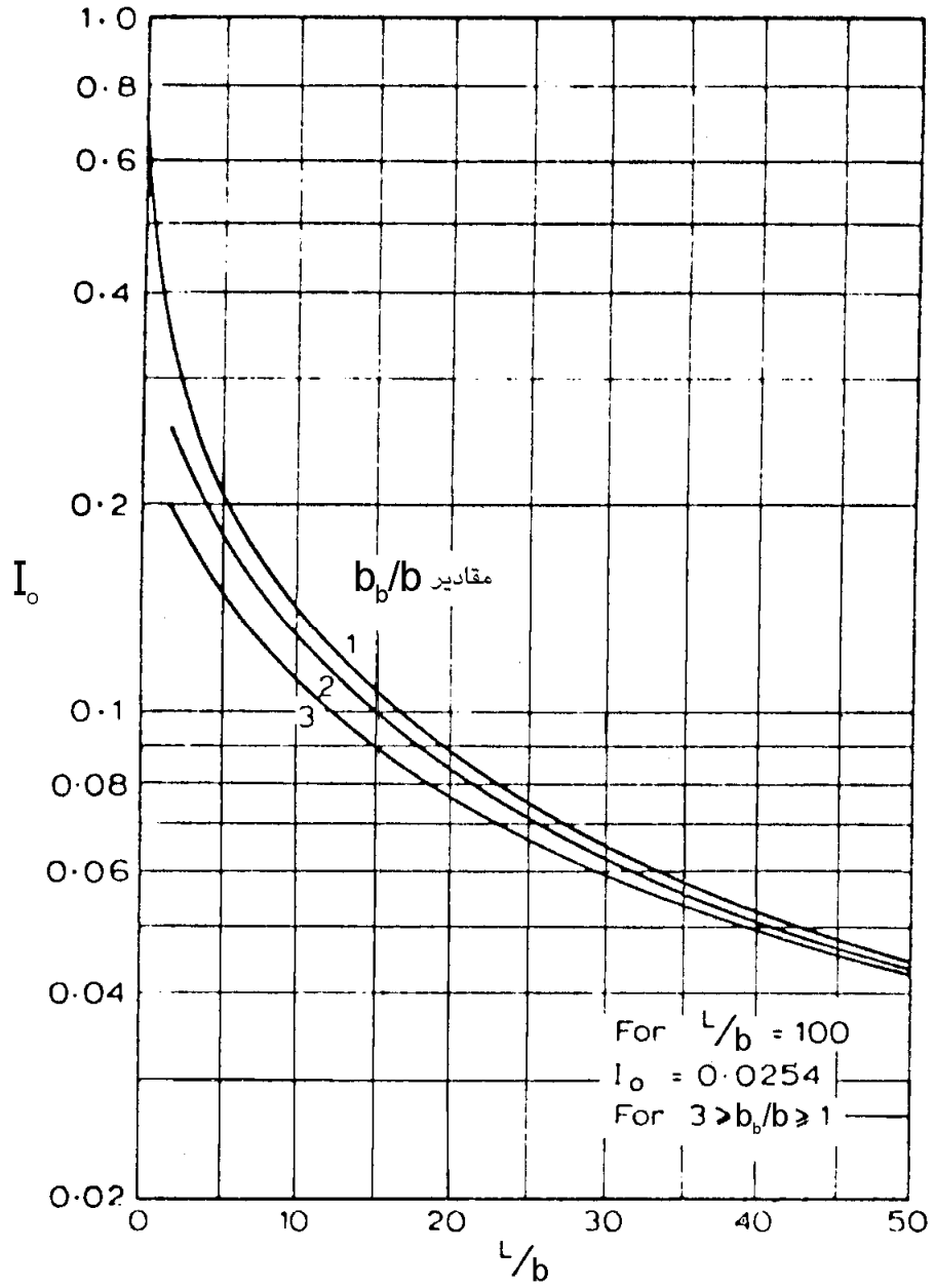
شکل ۳-۷ ضریب تأثیر نشست I_0
