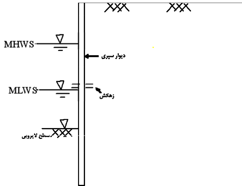
شکل ۳-۶ دیوار سپری طره‌ای
