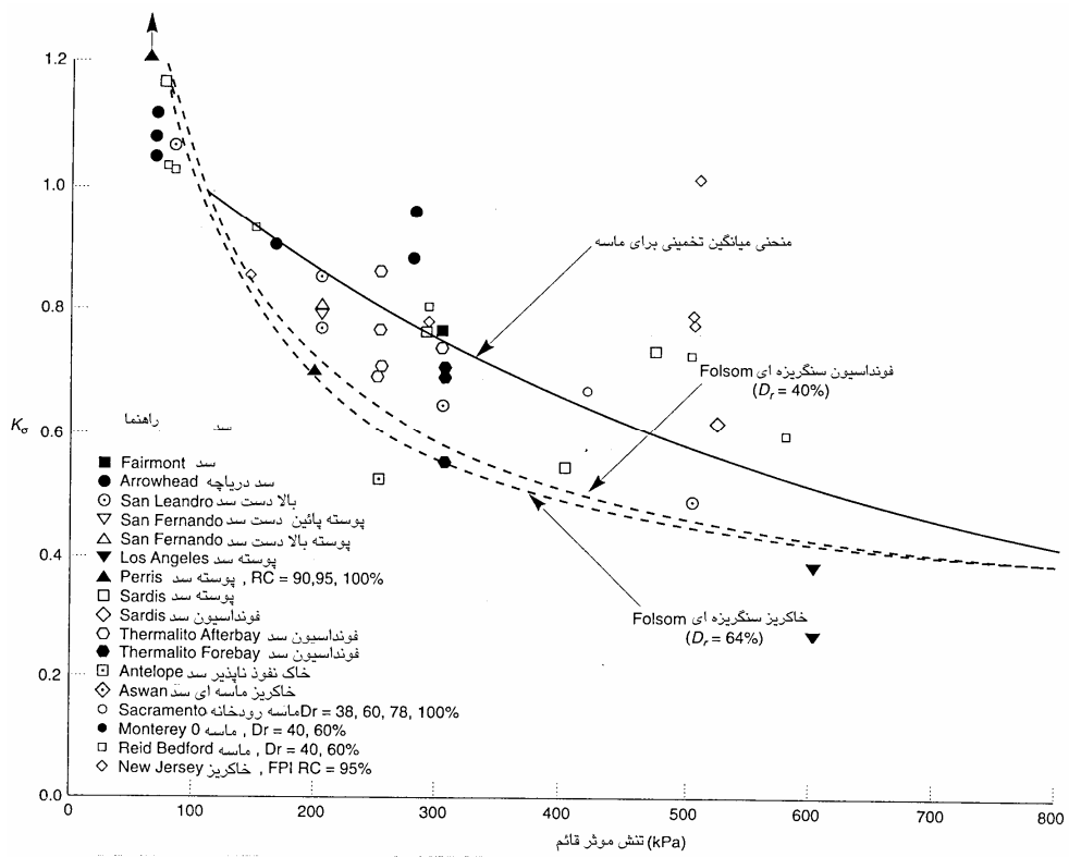
شکل ۳-۴ تغییرات ضریب اصلاح تنش برشی بر حسب نسبت تنش برشی اولیه به تنش مؤثر قائم
