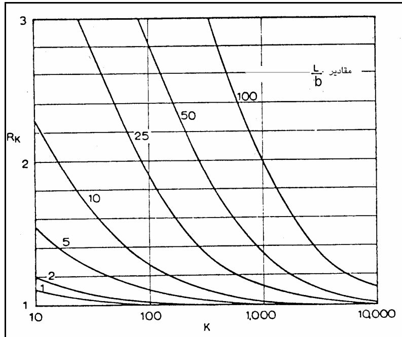
شکل ۳-۸ تغییرات ضریب اصلاح تراکم‌پذیری R_k نسبت به K = \frac{R_A E_P}{E_S}
