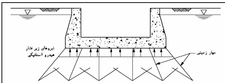
شکل ۶-۸ مهارهای تزریقی عمودی و مایل در زیر کف سازه‌های زیرزمینی برای مقابله با نیروهای زیر فشار
