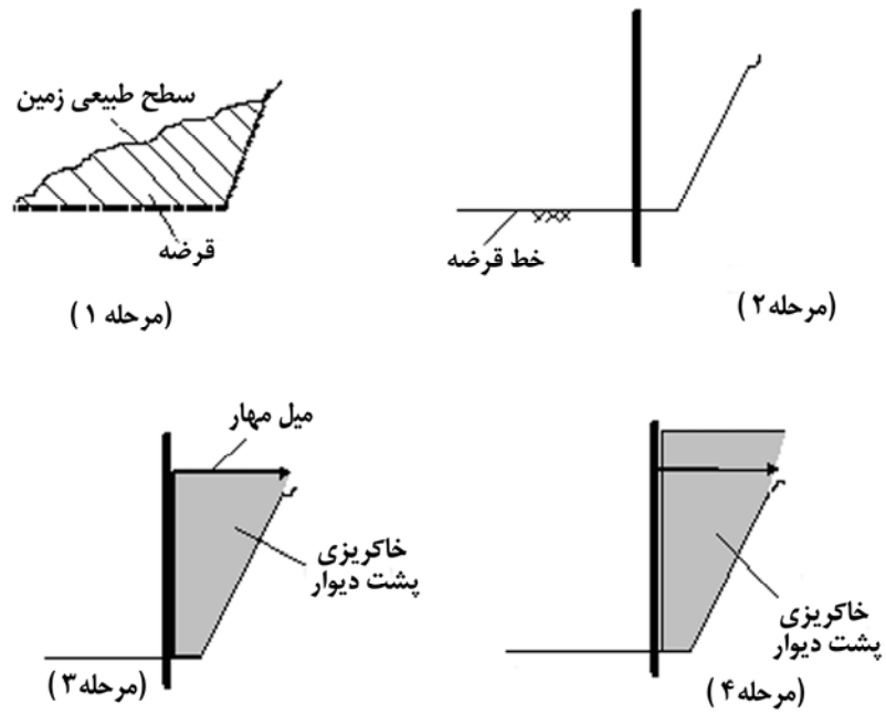
شکل ۴-۶ مراحل مختلف اجرای دیوار در حالت خاکریزی شده
