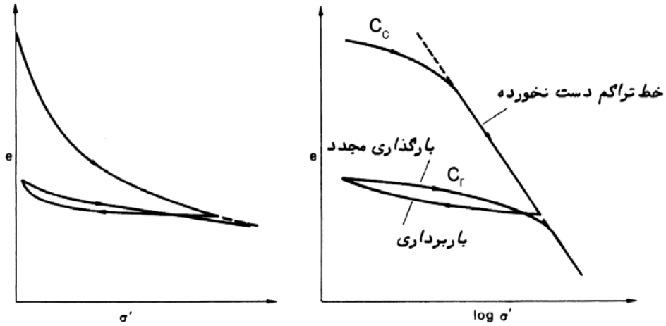
شکل ۲-۶ نمودار تحکیم اولیه و ثانویه
