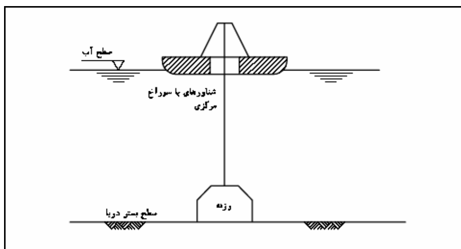
شکل ۵-۷ تحکیم دینامیکی در دریا
