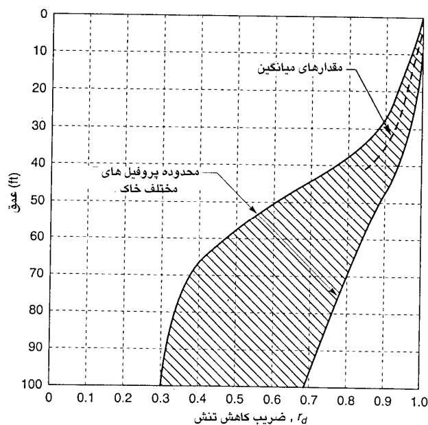
شکل ۴-۱ ضریب کاهش تنش در عمق
