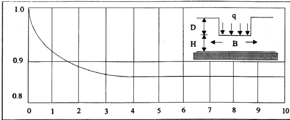
شکل ۲-۳ ضریب تأثیر زرفای پی
