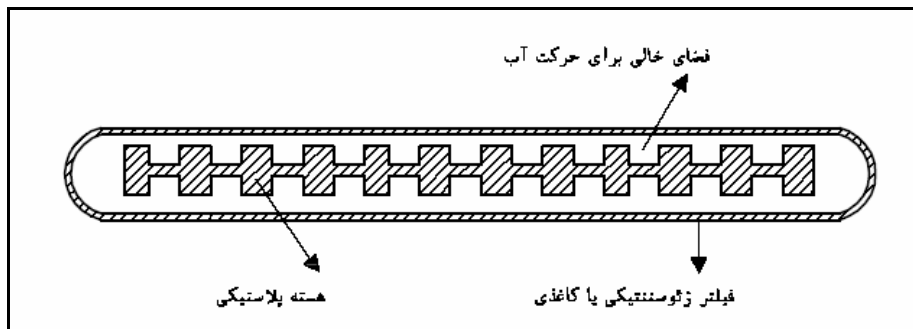
شکل ۷-۴ مثالی از مقطع یک نوار زهکش
