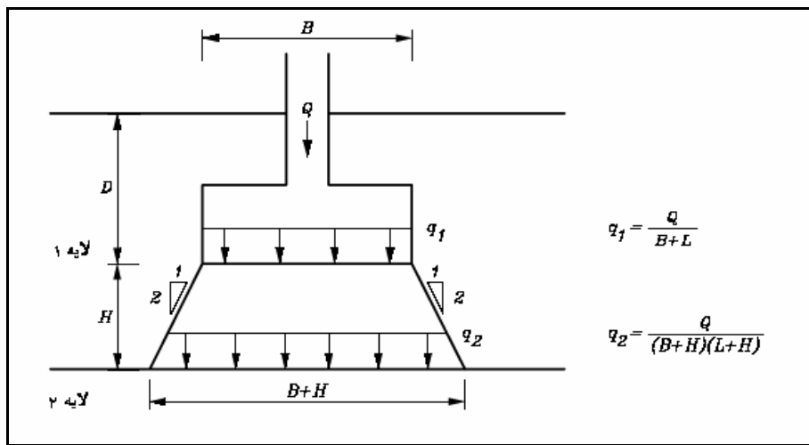
شکل ۲-۲ توزیع تنش زیر پی برای لایه اول و دوم
