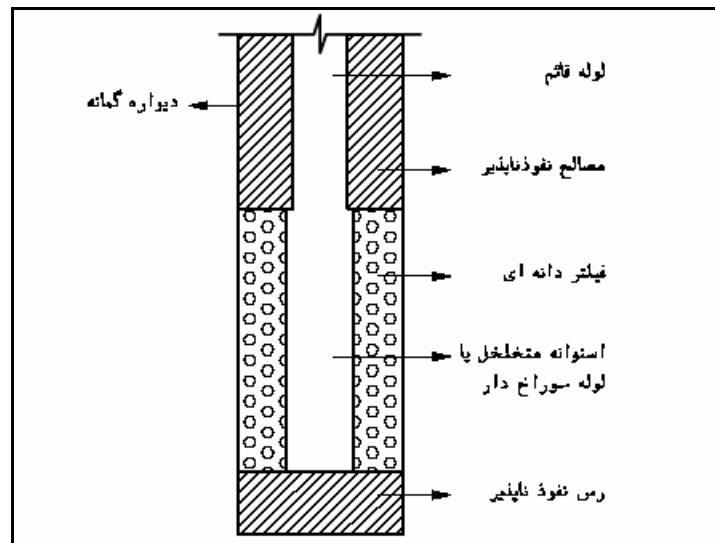
شکل ۱-۸ طرح شماتیک یک پیزومتر لوله‌ای قائم
