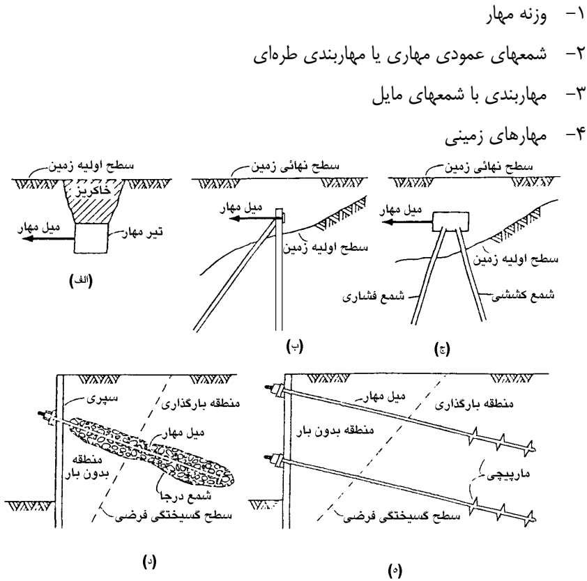
شکل ۶-۶ انواع مهاربندی
