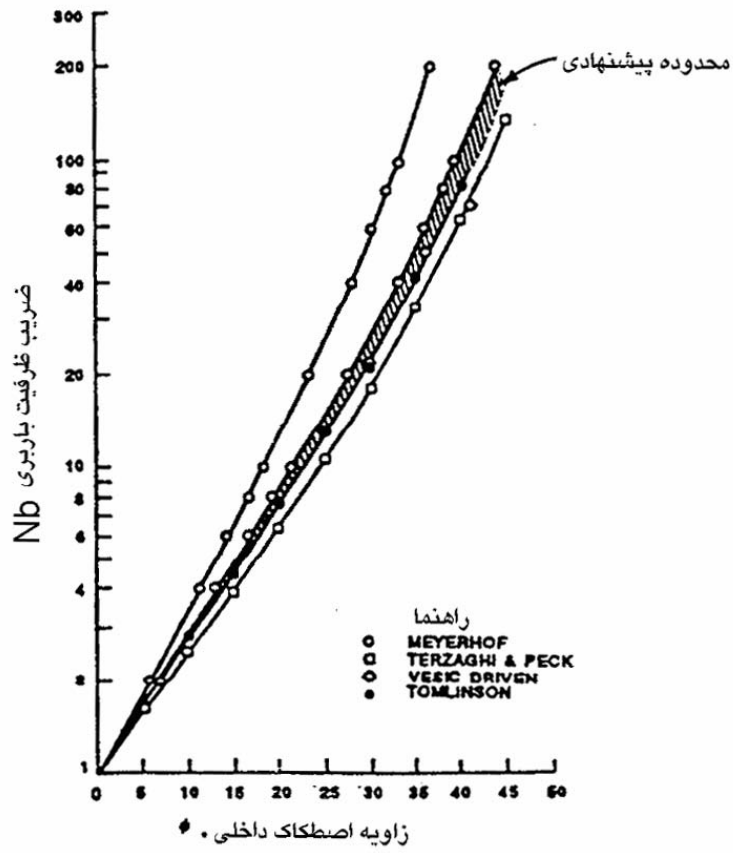
شکل ۳-۱ ضریب باربری نوک شمع
