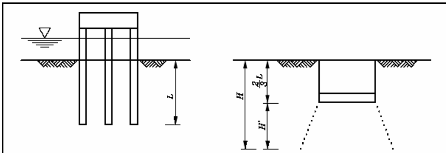
شکل ۱-۱ تعیین عمق گمانه برای گروه شمع (H' عمق گمانه برای پی فرضی، H عمق گمانه برای گروه شمع و L طول شمع می‌باشد)
