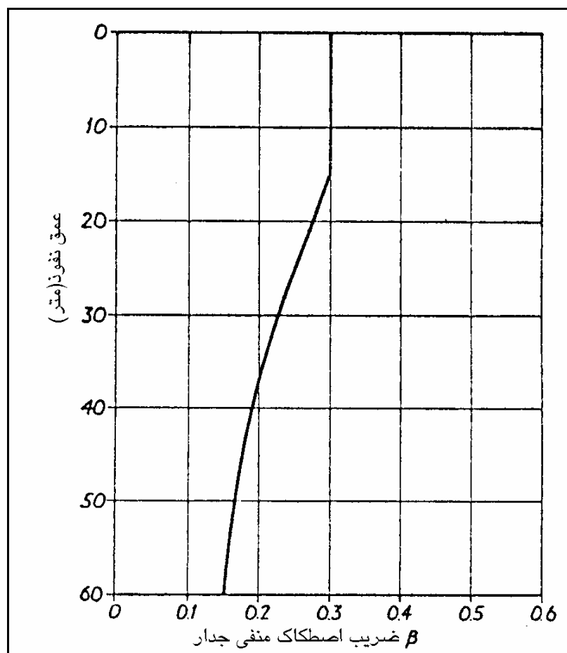
شکل ۳-۶ ضریب اصطکاک منفی جدار ( \beta ) برای شمعهای کوبیده شده در خاک رس
