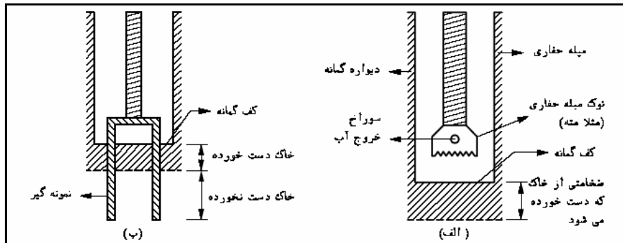
شکل ۱-۵ دست‌خوردگی خاک زیر گمانه (الف) در اثر حفاری، بخشی از خاک زیر گمانه دست‌خورده می‌شود. (ب) در اثر حفاری خاک دست‌خورده وارد نمونه‌گیر می‌شود.
