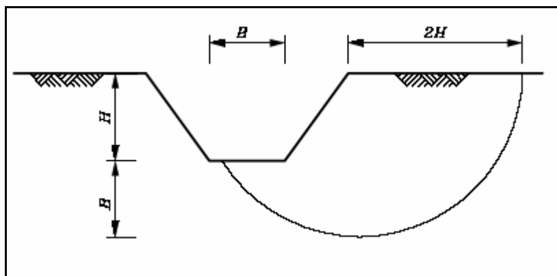
شکل ۳-۱ عمق گمانه برای گودبرداری‌ها
