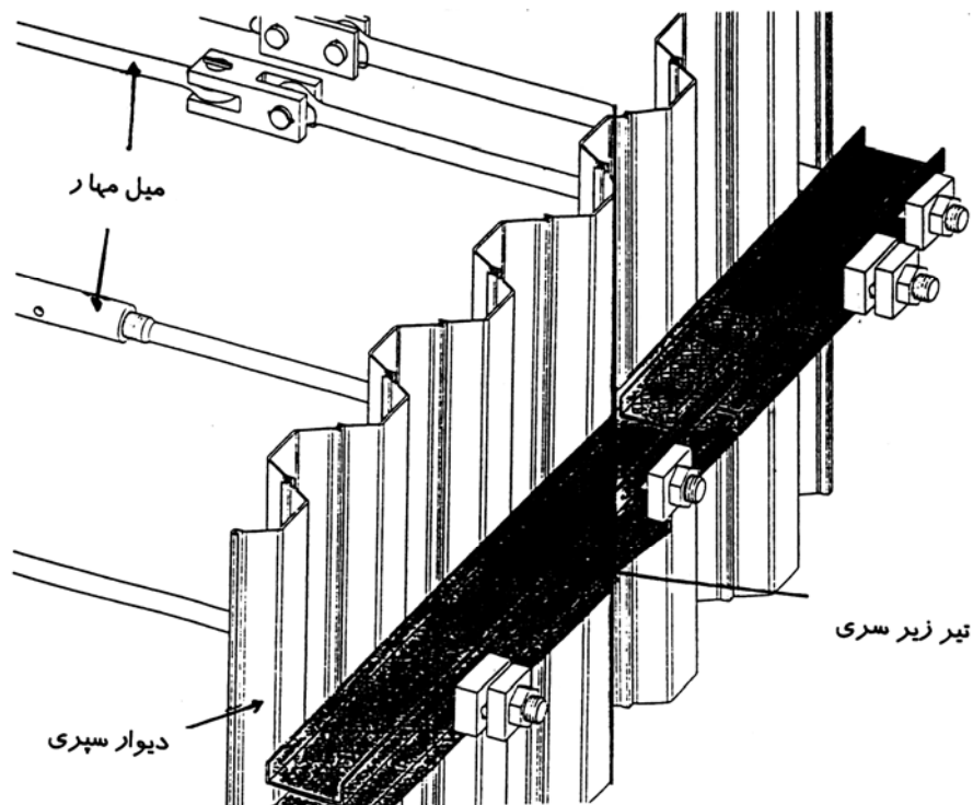
شکل ۶-۱۰ تیر زیر سری (تیر پشت‌بند) و میل مهار
