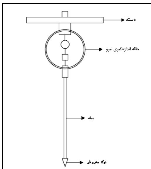
شکل ۱-۷ زمین کاو استاتیکی ساده
