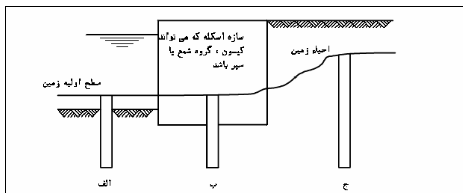
شکل ۴-۱ محل گمانه‌ها در امتداد عرضی، (الف) گمانه‌های جلوسازه، (ب) گمانه‌های زیرسازه و (ج) گمانه‌های پشت سازه
