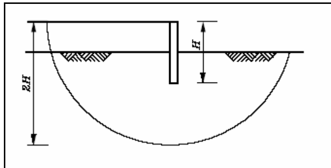
شکل ۱-۲ عمق گمانه برای ابنیه نگهدارنده خاک
