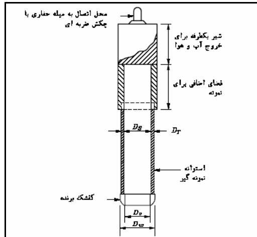
شکل ۹-۱ جزئیات اصلی نمونه گیر استوانه‌ای ته باز
