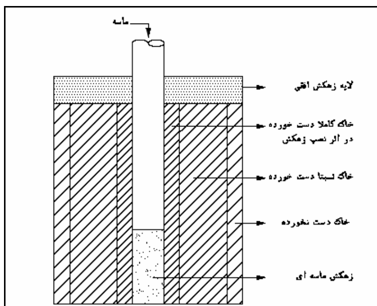
شکل ۷-۳ نصب زهکش قائم ماسه‌ای با لوله فلزی
