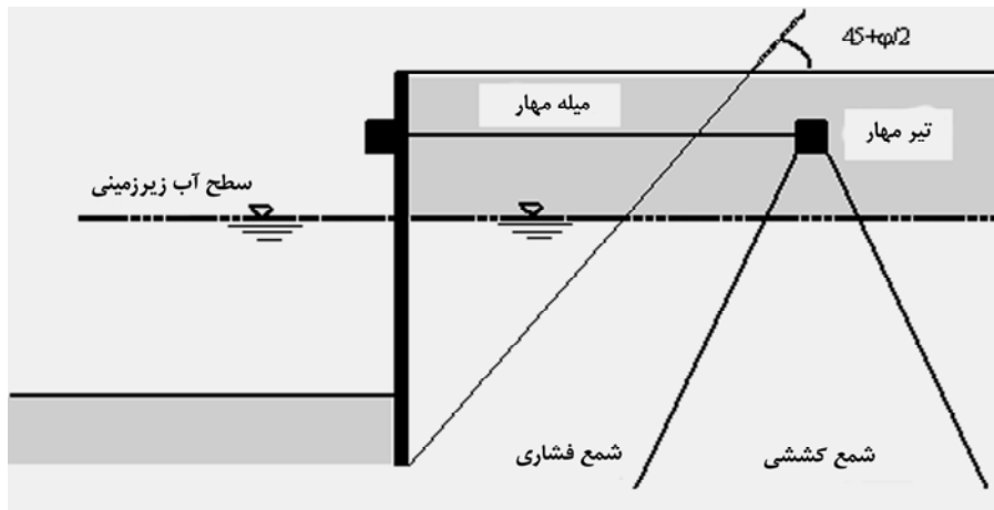
شکل ۶-۹ مهاربندی با شمعهای مایل
