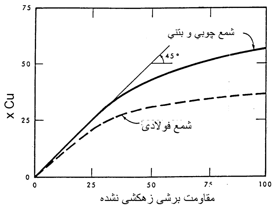
شکل ۳-۲ مقاومت سطح جانبی شمعها در رس
