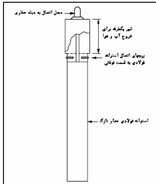
شکل ۱۰-۱ نمونه گیر جدار نازک
