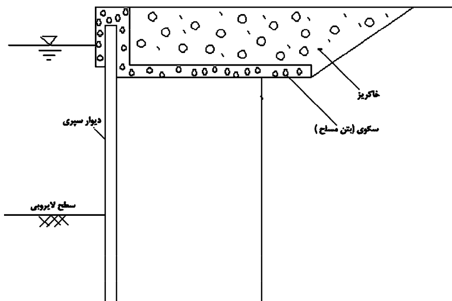
شکل ۶-۲ دیوار سپری با سکوی کاهنده
