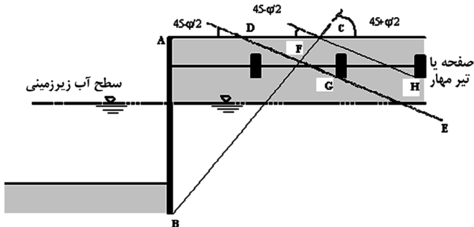
شکل ۶-۷ انواع قرارگیری میل‌مهار درون و خارج منطقه گسیختگی
