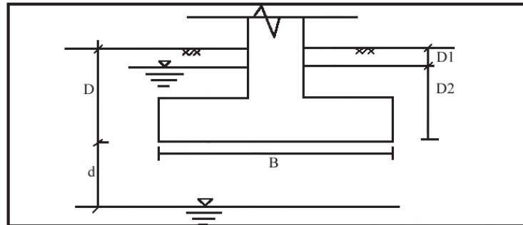
شکل ۱-۲ ترازهای مختلف سطح آب زیرزمینی نسبت به پی
