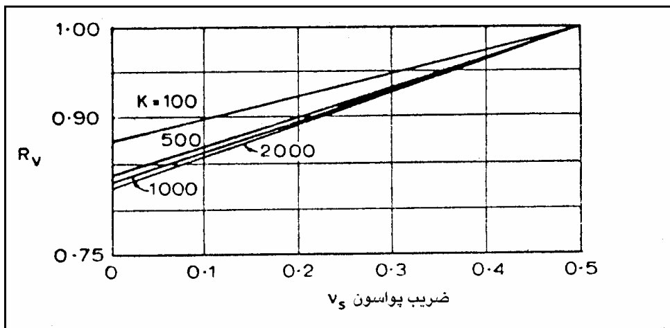
شکل ۳-۹ ضریب اصلاح نسبت پواسون، R_v
