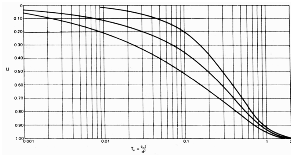
شکل ۲-۸ رابطه بین درجه تحکیم و ضریب زمان
