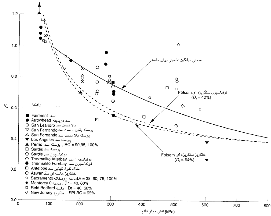
شکل ۴-۴ تغییرات ضریب اصلاح فشار مؤثر قائم بر حسب تنش مؤثر قائم
