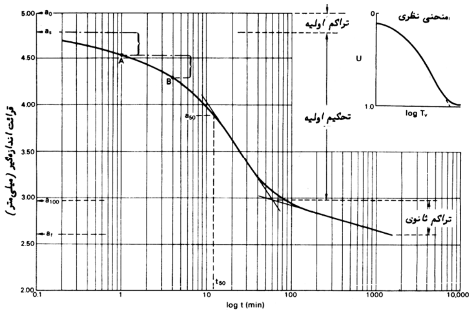
شکل ۲-۷ روش لگاریتم زمان
