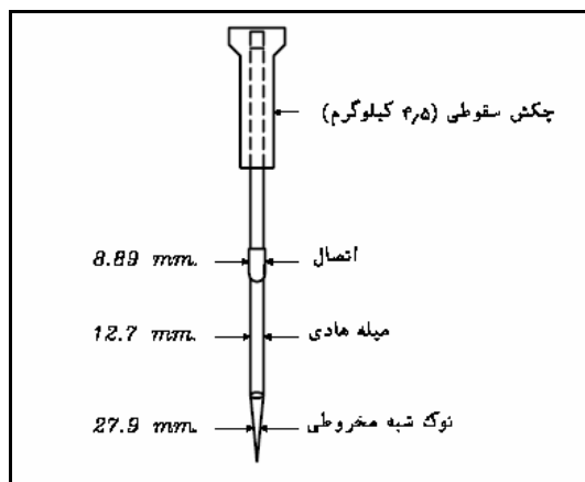
شکل ۱-۶ زمین کاو مکینتاش
