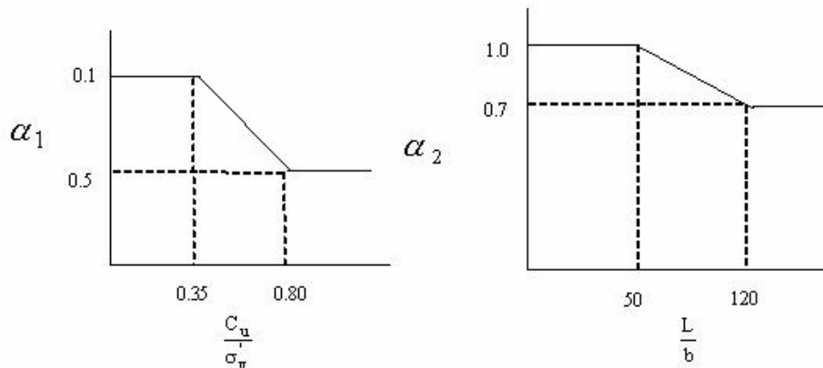
شکل ۳-۳ مقادیر \alpha_1 و \alpha_2 برای شمعیهای طویل (L طول شمع و b قطر شمع می‌باشد).
