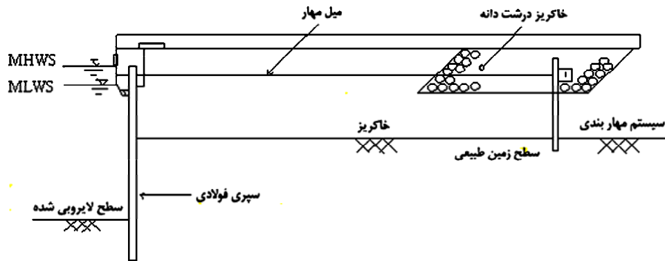
شکل ۶-۱ دیوار سپری مهار شده
