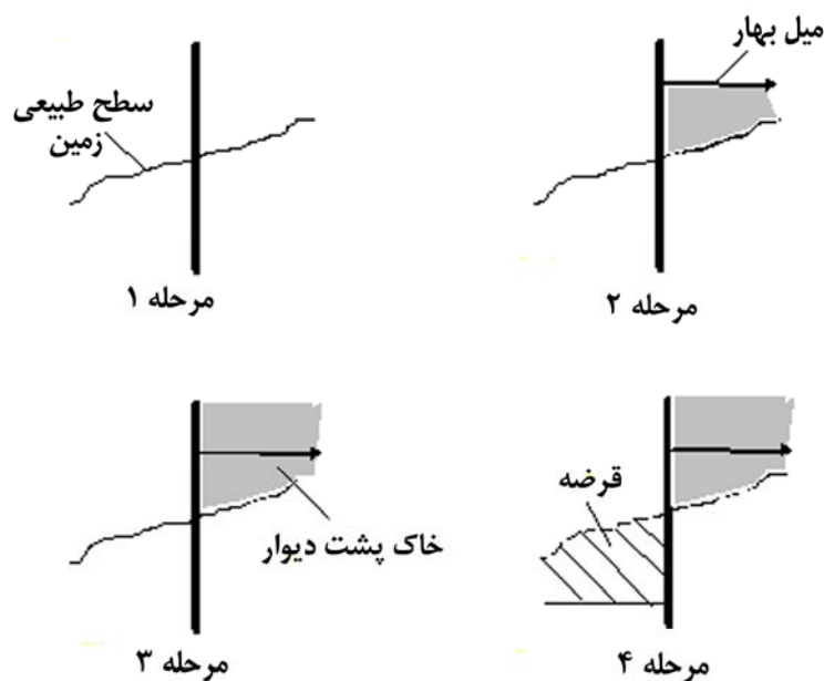
شکل ۵-۶ مراحل مختلف اجرای دیوار در حالت لایروبی شده
