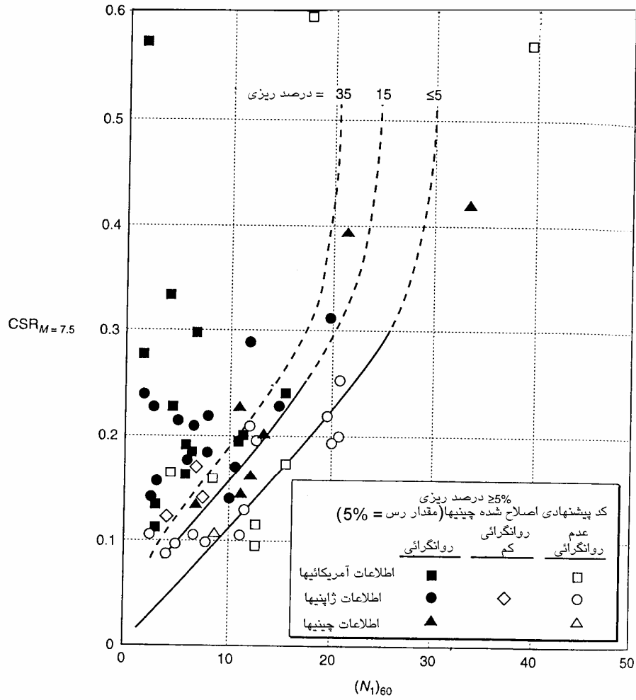
شکل ۴-۲ ارتباط بین مقاومت نفوذ استاندارد اصلاح شده و نسبت تنش سیکلی مقاوم برای زلزله‌ای به بزرگی ۷/۵ ریشتر
