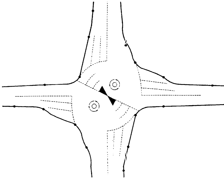
شکل ۷-۲- دو میدان کوچک همسطح که با ده فضای گردش عمودی بزرگ به یکدیگر مرتبط است.
