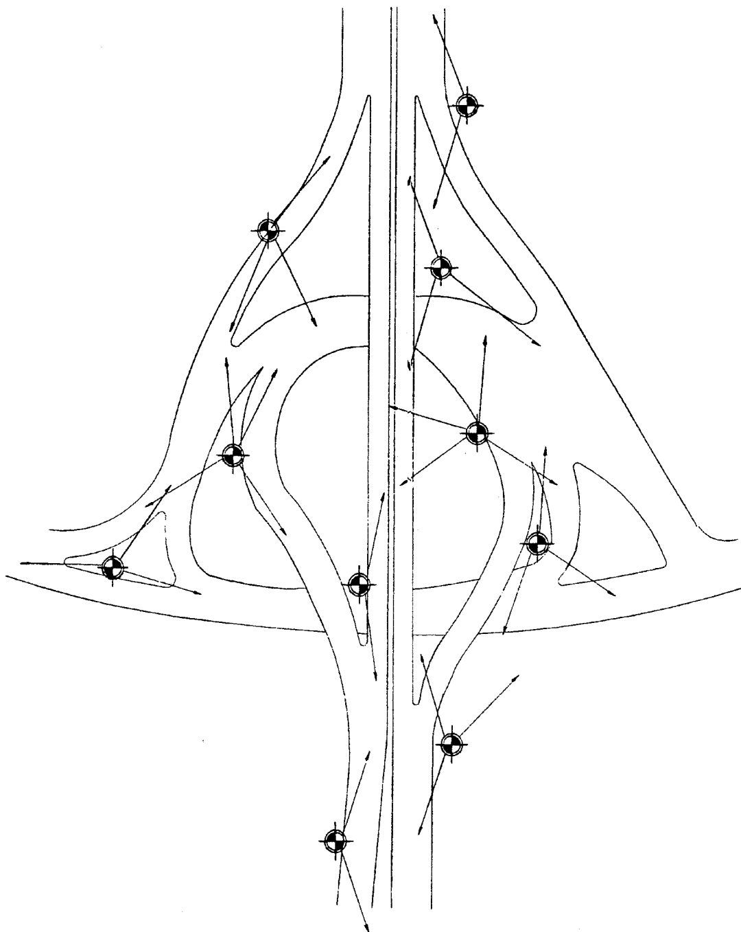
شکل ۸-۴- طرح نمونه‌ای از روشنائی تقاطعهای غیرهمسطح پیچیده با استفاده از پایه‌های بلند (توجه: فلشها، نشان‌دهنده جهت شعاع اصلی نور خروجی از چراغهای مستقر بر پایه بوده و تعداد آن ارتباطی به چراغهای نصب شده، ندارد)
