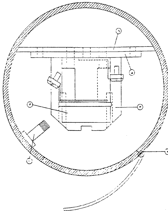
شکل ۱۲-۱۳- طرح نمونه جعبه تقسیم پایه‌های فلزی
