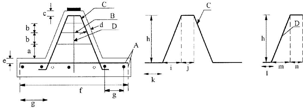
شکل ۱۳-۱۵- آرماتورهای فونداسیونها
