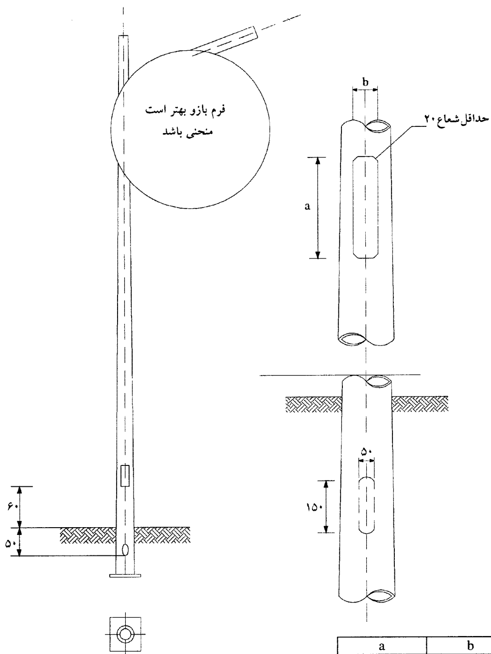
شکل ۱۳-۵- موقعیت محل جعبه فیوز
