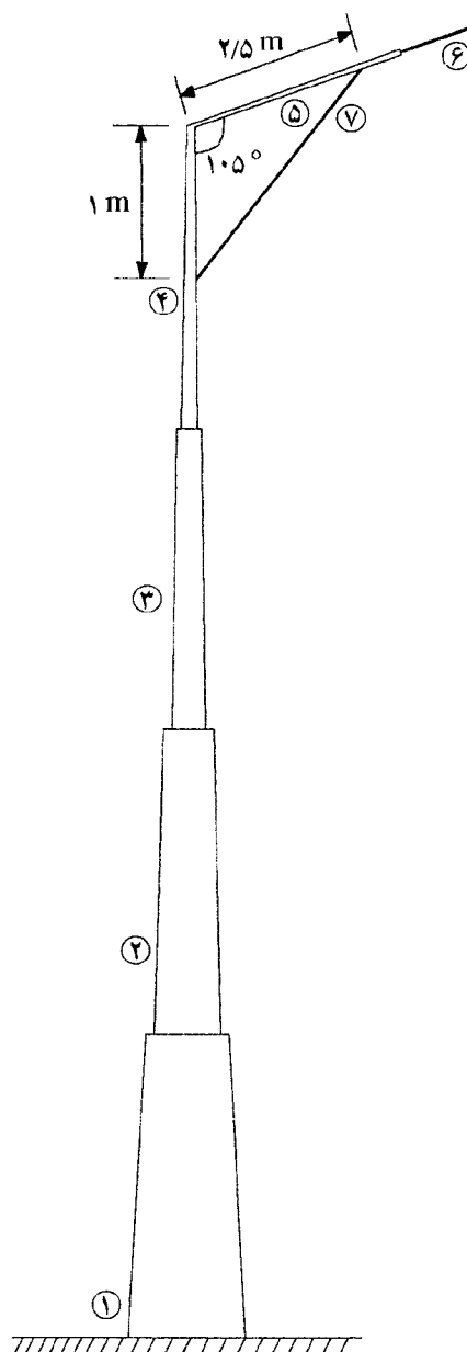
شکل ۱۳-۱۰- شماره قطعات مختلف پایه
