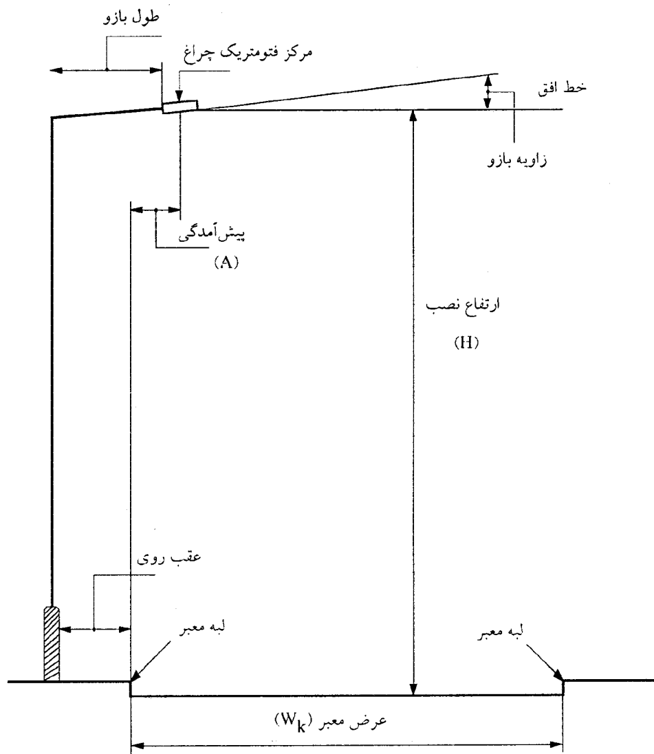
شکل ۱-۱- مشخصات قسمتهای مختلف پایه
