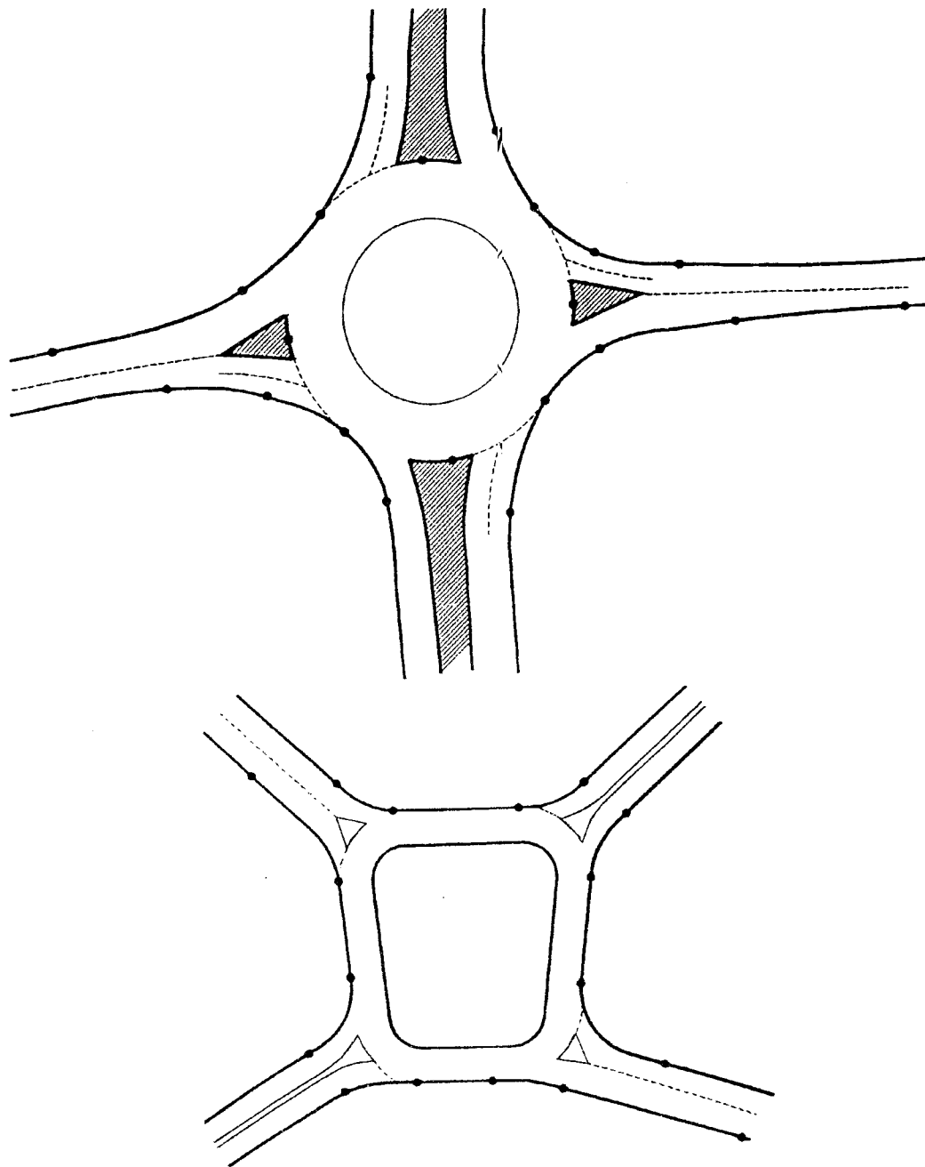
شکل ۷-۴- مثالهایی از میدین واقع در تقاطعهای چهار راه
