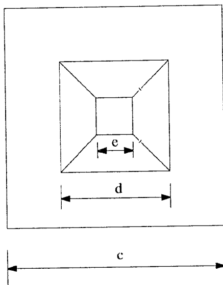
شکل ۱۳-۱۴- ابعاد فونداسیون‌ها
