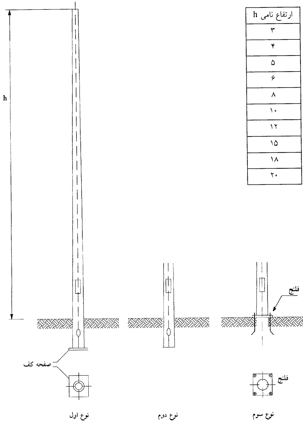
شکل ۱۳-۳- ابعاد اصلی پایه‌های بدون بازو (متر)
