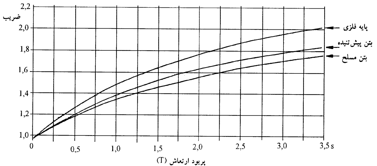
شکل ۱۳-۱- ضریب \beta برحسب پر یود ارتعاش پایه
