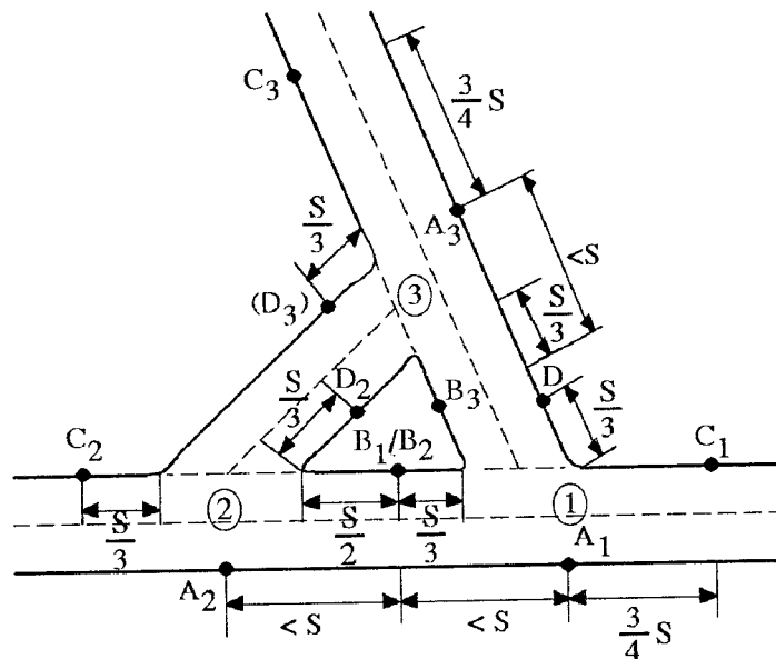
شکل ۶-۶-ب- تقاطع با جزیره ترافیکی مثلی
