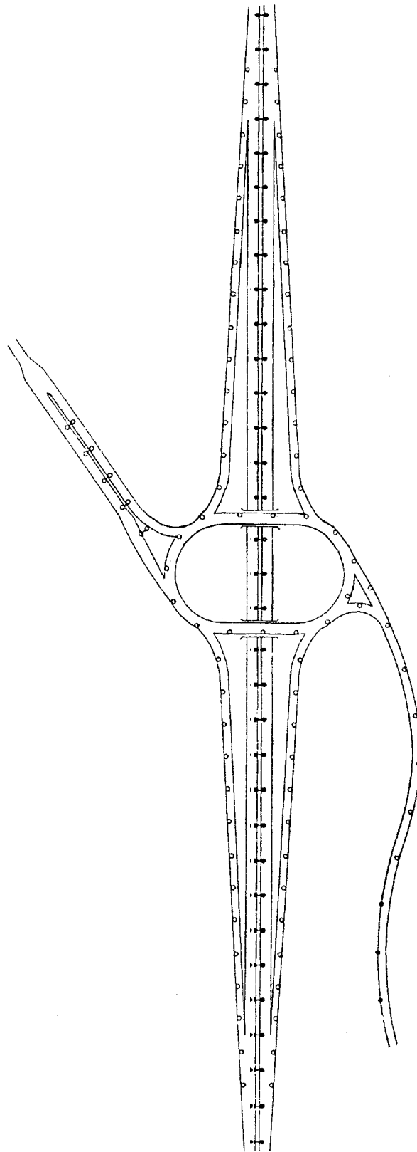
شکل ۸-۲- نمونه‌ای از طرح تامین روشنایی کامل تقاطع غیرهمسطح ساده
