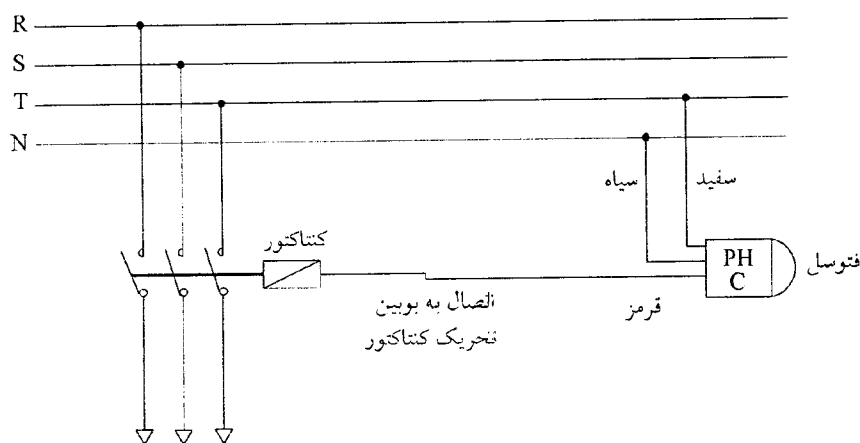
بطرف فیدرهای خروجی تغذیه روشنایی معابر
