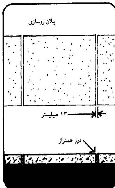
شکل ۳-۱۶- حداکثر عرض درز اجرایی رویه پیاده رو
