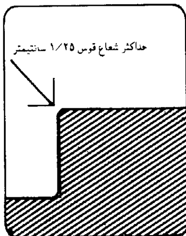
۳-۳۰- جزئیات دماغه پله
