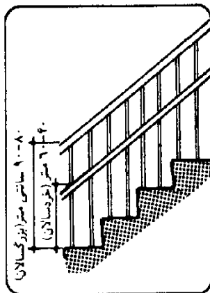
شکل ۳-۳۳- ارتفاع دستگیره و نرده پله و شیپراه
