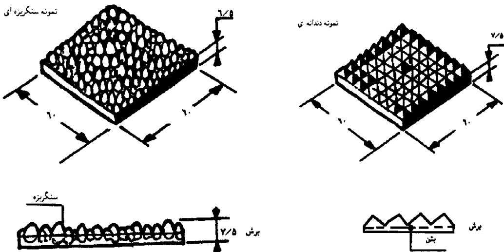
شکل ۳-۲۰- نمونه هایی از رویه درشت بافت پیاده رو (ابعاد به سانتیمتر)
