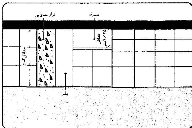
۳-۱۲- پله و شیبراه در پیاده رو
