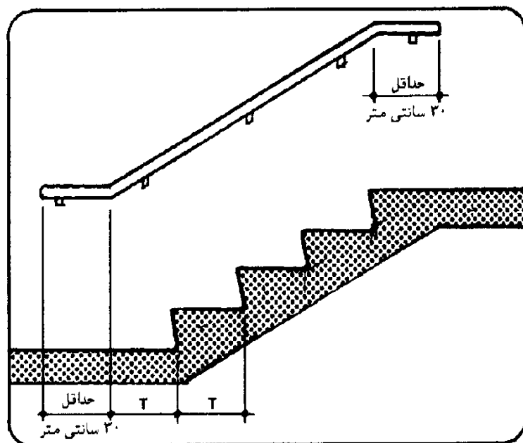
شکل ۳-۲۴- دنباله دستگیره
