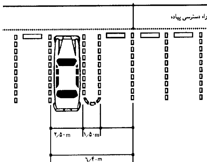
شکل ۳-۶۳- ابعاد فضای پارکینگ
