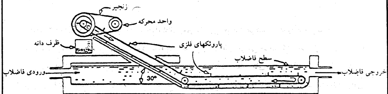
شکل ۱- مقطع یک حوض دانه‌گیری به روش تسمه نقاله و مجهز به زنجیر و پارونکهای جمع‌کننده دانه
