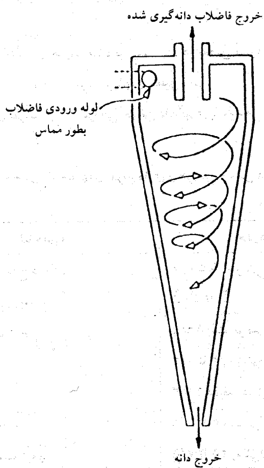
شکل ۴- دانه گیر سیکلونی
