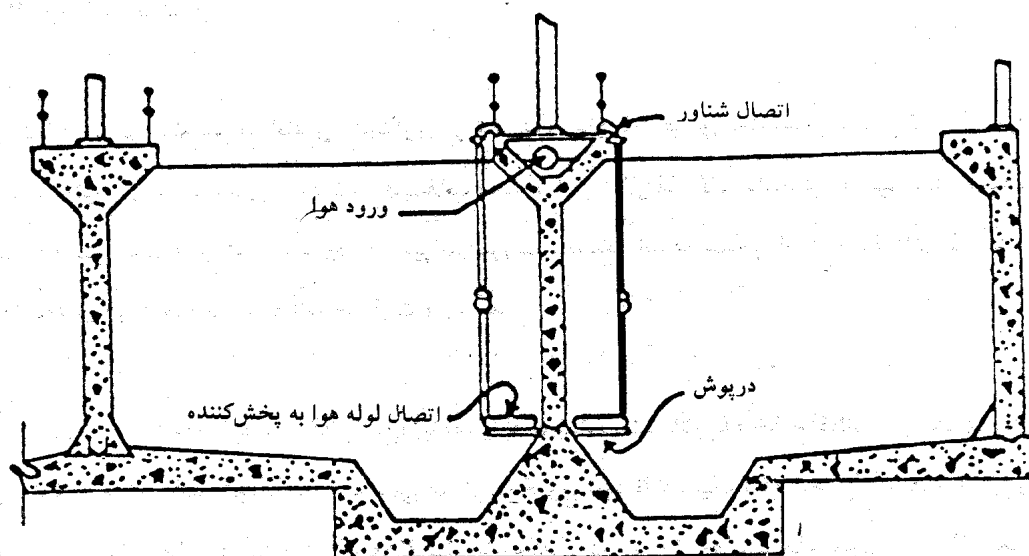
شکل ۳- مقطع حوض دانه گیر به روش هوادهی
