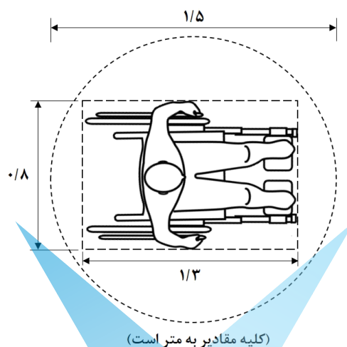
شکل ۲-۱- ابعاد صندلی‌های چرخ‌دار و فضای لازم برای دور زدن
