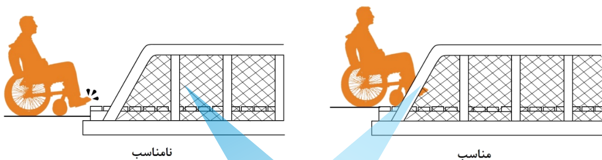
شکل ۵-۱- محل اتصال پیاده‌رو و ورودی پل‌های روگذر عابر پیاده
