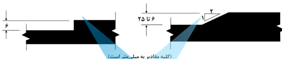
شکل ۹-۲- اختلاف سطح در روسازی پیاده‌رو
