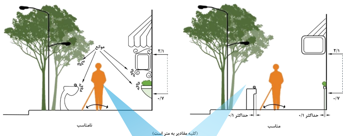
شکل ۲-۶- جانمایی مبلمان شهری در مسیر حرکت عابران پیاده
