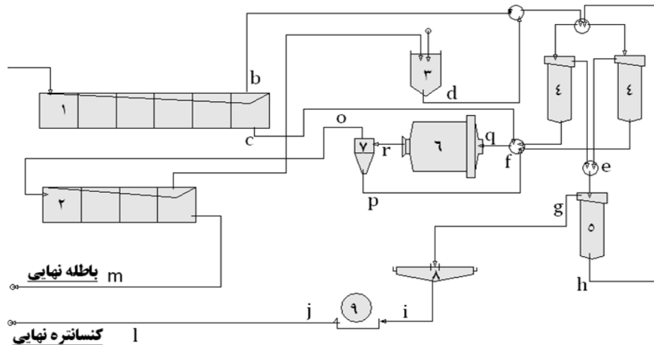
نام قسمتهای مختلف واحد فلوتاسیون و فیلترینگ
