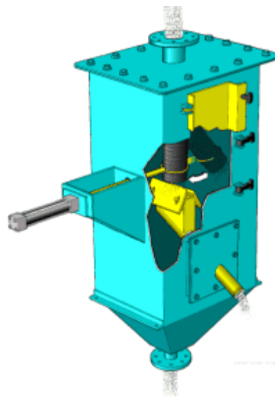
۴۵- برش دهنده یکپارچه (iceTM)
