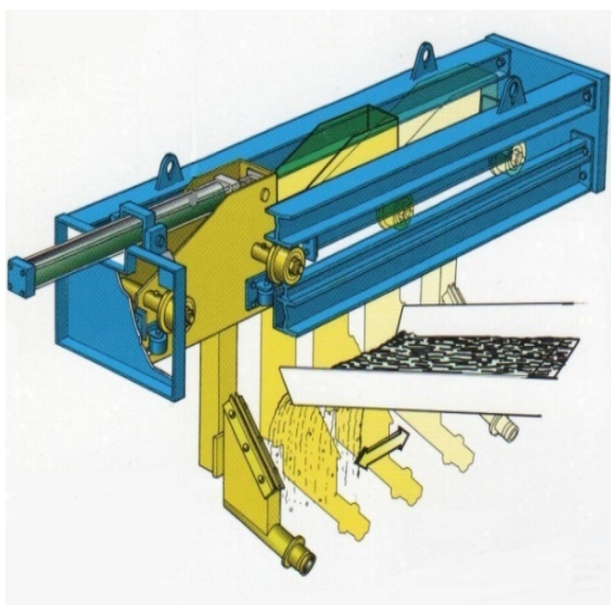
۴۶- نمونه‌گیر خطی مدل ۱۳۵۰ برای کارهای فوق‌العاده سنگین
