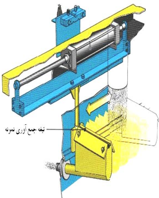
۴۴- نمونه‌گیر خطی مدل General duty 1100
