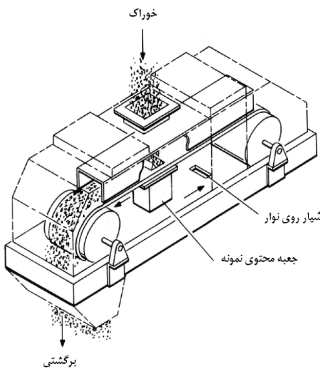
۱۸- نمونه‌گیر خطی با نوار شکاف‌دار
