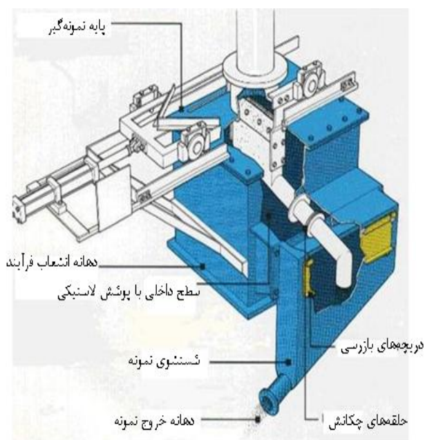
۴۸- نمونه گیر خطی با محفظه یکپارچه کاتر مدل ۱۵۰۰
