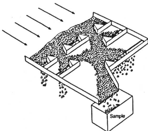
۱۴- نمونه‌گیر ثابت صفحه‌ای
