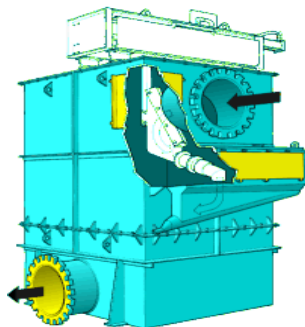
۴۹- نمونه گیر خطی برشی با محفظه (ICE) مدل ۱۳۵۰
