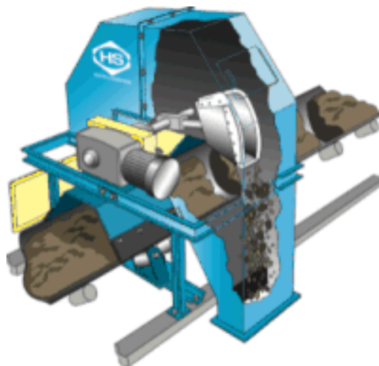
۳۱- نمونه گیرهای چرخشی - مدل ۴۵۰۰ با تقسیم کننده پیوسته نمونه
