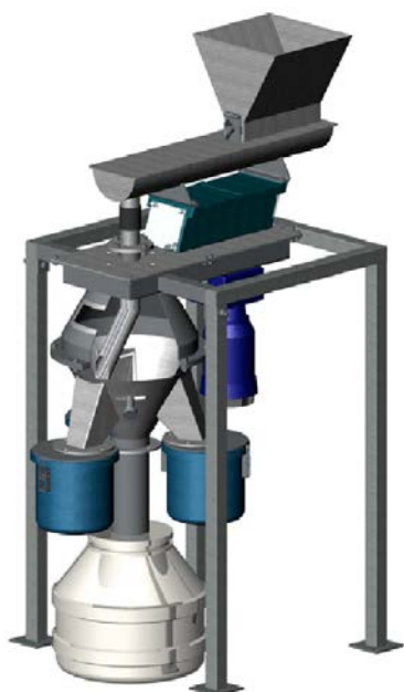
۸- نمونه‌گیر شکاف چرخشی
