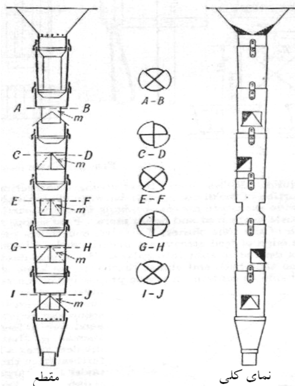
۱۱- مقطع لوله نمونه‌برداری
