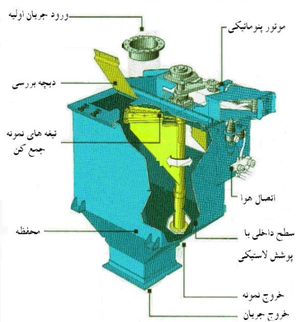
۵۰- نمونه گیرهای قوسی سری متناوب - مدل ۳۰۰۰
