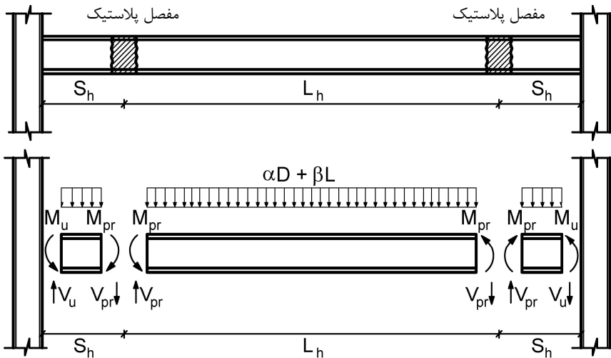
شکل ۱-۸-۳-۱۰ نمودار پیکره آزاد تیرهای باربر جانبی
