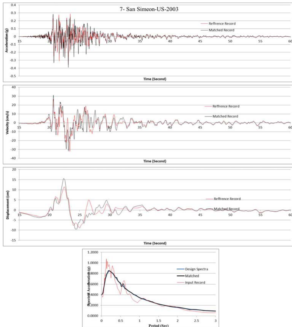
شکل ۴-۲۶- مقایسه رکورد انتخابی و تطبیق یافته با طیف طراحی در حوزه شتاب، سرعت و تغییر مکان برای رکورد San Simeon-
