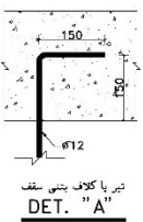
جزئیات اتصال به تیر یا کلاف بتنی S.C.: 1/10
