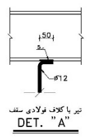
جزئیات اتصال به تیر یا کلاف فولادی S.C.: 1/10
