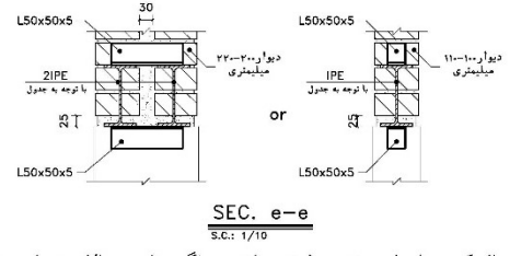
جزئیات اتصال به تیر یا کلاف بتنی S.C.: 1/10
