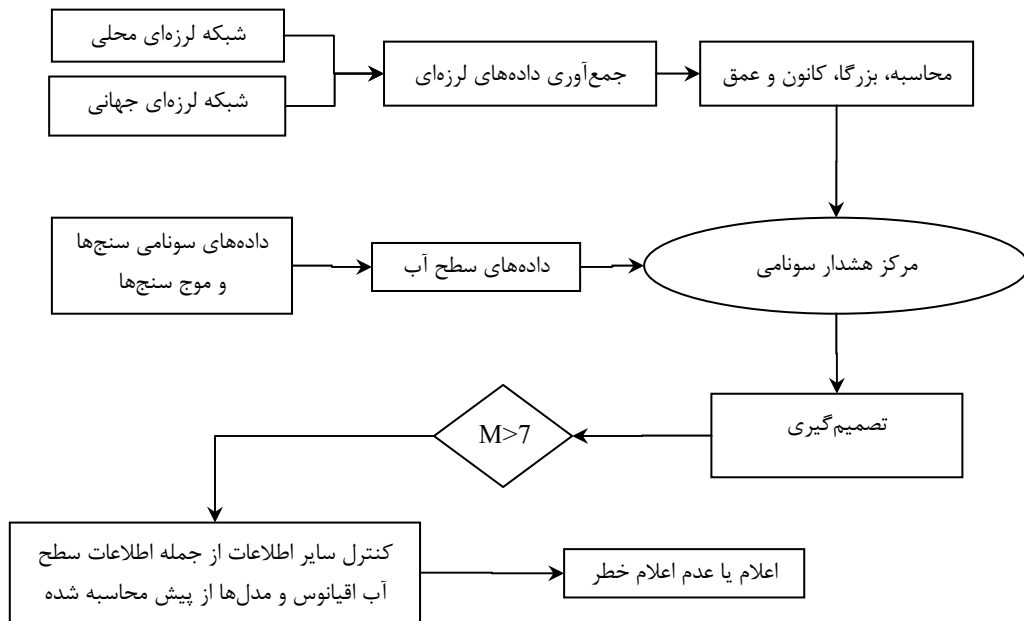
شکل ۴-۳- ساختار سامانه هشدار سونامی پیشنهادی برای سواحل سونامی خیز جنوب ایران
