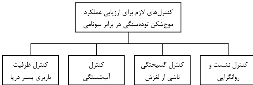
شکل ۳-۸- کنترل های لازم برای ارزیابی عملکرد موج شکن توده سنگی در برابر سونامی
