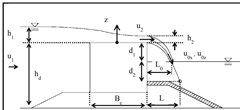
شکل ۳-۱۷- پارامترهای استفاده شده در تعیین نقطه سرریز جریان سونامی
