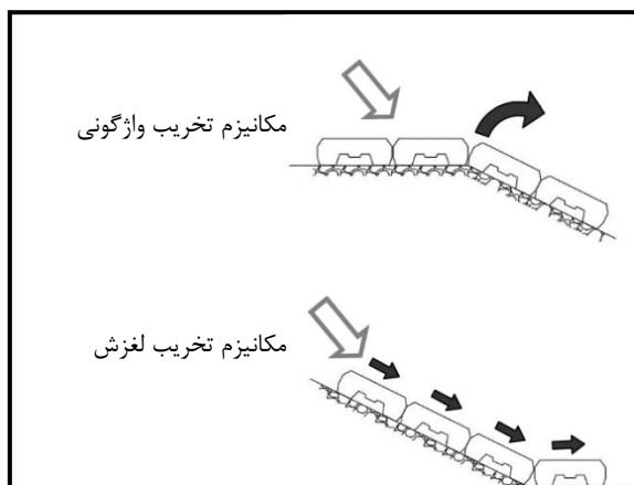
شکل ۳-۱۲- مکانیزم‌های تخریب آرمورهای مستقر بر روی بخش تقویت شده
