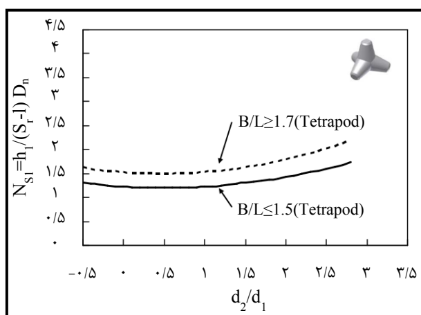
شکل ۳-۱۶- نمودار N_{S1} برحسب \frac{d_2}{d_1} برای آرمور بتنی Tetrapod
