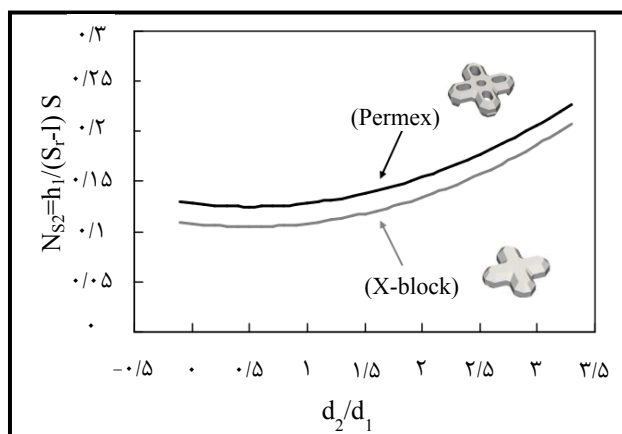
شکل ۳-۱۵- نمودار N_{S2} برحسب \frac{d_2}{d_1} برای آرمورهای بتنی Permex و X-block
