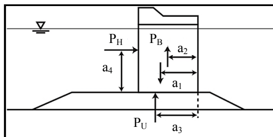
شکل ۳-۹- پارامترهای موثر در کنترل واژگونی
