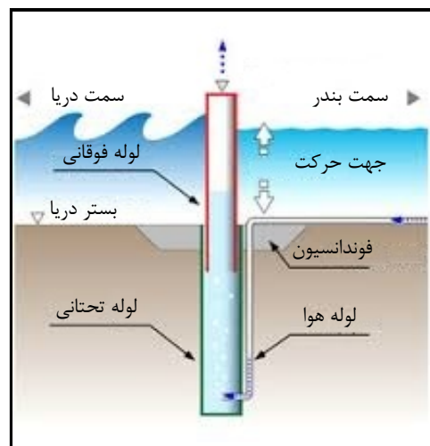
شکل ۴-۱- موج‌شکن تلسکوپی قائم
