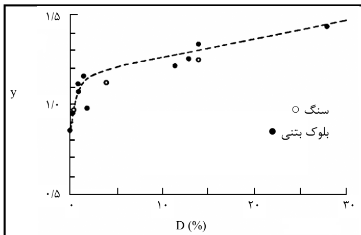
شکل ۳-۱- تغییر پارامتر متاثر از نوع تخریب قطعات سنگی (y) بر اساس نرخ تخریب آرمورها (D)
