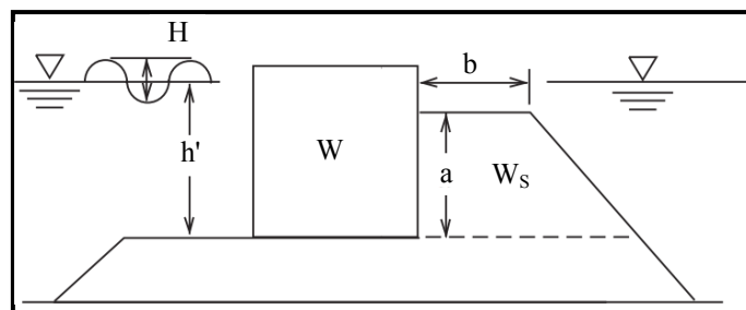
شکل ۳-۱۰- سطح مقاوم در برابر لغزش بخش تقویت شده
