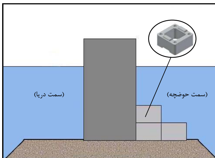
شکل ۳-۱۸- شکل شماتیک بلوک‌های SPF جهت پایداری در برابر لغزش
