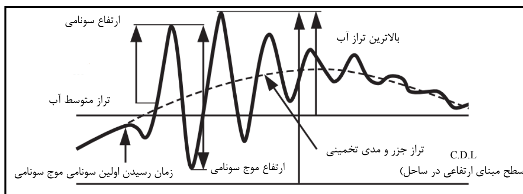
شکل ۱-۱- توصیف واژگان مربوط به سونامی در یک سری زمانی ثبت شده نوسانات سطح آب
