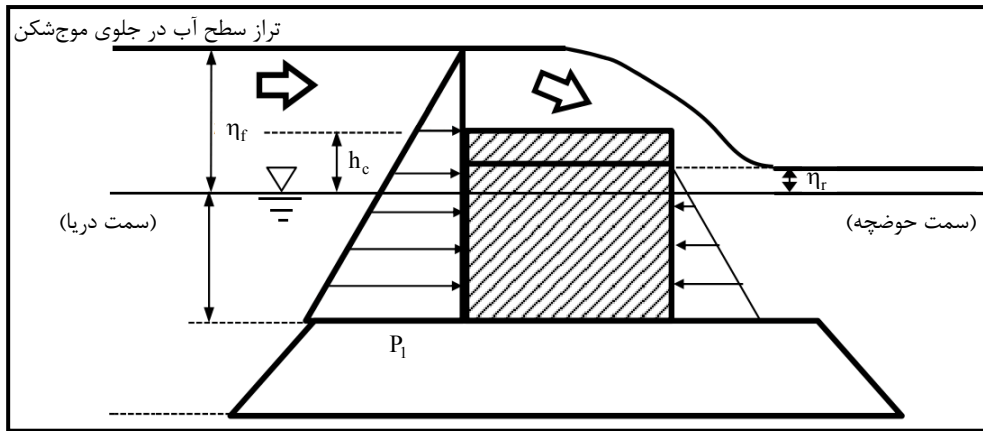
شکل ۳-۶- توزیع نیروی موج سونامی طرح در حالت سرریزی موج سونامی از روی موج شکن مرکب
