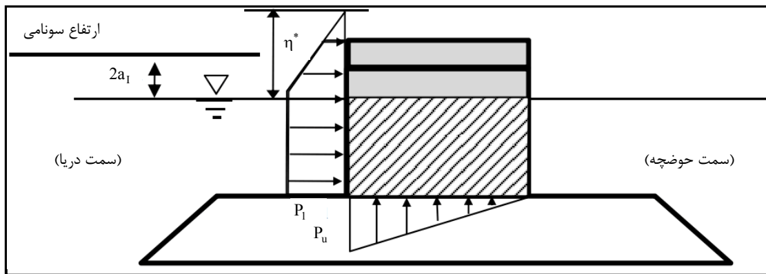
شکل ۳-۴- توزیع نیروی موج سونامی طرح در حالت تراز یکسان سطح آب در طرفین موج شکن مرکب بر مبنای روابط تانی موتو
