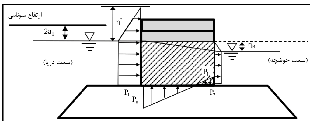
شکل ۳-۵- توزیع نیروی موج سونامی طرح در حالت تراز متفاوت سطح آب در طرفین موج‌شکن مرکب بر مبنای روابط تانی‌موتو
