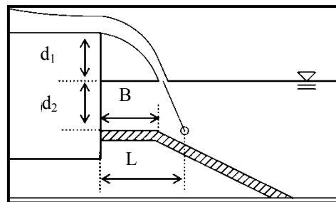
شکل ۳-۱۳- پارامترهای استفاده شده در تحلیل پایداری آرمورهای تقویتی
