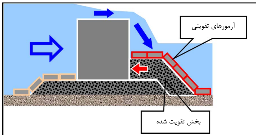
شکل ۳-۱۱- شکل شماتیک بخش تقویتی و بلوک‌های مستقر روی آن
