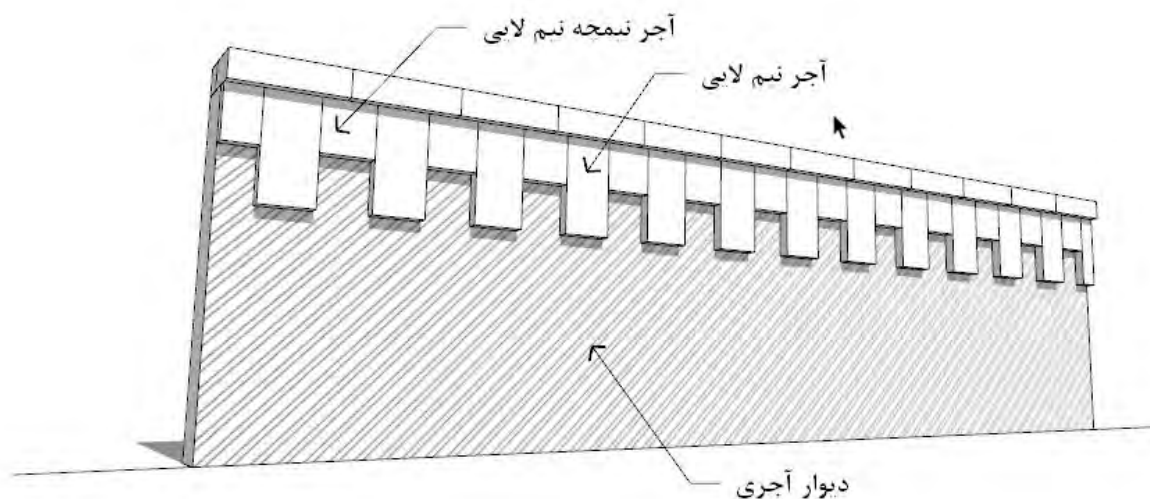
شکل ۱: نمونه دندان موشی در نمای آجری
