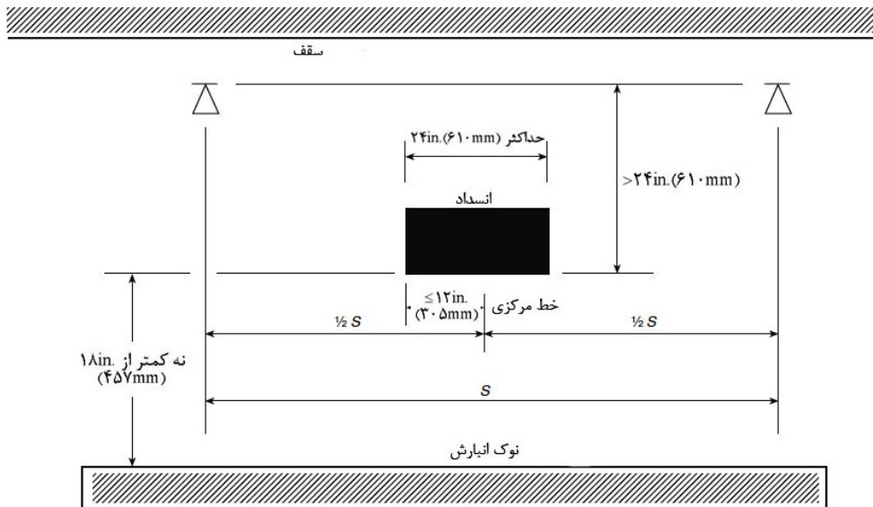
شکل ۸-۱۱-۵-۳ مانع بزرگتر از 24\text{in.} ( 610\text{mm} ) زیر اسپرینکلر (اسپرینکلرهای CMSA)
