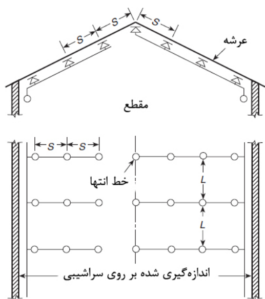
شکل ۸-۳-۱۰-الف- حداکثر فاصله بین اسپرینکلرها با سقف‌های شیب‌دار- چیدمان الف
