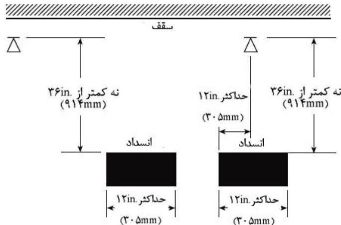
شکل ۸-۱۱-۵-۳ مانع بزرگتر از 36\text{in.} ( 914\text{mm} ) زیر اسپرینکلر (اسپرینکلرهای CMSA)
