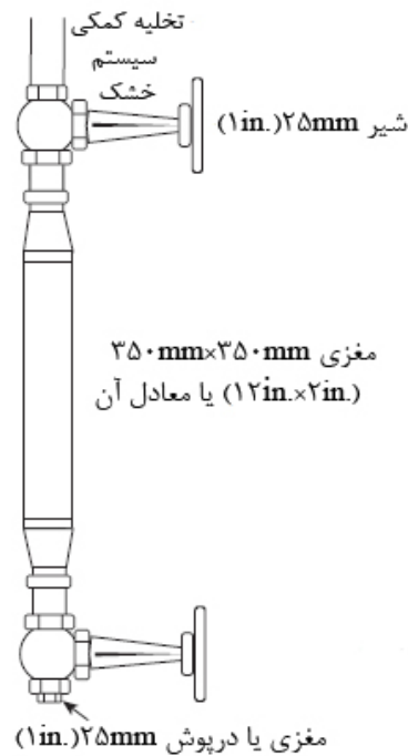
شکل ۵-۳-۵-۲-۱۶-۸- تخلیه کمکی سیستم خشک
