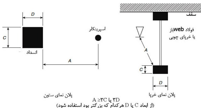
شکل ۸-۱۱-۵-۳-۱ حدافل فاصله از مانع (اسپرینکلرهای CMSA)
