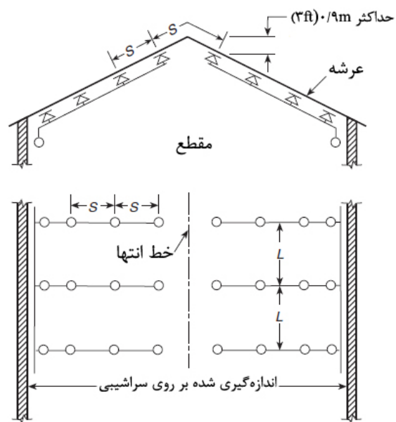
شکل ۸-۳-۱۰-ب- حداکثر فاصله بین اسپرینکلرها با سقف‌های شیب‌دار- چیدمان ب
