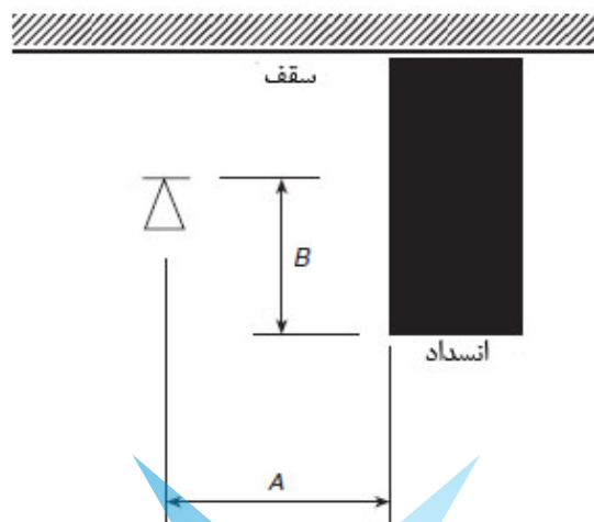
شکل ۸-۱۱-۵-۲-۱-۲ جانمایی اسپرینکلر از موانع برای جلوگیری از تاثیر آن بر تخلیه آب (اسپرینکلرهای CMSA)
