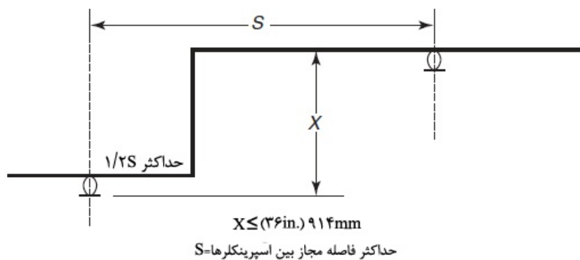
شکل ۸-۶-۴-۱-۳-ب - تغییر عمودی در ارتفاع سقف کمتر یا برابر با 914 \text{ mm (} 36 \text{ in.)}
