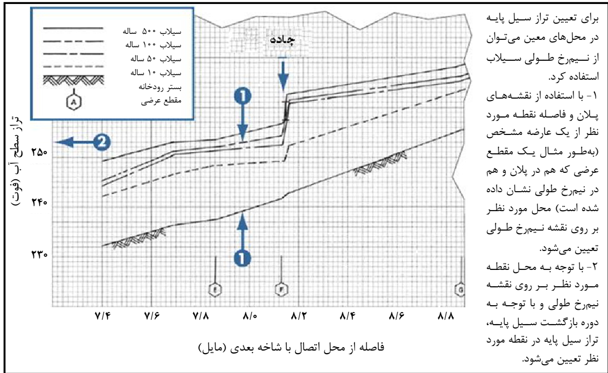
شکل ۴-۵- نیم‌رخ طولی تراز سطح آب برای سیلاب‌های با دوره بازگشت‌های مختلف [۱۲۳]
