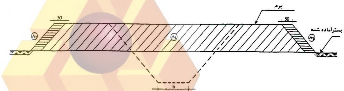
شکل ۴۰-۲. شمای مقطع خاکریزی
