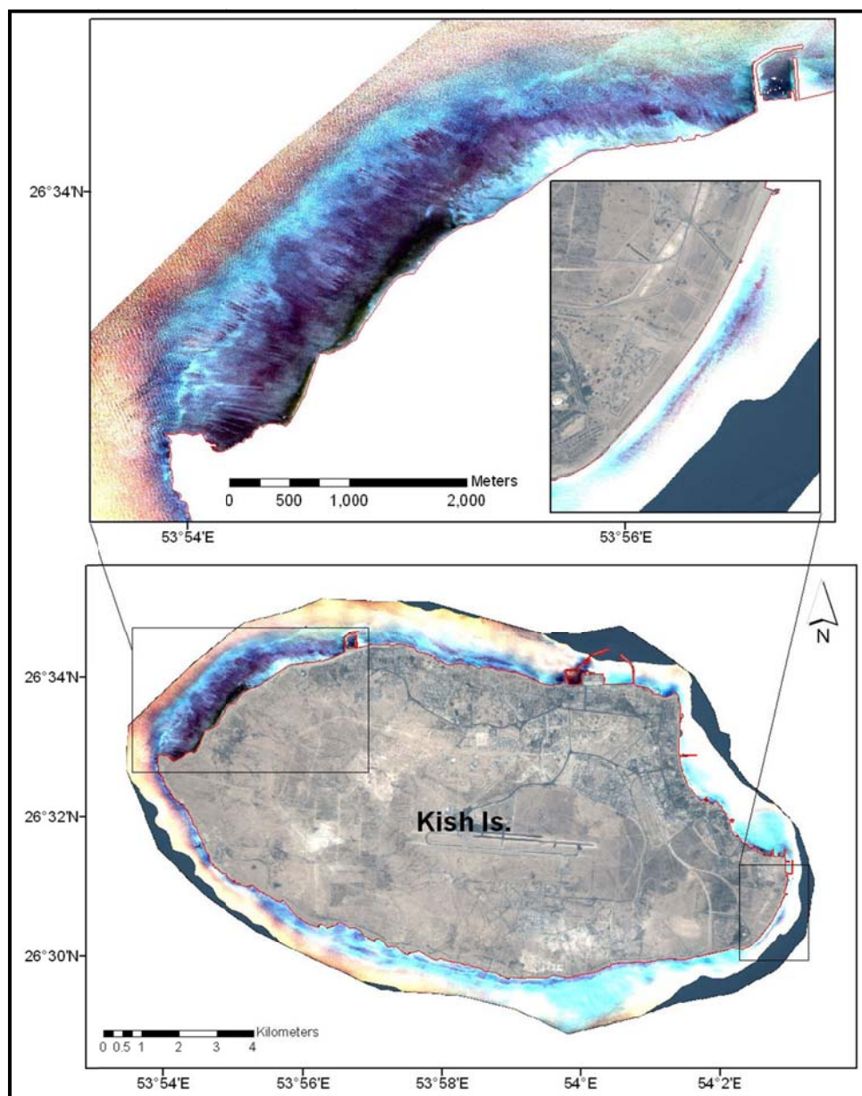
شکل ۳-۲۴- تأثیر تصحیح انعکاس ثبت شده در سنجنده ماهواره با استفاده از محاسبه ضرایب میرایی نور در هر باند تصویربرداری و به‌کارگیری آن در فرمول ۲ برای محاسبه انعکاس بستر در بارز شدن عوارض بستر
