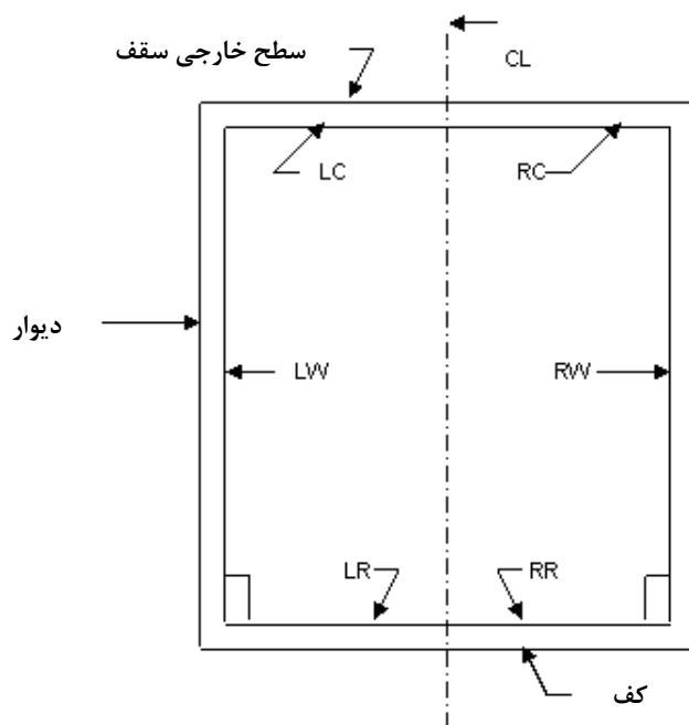
شکل ۴-۱- نام‌گذاری سطوح و حدود حفاریات با مقطع مستطیلی
