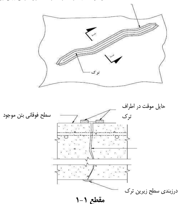
شکل ۱-۵- جزییات تعمیر ترک واقع در سطح افقی
