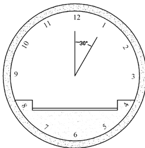
شکل ۴-۲- نام‌گذاری سطوح و حدود حفاریات با مقطع دایروی
