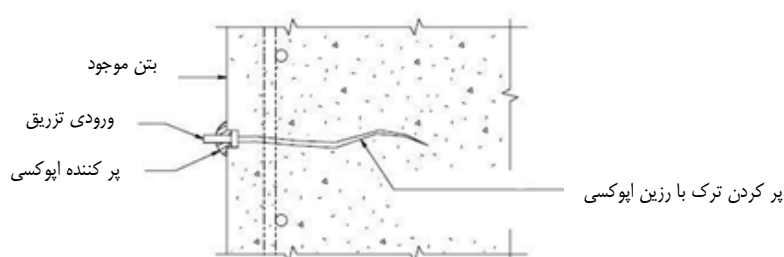
شکل ۵-۲- جزئیات تعمیر ترک قائم/ بالاسری
