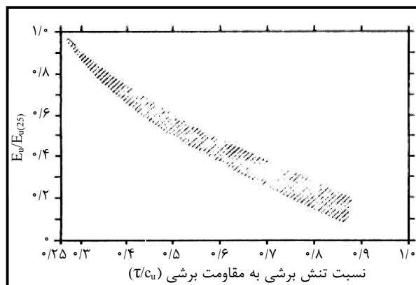
شکل ۹-۶ - کاهش مدول یانگ زهکشی نشده در رس‌های به طور عادی تحکیم یافته،
