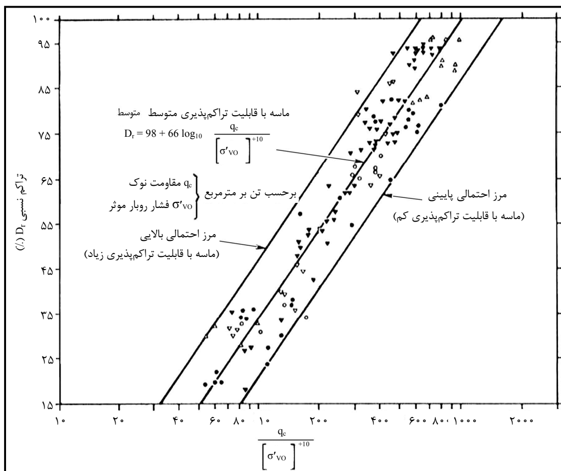
شکل ۳-۶- رابطه میان q_c و D_r برای ماسه عادی تحکیم یافته کوارتزی (دارای منشای کوارتزی) [۳]
