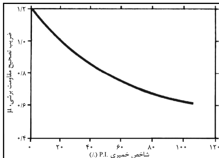
شکل ۶-۶- ضریب تصحیح مقاومت برشی از آزمایش برش پره‌ای [۳]
