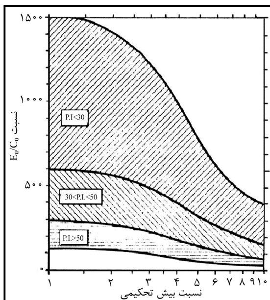
شکل ۸-۶ - نسبت مدول یانگ زهکشی نشده به مقاومت برشی، بر حسب نسبت بیش تحکیمی در رس‌ها [۳]
