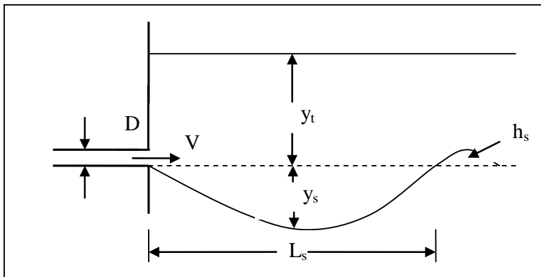
شکل ۸-۱- نمای کلی از یک جت مستغرق افقی
