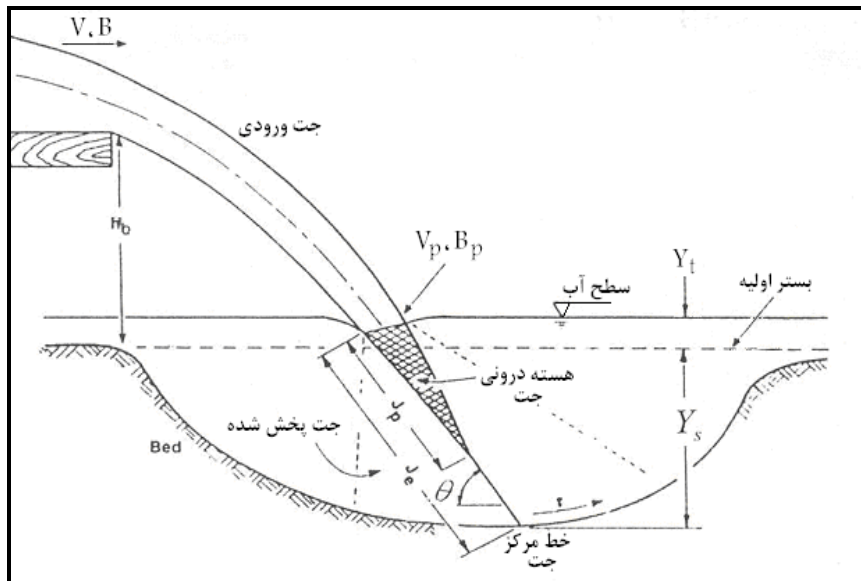
شکل ۷-۴- شکل و خصوصیات یک جت ریزشی مایل [۳۷]
