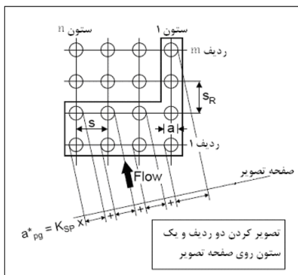
شکل ۴-۸- عرض تصویر شده شمع‌ها برای حالت کلی [۷۴]
