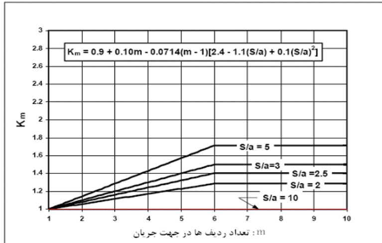
شکل ۴-۱۰- ضریب ردیف‌های هم راستا برای حالت خاص [۷۴]
