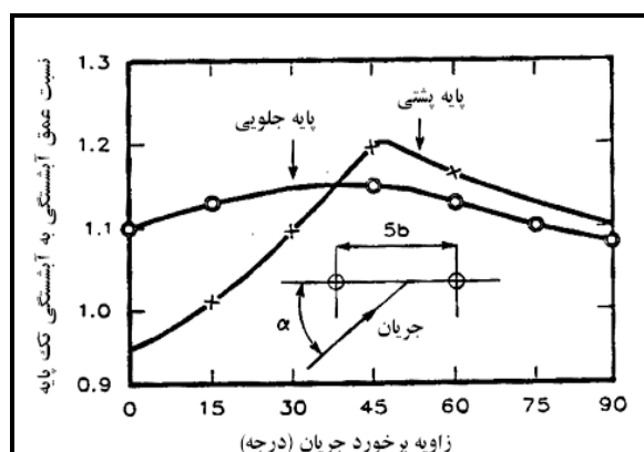
شکل ۴-۱۴- نمودار بین زاویه‌ی برخورد جریان با عمق آبخستگی در دو پایه [۳۵]
