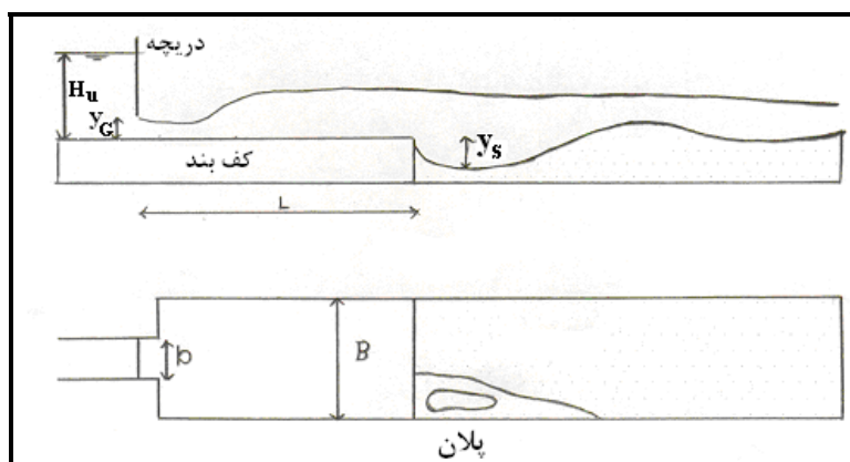
شکل ۷-۹- آبشستگی در پایین دست حوضچه آرامش با باز شدگی ناگهانی [۵۵]
