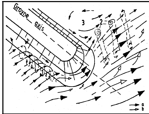
شکل ۵-۲- الگوی جریان اطراف یک آبشکن [۲۹]
