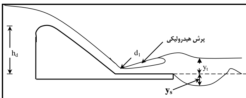
شکل ۹-۶- نمای آزمایشات فرهودی و اسمیت (۱۹۸۵-۱۹۸۲)
