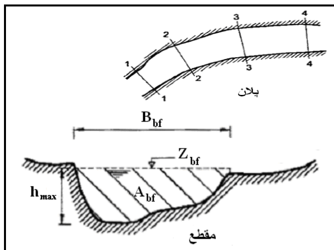
شکل ۳-۱- تعاریف شکل و هندسه مقطع رودخانه [۴۸]
