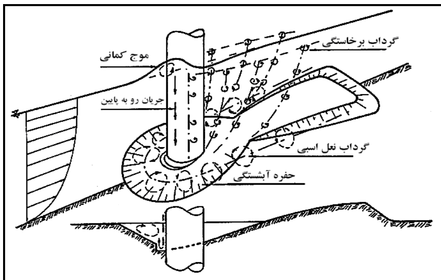
شکل ۴-۱- الگوی جریان در اطراف یک پایه استوانه‌ای [۱۶]
