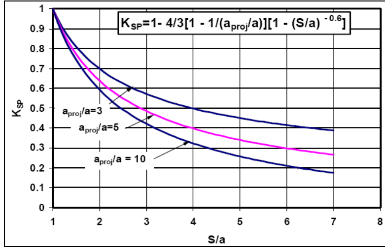
شکل ۴-۹- ضریب فاصله شمع‌ها [۷۴]
