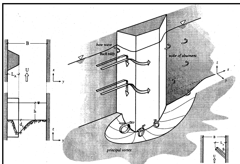
شکل ۵-۳- الگوی جریان در اطراف تکیه‌گاه [۱۳]
