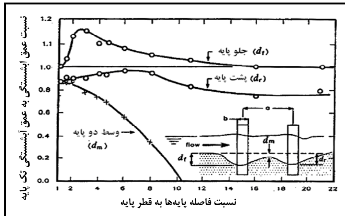
شکل ۴-۱۲- نمودار بین تغییر میزان آبشستگی و فاصله‌ی نسبی دو پایه در حالت در امتداد جریان [۳۵]
