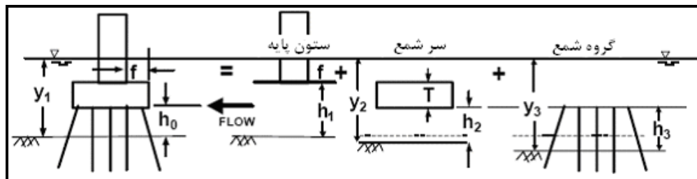
شکل ۴-۵ - اجزای پایه‌های پیچیده [۷۴]
