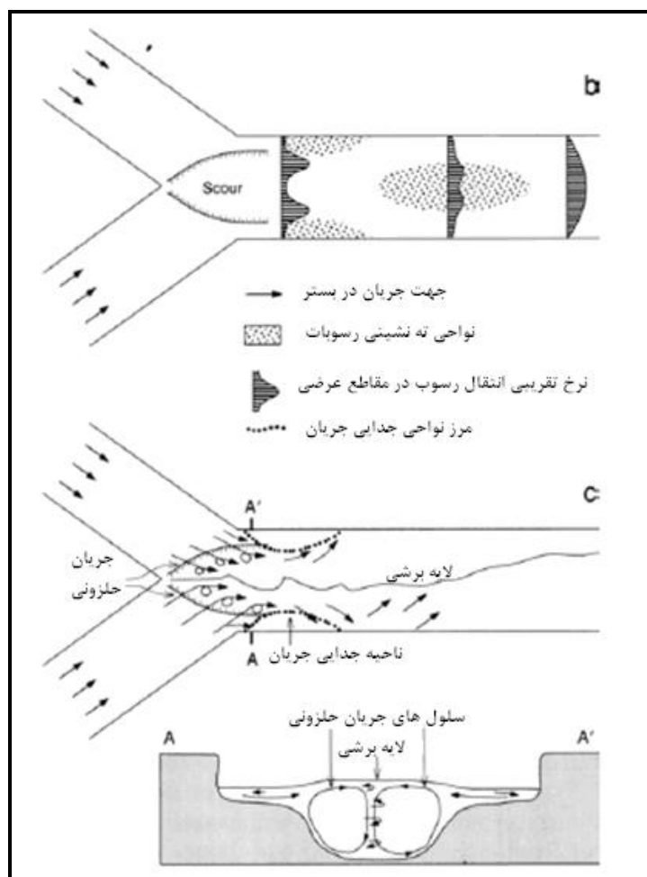
شکل ۱-۷- الگوی جریان، رسوب‌گذاری و فرسایش در تقاطع دو رودخانه
