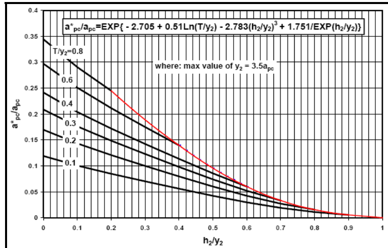
شکل ۴-۷- عرض معادل سر شمع [۷۴]
