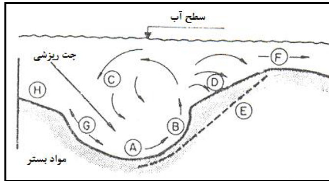
شکل ۷-۳- الگوی جریان جت ریزشی مایل داخل حفره آبشستگی
