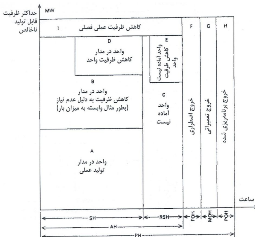
شکل پ ۹-۲: رابطه‌ی بین اصطلاحات زمانی و ظرفیت‌های نیروگاه
