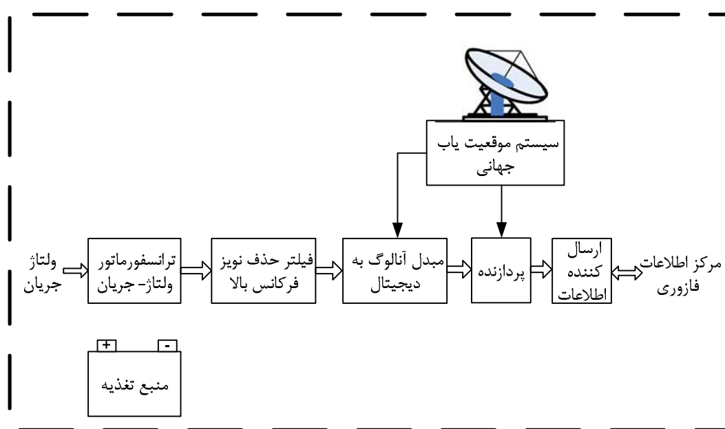
شکل ۵-۳: ساختار یک واحد اندازه‌گیری فازوری نمونه
