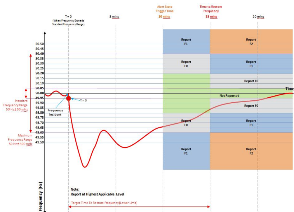
شکل پ ۱۴-۳: نمونه تغییرات فرکانس و نحوه گزارش در سازمان بهره‌برداران سیستم انتقال اروپا [۱۸۶]
